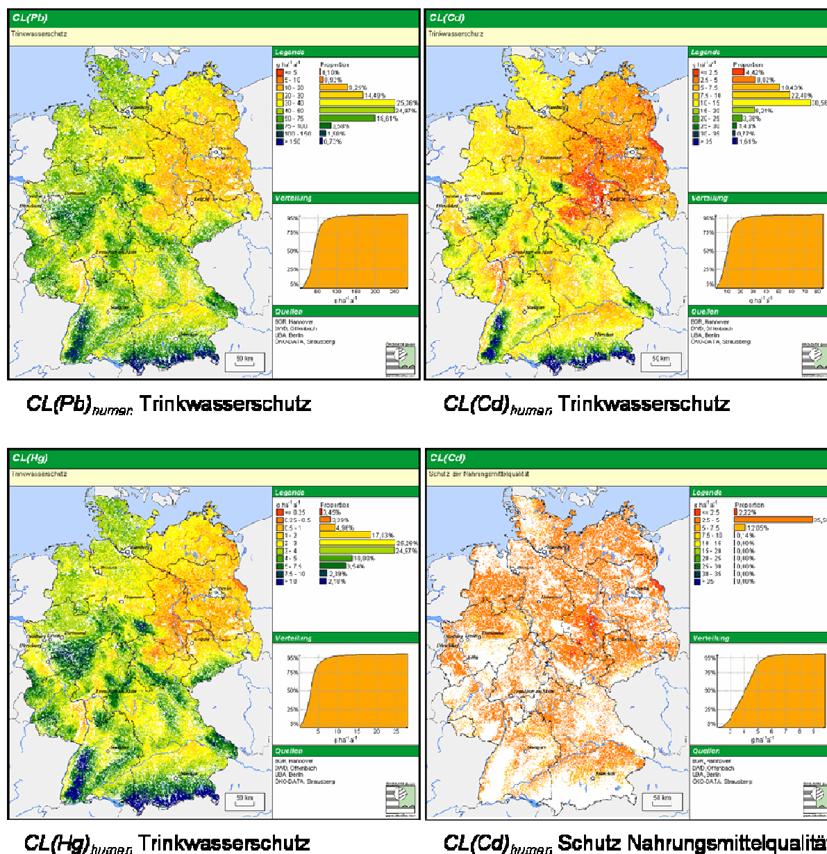
Abbildung Z2.10: Critical Loads zum Schutz der menschlichen Gesundheit ( CL(M)_{human} ) für Pb, Cd und Hg in Deutschland
