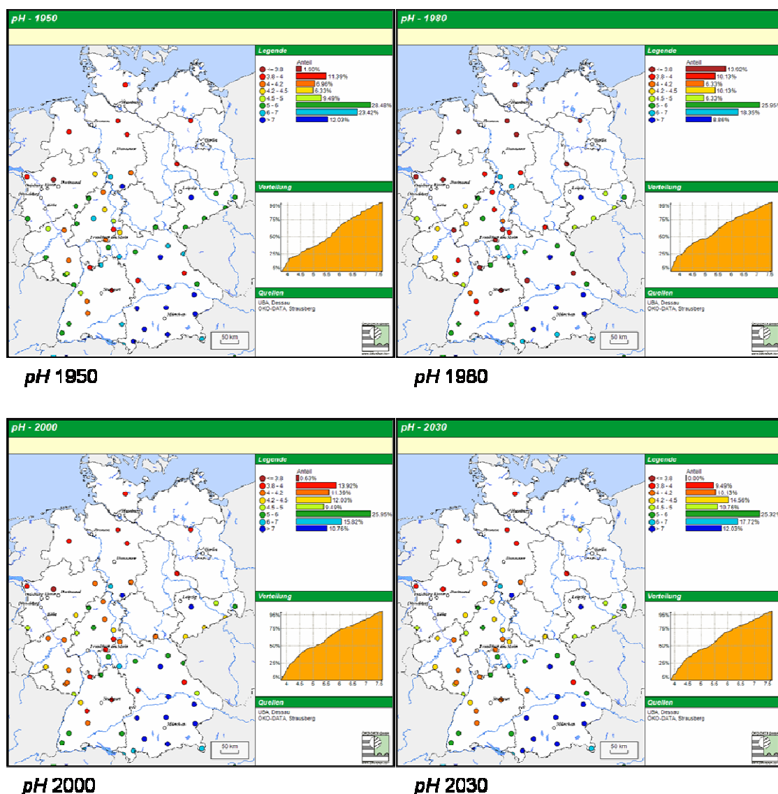
Abbildung Z2.12: pH-Wert an den Level-II-Plots im Ergebnis der VSD-Modellierung 1950, 1980, 2000, 2030
