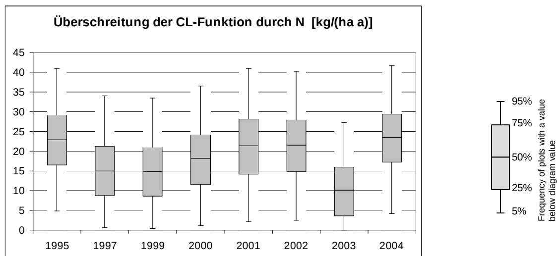
Abbildung Z2.8: Entwicklungstrend bei der Überschreitung der Critical Load Funktion durch Stickstoffeinträge
