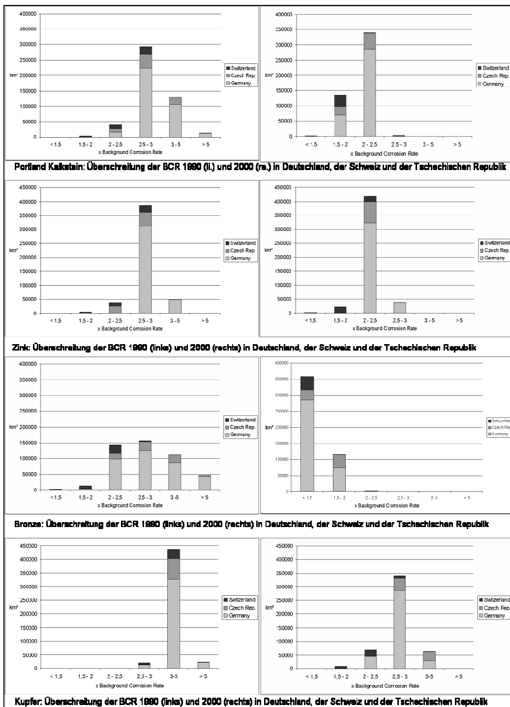
Abbildung Z2.17: Überschreitung der Background Corrosion Rate 1990 und 2000 in Deutschland, der Schweiz und der Tschechischen Republik für Portland Kalkstein, Zink, Bronze und Kupfer
