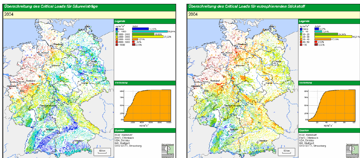
Abbildung Z2.9: Überschreitung der Critical Load Funktion durch Schwefel- (li.) und Stickstoffeinträge (re.) im Jahr 2004
