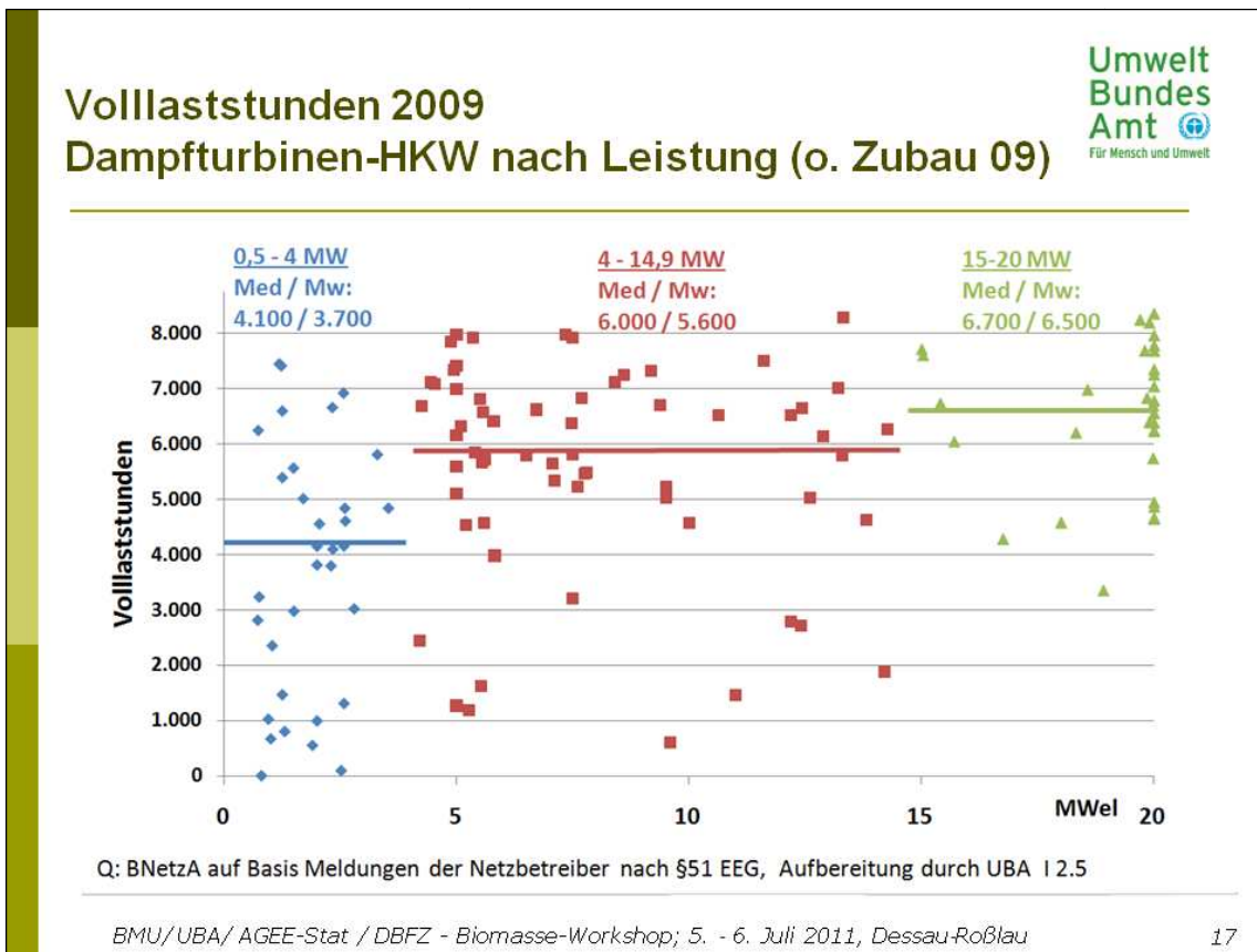
Abbildung 10: Rechnerische Volllaststunden der Biomasseheizkraftwerke mit Dampfturbine nach Leistungsklassen
