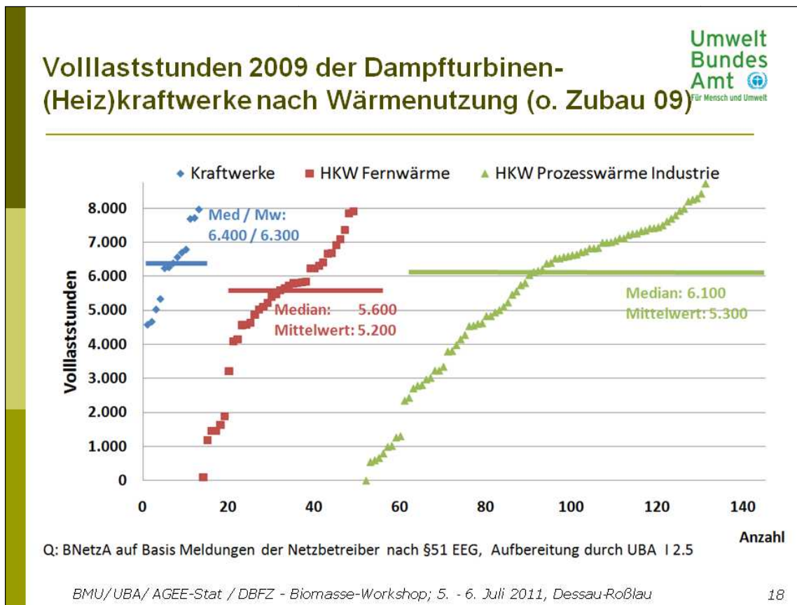
Abbildung 11: Rechnerische Volllaststunden der Biomasseheizkraftwerke mit Dampfturbine nach Wärmenutzung
