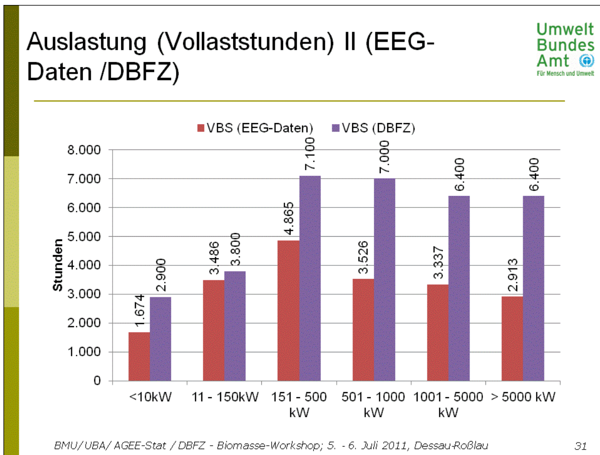
Abbildung 36: Gegenüberstellung der abgeleiteten Volllaststunden EEG-Daten und DBFZ
