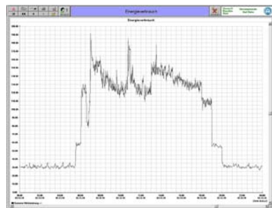
Lastkurve Energieverbrauch in Bad Elster
