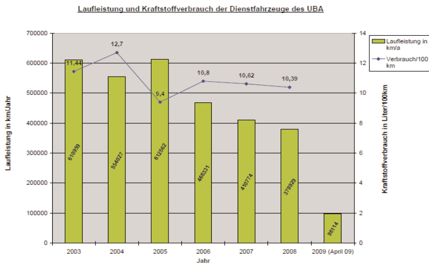
Abbildung 1: Laufleistung und Kraftstoff-verbrauch der Dienstfahrzeuge des UBA
