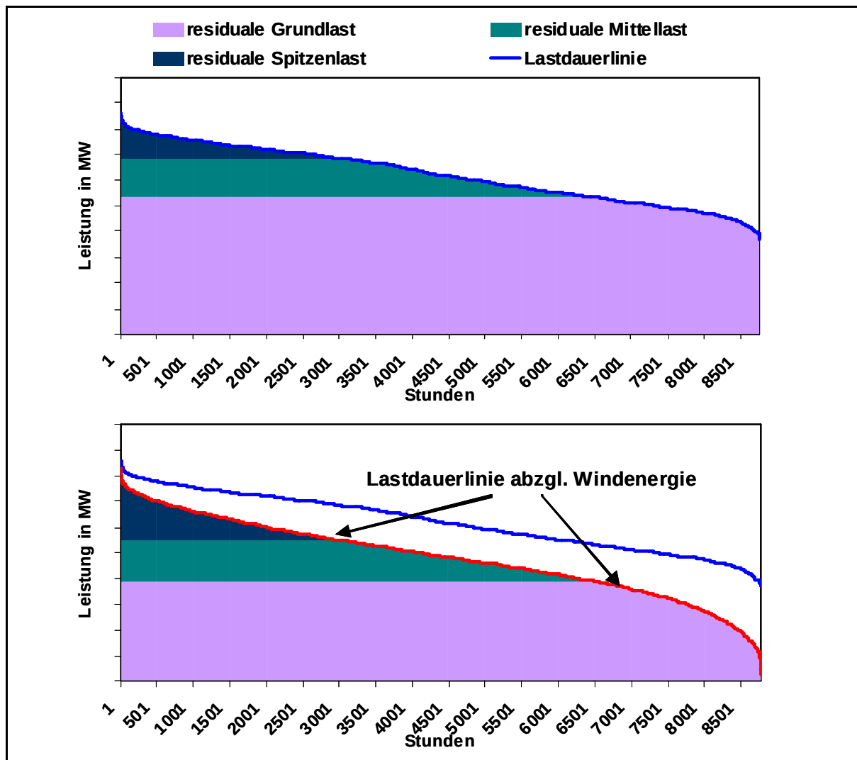
Abbildung 2: Veränderung der Lastdauerlinie durch Windenergieeinspeisung
