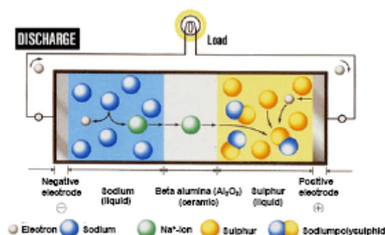
Abbildung 2-7: Funktionsweise einer Natrium-Schwefel-Batterie [Quelle: IERE, o.J.]
