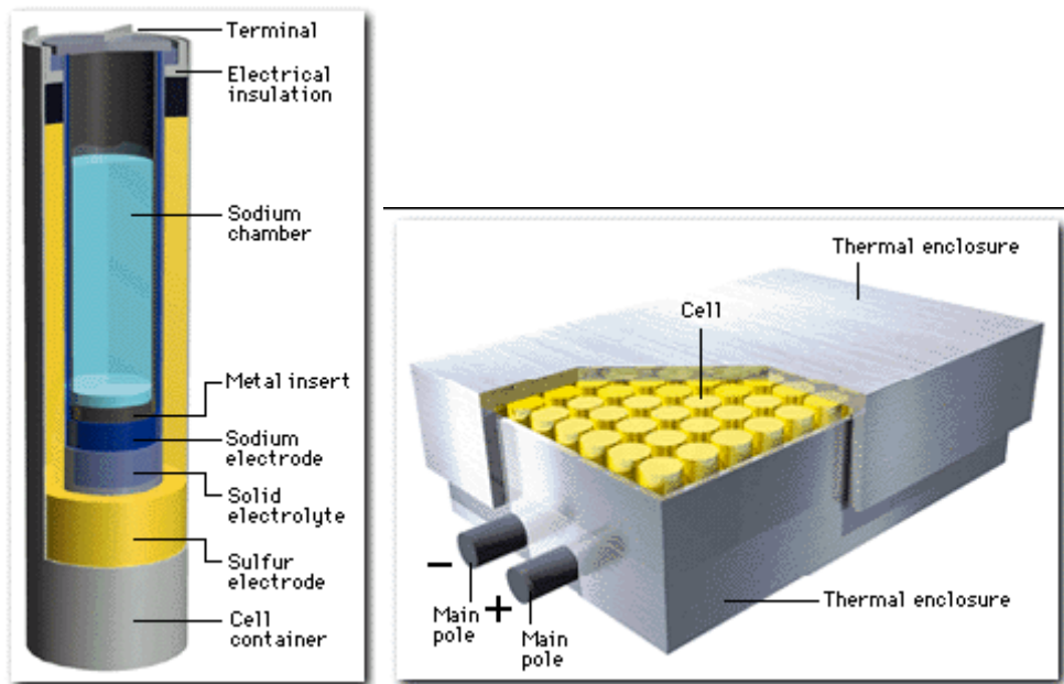
Abbildung 2-8: Natrium-Schwefel-Batterie [Eurosolar, 2006]
