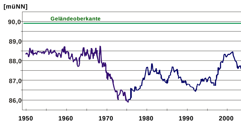
Grundwasserentwicklung im Hessischen Ried (1950-2004)
