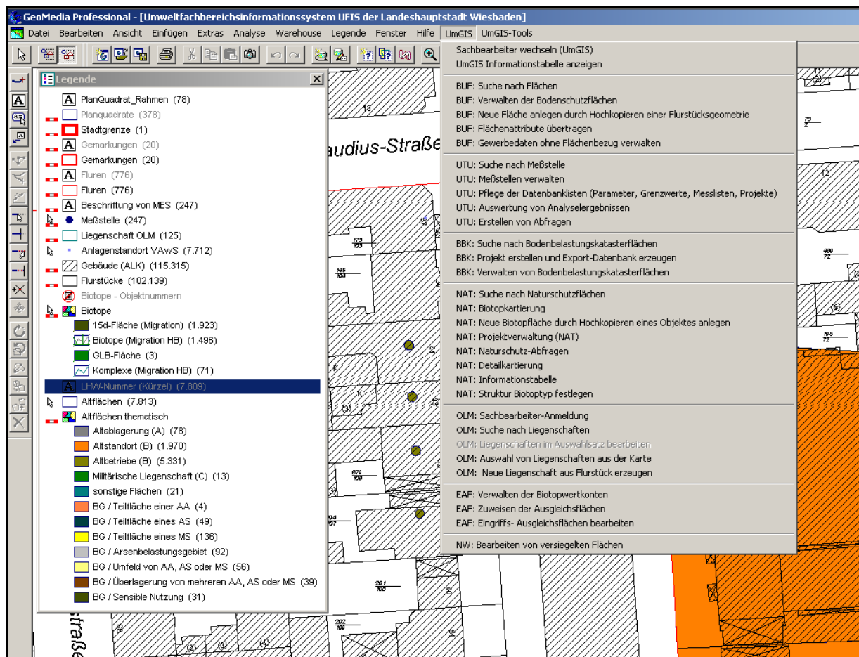
Abbildung 19: UFIS Menueauswahl
