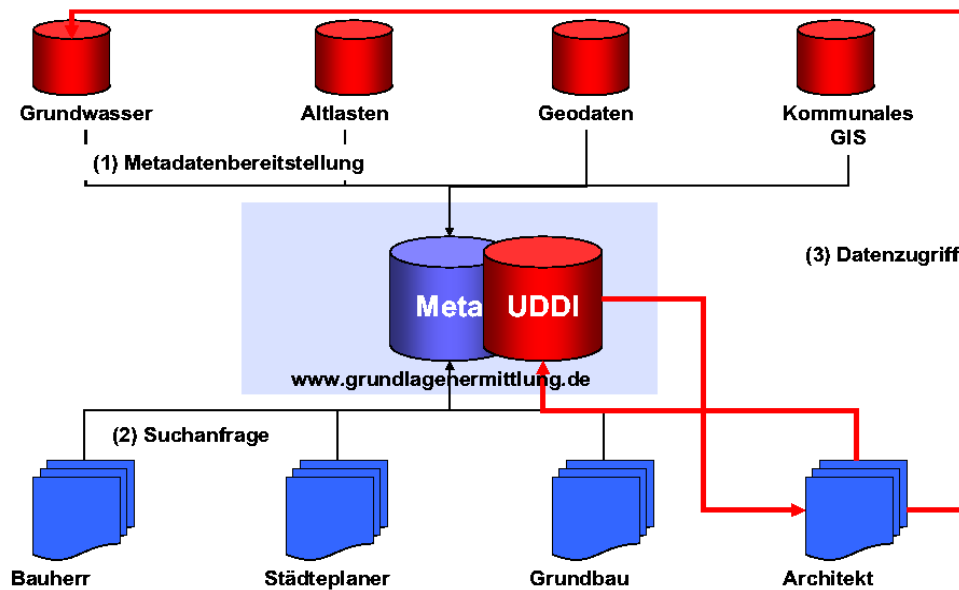
Abbildung 5: Systemarchitektur www.grundlagehermittlung.de
