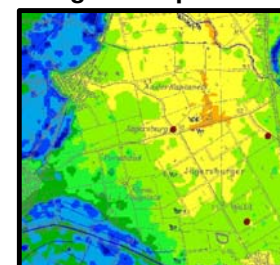
Flurabstandsplan
