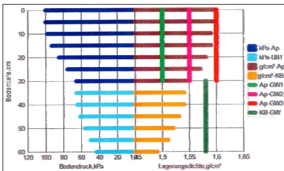
Abbildung 17: Beispiel für ein Bodendruck-Lagerungsdichteprofil für SVGK 3, Kontaktflächendruck = 100 kPa, Radlast = 20 kN, Bodenfeuchte = 90 % nFK, Kontaktfläche = 0,2 m 2 (aus Petelkau et al., 2000) 2 .
