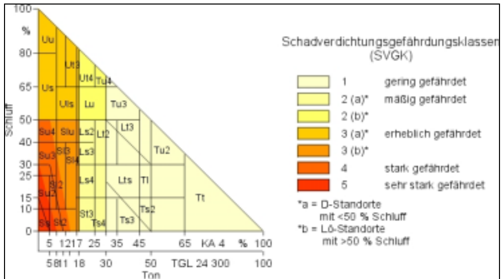
Abbildung 11: Gruppierung der Böden in Schadverdichtungsgefährdungsklassen in Abhängigkeit von der Bodenart (nach Petelkau et al., 2000).
