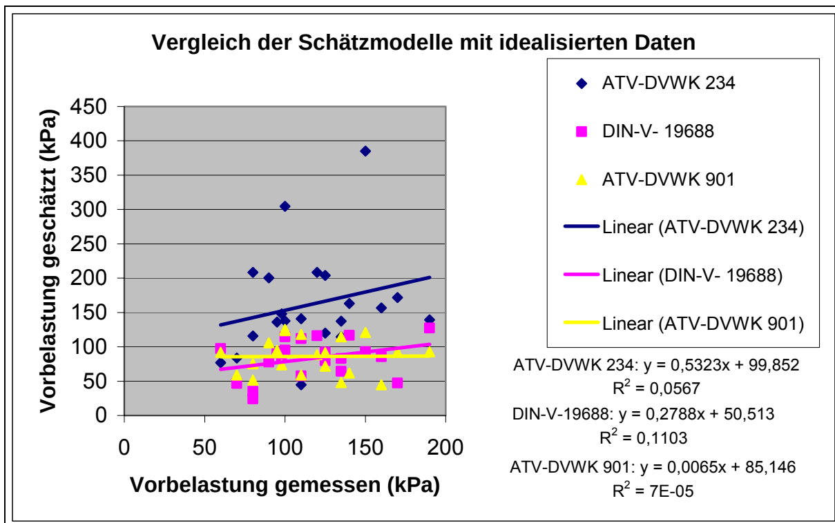
Abbildung 8: Vergleich der Schätzmodelle für die Vorbelastung nur mit idealisierten Variablen.
