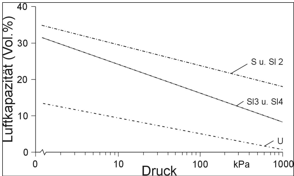
Abbildung 9: Beispiel für ein Nomogramm zur Abnahme der Luftkapazität ungestörter Bodenproben mit steigendem Druck im Ödometertest für den Erstverdichtungsbereich verschiedener Bodenartengruppen bei pF 2,5 (nach Lebert, 1989).
