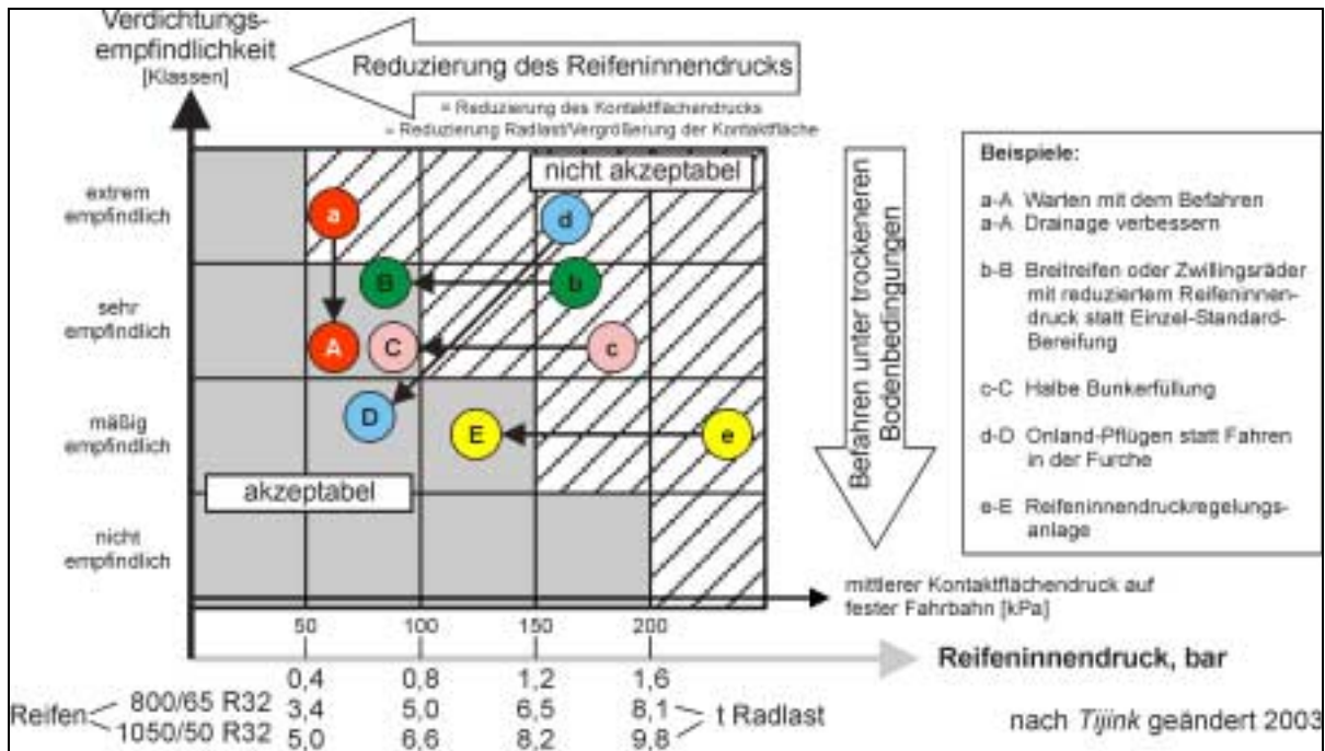
Abbildung 21: Vorschlag für ein Prüfkonzept der mechanischen Belastbarkeit des Bodens in Abhängigkeit von der Verdichtungsempfindlichkeit und dem Reifeninnendruck (Tijink, 2003, geändert).
