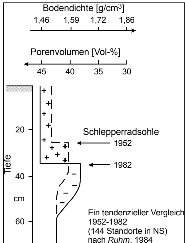
Abbildung 2: Zunahme der Lagerungsdichte und Abnahme des Gesamtporenvolumens von 144 niedersächsischen Ackerstandorten von 1952 bis 1982 (nach Ruhm, 1984) .
