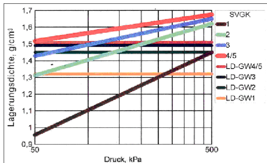
Abbildung 13: Erstverdichtungsgeraden von repräsentativen Bodenarten der Schadverdichtungsgefährdungsklassen (SVGK) unter Berücksichtigung der Lagerungsdichtegrenzwerte (LD-GW) (Bodenfeuchte 50 % nFK, aus Petelkau et al., 2000).
