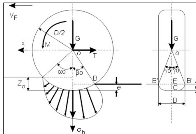
Abbildung 20: Schematische Darstellung der in das Modell nach Jaklinski (1999) eingehenden Parameter der Reifenverformung.
