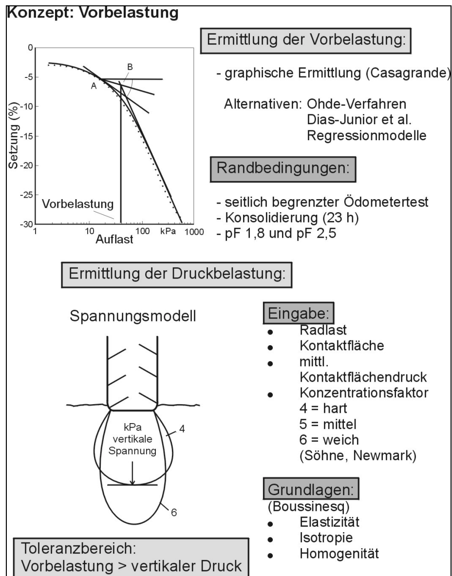
Abbildung 14: Gesamtübersicht der Ermittlung von Druckbelastbarkeit und Druckbelastung des Bodens mit dem Vorbelastungskonzept.
