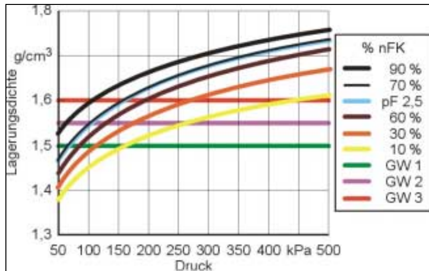
Abbildung 12: Druck-Verdichtungs-Kurven in Abhängigkeit von der Bodenfeuchte (% nFK) für die Bodenart SI3 in der Schadverdichtungsgefährdungsklasse 3 (GW 1–3 = Lagerungsdichtegrenzwert gestaffelt nach Stärke der Ertragseinbußen, aus Petelkau et al., 2000).
