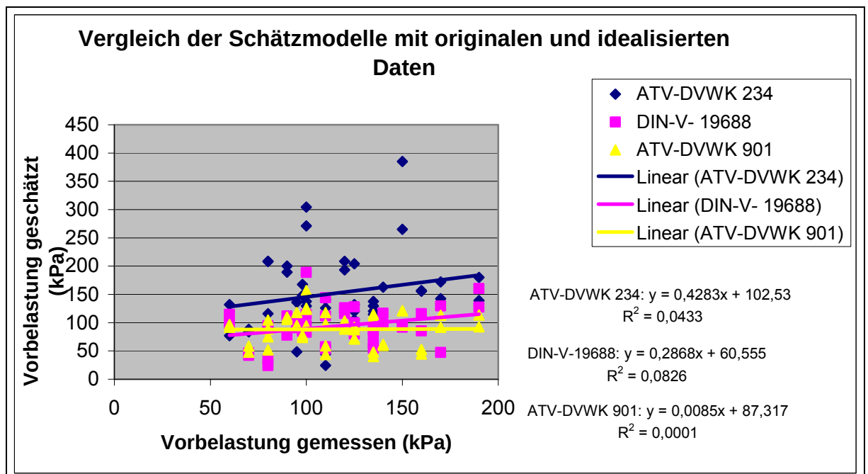
Abbildung 7: Vergleich der Schätzmodelle für die Vorbelastung mit originalen und idealisierten Variablen.
