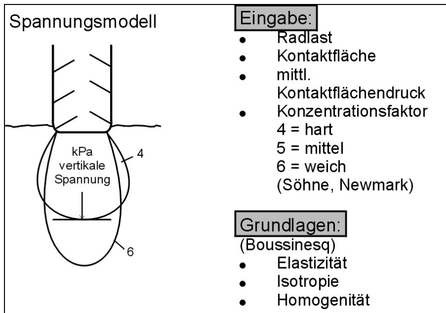
Abbildung 4: Spannungsmodell zur Berechnung des vertikalen Bodendruckes unter Annahme einer elliptischen (Söhne) oder kreisrunden Kontaktfläche (Newmark) auf der Grundlage der Theorien nach Boussinesq und Fröhlich.
