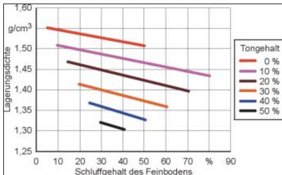
Abbildung 10: Obere Grenzwerte des optimalen Lagerungsdichtebereiches von Ap-Horizonten in Abhängigkeit von der Bodenart bei optimaler Humusversorgung (aus Petelkau et al., 2000).
