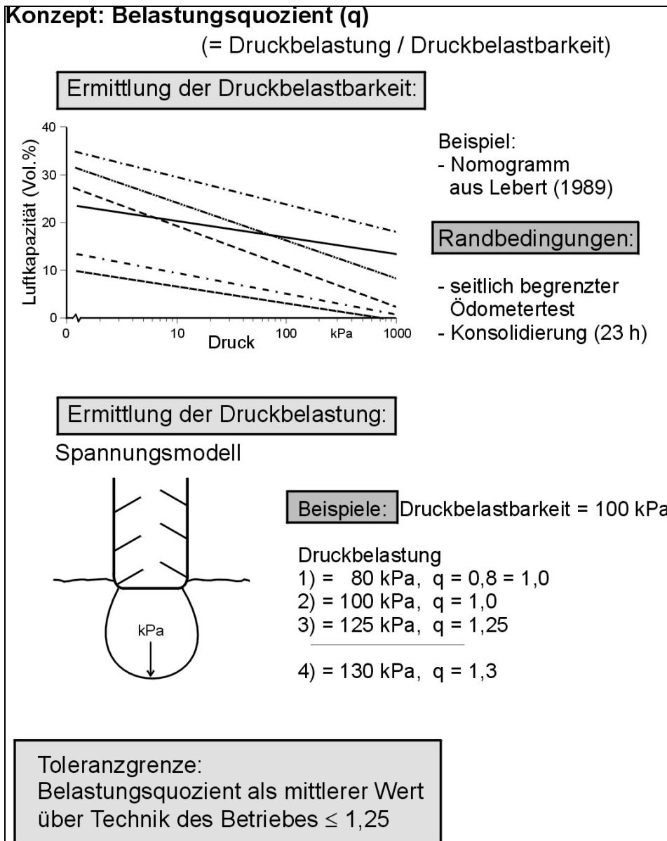
Abbildung 16: Gesamtübersicht zur Ermittlung des Belastungsquotienten.
