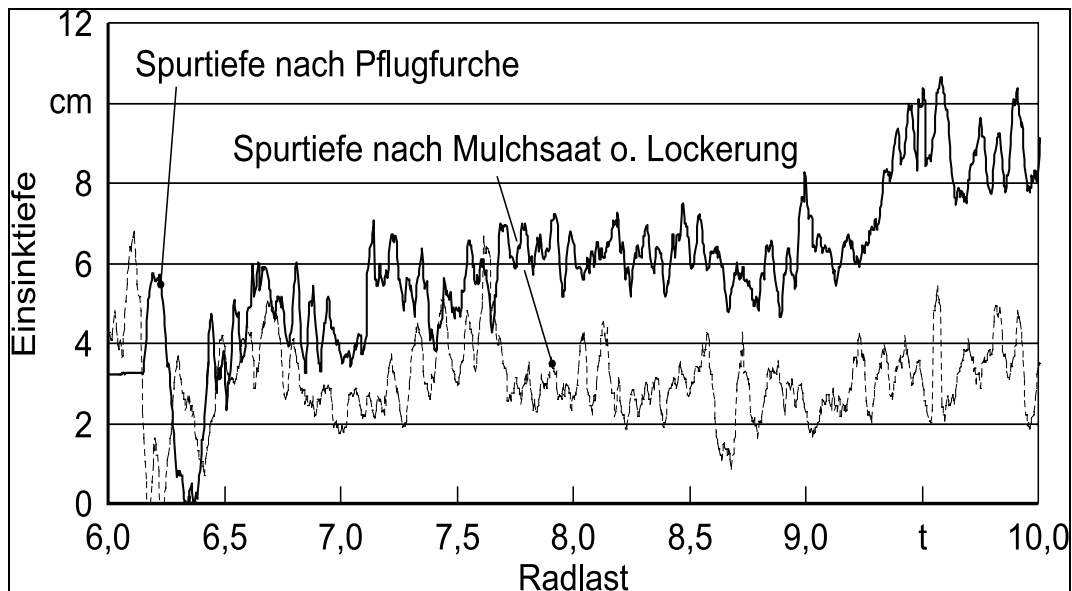
Abbildung 18: Spurtiefe eines 6-reihigen Köpfrödebunkers (Maximale Radlast: 10 t) in Abhängigkeit von der Bunkerfüllung für zwei Bodenbearbeitungsverfahren (nach Brunotte et al., 2000).
