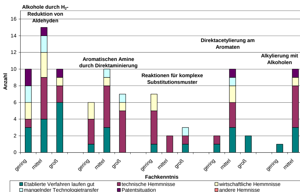
Abbildung 8.2-6b: Von den Experten genannte Hemmnisse des Einsatz neuer Katalysatoren bei den speziellen Reaktionstypen der Fragen 17-21
