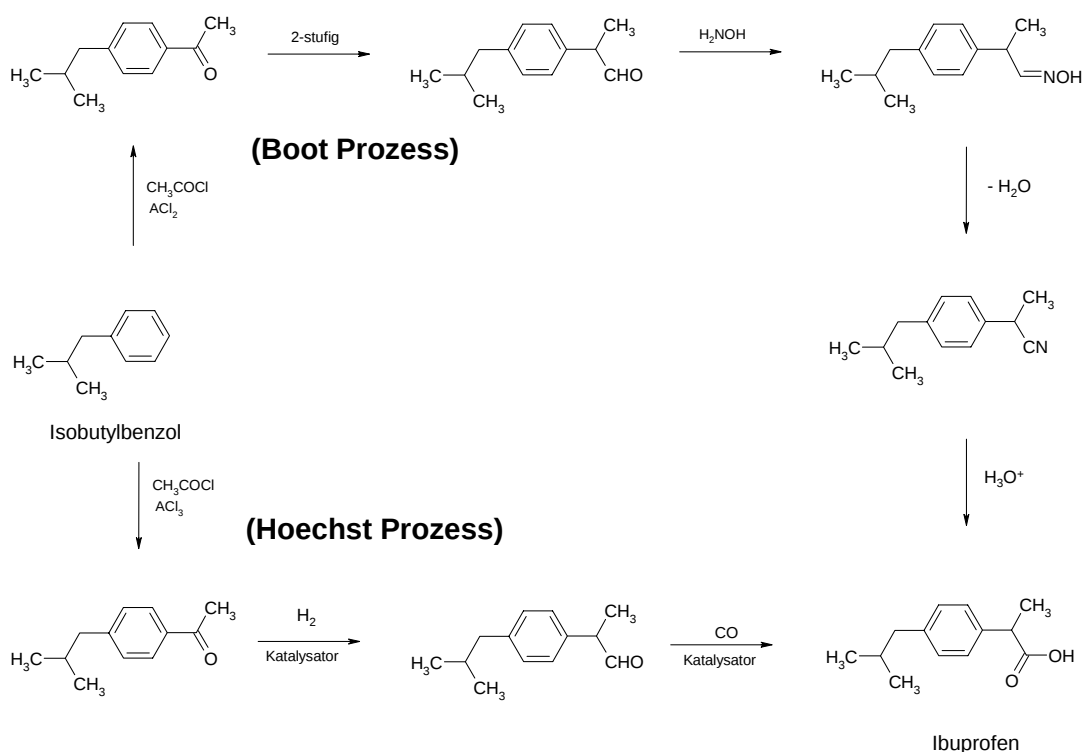
Abbildung 7.1-9: Klassische und verbesserte Syntheseroute für Ibuprofen
