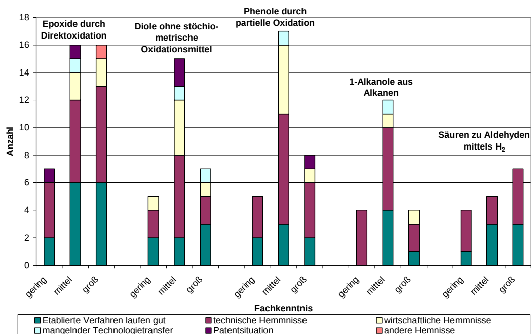
Abbildung 8.2-6a: Von den Experten genannte Hemmnisse für den Einsatz neuer Katalysatoren bei den speziellen Reaktionstypen der Fragen 12-16
