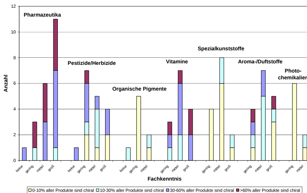
Abbildung 8.3-3: Bedeutung der Chiralität in den Chemiesparten
