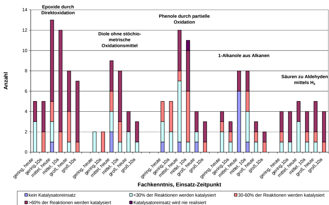
Abbildung 8.2-2a: Katalysatoreinsatz heute und in 10 Jahren bei den Reaktionstypen der Fragen 12-16
