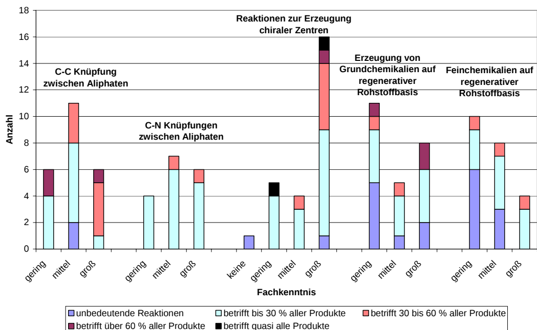
Abbildung 8.1-2b: Heutige Bedeutung in der chemischen Produktion bei den Reaktionstypen der Fragen 7-11
