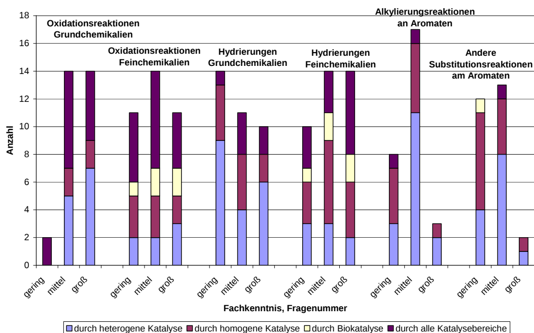
Abbildung 8.1-5a: Angaben zu erwarteten Verbesserungen von Reaktionstypen durch unterschiedliche Katalysatordisziplinen
