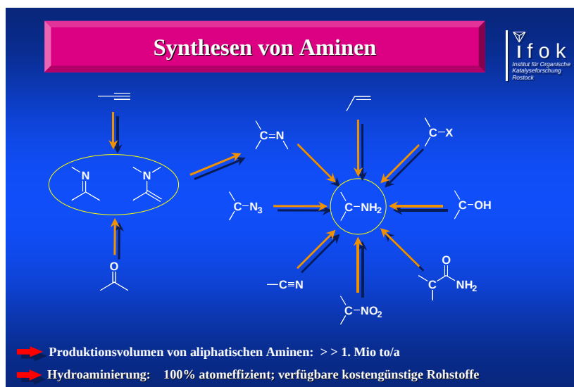
Abbildung 7.1-14: Möglichkeiten der Aminsynthese
