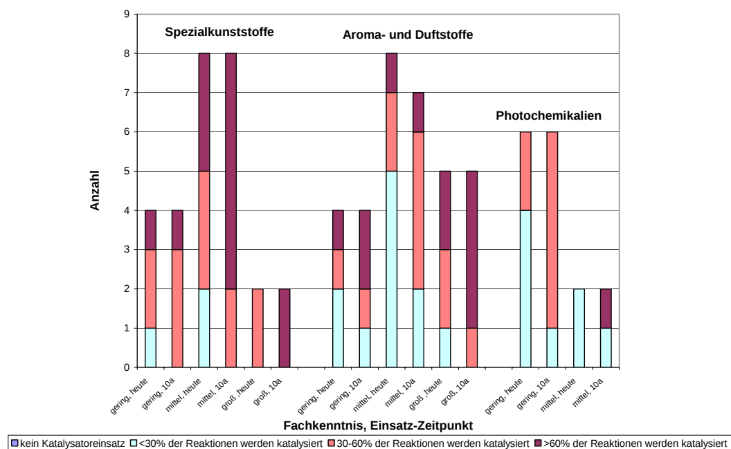
Abbildung 8.3-2b: Katalysatoreinsatz heute und in 10 Jahren in den Chemiesparten
