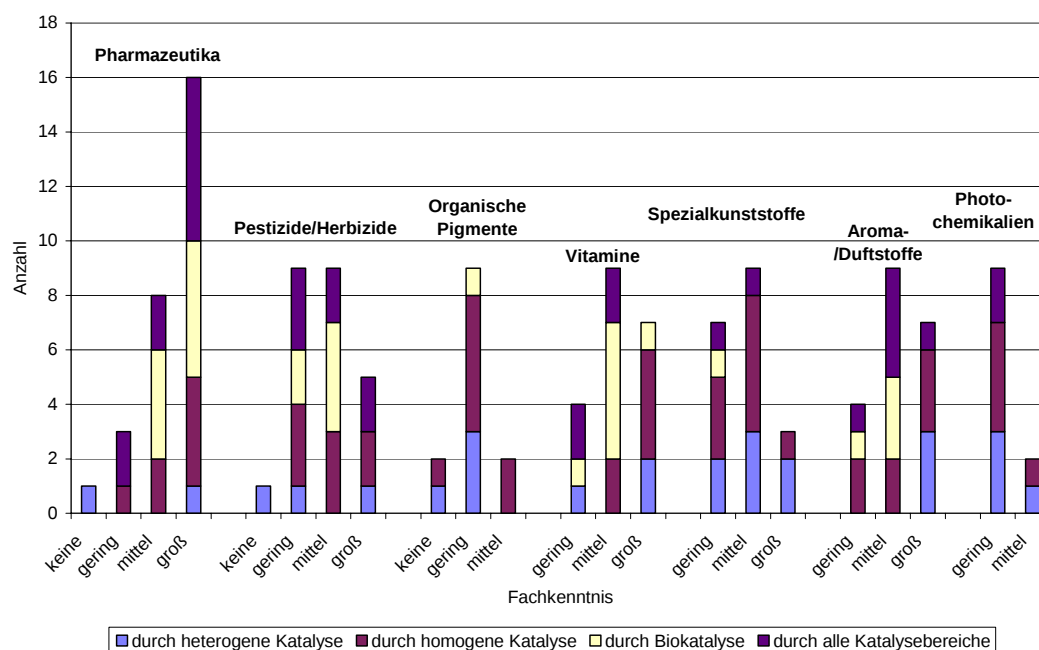
Abbildung 8.3-5: Angaben zur erwarteten Verbesserungen von Reaktionstypen durch unterschiedliche Katalysatordisziplinen
