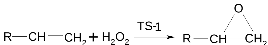
Abbildung 7.1-2: Heterogen-katalytische Herstellung von Epoxiden unter Verwendung von \text{H}_2\text{O}_2 als Oxidationsmittel
