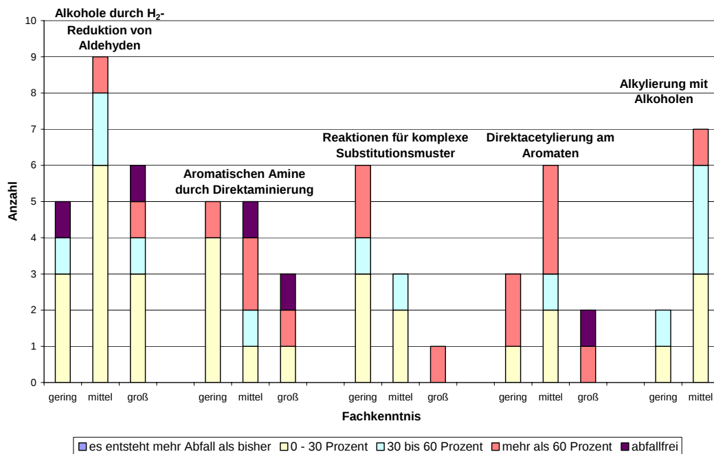
Abbildung 8.2-5b: Mögliche Abfalleinsparungen bei den speziellen Reaktionstypen der Fragen 17– 21
