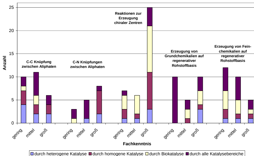
Abbildung 8.1-5b: Angaben zu erwarteten Verbesserungen von Reaktionstypen durch unterschiedliche Katalysatordisziplinen
