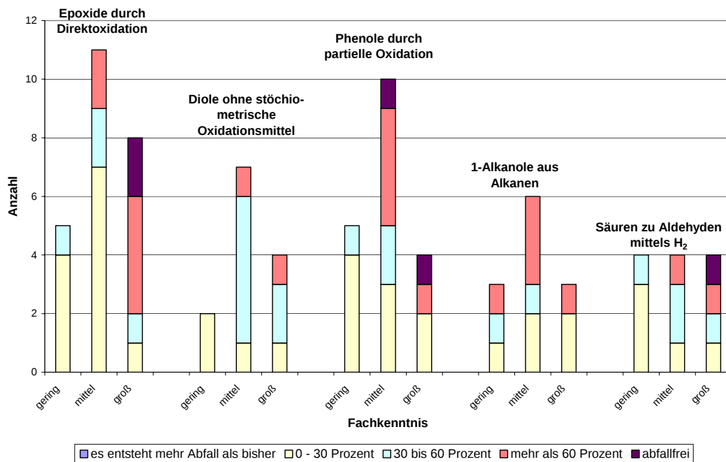
Abbildung 8.2-5a: Mögliche Abfalleinsparungen bei den speziellen Reaktionstypen der Fragen 12 – 16
