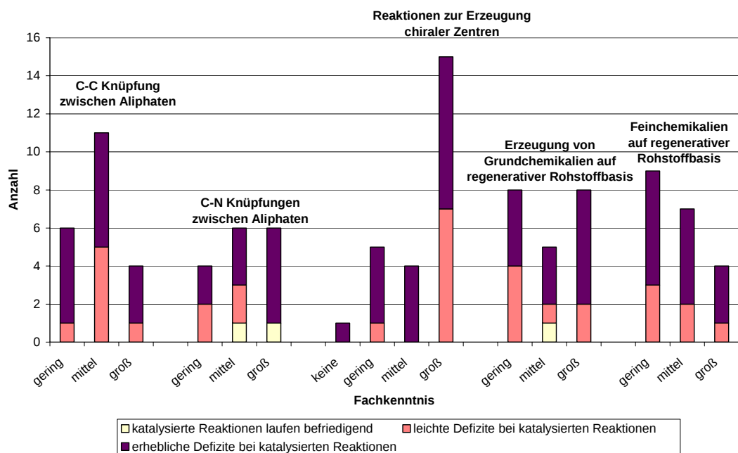
Abbildung 8.1-4b: Angaben zum Verbesserungspotenzial der Reaktionstypen
