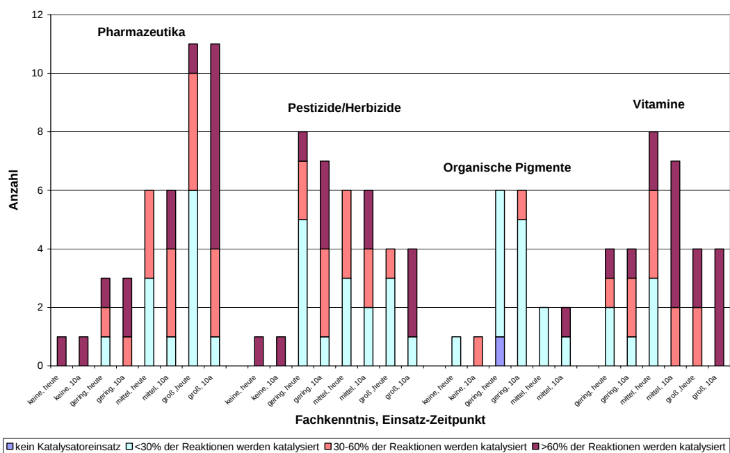
Abbildung 8.3-2a: Katalysatoreinsatz heute und in 10 Jahren in den Chemiesparten
