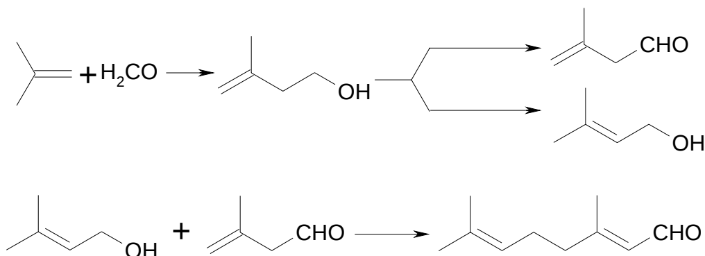
Abbildung 7.1-4: BASF-Citral-Prozess
