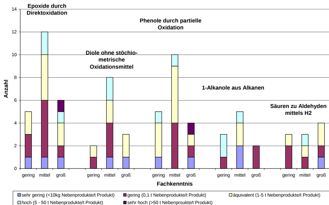
Abbildung 8.2-3a: Derzeitige Abfallmengen bei den speziellen Reaktionstypen der Fragen 12 - 16
