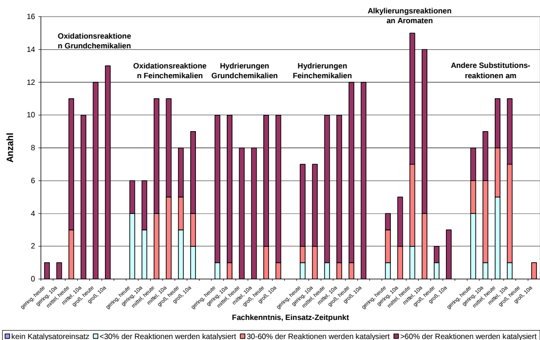
Abbildung 8.1-3a: Katalysatoreinsatz heute und in 10 Jahren bei den Reaktionstypen der Fragen 1-6
