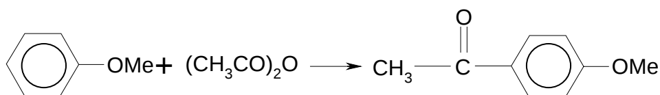
Abbildung 7.1-11: Acetylierung von Anisol
