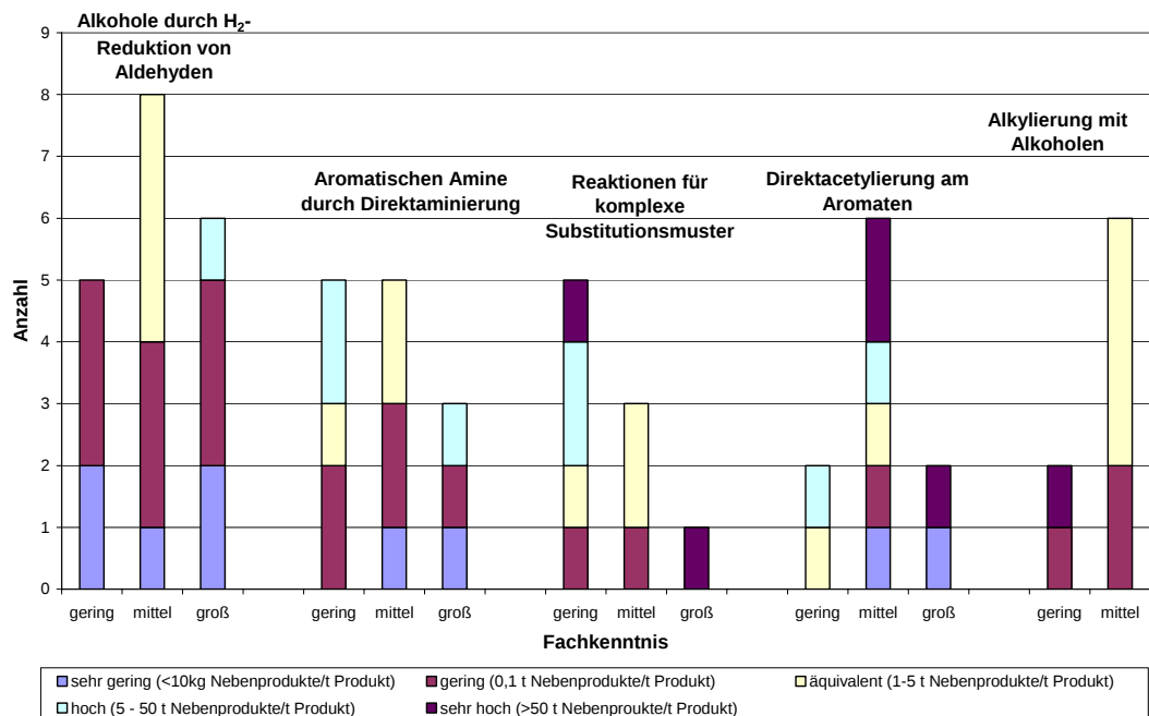
Abbildung 8.2-3b: Derzeitige Abfallmengen bei den speziellen Reaktionstypen der Fragen 17 - 21
