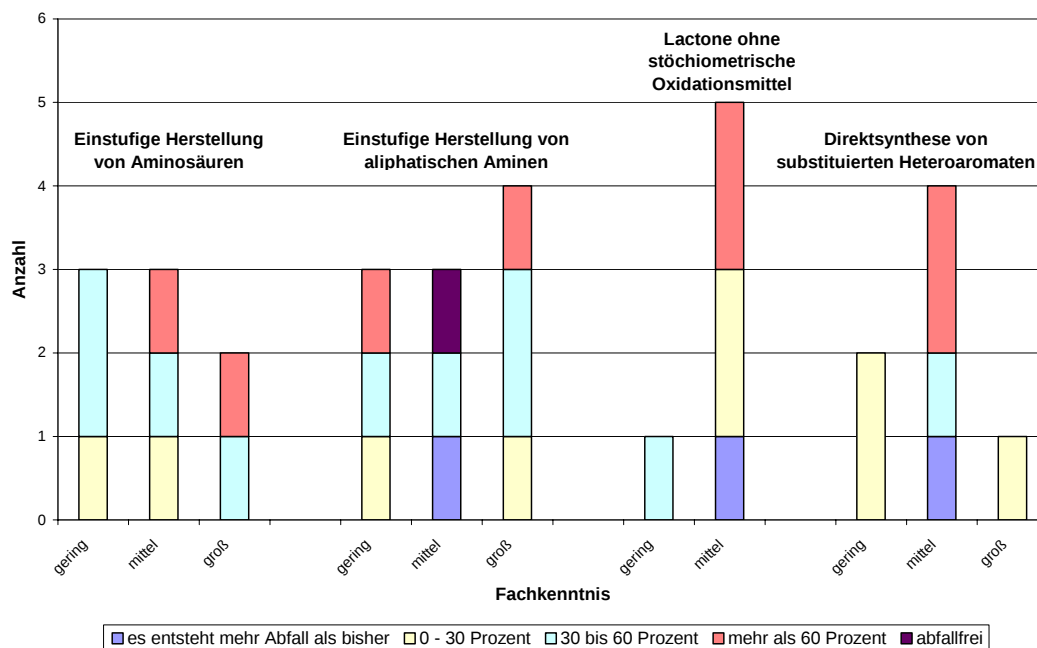
Abbildung 8.2-5c: Mögliche Abfalleinsparungen bei den speziellen Reaktionstypen der Fragen 22-25
