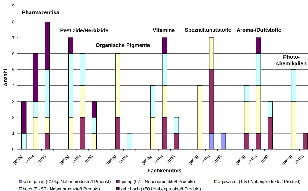
Abbildung 8.3-4: Derzeitige Abfallmengen in den Chemiesparten
