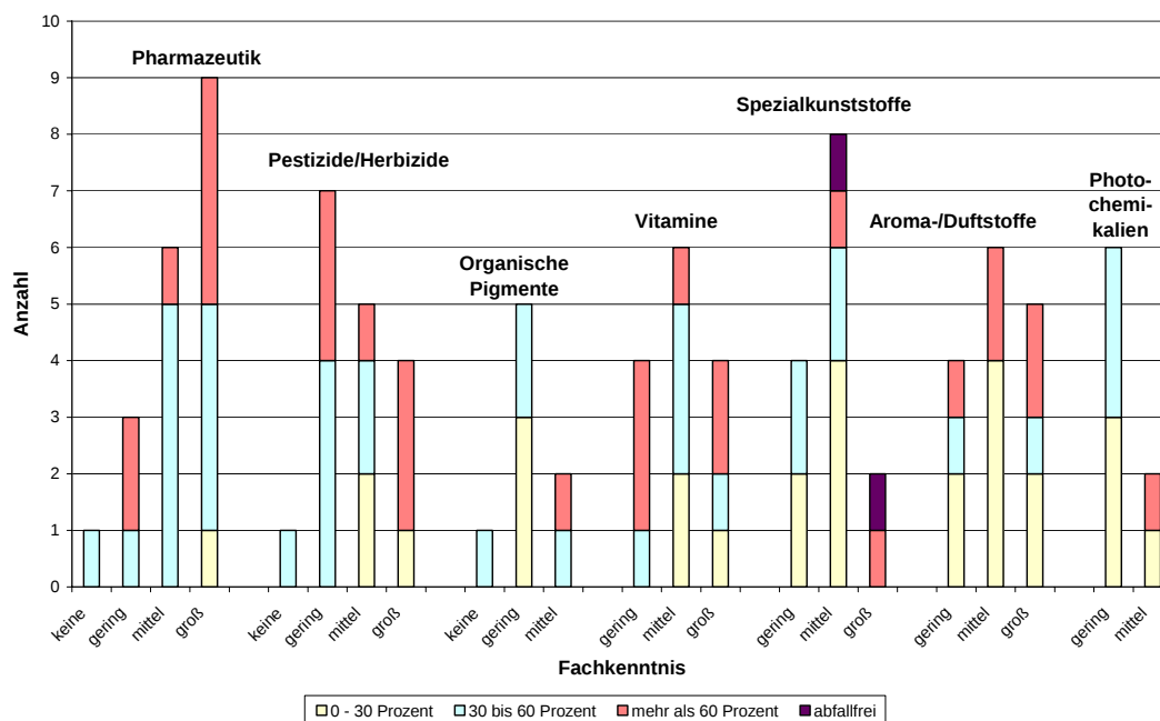
Abbildung 8.3-6: Mögliche Abfalleinsparungen in den Chemiesparten
