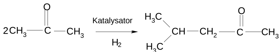
Abbildung 7.1-7: Fortgeschrittenes, einstufiges Katalyseverfahren bei der Herstellung von 4-Methyl-2-pentanon aus Aceton
