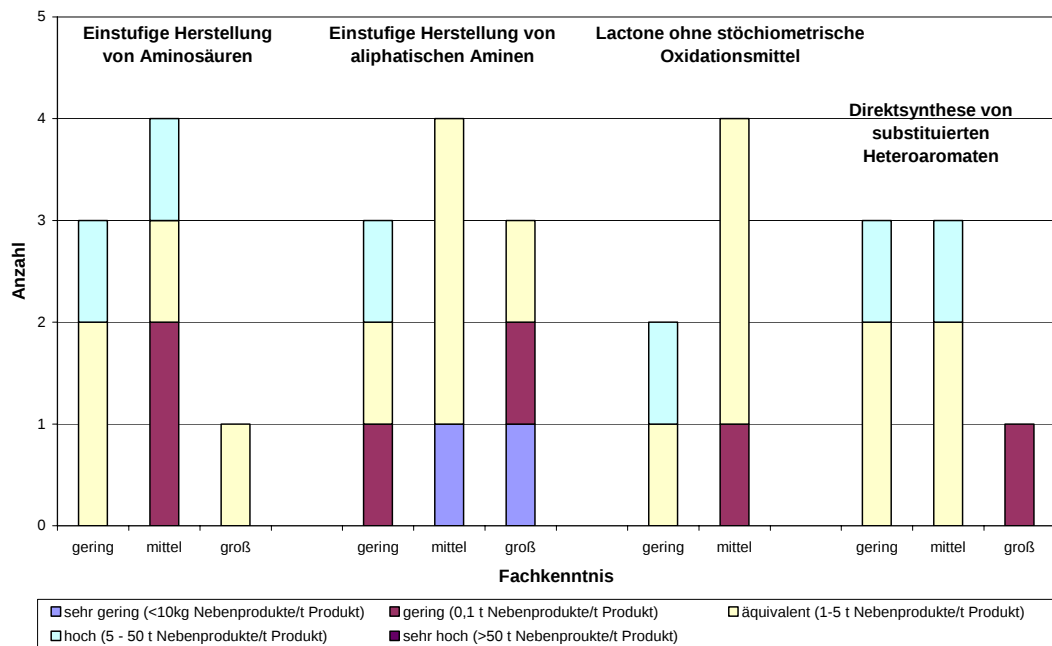
Abbildung 8.2-3c: Derzeitige Abfallmengen bei den speziellen Reaktionstypen der Fragen 22 – 25
