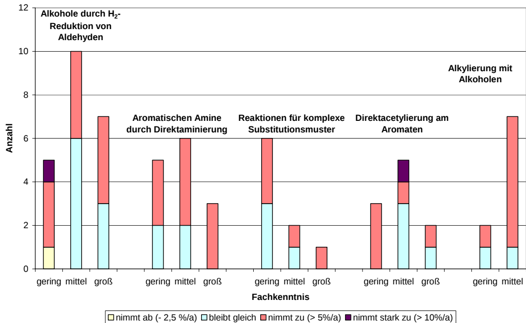
Abbildung 8.2-4b: Angaben zur Entwicklung der Produktionsmenge in den nächsten 10 Jahren für die Fragen 18 – 21
