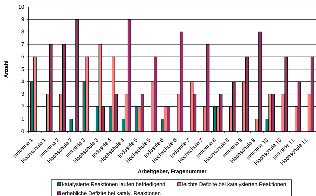
Abbildung 8.1-4c: Vergleich der Einschätzung der Experten zum Verbesserungspotenzial der Reaktionstypen nach Arbeitgeber
