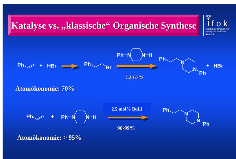
Abbildung 7.1-15: Klassische organische und katalytische Synthese von Aryl-ethyl-aryl-piparazinen
