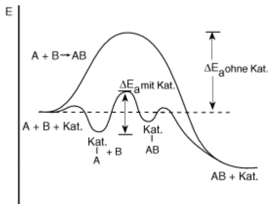
Abbildung 3.2-1: Potentielle Energie (E) entlang der Reaktionskoordinate bei unkatalysierter bzw. katalysierter Reaktion der Teilchen A und B zu AB.
