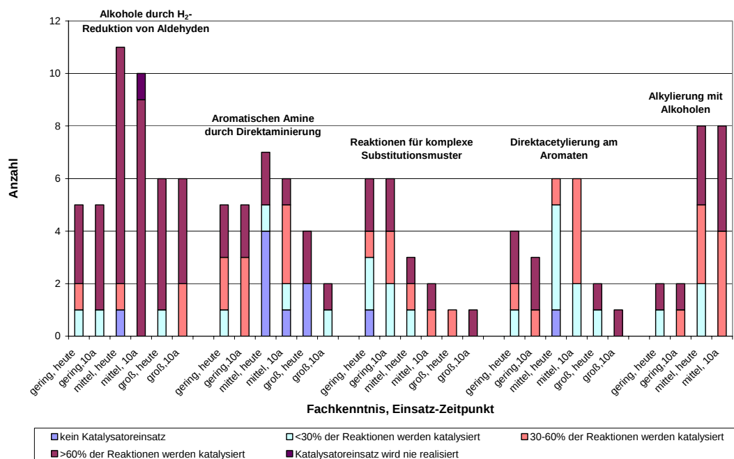
Abbildung 8.2-2b: Katalysatoreinsatz heute und in 10 Jahren bei den Reaktionstypen der Fragen 17-21
