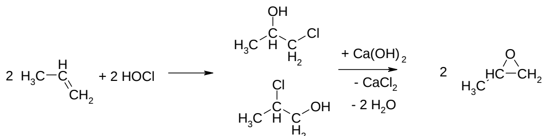
Abbildung 7.1-1: Klassische Synthese von Epoxiden über das Chlorhydrinverfahren
