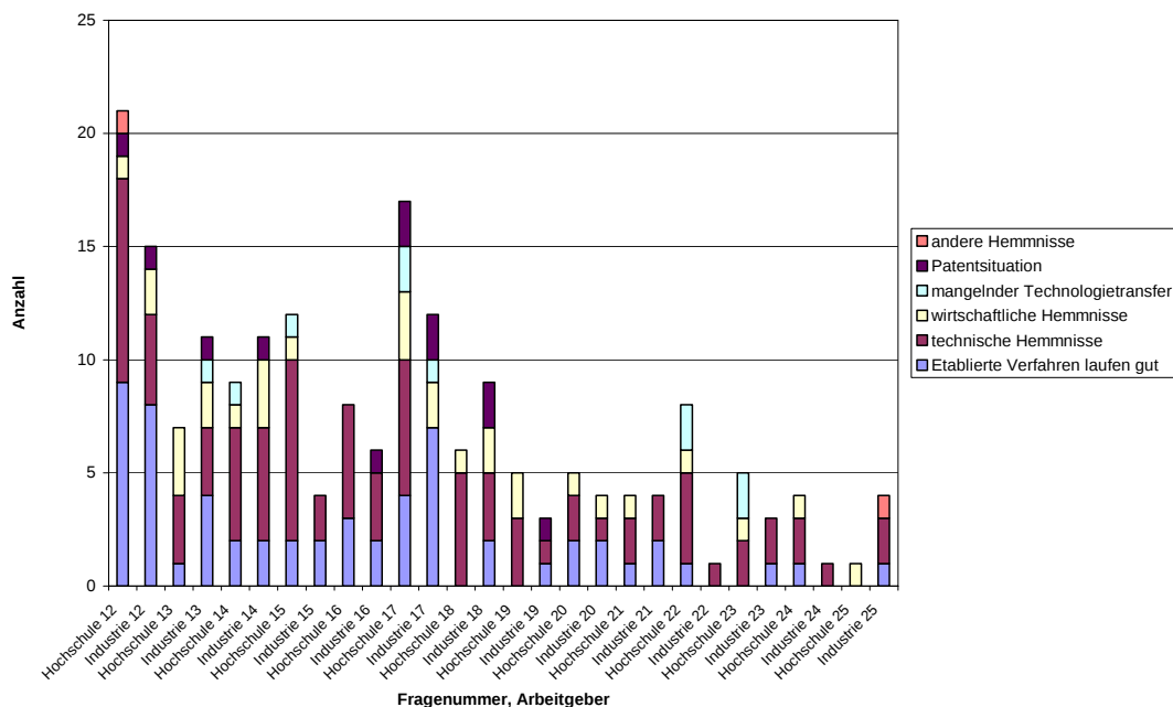
Abbildung 10-1: Von Experten aus Hochschule und Industrie genannte Hemmnisse des Einsatzes neuer Katalysatoren
