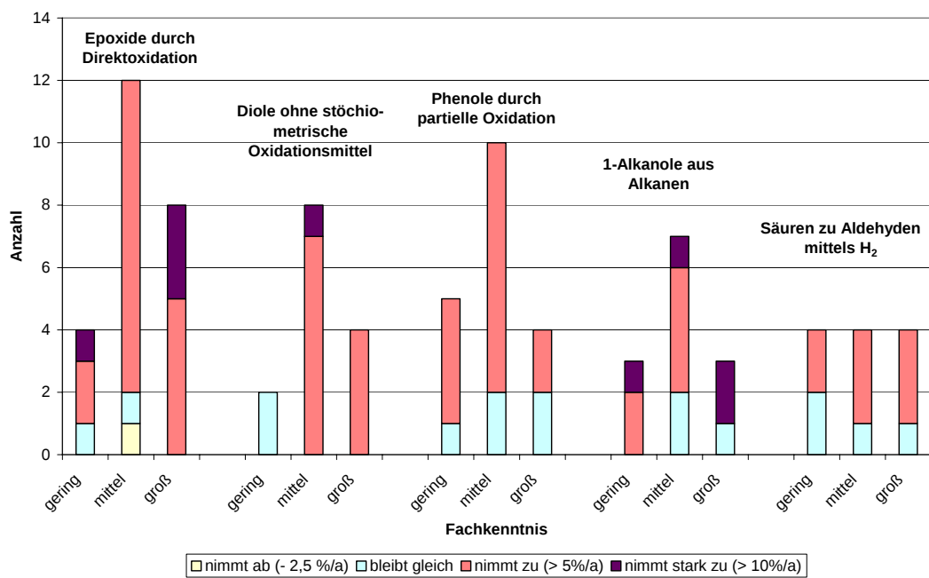
Abbildung 8.2-4a: Angaben zur Entwicklung der Produktionsmenge in den nächsten 10 Jahren für die Fragen 12 – 17
