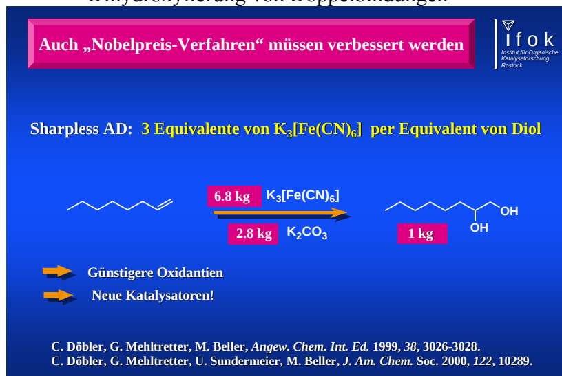
Abbildung 7.1-3: Katalytische Herstellung chiraler Diole durch asymmetrische Dihydroxylierung von Doppelbindungen
