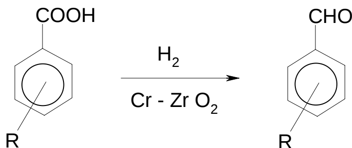
Abbildung 7.1-5: Gewinnung aromatischer Aldehyde durch direkte katalytische Hydrierung
