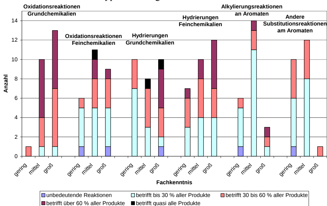
Abbildung 8.1-2a: Heutige Bedeutung in der chemischen Produktion bei den Reaktionstypen der Fragen 1-6
