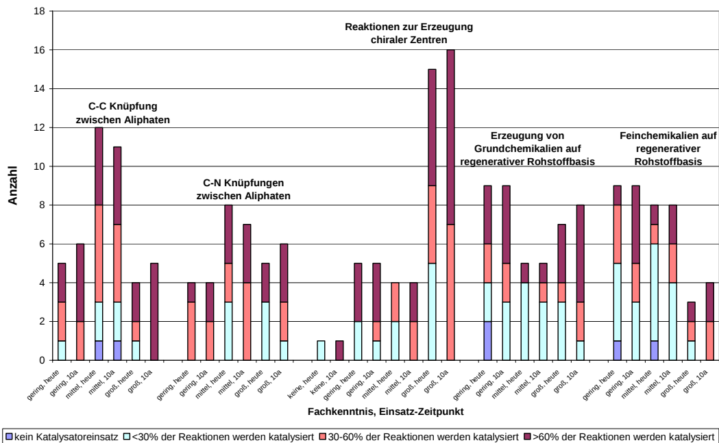
Abbildung 8.1-3b: Katalysatoreinsatz heute und in 10 Jahren bei den Reaktionstypen der Fragen 7-11
