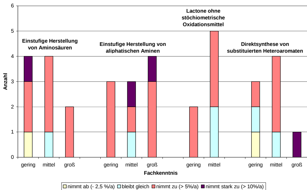
Abbildung 8.2-4c: Angaben zur Entwicklung der Produktionsmenge in den nächsten 10 Jahren für die Fragen 22 – 25
