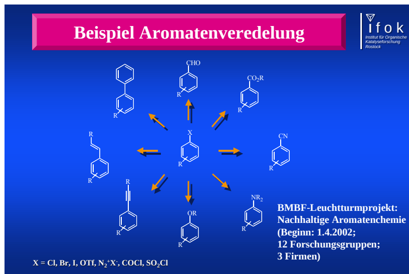
Abbildung 7.1-8: Direktfunktionalisierungen an Aromaten
