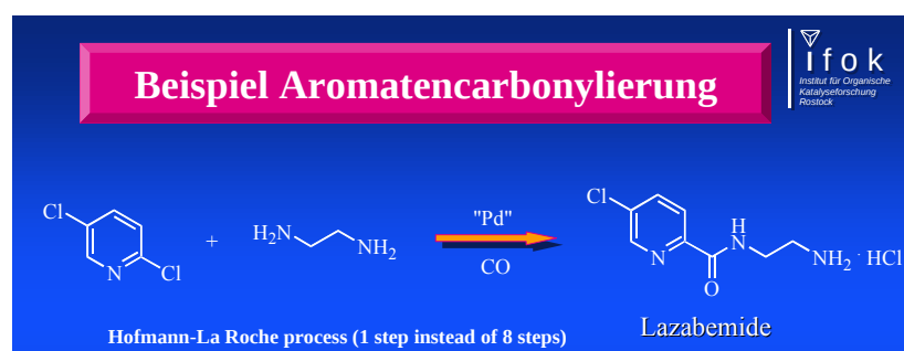
Abbildung 7.1-10: Einstufige katalytische Synthese von Lazabemid
