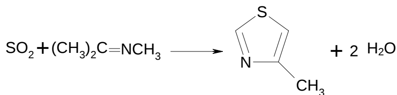
Abbildung 7.1-13: Aufbau eines substituierten Thiazols
