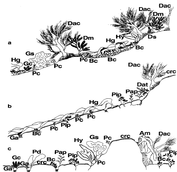
Abb. 3.4-8 Beispiel für sublitorale Lebensgemeinschaften unter zunehmendem Einfluß von Turbulenz und auflaufenden Eisbergen in der Niederen Antarktis (aus: Klöser et al. 1994)
