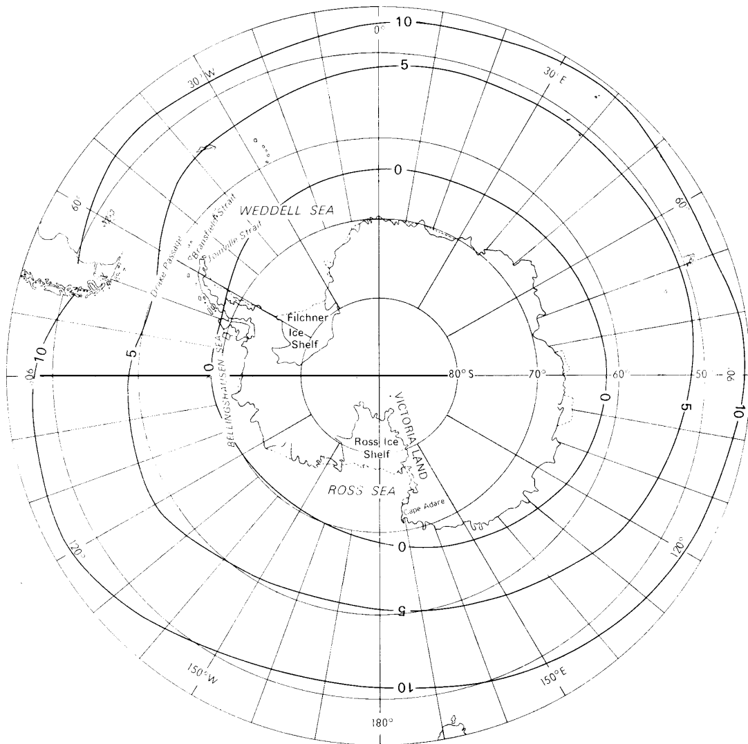
Isothermen der mittleren Lufttemperatur in °C im Januar [148]
