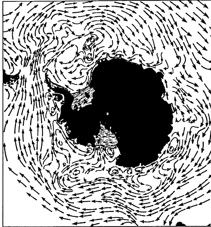
Abb. 3.4-2 Strömungen im antarktischen Ozean (aus Foster 1984)
