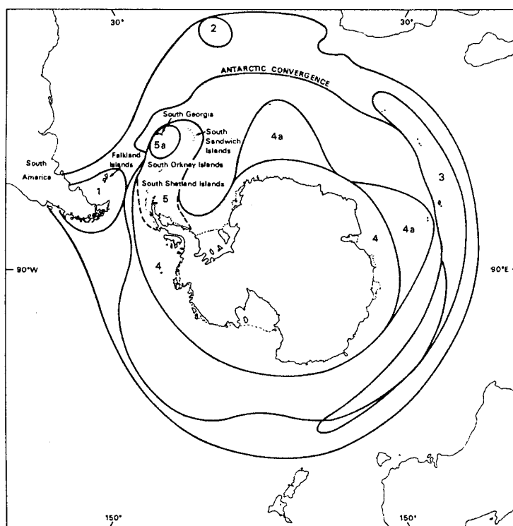
Abb. 3.2-1 Konventionelle Abgrenzung der Subantarktis, Niederen und Hoch-Antarktis (aus White 1984 nach Hedgpeth 1969)
