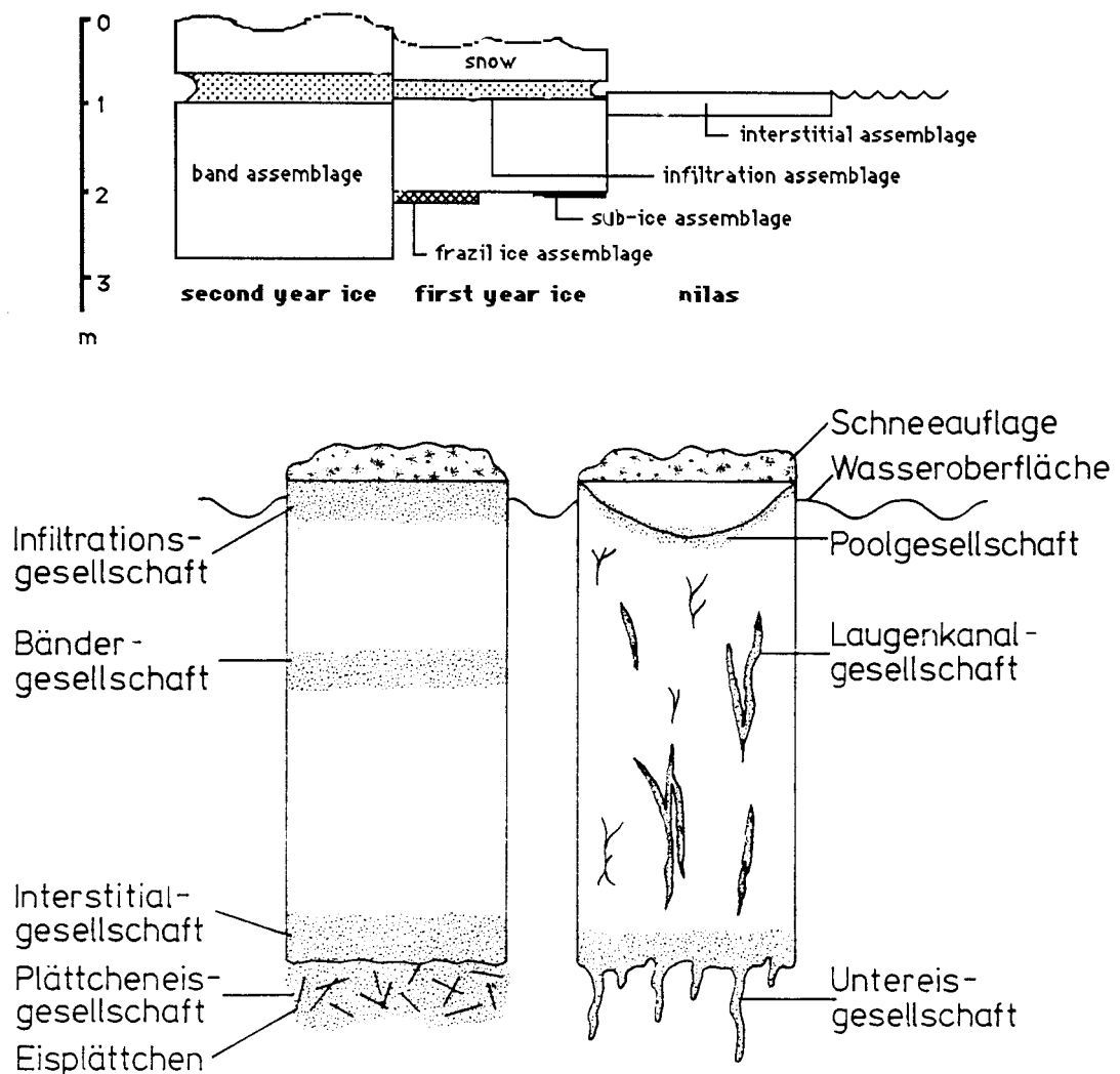
Abb. 3.4-4 Schema verschiedener Lebensgemeinschaften im Meereis (aus Bartsch 1989 nach Horner et al. 1988).
