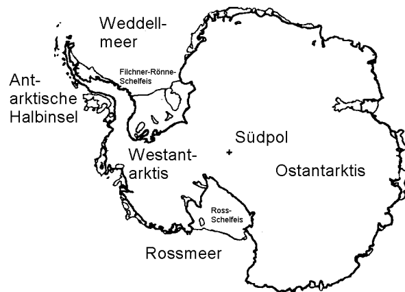
Abb. 3.2-2 Topographische Karte der Antarktis
