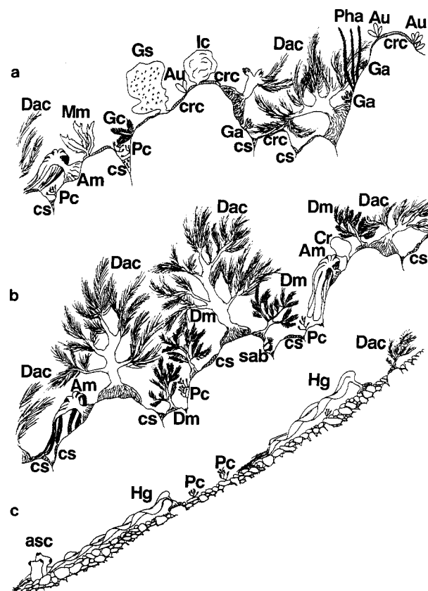
Abb. 3.4-6 Zonierung des Sublitorals in der Niederen Antarktis unter geschützten Bedingungen(aus: Klöser et al. 1994)
