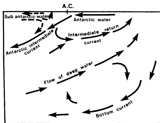
Abb. 3.4-1 Blockdiagramm der antarktischen Wassermassen und Strömungssysteme (aus Hempel 1985 nach Gordon & Goldberg 1970).
