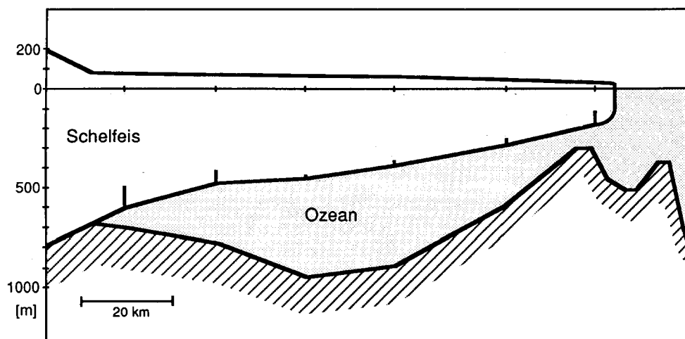
Abb. 3.2-3 Blockbild zum Aufbau einer Schelfeisküste (aus Kipfstuhl 1991, verändert)
