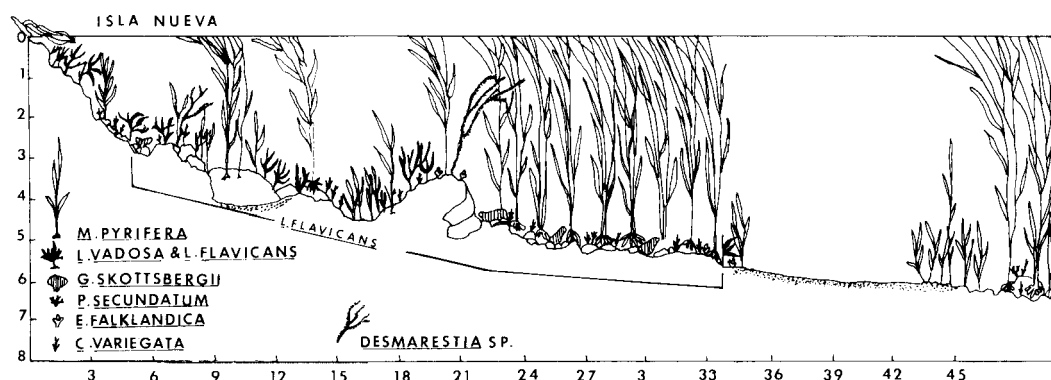
Abb. 3.4-5 Beispiel für die Zonierung im Litoral und Sublitoral an einer subantarktischen Küste: Isla Nueva am östlichen Ausgang des Beagle-Kanals (aus Santelices 1989). 12
