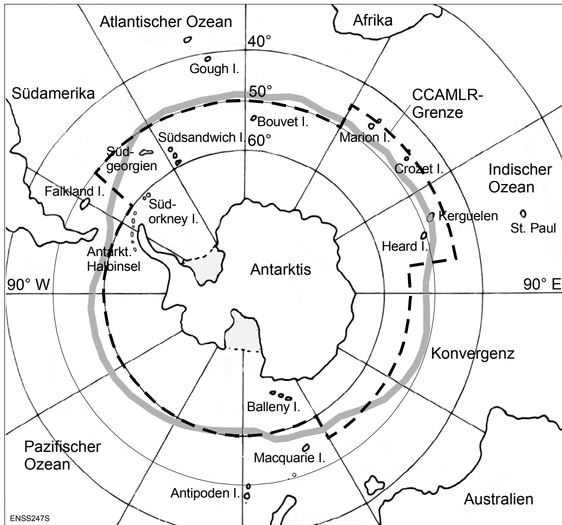
Abb. 3-1 Übersichtskarte des Antarktisgebiets mit Antarktischer Konvergenz
