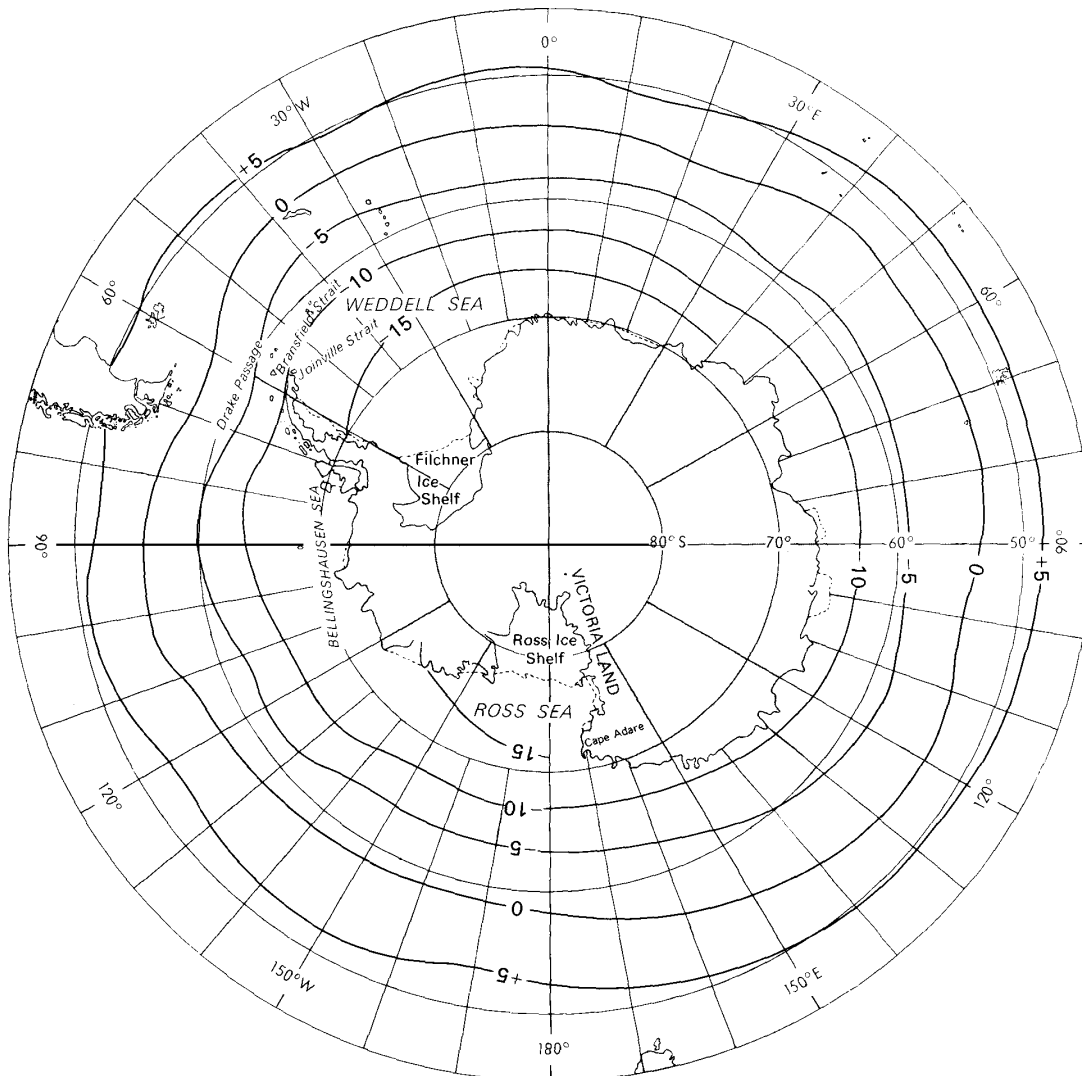
Isothermen der mittleren Lufttemperatur in °C im Juli [148]
