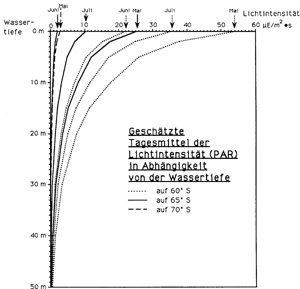
Abb. 3.4-3 Winterliche Lichtbedingungen in Abhängigkeit verschiedener Breiten (aus Klöser 1990).
