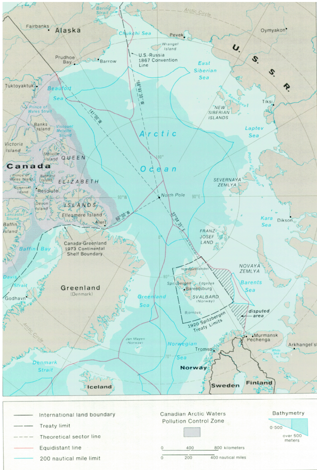
Abb. 3.5-1 Nordpolargebiet (nach CIA 1978)
