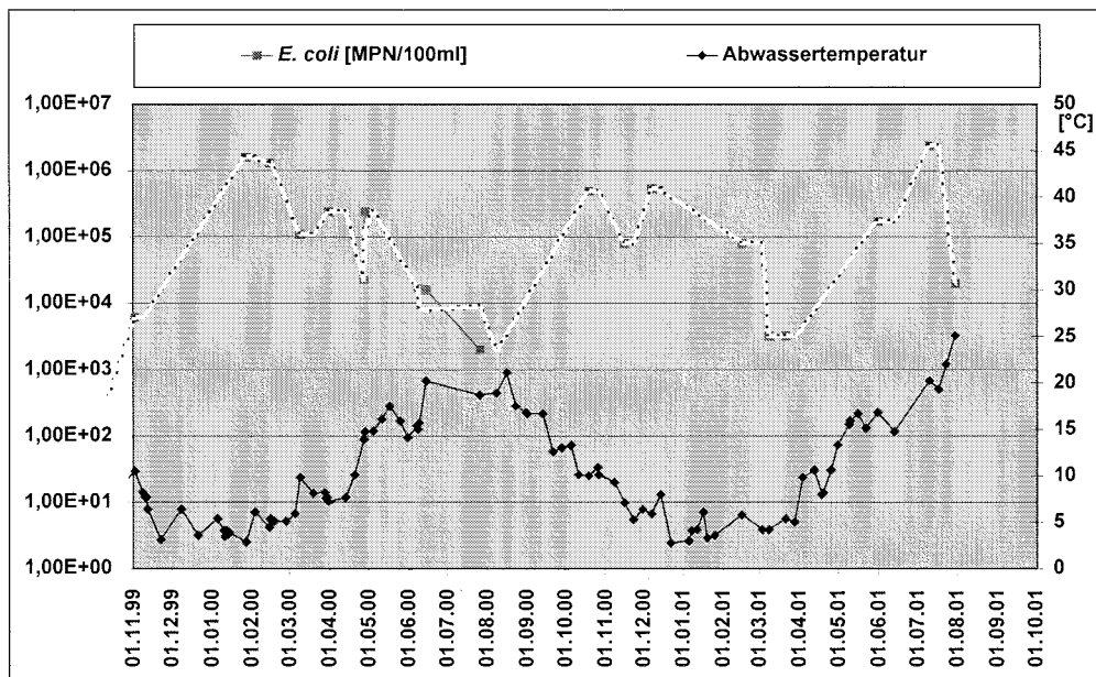
Abb. 5.3.5: Konzentration von E. coli im Vergleich zur Abwassertemperatur, Ablauf Teich 2 Anlage Ettenbüttel
