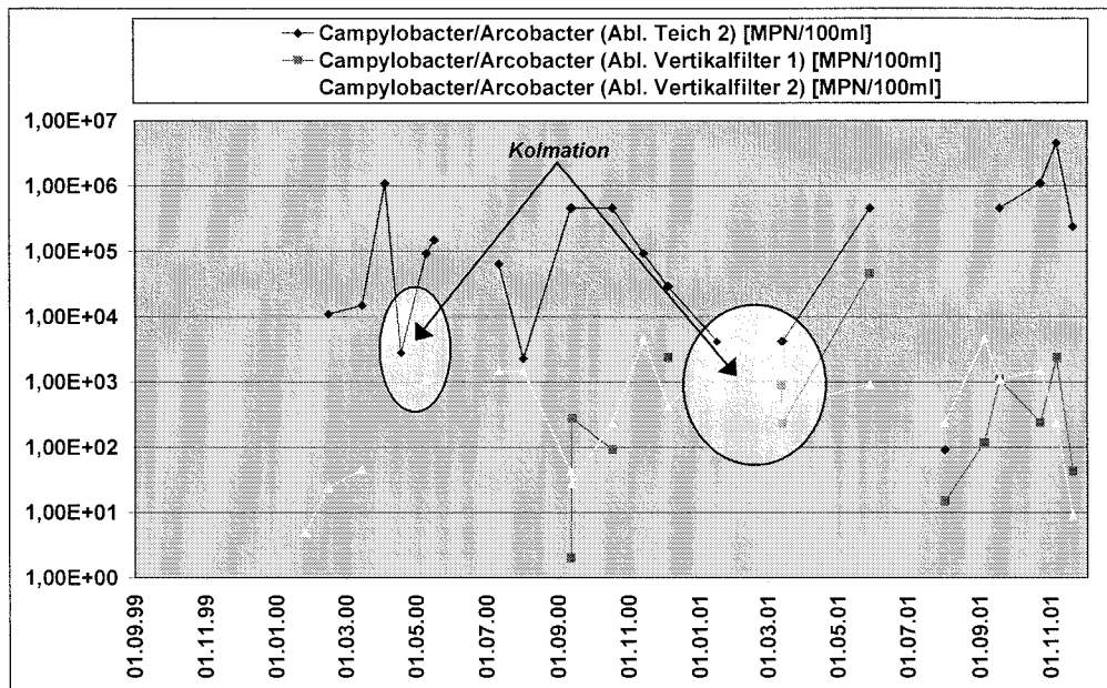
Abb. 5.3.7: Konzentrationen von Campylobacter/Arcobacter in Abläufen Vorklärung, Vertikalfilter 1 und Vertikalfilter 2, Anlage Ettenbüttel
