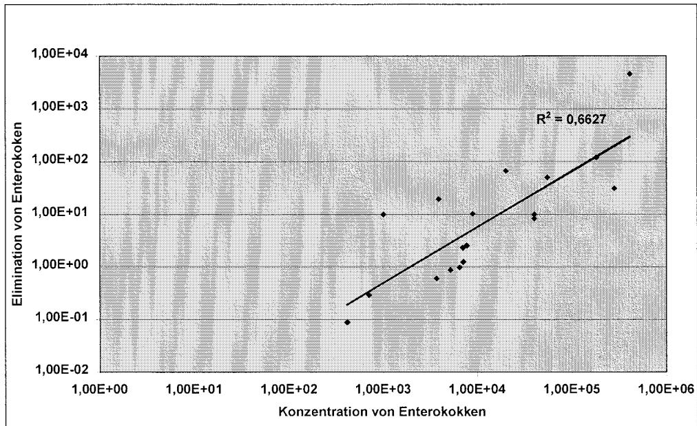
Anhang 4, Abb. 5.3.14: Elimination von Enterokokken im Vergleich zur Zulaufkonzentration, Vertikalfilter 1, Anlage Ettenbüttel
