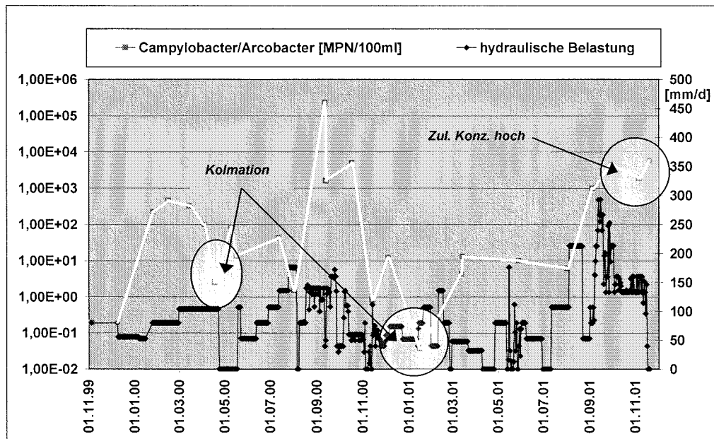
Anhang 4, Abb. 5.3.22: Elimination von Campylobacter/Arcobacter im Vergleich zur hydraulischen Belastung, Vertikalfilter 2, Anlage Ettenbüttel
