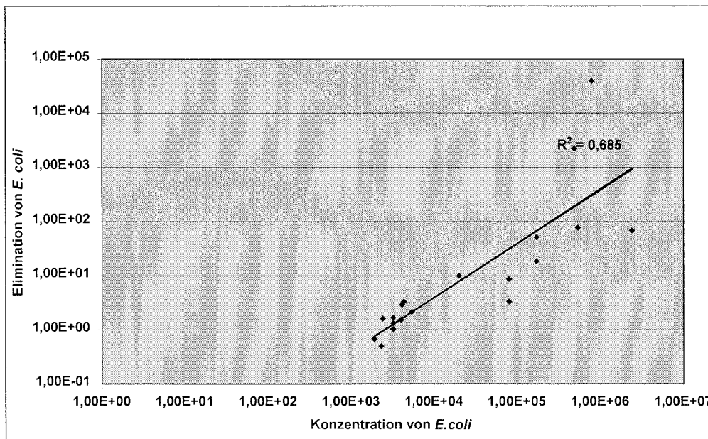
Abb. 5.3.6: Elimination von E. coli im Vergleich zur Zulaufkonzentration, Vertikalfilter 1 Anlage Ettenbüttel
