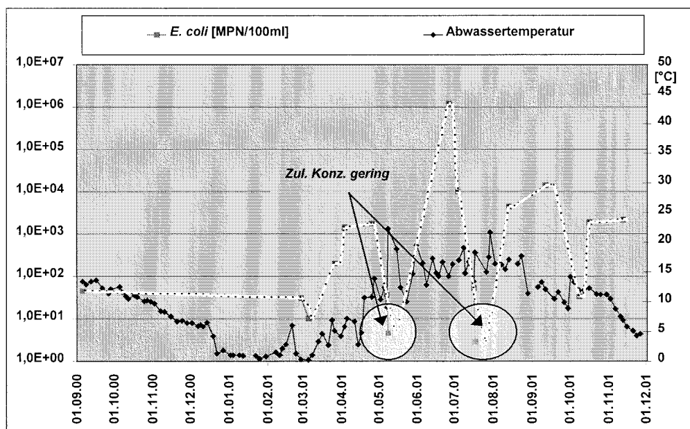
Abb. 5.4.8: Elimination von E. coli im Vergleich zur Abwassertemperatur, Horizontalfilter 1 Anlage See
