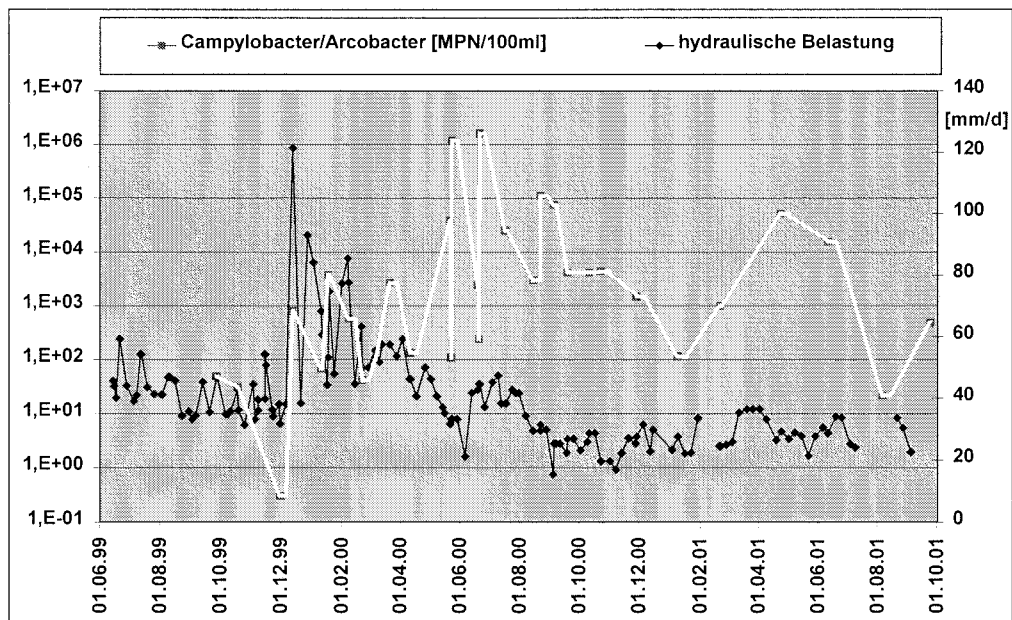
Anhang 4, Abb. 5.2.22: Elimination von Campylobacter/Arcobacter im Vergleich zur hydraulischen Belastung, Horizontalfilter, Anlage Wiedersberg
