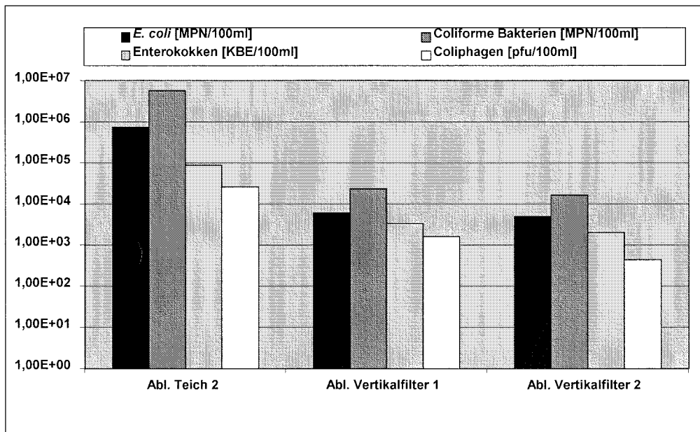
Abb. 5.3.1 Mikrobiologische Untersuchungsergebnisse Indikatororganismen (Mittelwerte), Anlage Ettenbüttel
