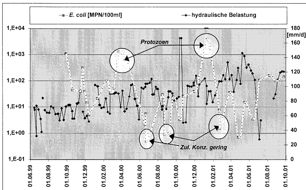
Abb. 5.2.11: Elimination von E. coli im Vergleich zur hydraulischen Belastung, Vertikalfilter Anlage Wiedersberg
