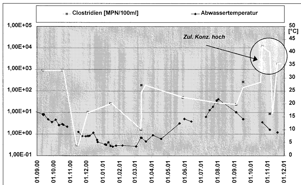
Anhang 4, Abb. 5.3.17: Elimination von Clostridien im Vergleich zur Abwassertemperatur, Vertikalfilter 1, Anlage Ettenbüttel
