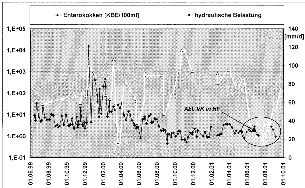
Abb. 5.2.14: Elimination von Enterokokken im Vergleich zur hydraulischen Belastung, Horizontalfilter Anlage Wiedersberg
