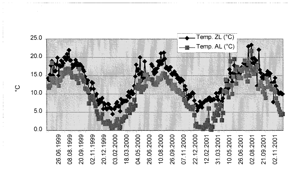
Abb. 4.5: Abwassertemperatur Anlage See
