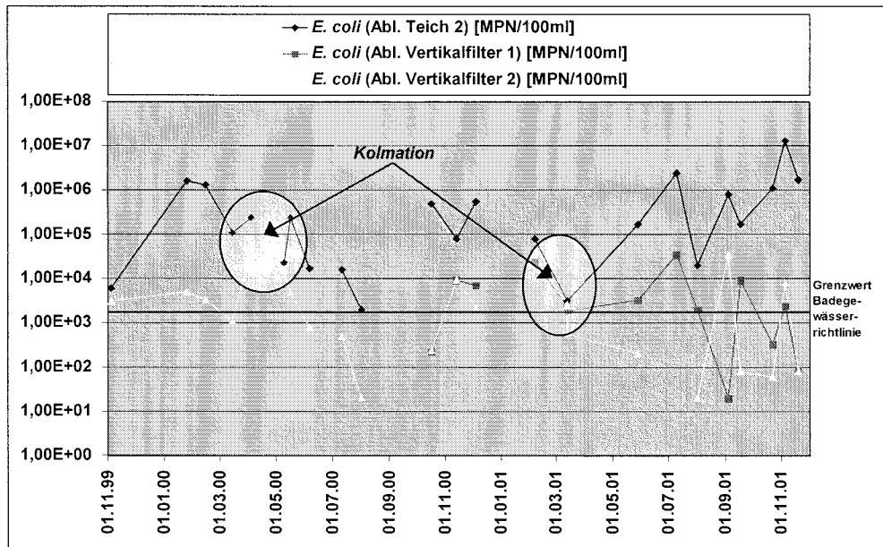
Abb. 5.3.3: Konzentrationen von E. coli in Abläufen Vorklärung, Vertikalfilter 1 und Vertikalfilter 2, Anlage Ettenbüttel
