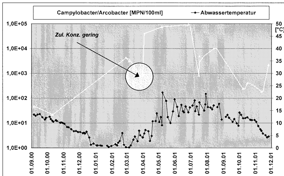
Anhang 4, Abb. 5.4.14: Elimination von Campylobacter/Arcobacter im Vergleich zur Abwassertemperatur, Horizontalfilter 1, Anlage See
