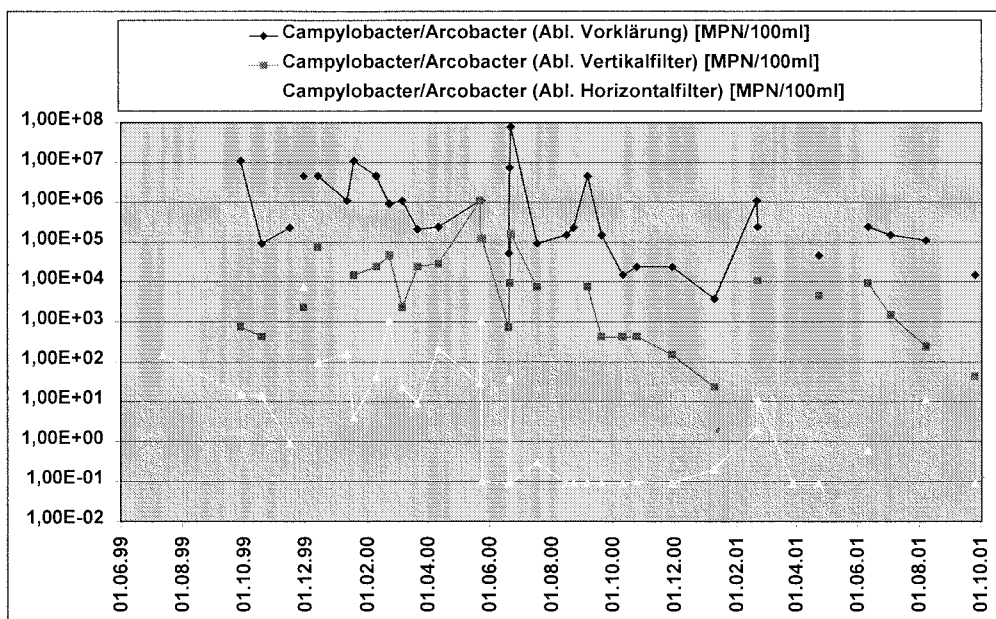
Abb. 5.2.8: Konzentrationen von Campylobacter/Arcobacter in Abläufen Vorklärung, Vertikal- und Horizontalfilter, Anlage Wiedersberg
