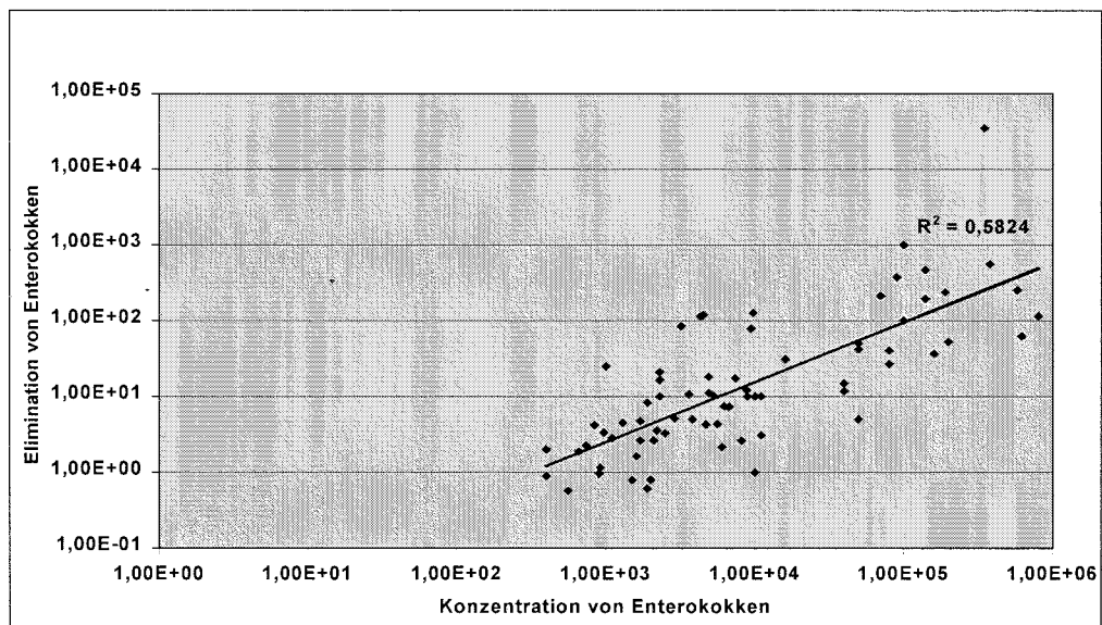
Abb. 5.2.7: Elimination von Enterokokken im Vergleich zur Zulaufkonzentration, Vertikalfilter Anlage Wiedersberg
