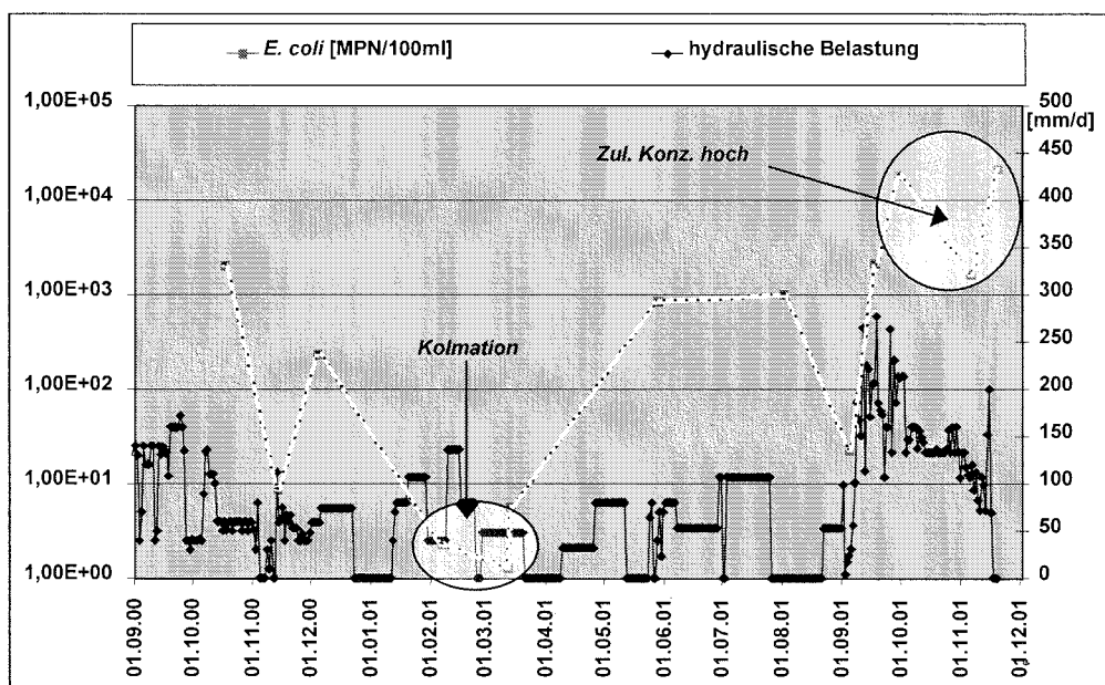
Abb. 5.3.10: Elimination von E. coli im Vergleich zur hydraulischen Belastung, Vertikalfilter 1 Anlage Ettenbüttel
