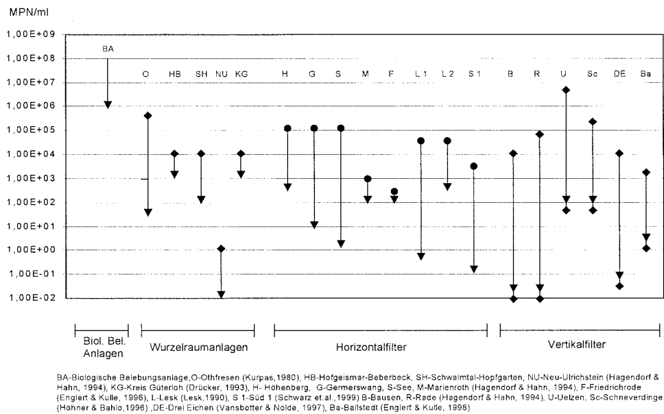
Abb. 3.1: Verminderung von E. coli im Abwasser durch Bewachsene Bodenfilter
