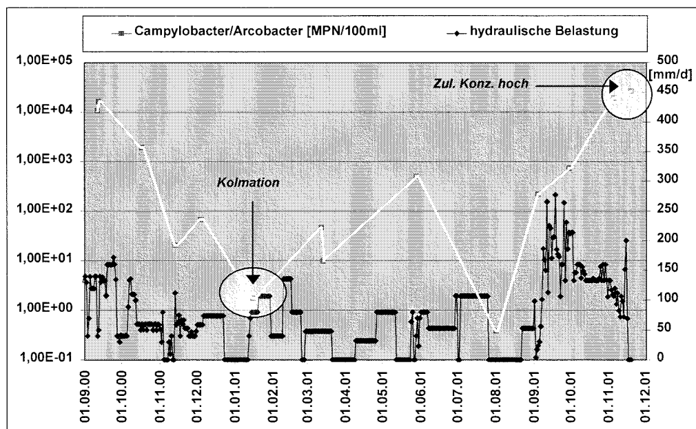
Anhang 4, Abb. 5.3.19: Elimination von Campylobacter/Arcobacter im Vergleich zur hydraulischen Belastung, Vertikalfilter 1, Anlage Ettenbüttel
