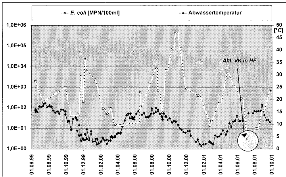
Anhang 4, Abb. 5.2.19: Elimination von E. coli im Vergleich zur Abwassertemperatur, Horizontalfilter, Anlage Wiedersberg
