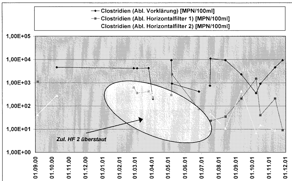
Anhang 4, Abb. 5.4.13: Konzentrationen von Clostridien in Abläufen Vorklärung, Horizontalfilter 1 und Horizontalfilter 2, Anlage See
