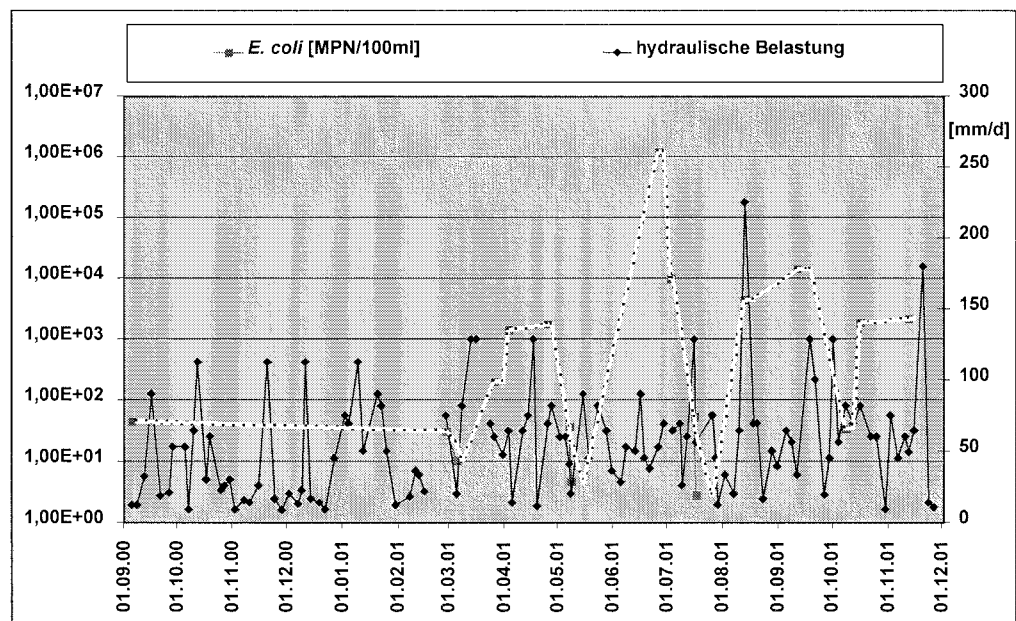
Anhang 4, Abb. 5.4.16: Elimination von E. coli im Vergleich zur hydraulischen Belastung, Horizontalfilter 1, Anlage See
