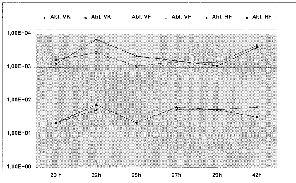
Abb. 5.1.2: Konzentrationen von E. coli in Abhängigkeit von der Standzeit (20 – 24 h), Anlage Wiedersberg
