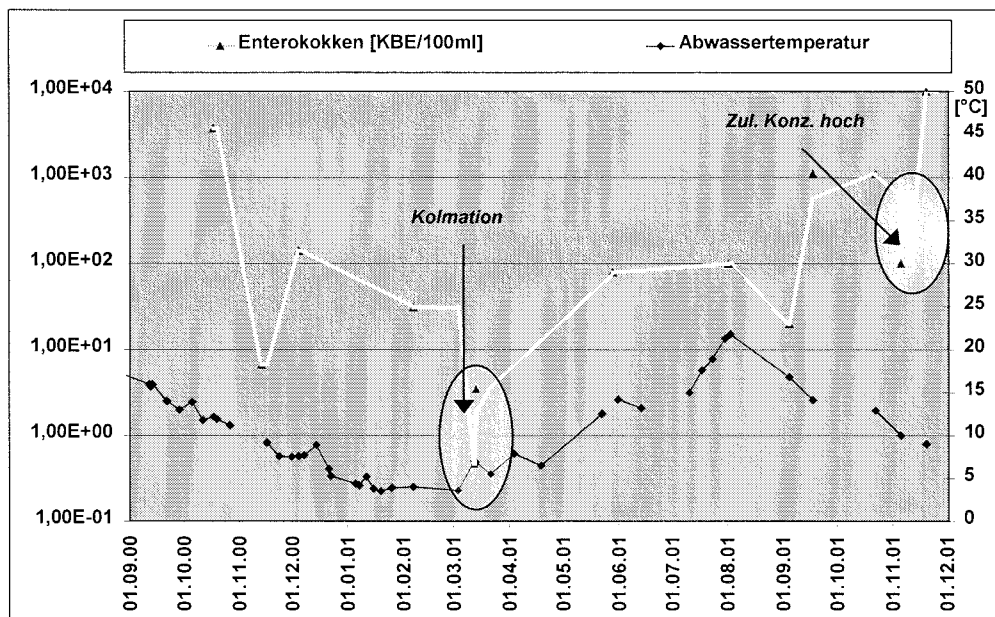
Anhang 4, Abb. 5.3.16: Elimination von Enterokokken im Vergleich zur Abwassertemperatur, Vertikalfilter 1, Anlage Ettenbüttel
