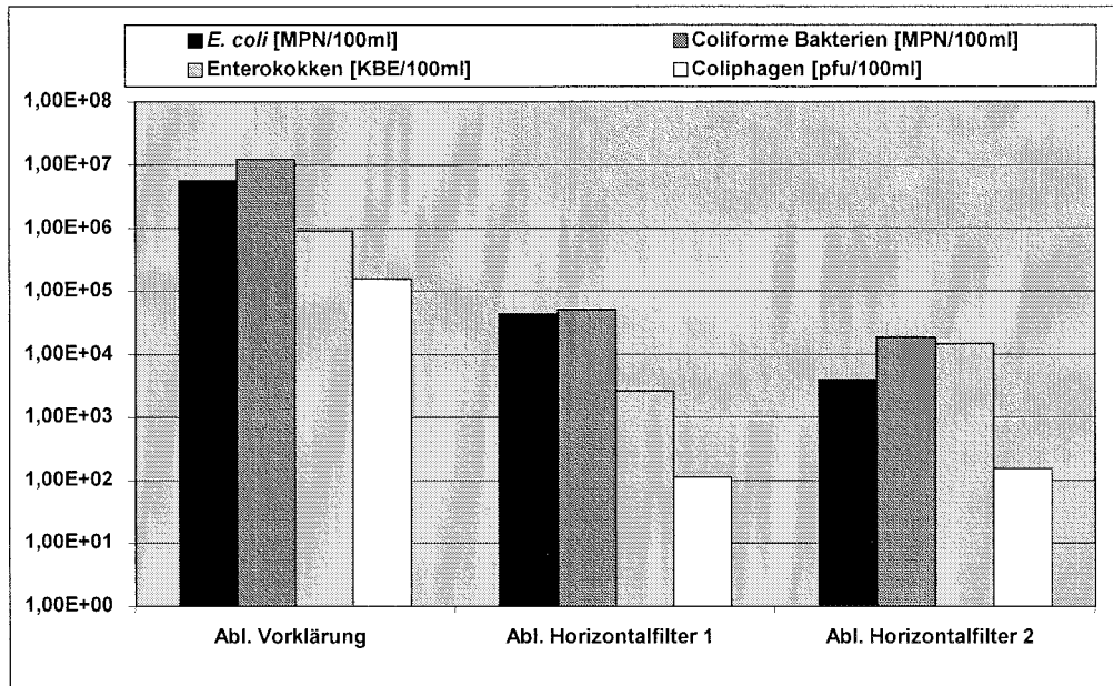
Abb. 5.4.4: Mikrobiologische Untersuchungsergebnisse Indikatororganismen (Mittelwerte), Anlage See
