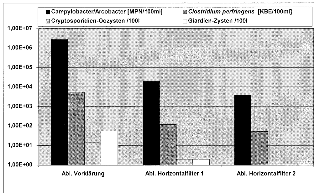
Abb. 5.4.5: Mikrobiologische Untersuchungsergebnisse pathogene Mikroorganismen (Mittelwerte), Anlage See
