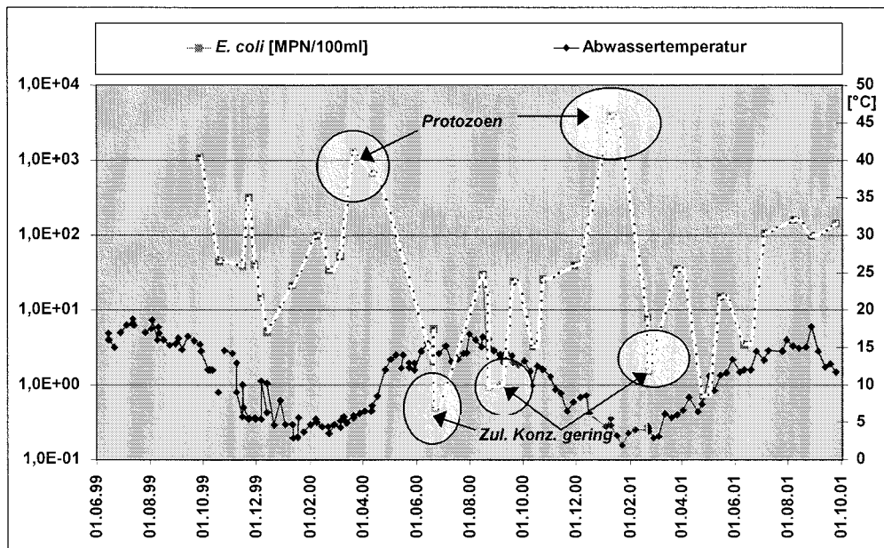
Abb. 5.2.10: Elimination von E. coli im Vergleich zur Abwassertemperatur, Vertikalfilter Anlage Wiedersberg
