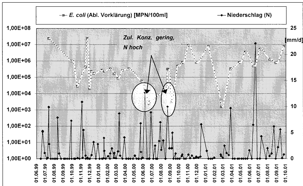
Abb. 5.2.5: Konzentrationen von E. coli im Ablauf Vorklä rung im Vergleich zum Niederschlag, Anlage Wiedersberg
