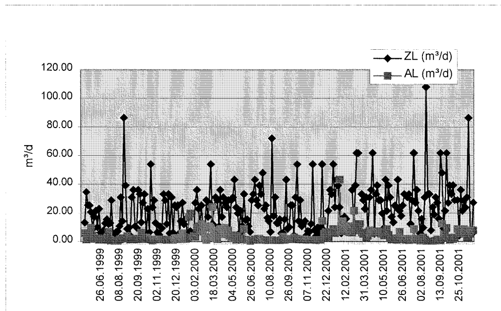
Abb. 4.4: Hydraulische Belastung Anlage See
