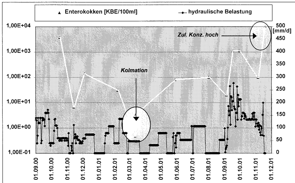
Anhang 4, Abb. 5.3.18: Elimination von Enterokokken im Vergleich zur hydraulischen Belastung, Vertikalfilter 1, Anlage Ettenbüttel
