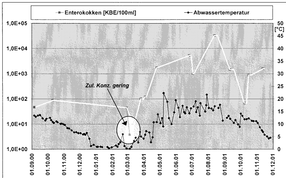
Abb. 5.4.9: Elimination von Enterokokken im Vergleich zur Abwassertemperatur, Horizontalfilter 1 Anlage See
