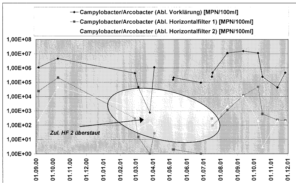
Anhang 4, Abb. 5.4.12: Konzentration von Campylobacter/Arcobacter in Abläufen Vorklärung, Horizontalfilter 1 und Horizontalfilter 2, Anlage See
