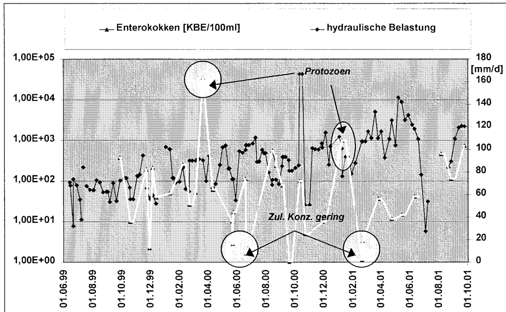
Anhang 4, Abb. 5.2.17: Elimination von Enterokokken im Vergleich zur hydraulischen Belastung, Vertikalfilter, Anlage Wiedersberg
