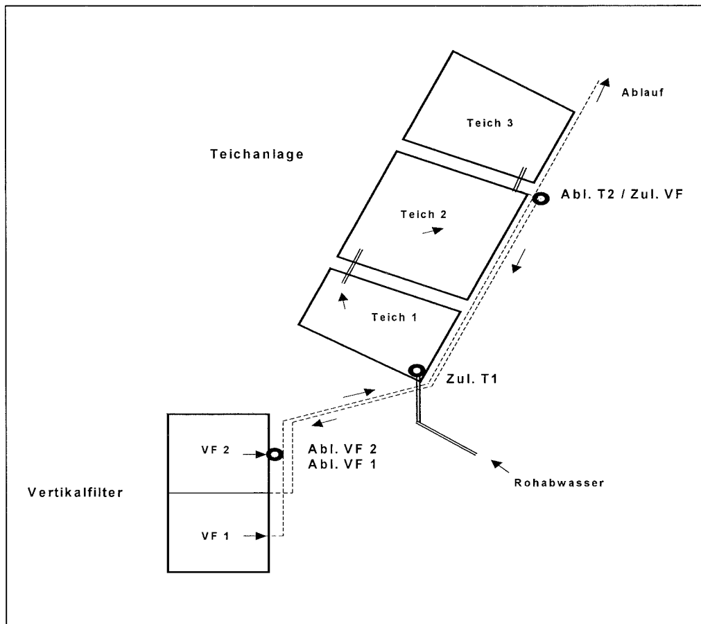
Abb. 4.2: Lageplan Anlage Ettenbüttel mit Probenahmestellen
