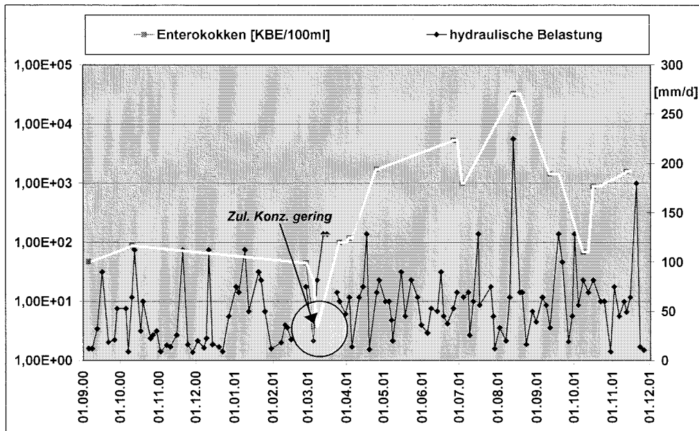
Abb. 5.4.10: Elimination von Enterokokken im Vergleich zur hydraulischen Belastung, Horizontalfilter 1 Anlage See
