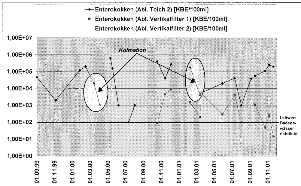
Abb. 5.3.4: Konzentrationen von Enterokokken in Abläufen Vorklärung, Vertikalfilter 1 und Vertikalfilter 2, Anlage Ettenbüttel
