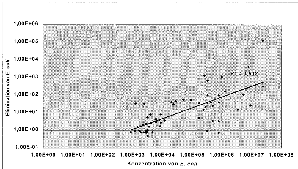
Abb. 5.2.6: Elimination von E. coli im Vergleich zur Zulaufkonzentration, Vertikalfilter Anlage Wiedersberg
