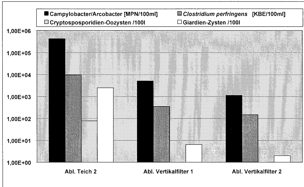
Abb. 5.3.2: Mikrobiologische Untersuchungsergebnisse pathogene Mikroorganismen (Mittelwerte), Anlage Ettenbüttel
