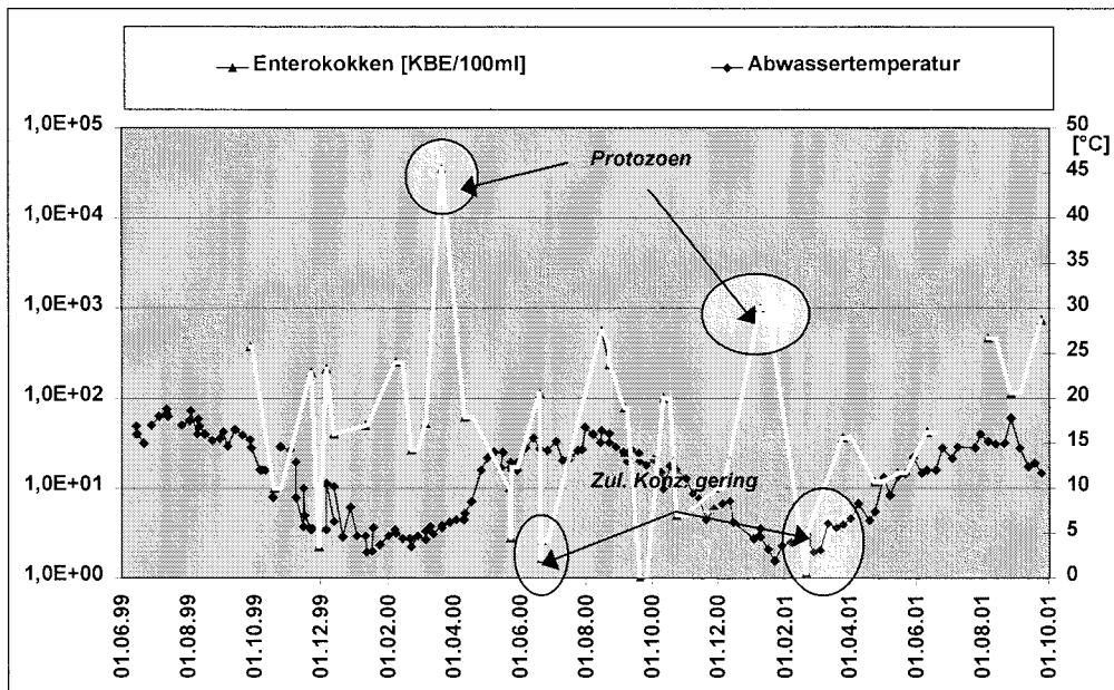
Anhang 4, Abb. 5.1.15: Elimination von Enterokokken im Vergleich zur Abwassertemperatur, Vertikalfilter, Anlage Wiedersberg
