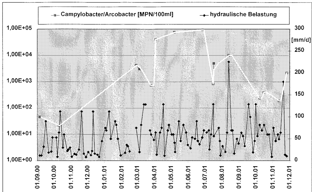
Anhang 4, Abb. 5.4.17: Elimination von Campylobacter/Arcobacter im Vergleich zur hydraulischen Belastung, Horizontalfilter 1, Anlage See
