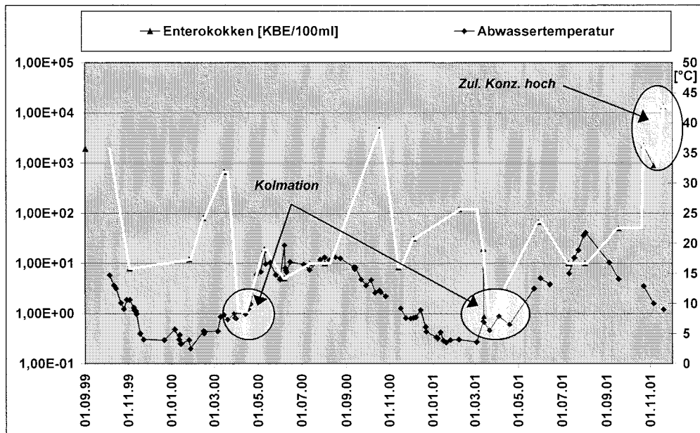
Anhang 4, Abb. 5.3.20: Elimination von Enterokokken im Vergleich zur Abwassertemperatur, Vertikalfilter 2, Anlage Ettenbüttel
