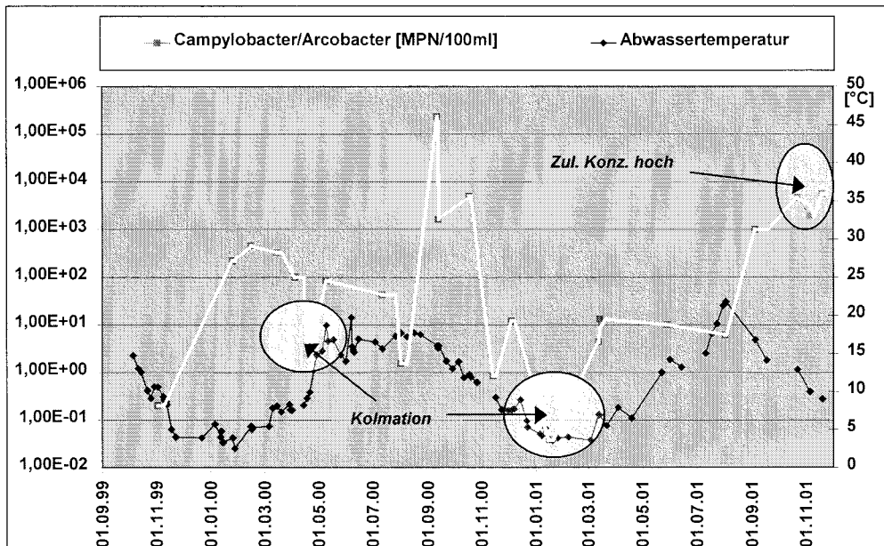
Abb. 5.3.12: Elimination von Campylobacter/Arcobacter im Vergleich zur Abwassertemperatur, Vertikalfilter 2 Anlage Ettenbüttel
