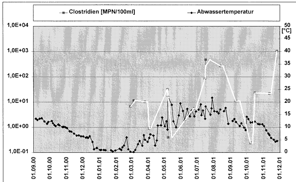
Anhang 4, Abb. 5.4.15: Elimination von Clostridien im Vergleich zur Abwassertemperatur, Horizontalfilter 1, Anlage See
