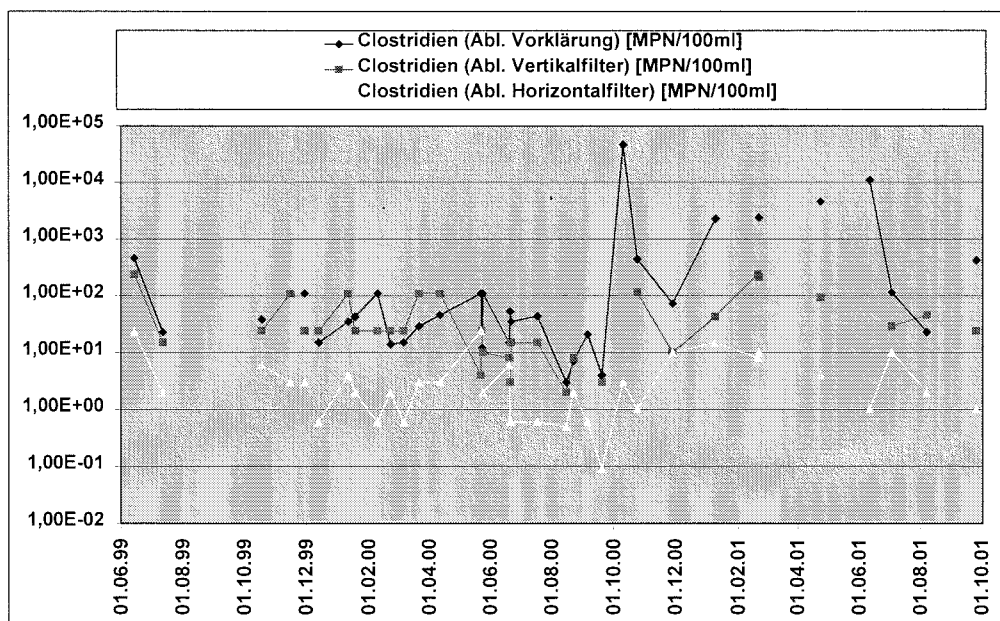
Abb. 5.2.9: Konzentrationen von Clostridien in Abläufen Vorklärung, Vertikal- und Horizontalfilter, Anlage Wiedersberg
