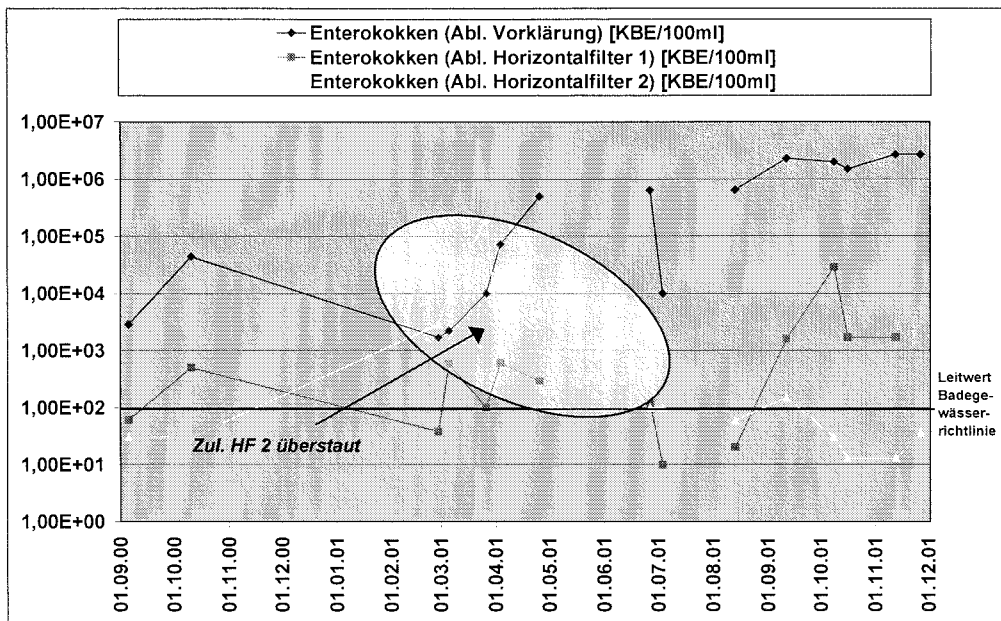
Anhang 4, Abb. 5.4.11: Konzentration von Enterokokken in Abläufen der Vorklärung, Horizontalfilter 1 und Horizontalfilter 2, Anlage See
