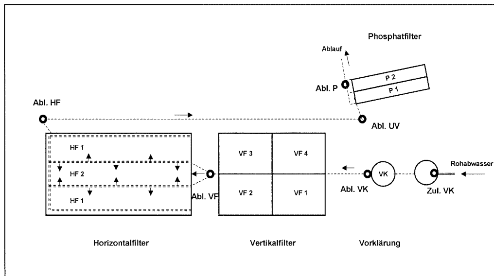
Abb. 4.1: Lageplan Anlage Wiedersberg mit Probenahmestellen
