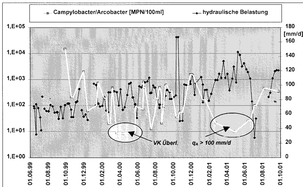
Abb. 5.2.12: Elimination von Campylobacter / Arcobacter im Vergleich zur hydraulischen Belastung, Vertikalfilter Anlage Wiedersberg
