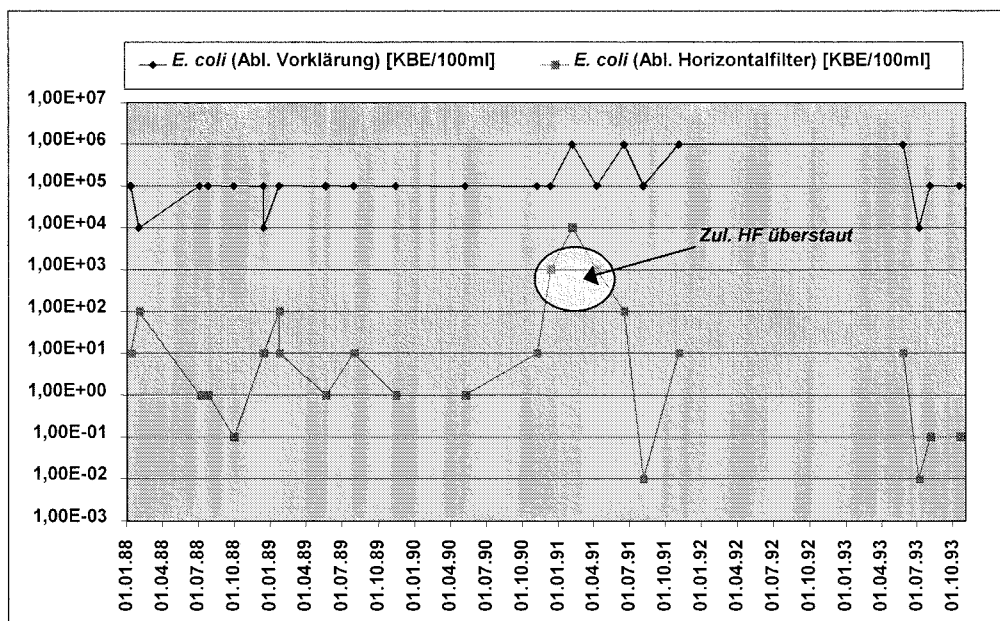
Abb. 5.4.1: Konzentrationen von E. coli in Abläufen Vorklärung und Horizontalfilter 2, Anlage See (Altdaten)
