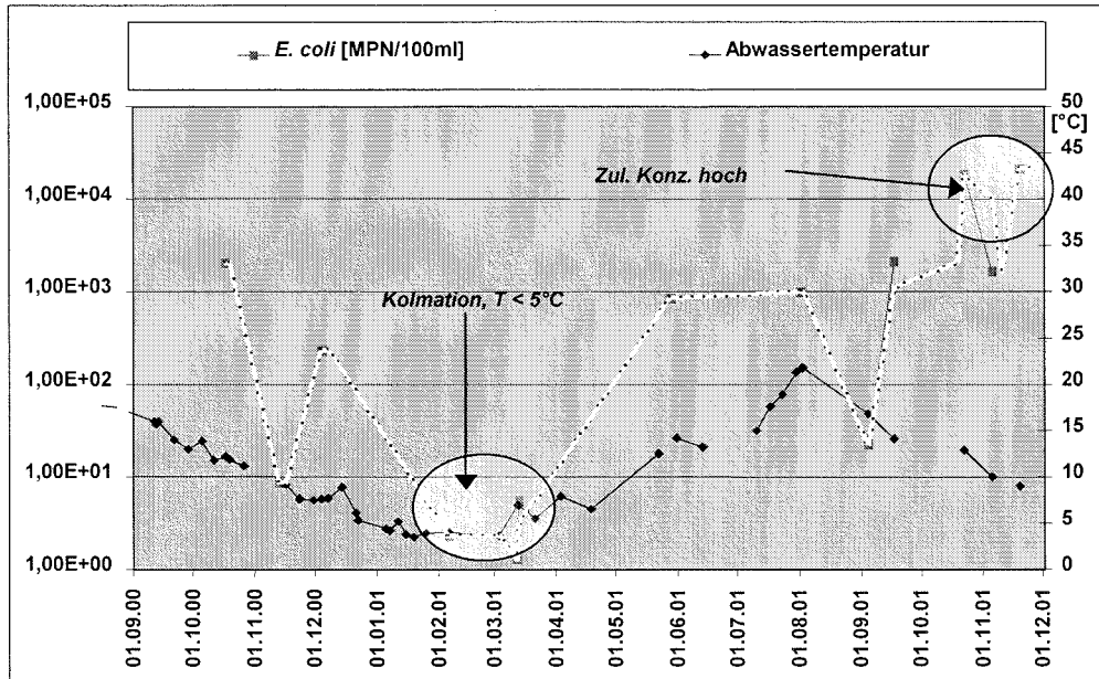
Abb. 5.3.8: Elimination von E.coli im Vergleich zur Abwassertemperatur, Vertikalfilter 1 Anlage Ettenbüttel
