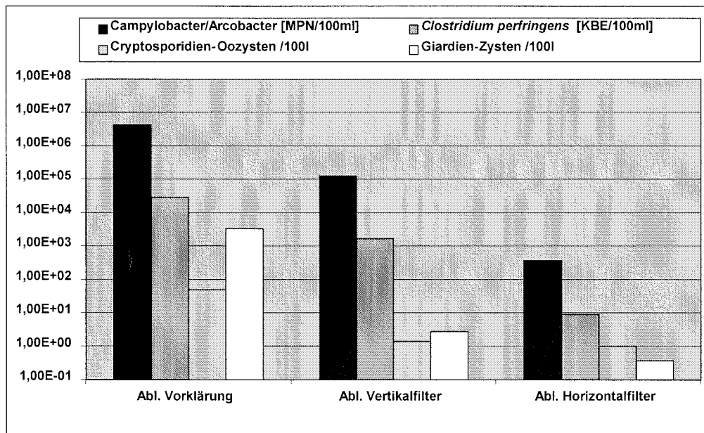
Abb. 5.2.2: Mikrobiologische Untersuchungen Anlage Wiedersberg, pathogene Mikroorganismen (Mittelwerte)
