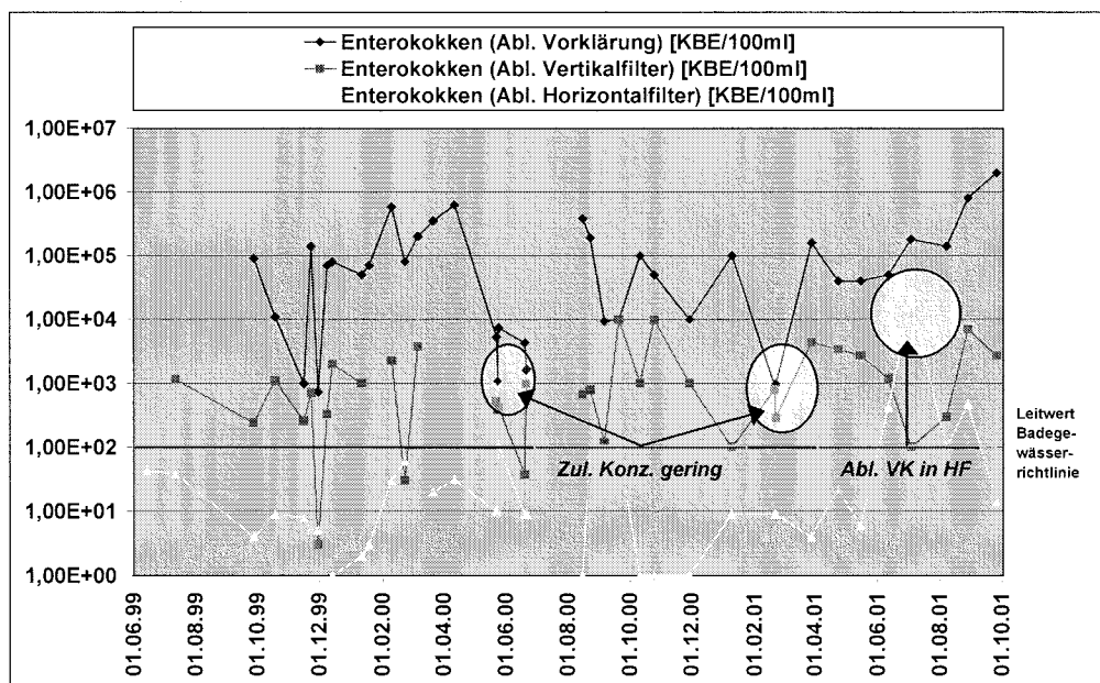
Abb. 5.2.4: Konzentrationen von Enterokokken in Abläufen Vorklärung, Vertikal- und Horizontalfilter, Anlage Wiedersberg
