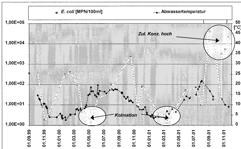
Abb. 5.3.11: Elimination von E. coli im Vergleich zur Abwassertemperatur, Vertikalfilter 2 Anlage Ettenbüttel
