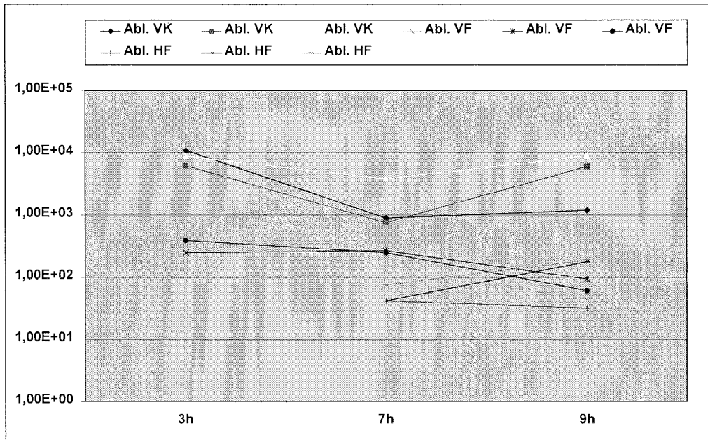
Abb. 5.1.1: Konzentrationen von Enterokokken in Abhängigkeit von der Standzeit (3 - 9 h), Anlage Wiedersberg
