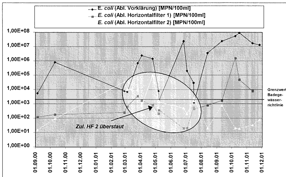
Abb. 5.4.6: Konzentrationen von E. coli in Abläufen Vorklärung, Horizontalfilter 1 und Horizontalfilter 2, Anlage See
