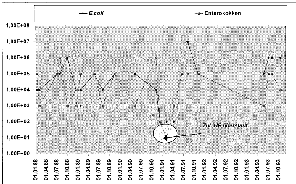
Abb. 5.4.3: Elimination von E. coli und Enterokokken Horizontalfilter 2, Anlage See (Altdaten)
