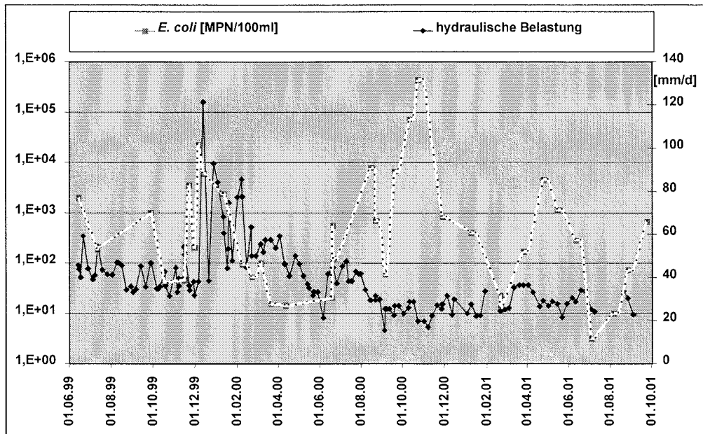
Anhang 4, Abb. 5.2.21: Elimination von E. coli im Vergleich zur hydraulischen Belastung, Horizontalfilter, Anlage Wiedersberg
