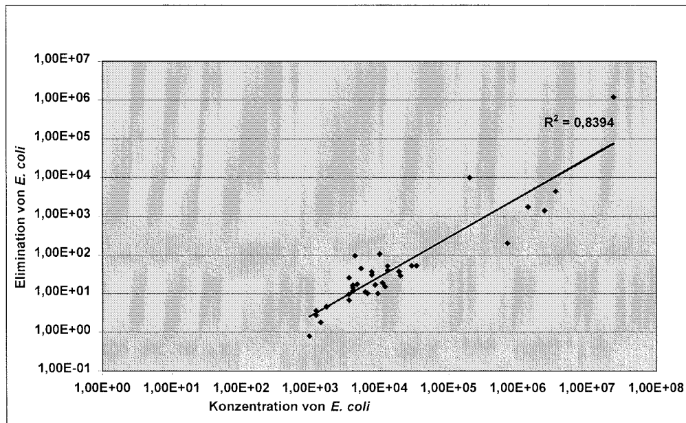
Abb. 5.4.7: Elimination von E. coli im Vergleich zur Zulaufkonzentration, Horizontalfilter 1 Anlage See
