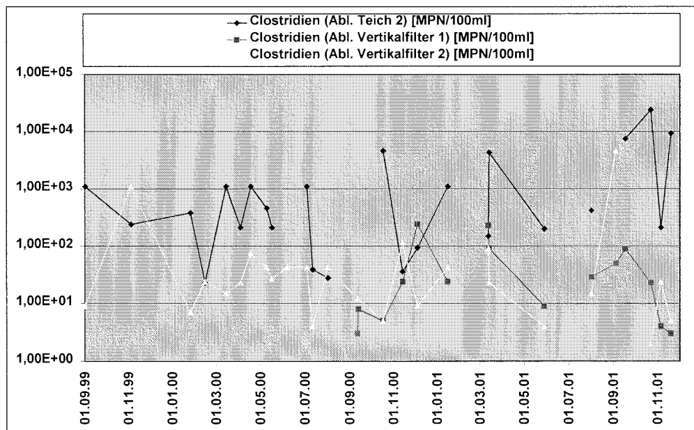
Anhang 4, Abb. 5.3.15: Konzentrationen von Clostridien in Abläufen Vorklä rung, Vertikalfilter 1 und Vertikalfilter 2, Anlage Ettenbüttel
