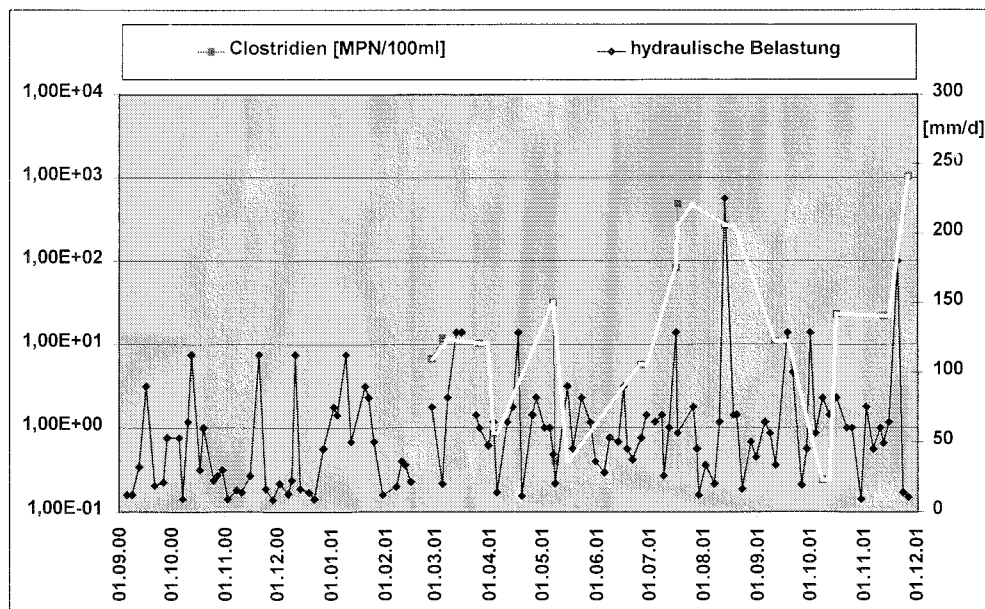
Anhang 4, Abb. 5.4.18: Elimination von Clostridien im Vergleich zur hydraulischen Belastung, Horizontalfilter 1, Anlage See
