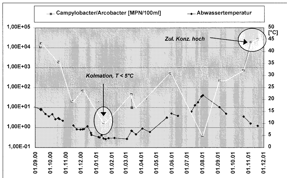
Abb. 5.3.9: Elimination von Campylobacter/Arcobacter im Vergleich zur Abwassertemperatur, Vertikalfilter 1 Anlage Ettenbüttel
