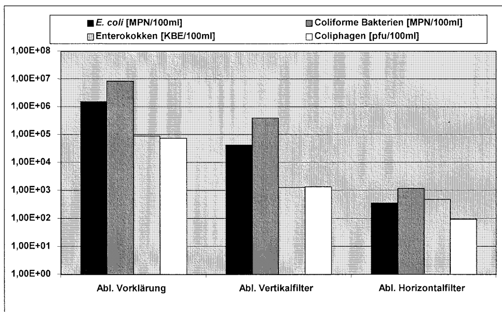
Abb. 5.2.1: Mikrobiologische Untersuchungsergebnisse Indikatororganismen (Mittelwerte), Anlage Wiedersberg
