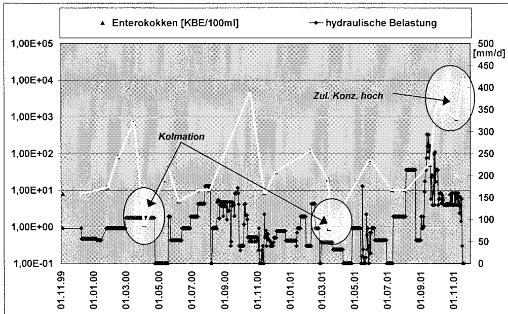
Abb. 5.3.13: Elimination von Enterokokken im Vergleich zur hydraulischen Belastung, Vertikalfilter 2 Anlage Ettenbüttel
