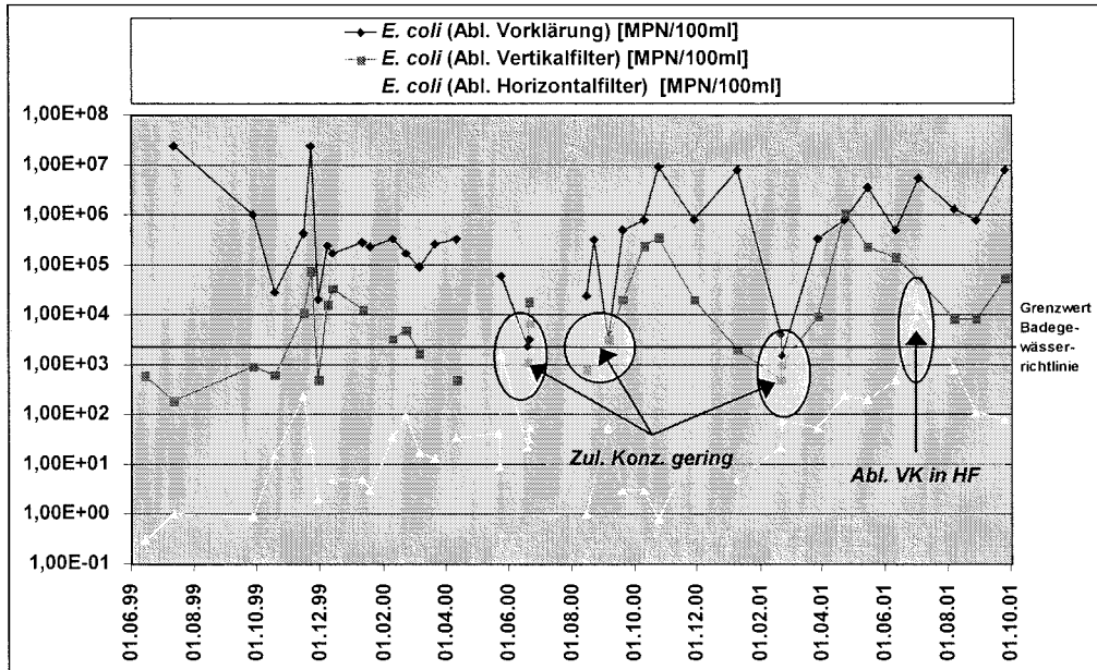
Abb. 5.2.3: Konzentrationen von E. coli in Abläufen Vorklärung, Vertikal- und Horizontalfilter, Anlage Wiedersberg
