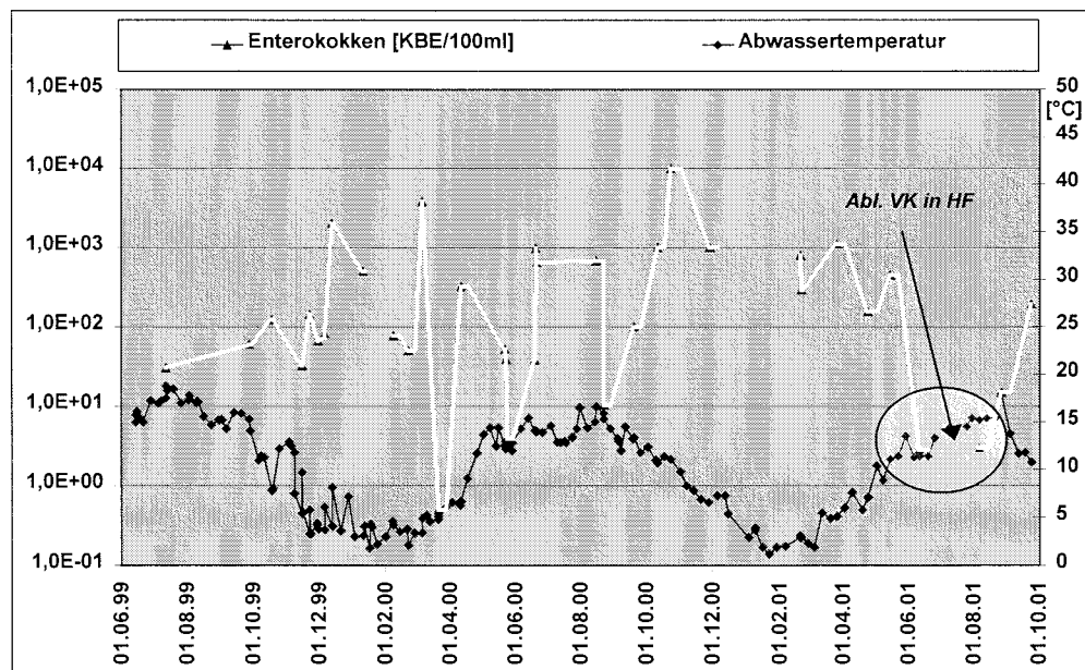
Anhang 4, Abb. 5.2.20: Elimination von Enterokokken im Vergleich zur Abwassertemperatur, Horizontalfilter, Anlage Wiedersberg
