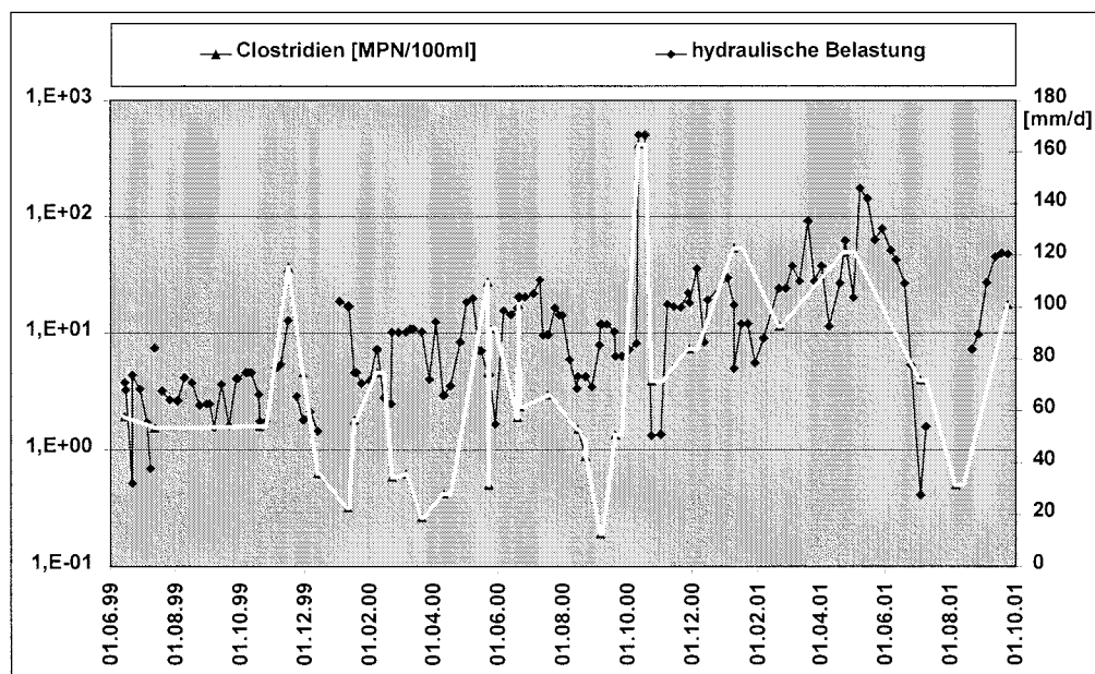
Anhang 4, Abb. 5.2.18: Elimination von Clostridien im Vergleich zur hydraulischen Belastung, Vertikalfilter, Anlage Wiedersberg
