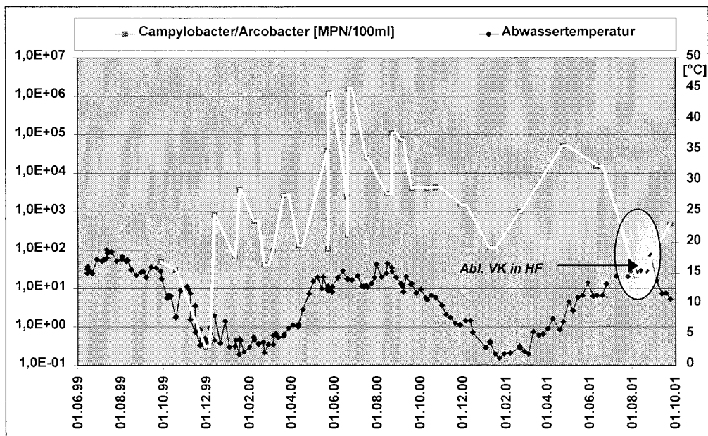
Abb. 5.2.13: Elimination von Campylobacter/Arcobacter im Vergleich zur Abwassertemperatur, Horizontalfilter Anlage Wiedersberg
