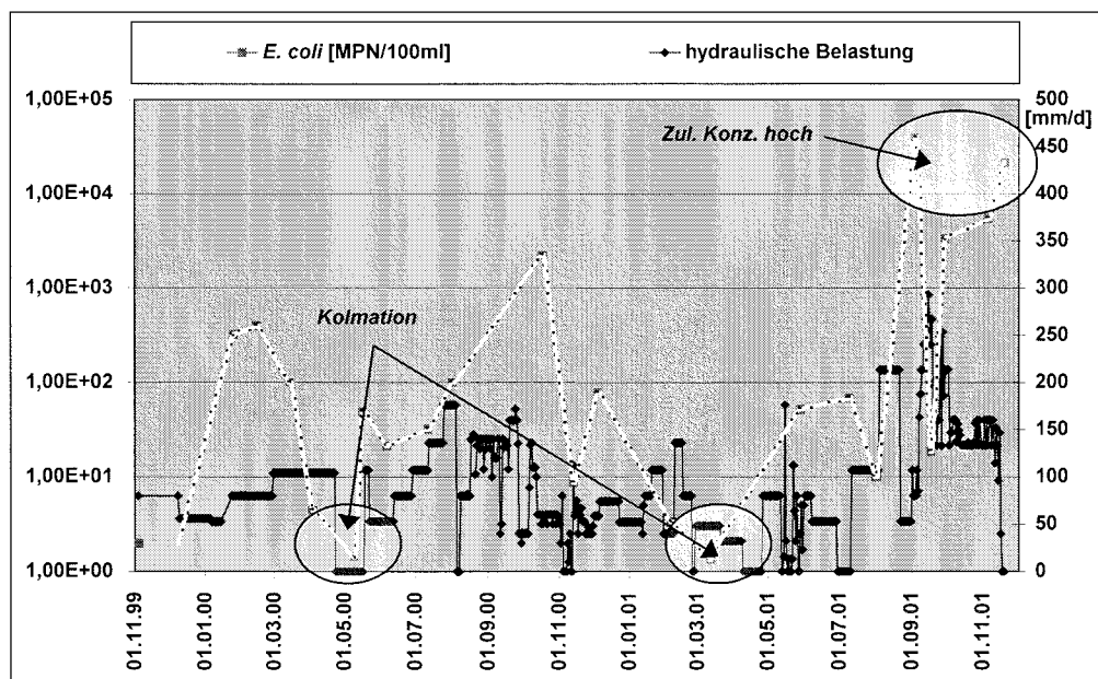
Anhang 4, Abb. 5.3.21: Elimination von E. coli im Vergleich zur hydraulischen Belastung, Vertikalfilter 2, Anlage Ettenbüttel
