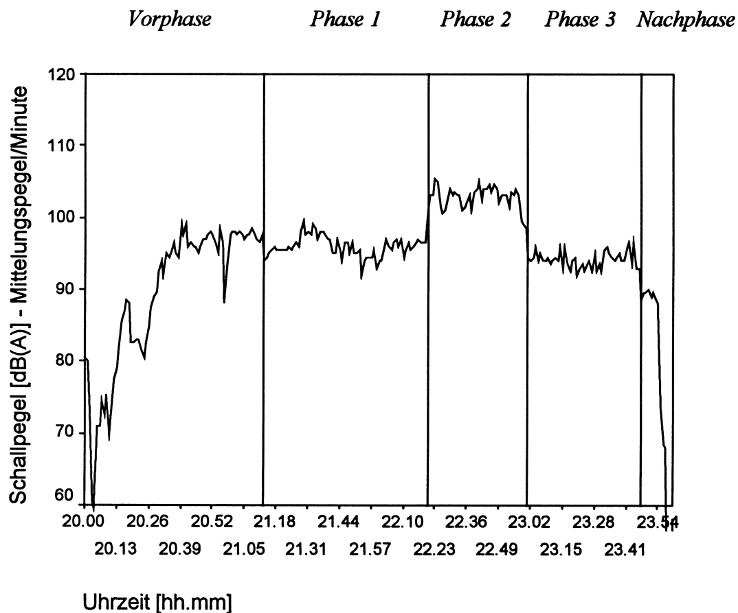
Abb. 3-1: Zeitverlauf des Musikschallpegels in der Diskothek (Tanzfläche)
