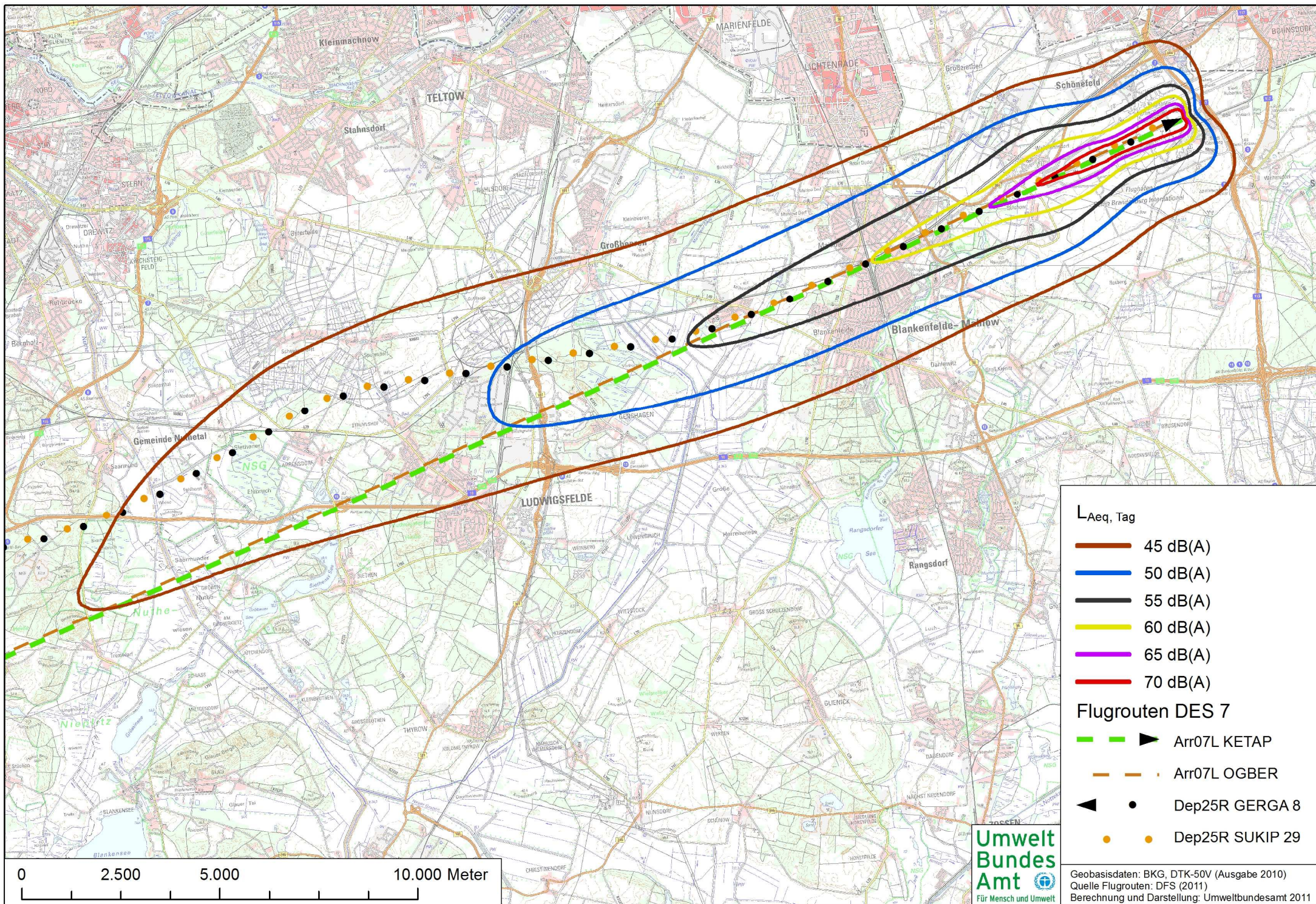
Abb. 19: Lärmkonturen bei Verlegung der Wannseerouten auf die Umgehungsroutes;
