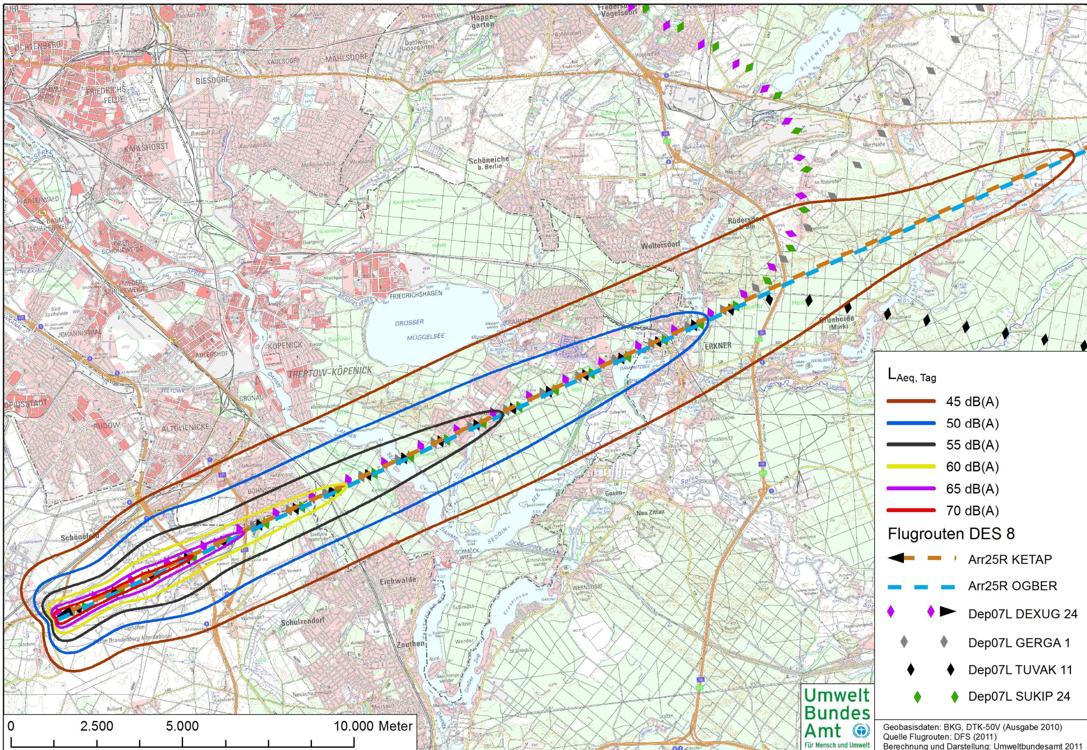
Abb. 15: Lärmkonturen bei Verlegung der Müggelseerouten auf die Umgehungsrouen; Tag
