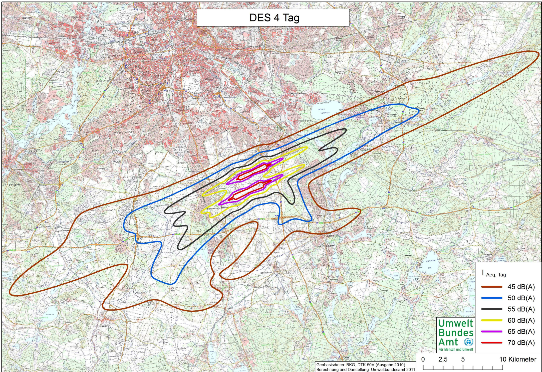
Abb. 25: Lärmkonturen einer alternativen Routenführung (ohne Müggelseeüberflug), DES 4; Tag
