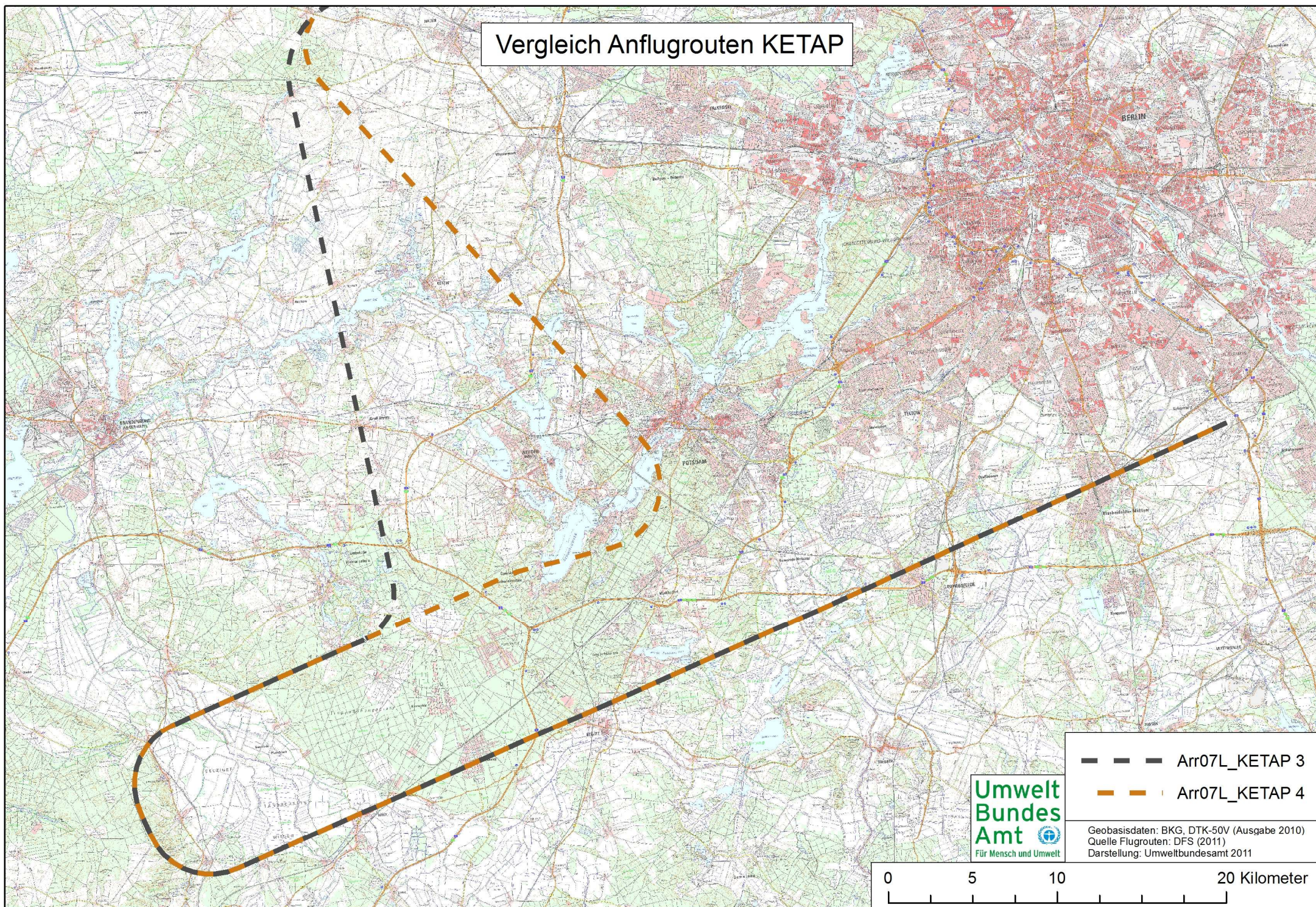
Abb. 10: Verläufe der Flugrouten KETAP 3 und KETAP 4
