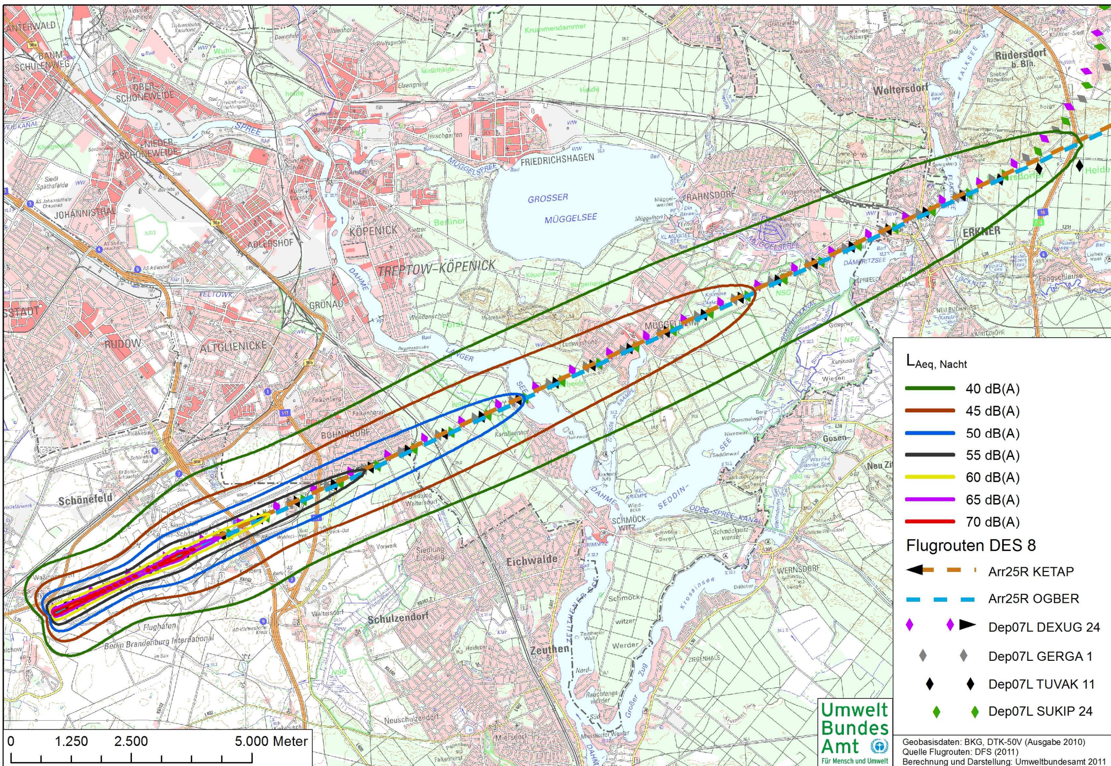
Abb. 17: Lärmkonturen bei Verlegung der Müggelseerouten auf die Umgehungsroute; Nacht
