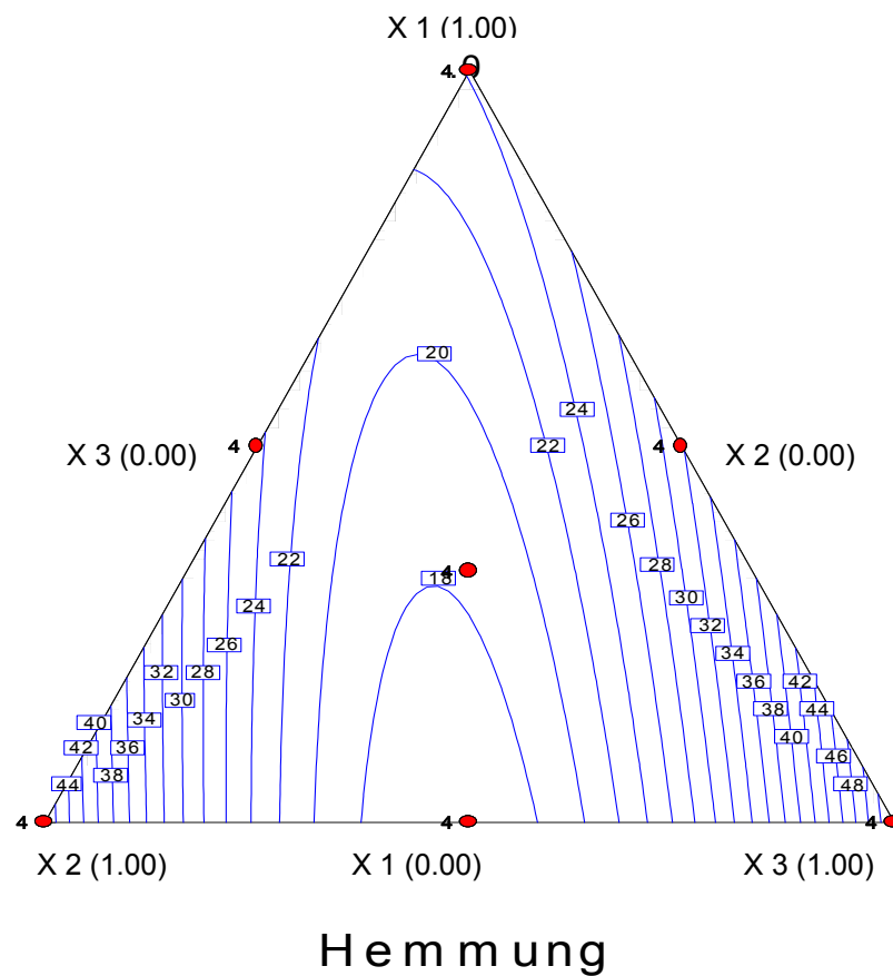
Abbildung 1b: Simplex-Effektfläche (quadratisches Polynom) für das Gemisch aus PMBS, Hexanol und Hexachlorophen in der 2-D-Darstellung. Die „Höhenlinien“ sind die errechneten Verläufe der Vermehrungshemmung. Die Zahlen in den Kästchen geben den jeweiligen %-Wert der Hemmung an
