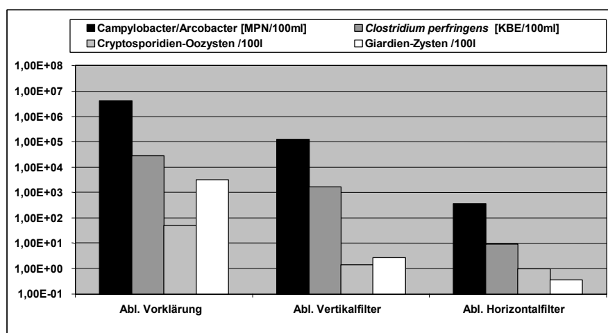
Abbildung 2: Anlage Wiedersberg: Konzentrationen von pathogenen Mikroorganismen (Mittelwerte) nach verschiedenen Behandlungsstufen (auf der Abszisse sind die \log_{10} -Stufen aufgetragen)
