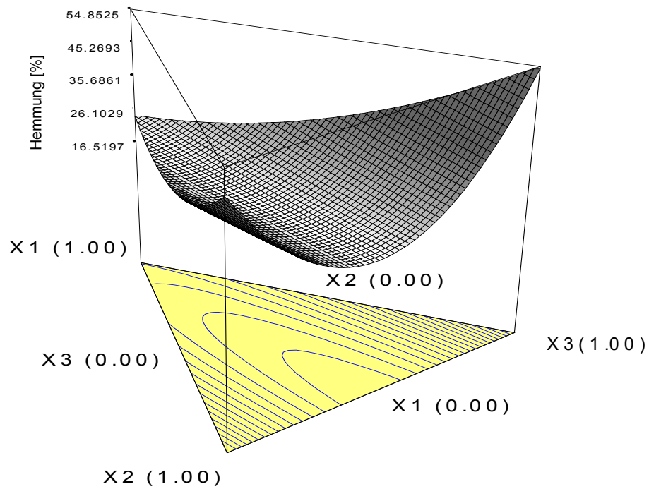
Abbildung 1a: Simplex-Effektfläche (quadratisches Polynom) für das Gemisch aus PMBS, Hexanol und Hexachlorophen in der 3-D-Darstellung
