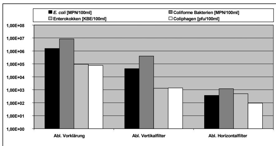
Abbildung 1: Anlage Wiedersberg: Konzentrationen von Indikatororganismen (Mittelwerte) nach verschiedenen Behandlungsstufen (auf der Abszisse sind die \log_{10} -Stufen aufgetragen)
