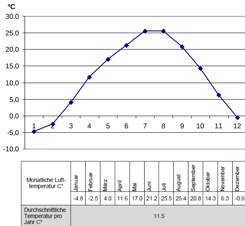
Abb. 3.13: Kurve der monatlichen Lufttemperatur in der Stadt Echmiadzin und im Dorf Mkhchyan
