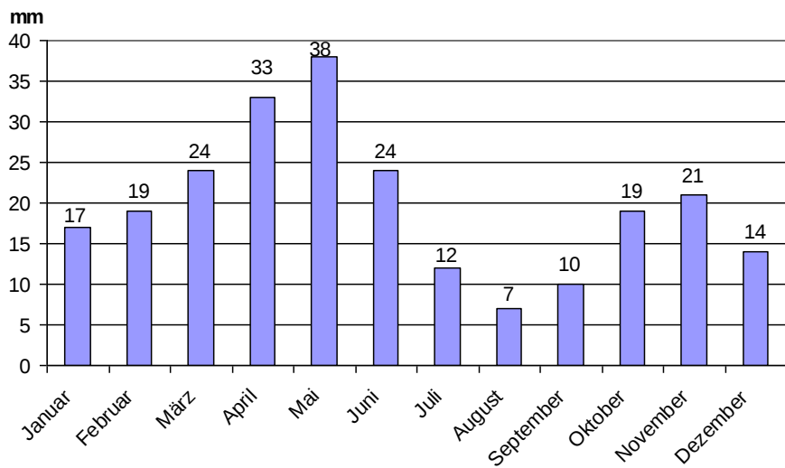
Abb. 3.8: Niederschlagsschwankungen in Talin
