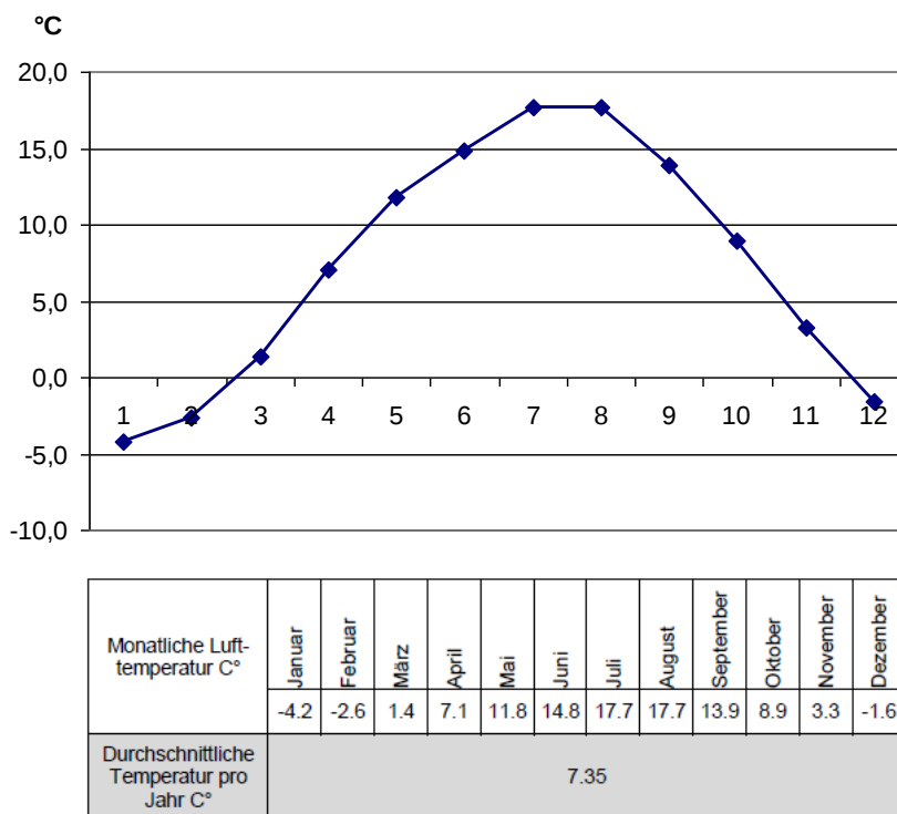
Abb. 3.14: Kurve der monatlichen Lufttemperatur in der Stadt Vanadzor
