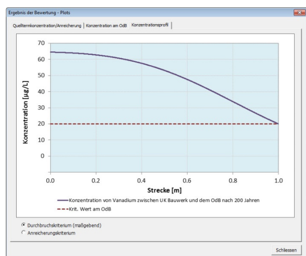
Abbildung 4-6: Ergebnisgrafiken nach einer individuellen Bewertung unter Berücksichtigung einer einzelnen materialrelevanten Stoffkomponente (Vanadium) eines MEB (RC-2): Konzentrationsdurchbruchskurve am OdB (links oben), Konzentrationsprofil entlang der Sickerstrecke (rechts oben) sowie Entwicklung der Konzentration im Quellterm und der Stoffanreicherung (links unten), jeweils für die maximal zulässige Quelltermkonzentration in der Bauweise B5 bei sandigem Unterboden für das maßgebende Durchbruchskriterium.
