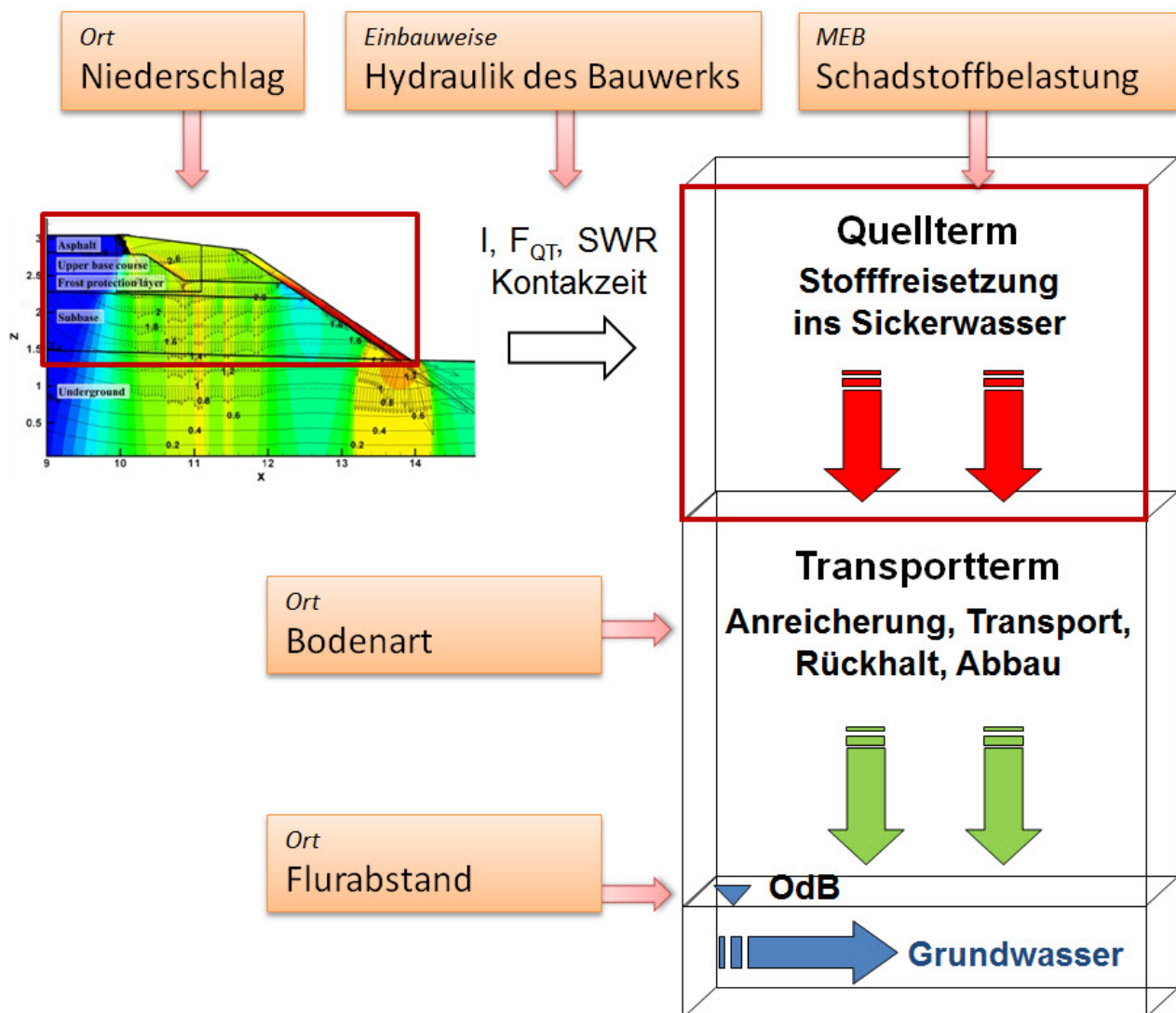
Abbildung 4-10: Schematische Darstellung der Einflussgrößen bei der Ableitung von medianschutzbasierten Einbauwerten.
