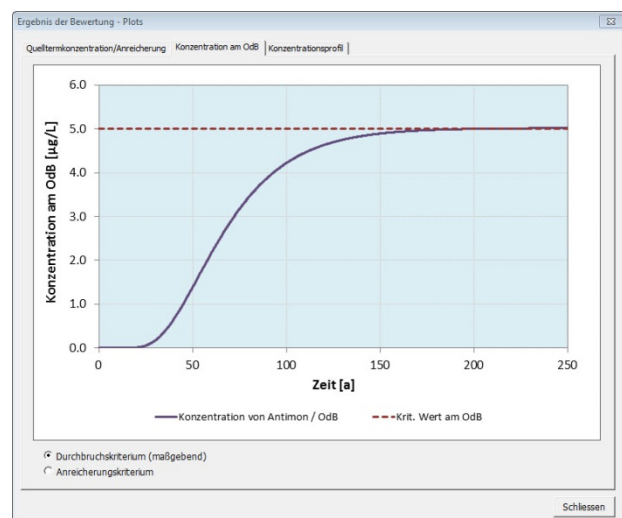
Abbildung 4-12: Ergebnisplots der individuellen Bewertung für Antimon in CUM-1 in der Einbauweise 14a für einen Quellterm mit konstanter Stofffreisetzung: Entwicklung der Konzentration im Quellterm und der Stoffanreicherung (links) und Konzentrationsdurchbruchskurve am OdB (rechts).
