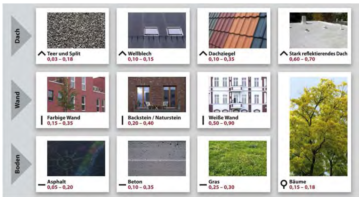
Abb. 7.04: Albedowerte verschiedener Oberflächen (SENATSVRWALTUNG FÜR STADTENTWICKLUNG [Hrsg.] 2011)
