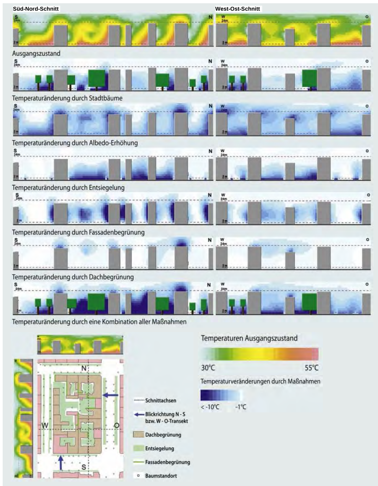
Abb. 7.05: Temperaturverteilung und -änderung durch bauliche Maßnahmen zum Zeitpunkt 12 Uhr Mittags für einen beispielhaften Baublock (GEO-NET 2010, veröffentlicht in SENATSVORWORT FÜR STADTENTWICKLUNG [Hrsg.] 2011)
