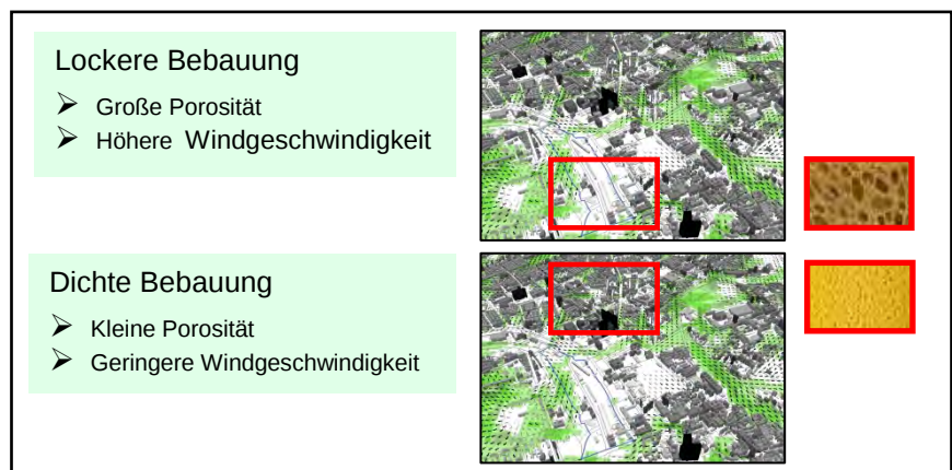
Abb. 4.02: Einfluss der Bebauungsdichte auf die Strömungsgeschwindigkeit
