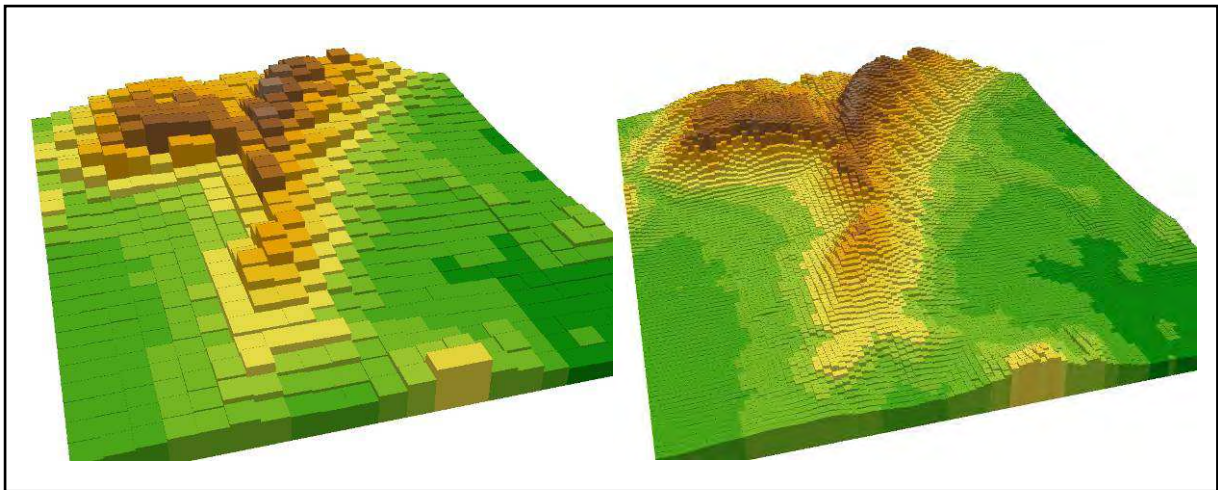
Abb. 4.01: Unterschiedliche Rasterweiten (links: 500 m x 500 m; rechts: 100 m x 100 m) bei einem digitalem Geländehöhenmodell
