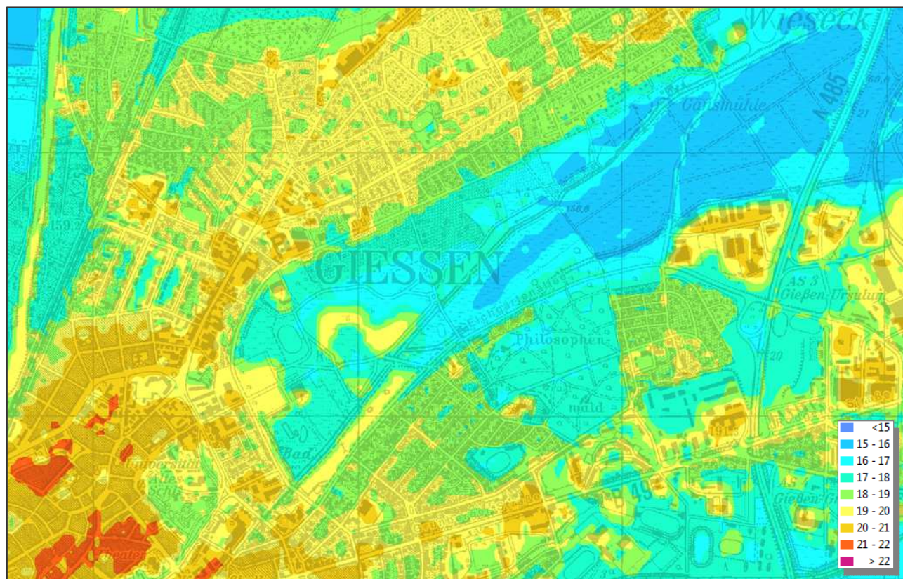
Abb. 5.02: Ausschnitt des Temperaturfeldes zum Zeitpunkt 4 Uhr morgens, unterlegt mit der Topographischen Stadtkarte (HLBG 2003)
