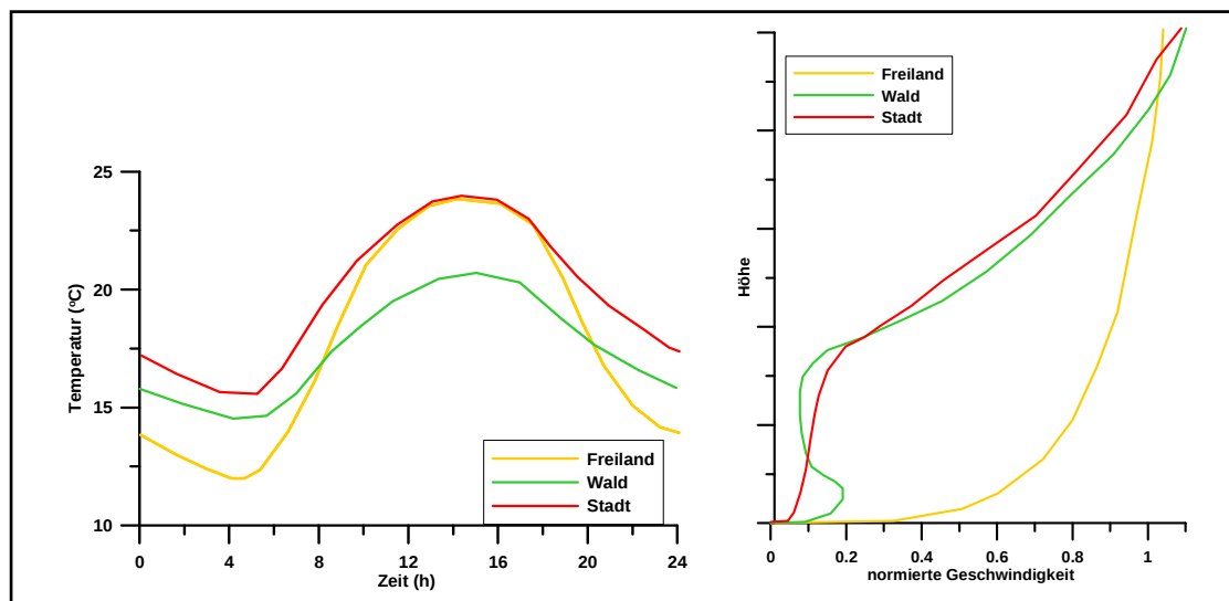
Abb. 4.05: Temperaturverlauf und Vertikalprofil der Windgeschwindigkeit zur Mittagszeit für verschiedene Landnutzungen
