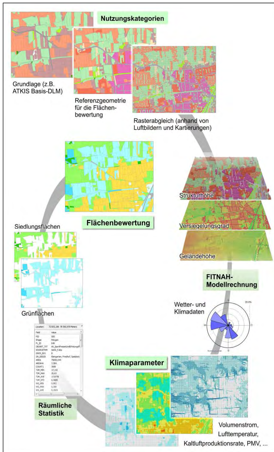
Abb. 4.11: Schematisierter Verfahrensablauf zur flächenhaften Bewertung der Referenzgeometrie
