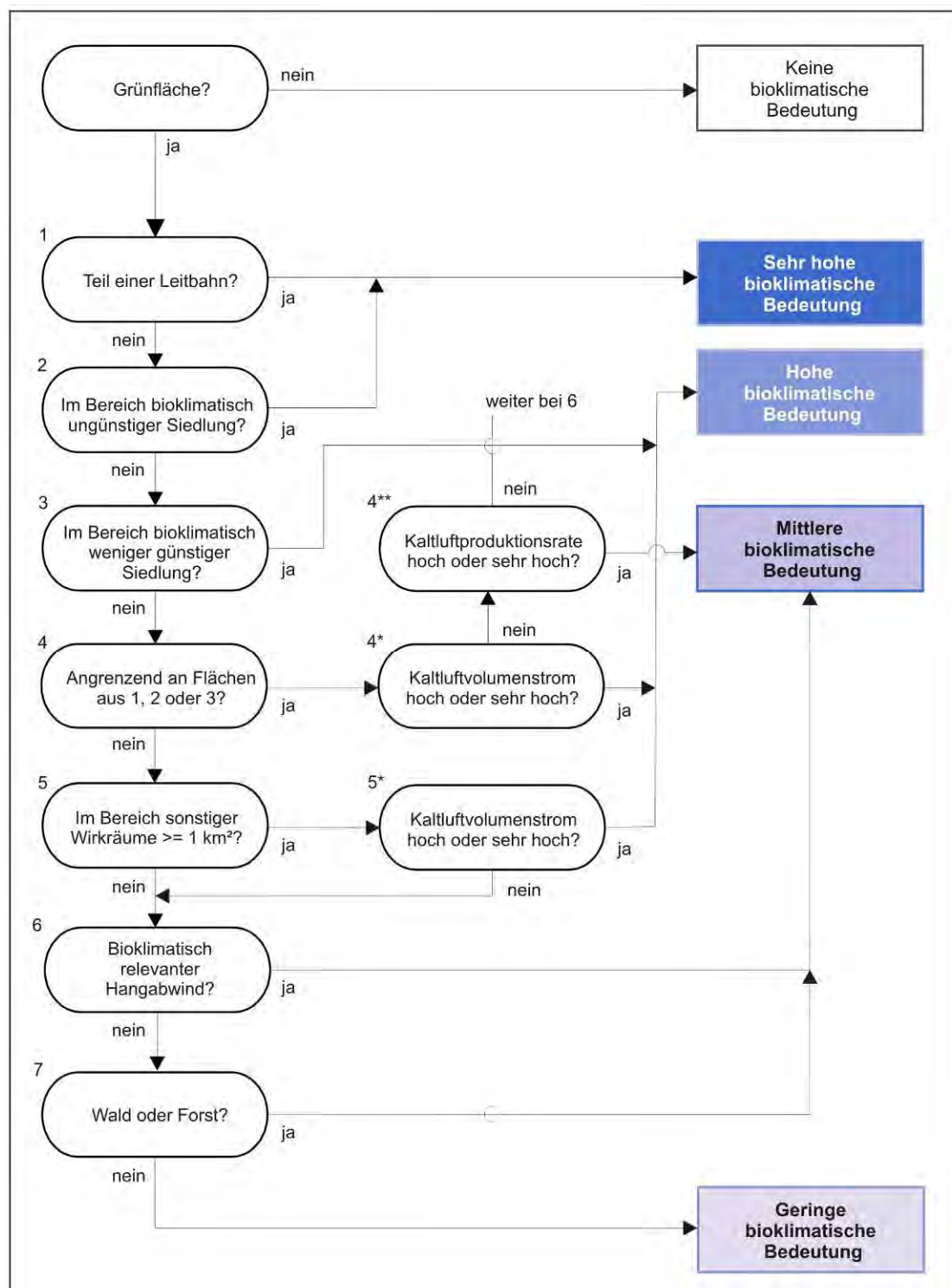
Abb. 4.12: Vereinfachtes Verknüpfungsmodell zur Ermittlung der bioklimatischen Bedeutung der Grünflächen
