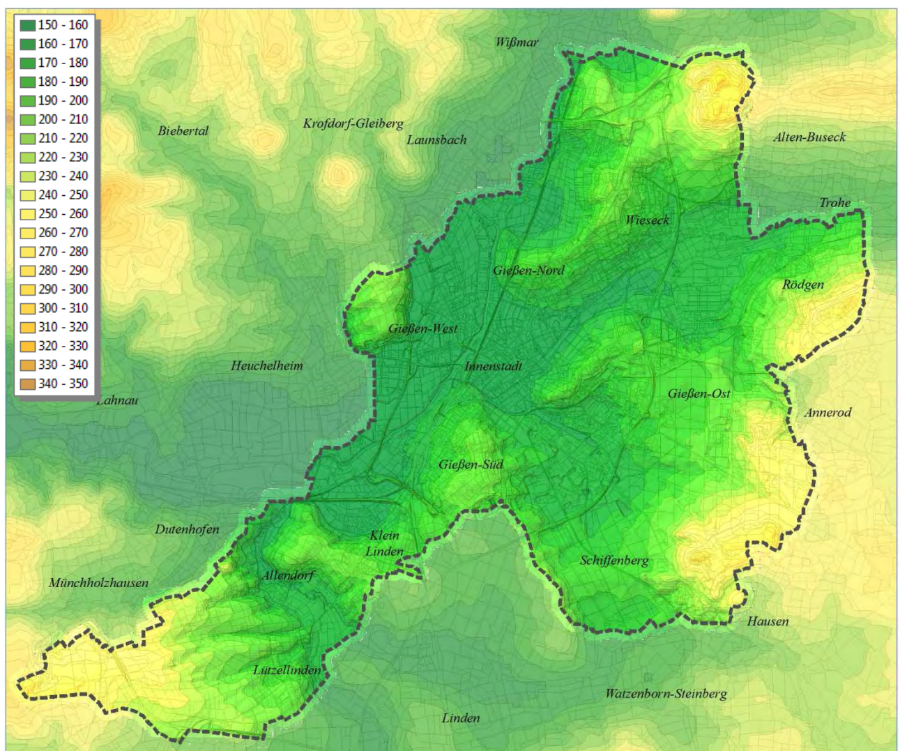
Abb. 3.01: Geländehöhe im Untersuchungsraum (in m ü. NN)
