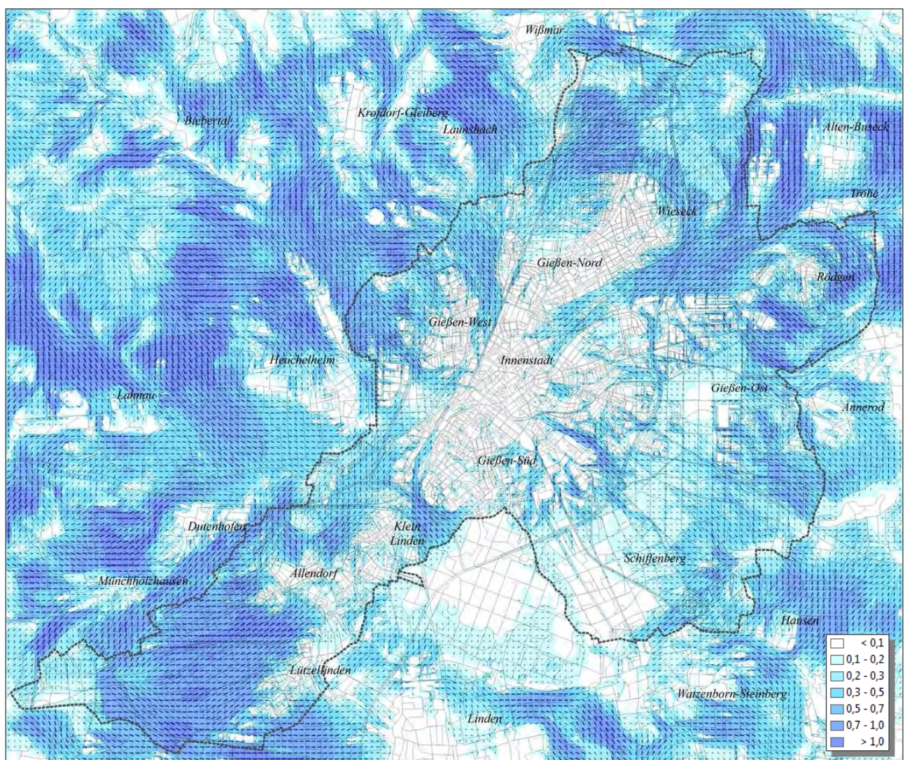
Abb. 5.05: Strömungsgeschwindigkeit (m/s) und Richtung zum Zeitpunkt 4 Uhr morgens (2 m ü. Grund). Die Vektoren sind auf eine Auflösung von 100 m aggregiert.
