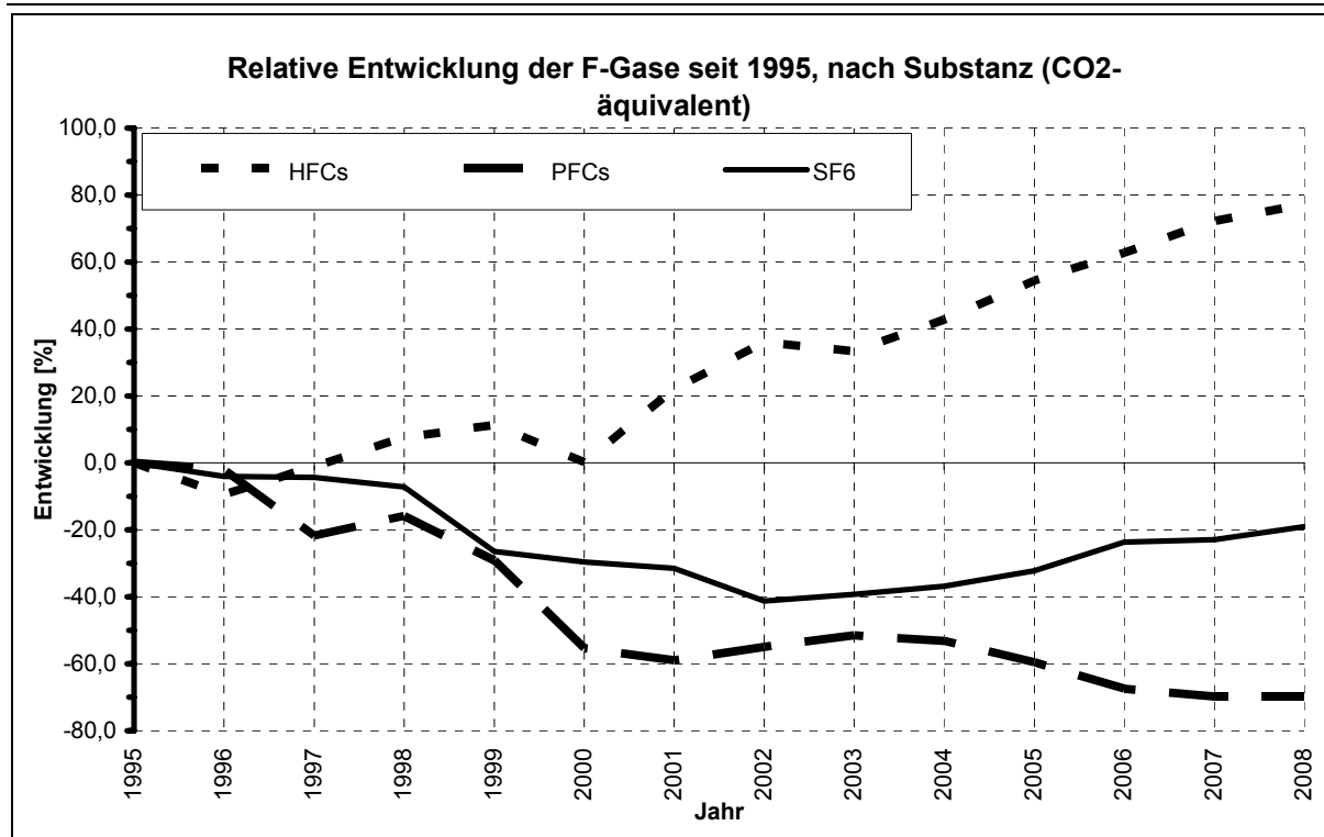
Abbildung 18: Relative Entwicklung der F-Gase gegenüber 1995
