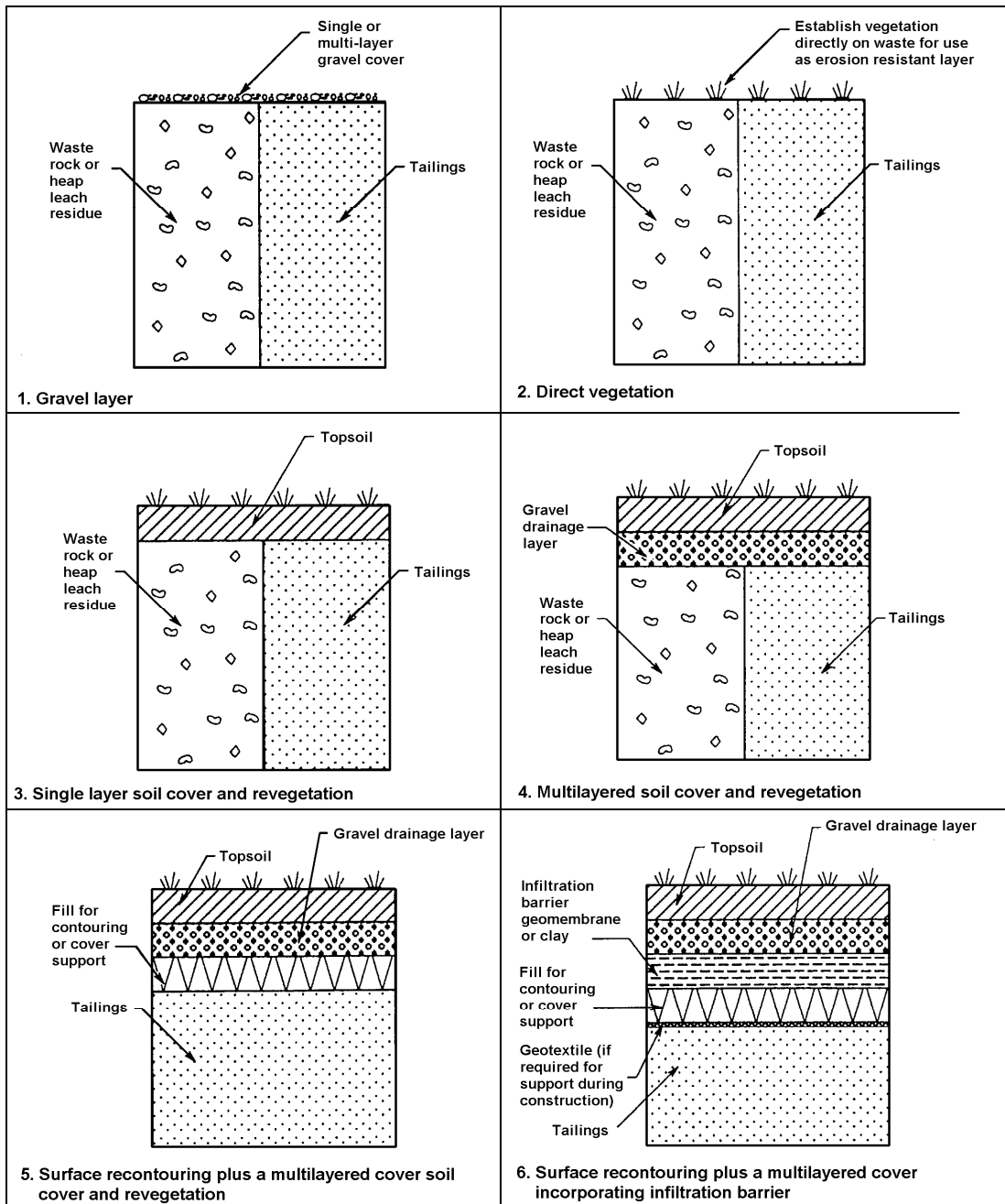
Abb. 4.4: Typische Abdeckungen von Bewirtschaftungsflächen von Aufbereitungsrückständen [11, EPA, 1995]
