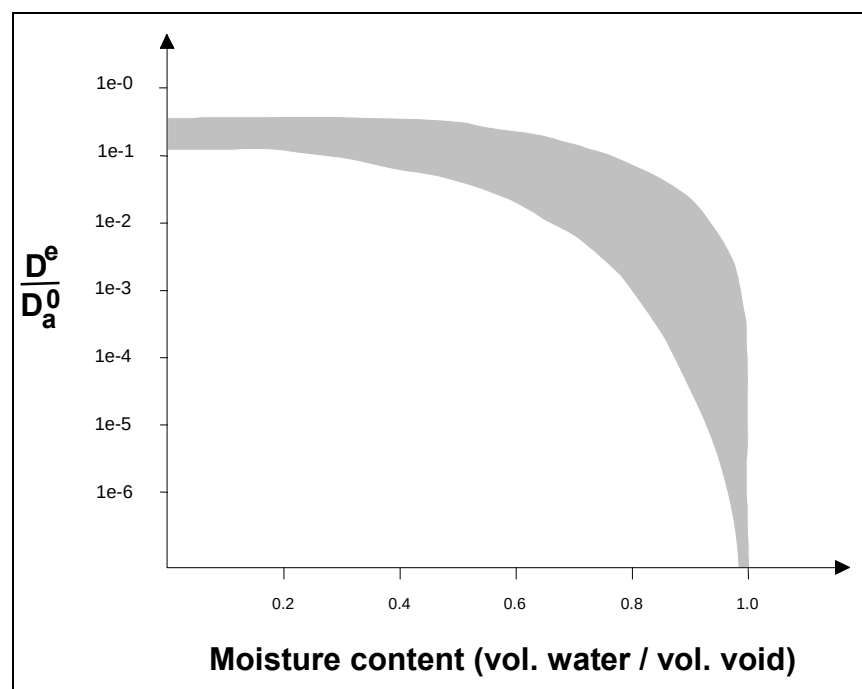
Abb. 4.6: Verhältnis zwischen dem effektiven Diffusionskoeffizienten in einem teilweise mit Wasser gesättigten poriger Stoff und Diffusion in Luft
