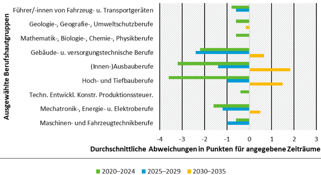
Abbildung 34: Veränderung des Fachkräfteindikators in Folge der erhöhten energetischen Sanierungsrate
