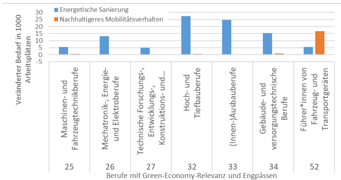
Abbildung 2: Stärkste Veränderung des Arbeitskräftebedarfs in den Szenarien „Energetische Sanierung“ und „Nachhaltigeres Mobilitätsverhalten“
