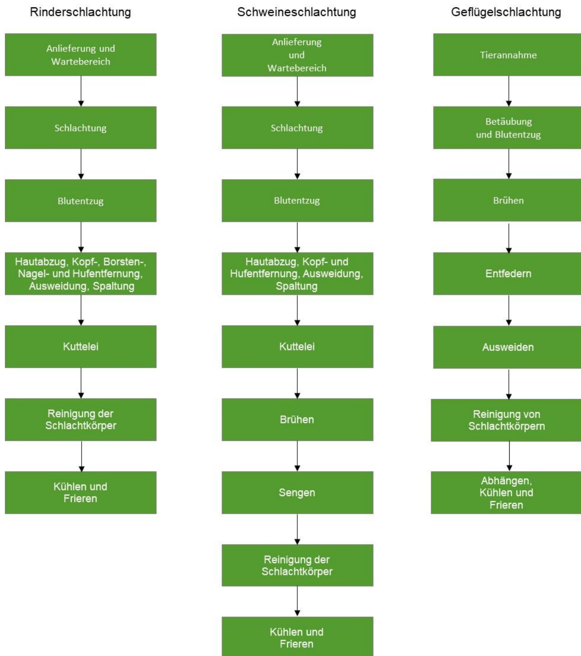
Abbildung 2: Emissionsrelevante Produktionsprozesse in Schlachthanlagen
