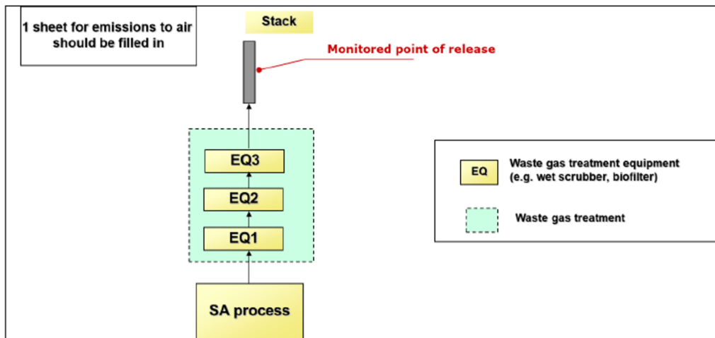
Abbildung 12: Schematische Darstellung der relevanten Messstellen für Emissionen in die Luft bei einer Messstelle (1) und bei zwei Messstellen (2)
