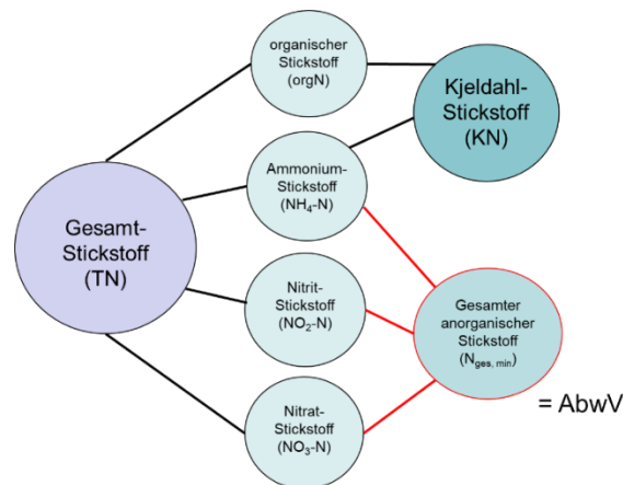
Abbildung 8: Aufteilung der verschiedenen Stickstoffkomponenten auf die Summenparameter TN, KN und N_{ges,min}
