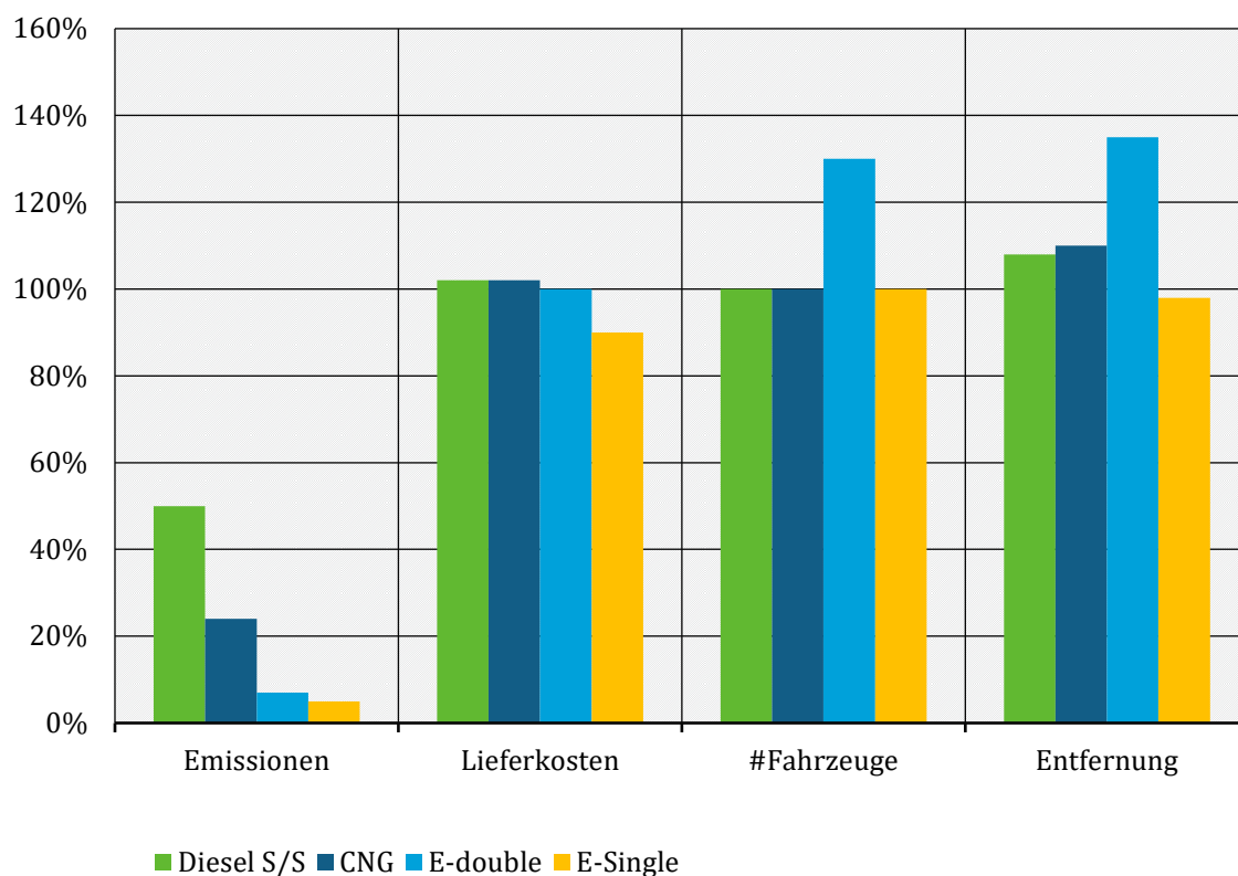
Abbildung 12: Vergleich verschiedener Antriebstechniken in Bezug auf ausgewählte KPIs
