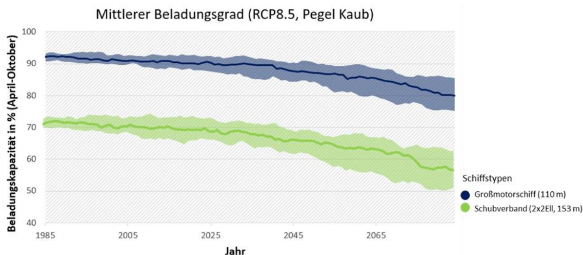
Abbildung 7: Potenzielle mittlere Beladungsgrade für häufige Schiffstypen für den Pegel Kaub während des hydrologischen Sommerhalbjahres für den Zeitraum 1985 bis 2085
