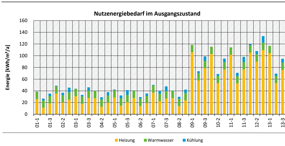
Abbildung 109: Nutzenergiebedarf der Wohnungen der Variante SQ2 (mit Gebäudekühlung) des Frankfurter Quartiers
