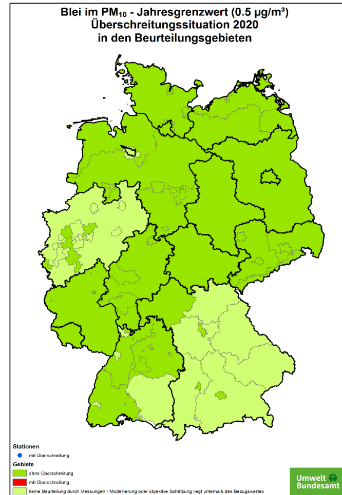
Abbildung 4: Gebietsbezogene Beurteilung für Blei in der PM 10 -Fraktion, Schutz der menschlichen Gesundheit
