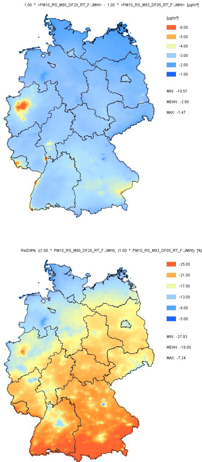
Abbildung 5-5 Absolute (oben, \mu\text{g}/\text{m}^3 ) und relative (unten, %) Änderung der PM10-Jahresmittelwerte als Folge der Emissionsentwicklung 2005 nach 2020. Verkehrsmodell TREMOD 5.04. MIN, MEAN und MAX geben den Konzentrationsänderungsbereich (MIN und MAX) sowie die mittlere Konzentrationsänderung (MEAN) über Deutschland an. Meteorologische Referenz ist 2005.
