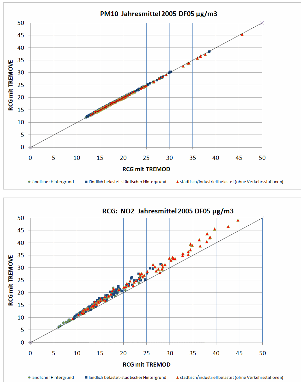
Abbildung 4-8 Vergleich der berechneten PM10- und NO 2 -Jahresmittelwerte 2005 mit Verkehrsemissionen nach TREMOD 4.17M und Verkehrsemissionen nach TREMOVE 2.7 an den für Abbildung 4-6 und Abbildung 4-7 verwendeten Stationen.
