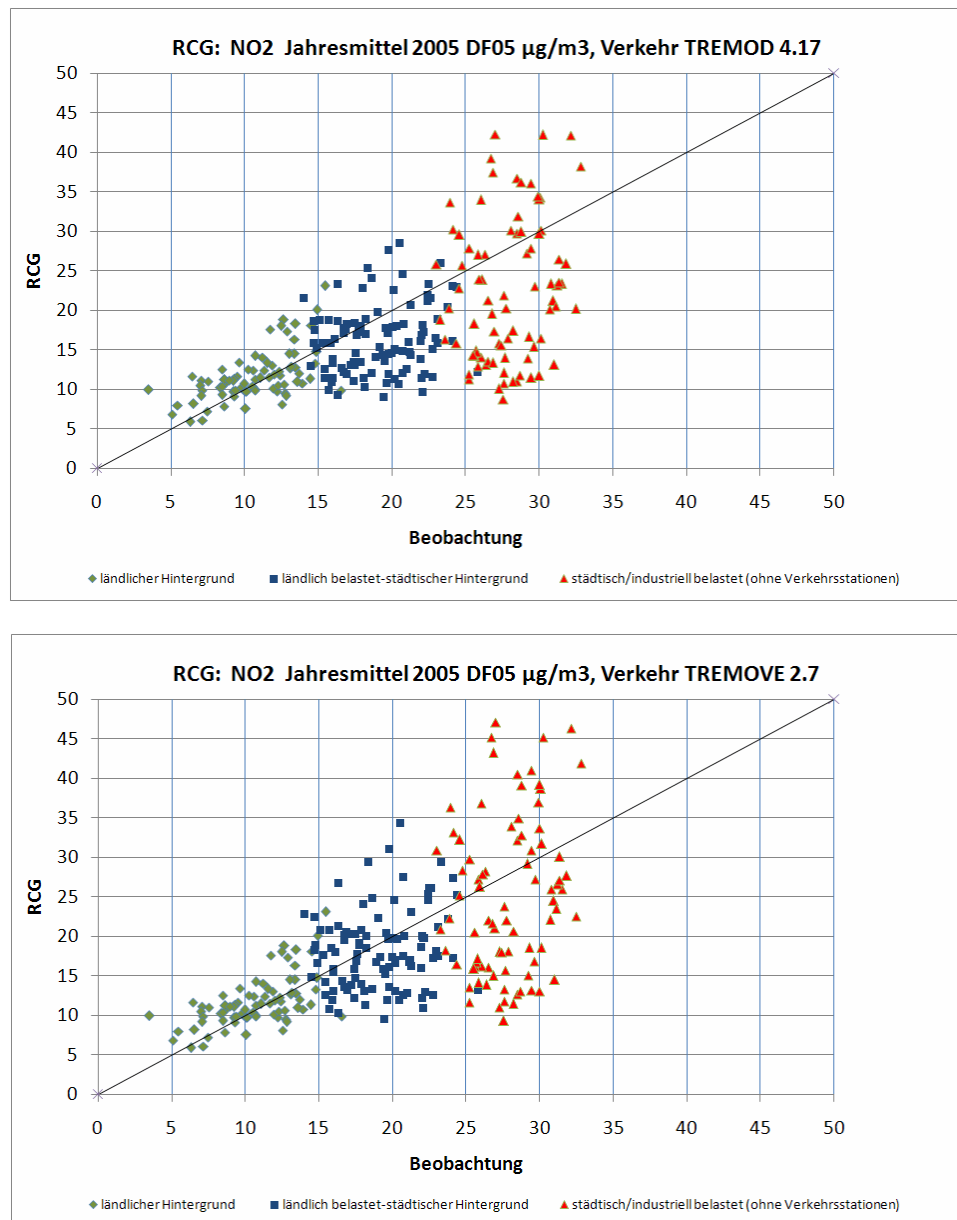
Abbildung 4-7 Vergleich der berechneten NO 2 -Jahresmittelwerte 2005 mit Beobachtungen. Oben: Verkehrsemissionen nach TREMOD 4.17M, unten Verkehrsemissionen nach TREMOVE 2.7.
