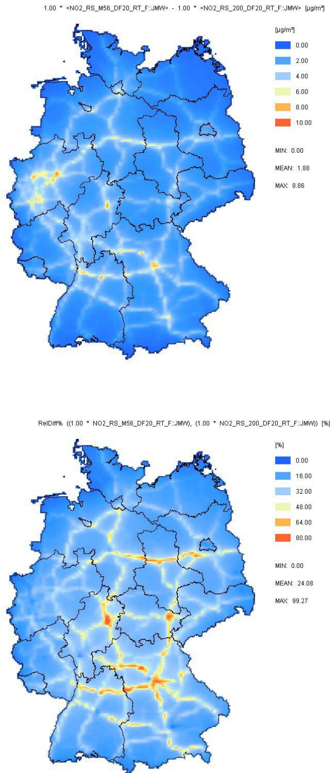
Abbildung 4-16 Absolute (oben, \mu\text{g}/\text{m}^3 ) und relative (unten, %) Änderung der \text{NO}_2 -Jahresmittelwerte 2020 als Folge des Austauschs der Verkehrsemissionen (TREMOD 4.17M durch TREMOVE 2.7 ersetzt). MIN, MEAN und MAX geben den Konzentrationsänderungsbereich (MIN und MAX) sowie die mittlere Konzentrationsänderung (MEAN) über Deutschland an. Meteorologische Referenz ist 2005.
