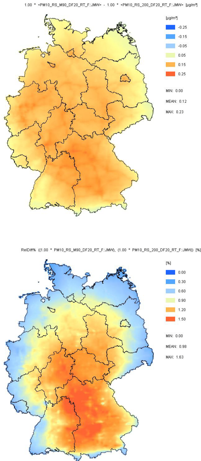
Abbildung 5-3 Absolute (oben, \mu\text{g}/\text{m}^3 ) und relative (unten, %) Änderung der PM10-Jahresmittelwerte 2020 als Folge des Austauschs der Verkehrsemissionen (TREMOD 4.17M durch TREMOD 5.04 ersetzt). MIN, MEAN und MAX geben den Konzentrationsänderungsbereich (MIN und MAX) sowie die mittlere Konzentrationsänderung (MEAN) über Deutschland an. Meteorologische Referenz ist 2005.
