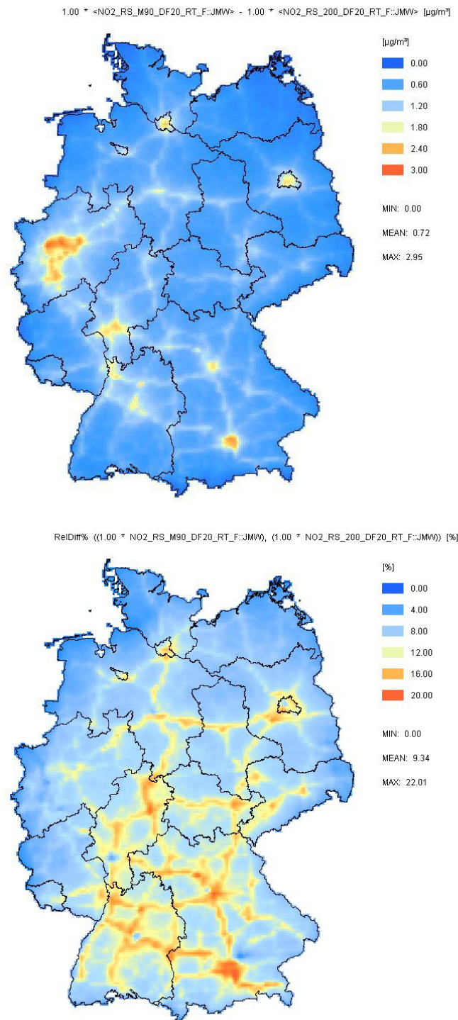
Abbildung 5-4 Absolute (oben, \mu\text{g}/\text{m}^3 ) und relative (unten, %) Änderung der \text{NO}_2 -Jahresmittelwerte 2020 als Folge des Austauschs der Verkehrsemissionen (TREMOD 4.17M durch TREMOD 5.04 ersetzt). MIN, MEAN und MAX geben den Konzentrationsänderungsbereich (MIN und MAX) sowie die mittlere Konzentrationsänderung (MEAN) über Deutschland an. Meteorologische Referenz ist 2005.
