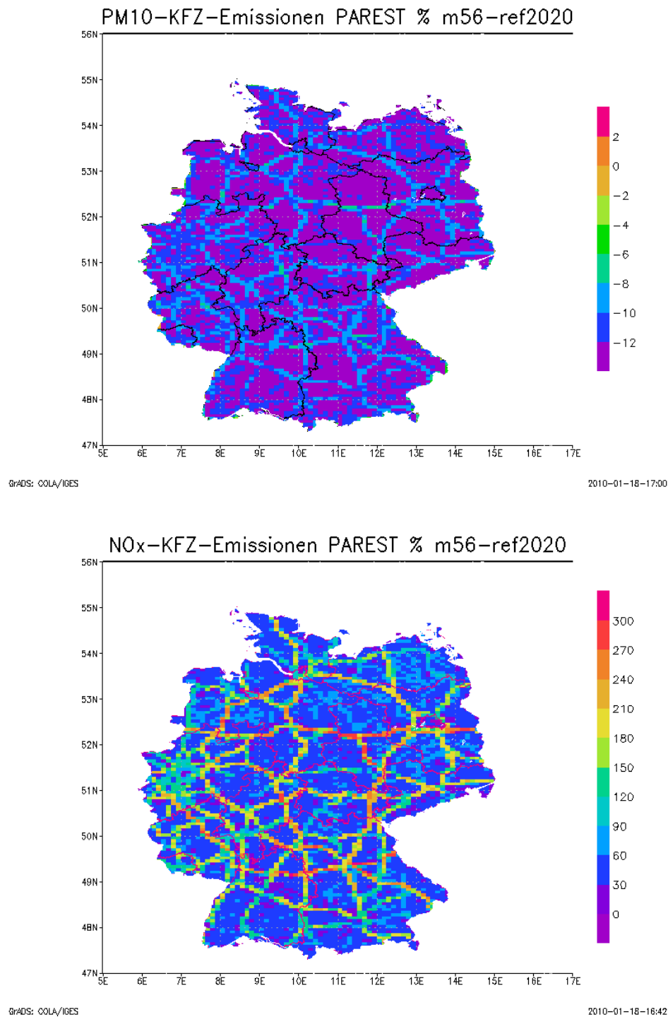
Abbildung 3-2 TREMOVE 2.7-Verkehrsemissionen relativ zu den TREMOD 4.17M-Verkehrsemissionen für die Referenz 2020. Angaben in %. Oben verkehrsbedingte PM10-Emissionen, unten verkehrsbedingte NO x -Emissionen.
