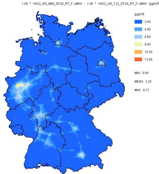
Abbildung 5-7 Absoluter Beitrag ( \mu\text{g}/\text{m}^3 ) der Verursachergruppe „Road transport total“ (SNAP 7) zu den \text{NO}_2 -Jahresmitteln der Referenz 2020. Verkehrsemissionen nach TREMOD 5.04.
