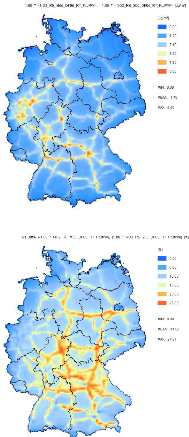
Abbildung 4-5 Absolute (oben, \mu\text{g}/\text{m}^3 ) und relative (unten, %) Änderung der \text{NO}_2 -Jahresmittelwerte 2005 als Folge des Austauschs der Verkehrsemissionen (TREMOD 4.17M durch TREMOVE 2.7 ersetzt). MIN, MEAN und MAX geben den Konzentrationsänderungsbereich (MIN und MAX) sowie die mittlere Konzentrationsänderung (MEAN) über Deutschland an. Meteorologische Referenz ist 2005.
