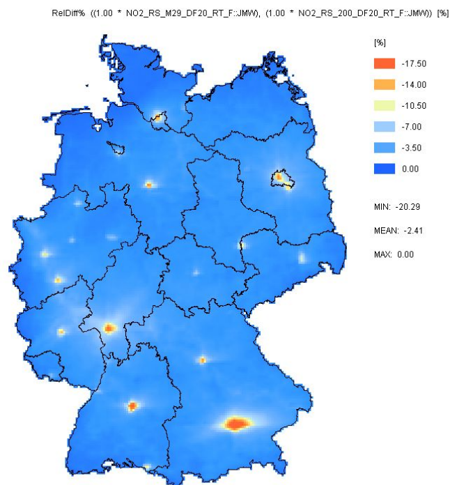
Abbildung 5-38 Relative Änderung der NO 2 -Jahresmittelwerte in % bezogen auf die Referenz 2020 für Maßnahmenpaket M29 (MFR-Sonstiger Verkehr, SNAP 8). Die Änderung wird berechnet als: M29-Referenz 2020. Negative Zahlen sind Abnahmen. MIN, MEAN und MAX geben den Prozentbereich (MIN und MAX) der Änderung sowie die mittlere Änderung (MEAN) über Deutschland an.
