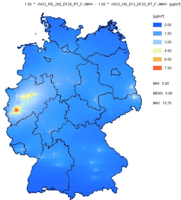
Abbildung 5-4 Beitrag (µg/m 3 ) der Verursacherguppe „Energy transformation“ (SNAP 1) zu den NO 2 -Jahresmitteln der Referenz 2020 (siehe Abbildung 4-1).
