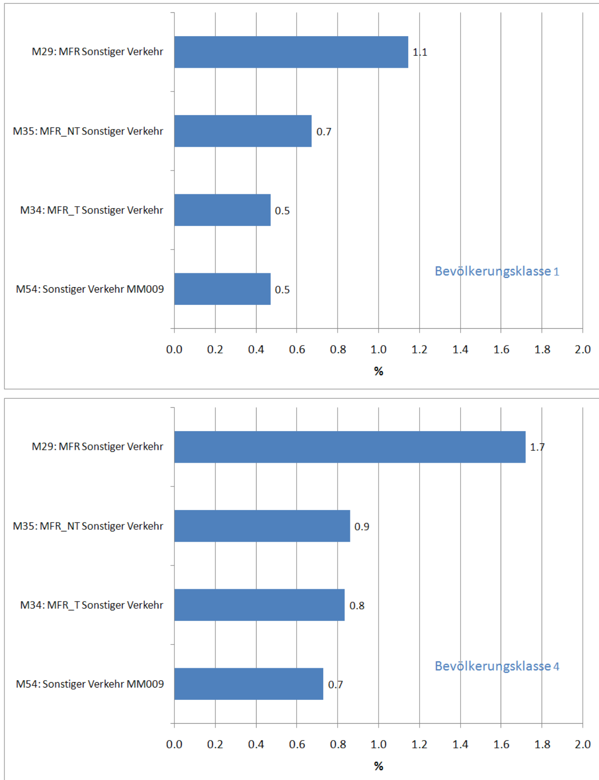
Abbildung 6-11 Bevölkerungsgewichtete relative PM10-Minderungspotenziale aller Szenarien der Verursachergruppe Sonstiger Verkehr für die Bevölkerungsklassen 1 und 4. Die Potenziale geben für jede Maßnahme das Potenzial in % der Minderung an, die für die Referenz 2020 (PM10-Minderung von 2005 bis 2020=100%) berechnet wird.
