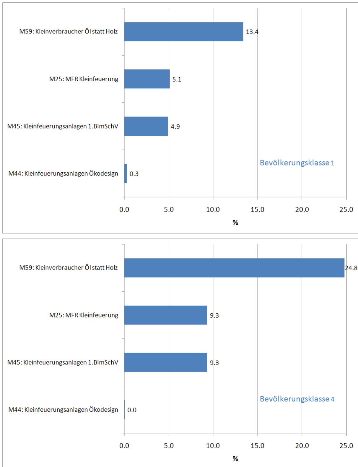
Abbildung 7-13 Bevölkerungsgewichtete relative PM2.5-Minderungspotenziale aller Szenarien der Verursachergruppe Kleinverbraucher für die Bevölkerungsklassen 1 und 4. Die Potenziale geben für jede Maßnahme das Potenzial in % der Minderung an, die für die Referenz 2020 (PM2.5-Minderung von 2005 bis 2020) berechnet wird.
