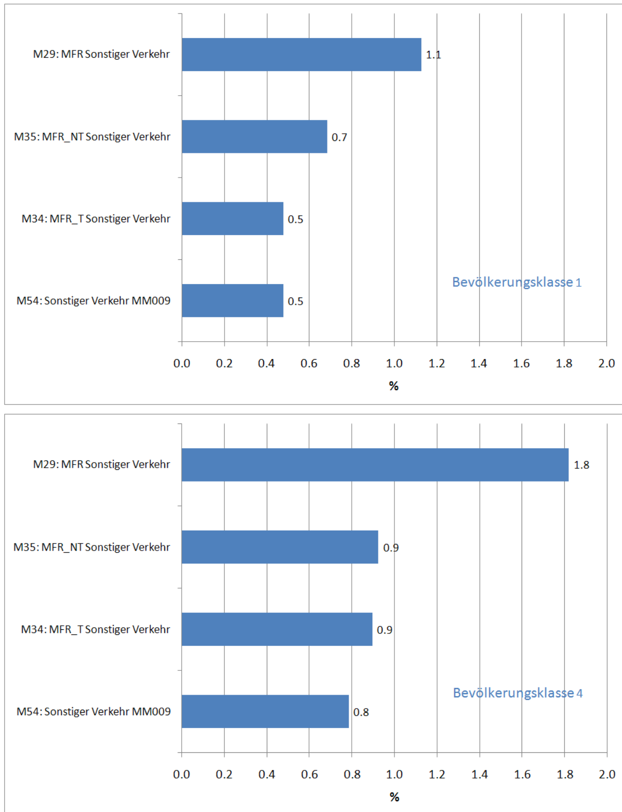
Abbildung 7-17 Bevölkerungsgewichtete relative PM2.5-Minderungspotenziale aller Szenarien der Verursachergruppe Sonstiger Verkehr für die Bevölkerungsklassen 1 und 4. Die Potenziale geben für jede Maßnahme das Potenzial in % der Minderung an, die für die Referenz 2020 (PM2.5-Minderung von 2005 bis 2020) berechnet wird.
