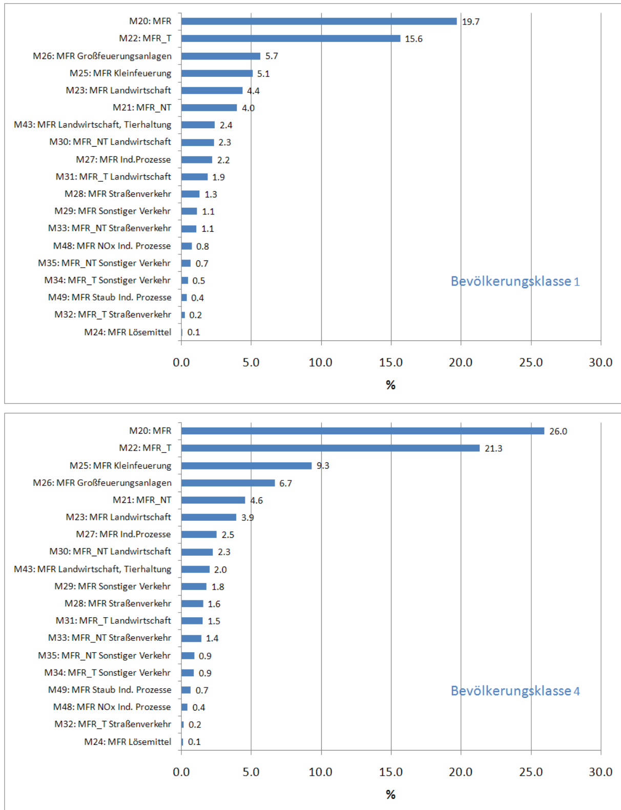
Abbildung 7-11 Bevölkerungsgewichtete relative PM 2.5 -Minderungspotenziale aller MFR-Szenarien für die Bevölkerungsklassen 1 und 4. Die Potenziale geben für jede Maßnahme das Potenzial in % der Minderung an, die für die Referenz 2020 (PM 2.5 -Minderung von 2005 bis 2020) berechnet wird.
