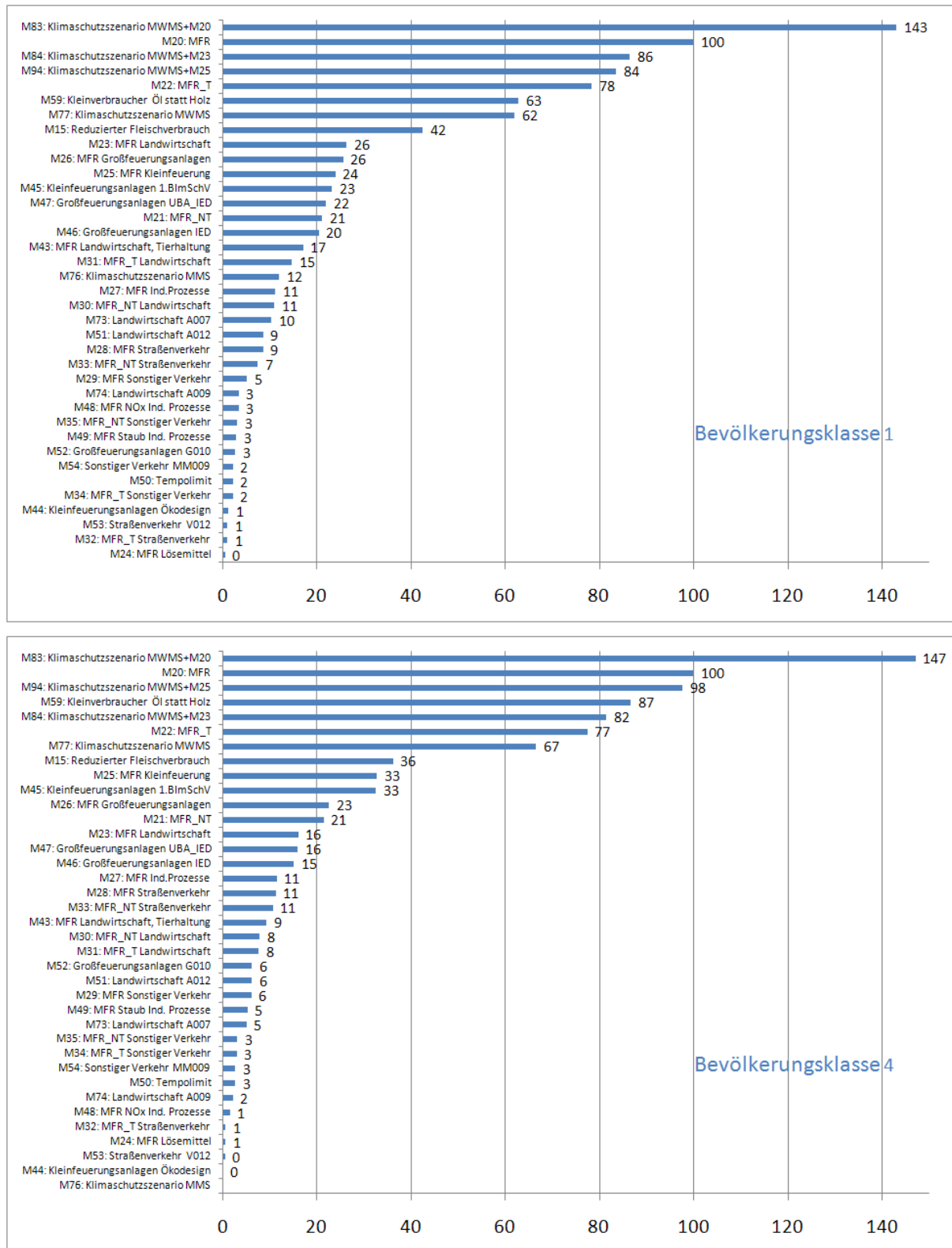
Abbildung 6-3 Bevölkerungsgewichtete relative PM10-Minderungspotenziale für die Bevölkerungsklassen 1 und 4. Die Potenziale geben für jede Maßnahme das Potenzial in % des Potenzials an, das für das MFR-Szenario M20 (=100%) berechnet wird.
