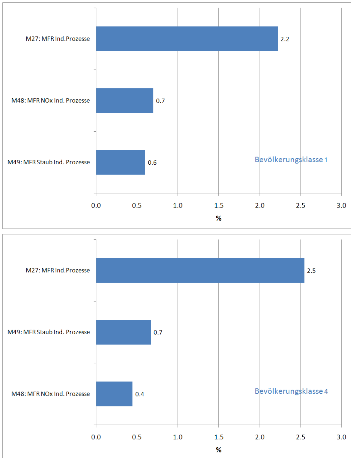
Abbildung 7-15 Bevölkerungsgewichtete relative PM 2.5 -Minderungspotenziale aller Szenarien der Verursachergruppe Industrielle Prozesse für die Bevölkerungsklassen 1 und 4. Die Potenziale geben für jede Maßnahme das Potenzial in % der Minderung an, die für die Referenz 2020 (PM 2.5 -Minderung von 2005 bis 2020) berechnet wird.
