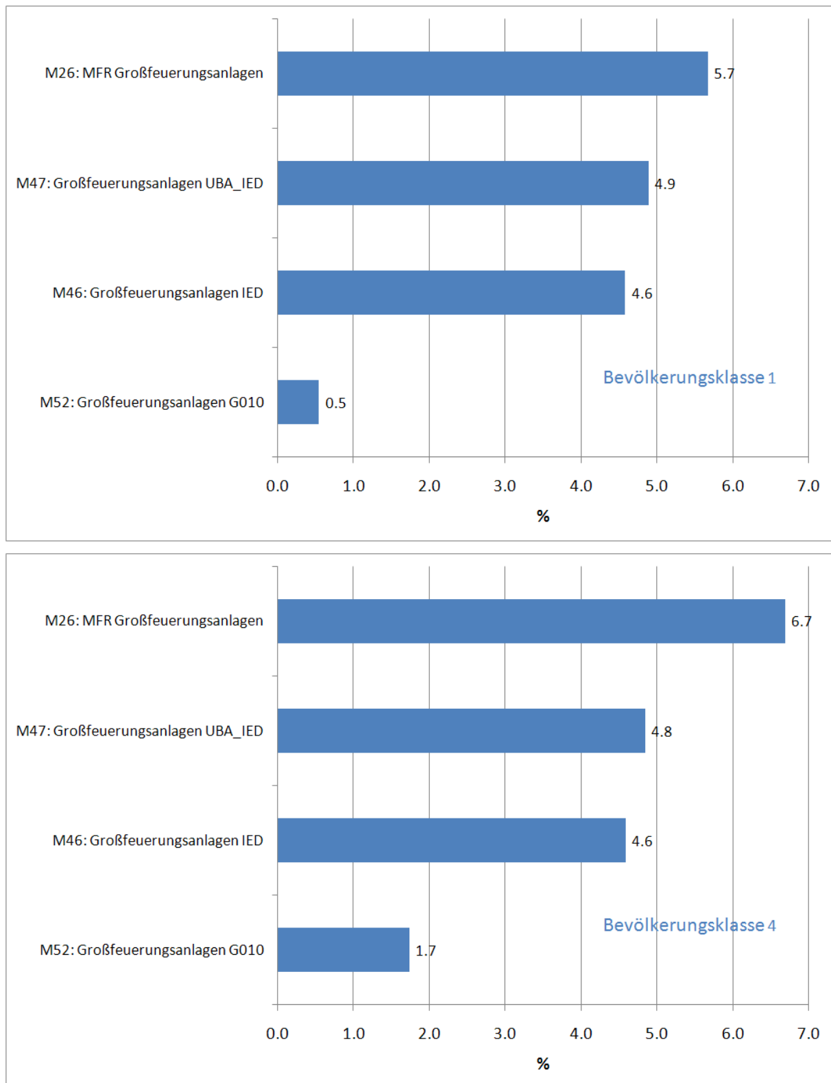
Abbildung 7-14 Bevölkerungsgewichtete relative PM2.5-Minderungspotenziale aller Szenarien der Verursachergruppe Großfeuerungsanlagen für die Bevölkerungsklassen 1 und 4. Die Potenziale geben für jede Maßnahme das Potenzial in % der Minderung an, die für die Referenz 2020 (PM2.5-Minderung von 2005 bis 2020) berechnet wird.
