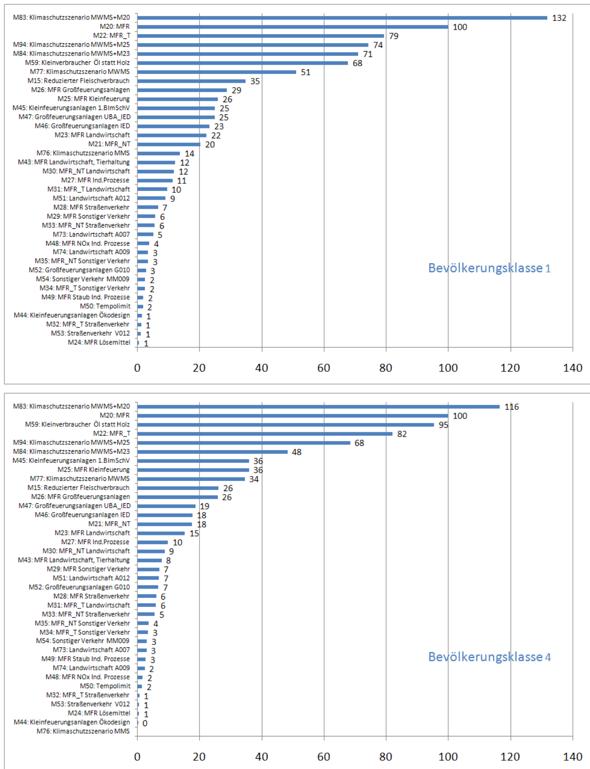
Abbildung 7-9 Bevölkerungsgewichtete relative PM 2.5 -Minderungspotenziale für die Bevölkerungsklassen 1 und 4. Die Potenziale geben für jede Maßnahme das Potenzial in % des Potenzials an, das für das MFR-Szenario M20 (=100%) berechnet wird.
