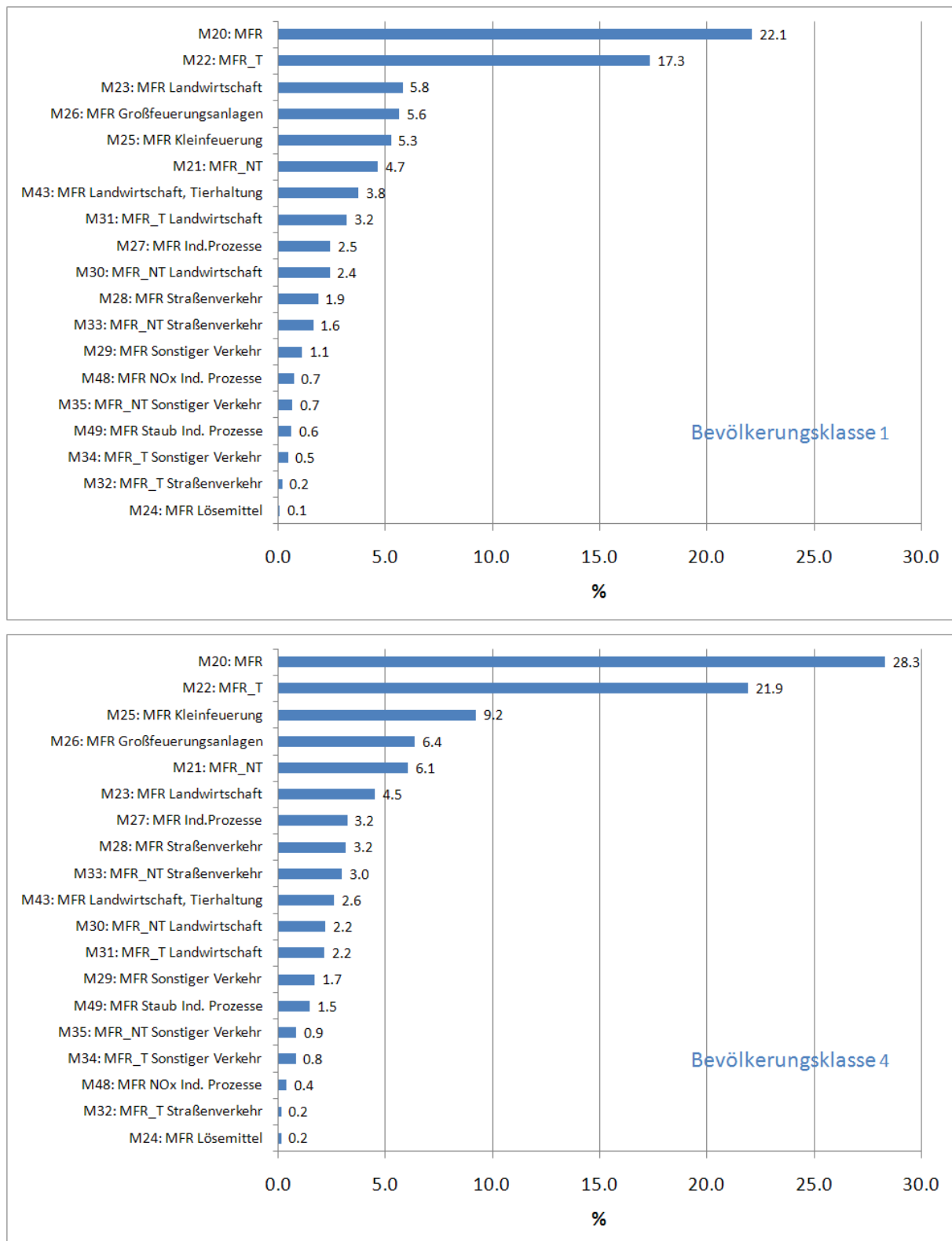
Abbildung 6-5 Bevölkerungsgewichtete relative PM10-Minderungspotenziale aller MFR-Szenarien für die Bevölkerungsklassen 1 und 4. Die Potenziale geben für jede Maßnahme das Potenzial in % der Minderung an, die für die Referenz 2020 (PM10-Minderung von 2005 bis 2020=100%) berechnet wird.
