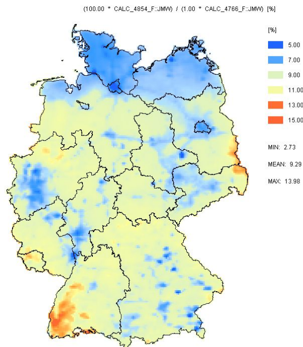
Abbildung 5-43 Ausschöpfung in % des maximal möglichen Minderungspotenzial (-100% aller deutschen Emissionen) durch das MFR-Szenario technische Maßnahmen, M22. MIN, MEAN und MAX geben den Prozentbereich (MIN und MAX) der Änderung sowie die mittlere Änderung (MEAN) über Deutschland an.
