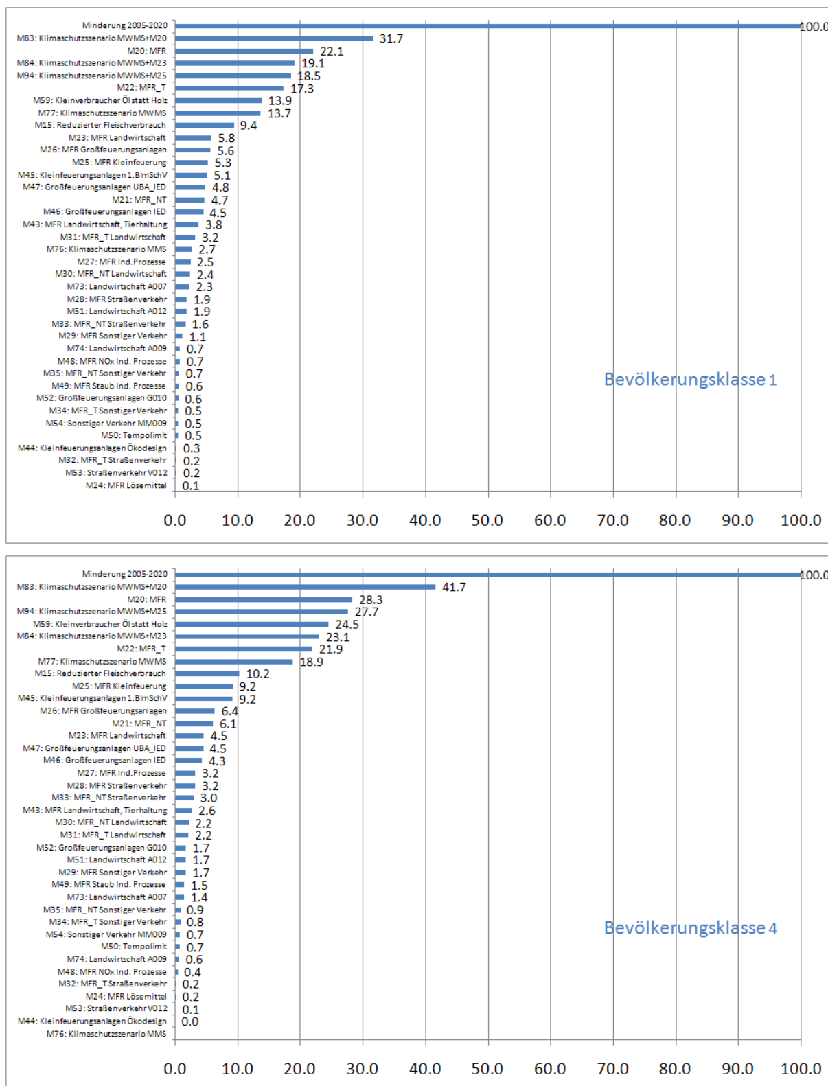
Abbildung 6-4 Bevölkerungsgewichtete relative PM10-Minderungspotenziale für die Bevölkerungsklassen 1 und 4. Die Potenziale geben für jede Maßnahme das Potenzial in % der Minderung an, die für die Referenz 2020 (PM10-Minderung von 2005 bis 2020=100%) berechnet wird.
