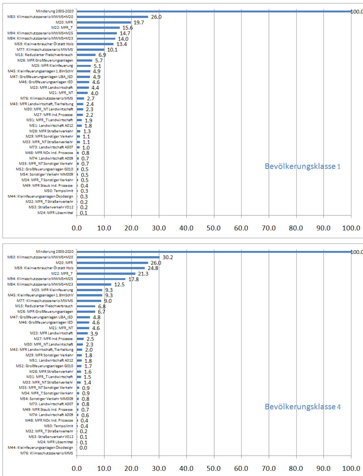
Abbildung 7-10 Bevölkerungsgewichtete relative PM 2.5 -Minderungspotenziale für die Bevölkerungsklassen 1 und 4. Die Potenziale geben für jede Maßnahme das Potenzial in % der Minderung an, die für die Referenz 2020 (PM 2.5 -Minderung von 2005 bis 2020=100%) berechnet wird.
