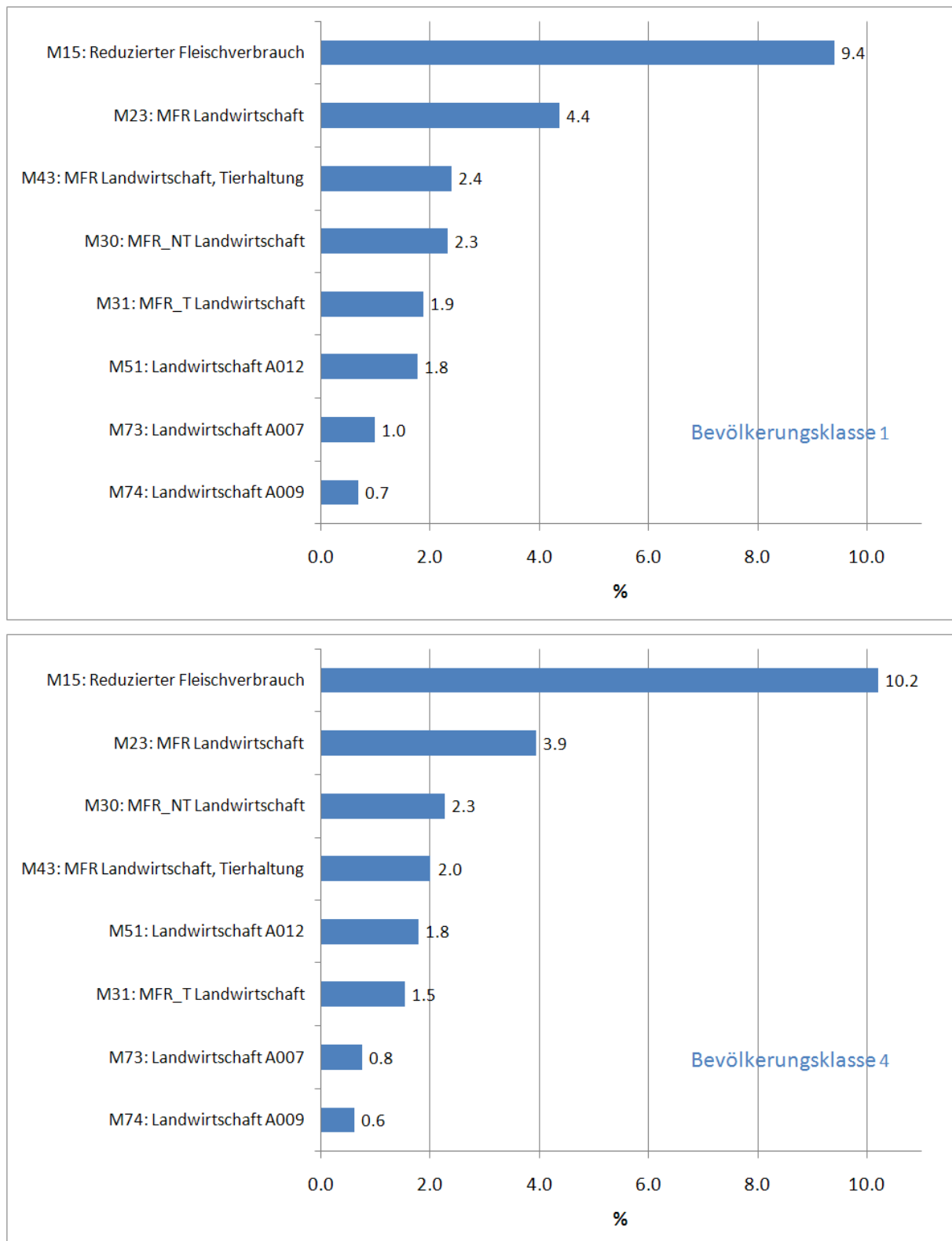
Abbildung 7-12 Bevölkerungsgewichtete relative PM2.5-Minderungspotenziale aller Szenarien der Verursachergruppe Landwirtschaft für die Bevölkerungsklassen 1 und 4. Die Potenziale geben für jede Maßnahme das Potenzial in % der Minderung an, die für die Referenz 2020 (PM2.5-Minderung von 2005 bis 2020) berechnet wird.
