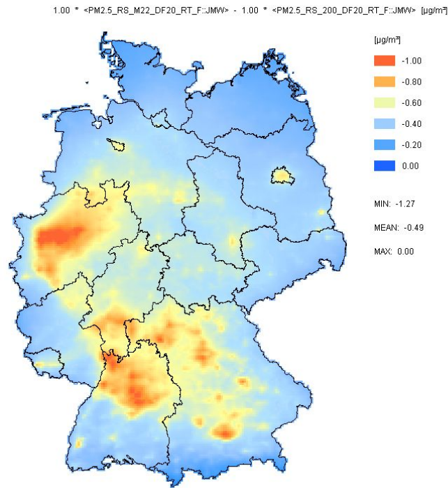
Abbildung 7-5 Absolute Änderung der PM2.5-Jahresmittelwerte in µg/m³ bezogen auf die Referenz 2020 für Maßnahmenpaket M22 (MFR-Szenario, technische Maßnahmen). Die Änderung wird berechnet als: M22-Referenz 2020. Negative Zahlen sind Abnahmen. MIN, MEAN und MAX geben den Konzentrationsbereich (MIN und MAX) der Änderung sowie die mittlere Änderung (MEAN) über Deutschland.
