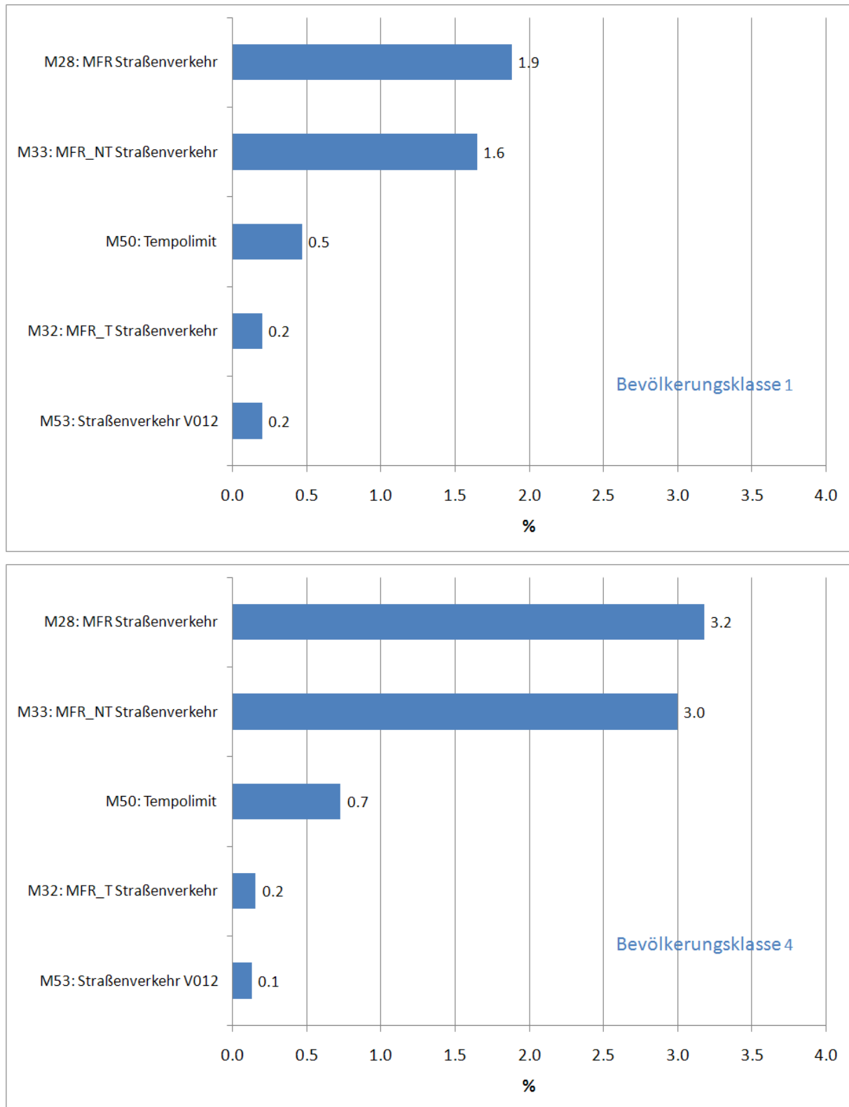
Abbildung 6-10 Bevölkerungsgewichtete relative PM10-Minderungspotenziale aller Szenarien der Verursachergruppe Straßenverkehr für die Bevölkerungsklassen 1 und 4. Die Potenziale geben für jede Maßnahme das Potenzial in % der Minderung an, die für die Referenz 2020 (PM10-Minderung von 2005 bis 2020=100%) berechnet wird.
