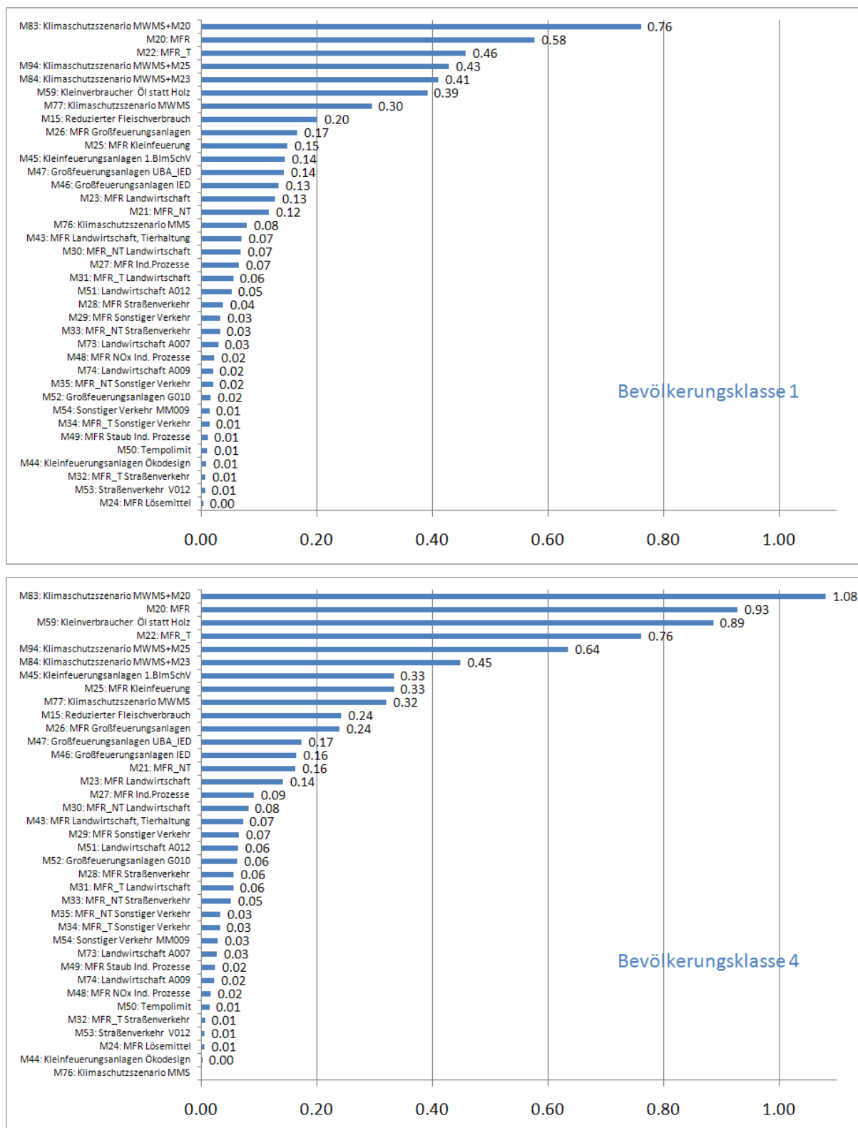
Abbildung 7-7 Bevölkerungsgewichtete PM 2.5 -Minderungspotenziale für die Bevölkerungsklassen 1 und 4. Die Potenziale geben für jede Maßnahme die berechnete absolute Änderung (Abnahmen sind positiv) der PM 2.5 -Jahresmittelwerte in µg/m 3 bezogen auf die Referenz 2020 an.
