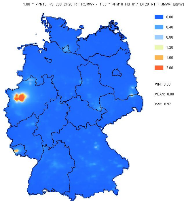
Abbildung 5-12 Beitrag ( \mu\text{g}/\text{m}^3 ) der Verursacherguppe „Extractions of fossil fuels“ (SNAP 5) zu den PM10-Jahresmitteln der Referenz 2020 (siehe Abbildung 4-1).
