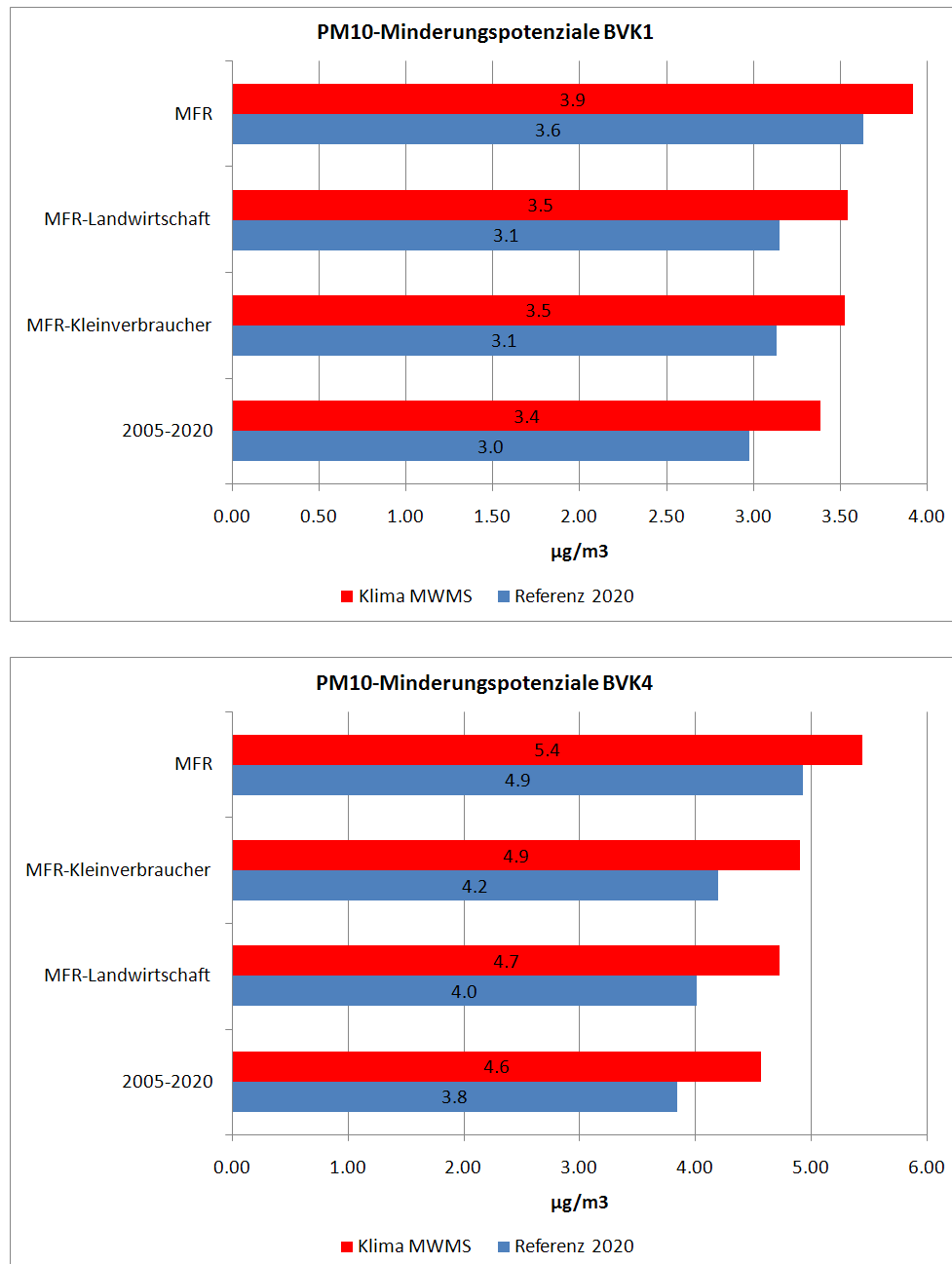
Abbildung 8-2 Absolute Minderungen der PM10-Jahresmittelwerte in \mu\text{g}/\text{m}^3 , die aufgrund der Emissionsentwicklung 2005 bis 2020 (Referenz 2020 und Klimaschutzszenario MWMS) und durch die zusätzlichen Maßnahmen des MFR-Szenarios (M20 und M83), des MFR-Szenarios Landwirtschaft (M23 und M84) und des MFR-Szenarios Kleinf Feuerungsanlagen (M25 und M94) erreicht werden können. Mittlere bevölkerungsgewichtete Abnahmen der Jahresmittelwerte für die 6 Bewertungsklassen. Ländliche Regionen (BVK1) und Ballungsräume (BVK4).
