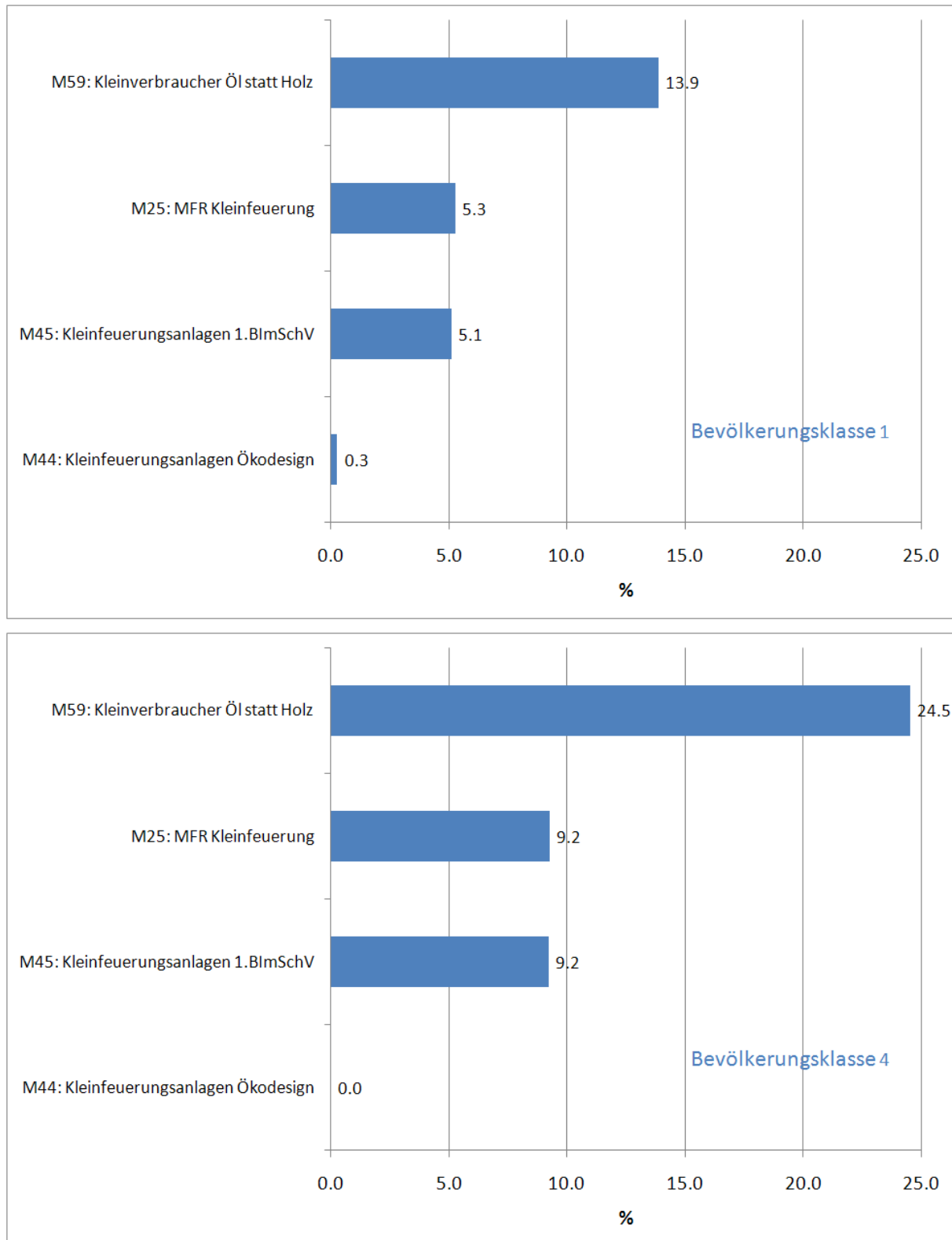
Abbildung 6-7 Bevölkerungsgewichtete relative PM10-Minderungspotenziale aller Szenarien der Verursachergruppe Kleinverbraucher für die Bevölkerungsklassen 1 und 4. Die Potenziale geben für jede Maßnahme das Potenzial in % der Minderung an, die für die Referenz 2020 (PM10-Minderung von 2005 bis 2020=100%) berechnet wird.
