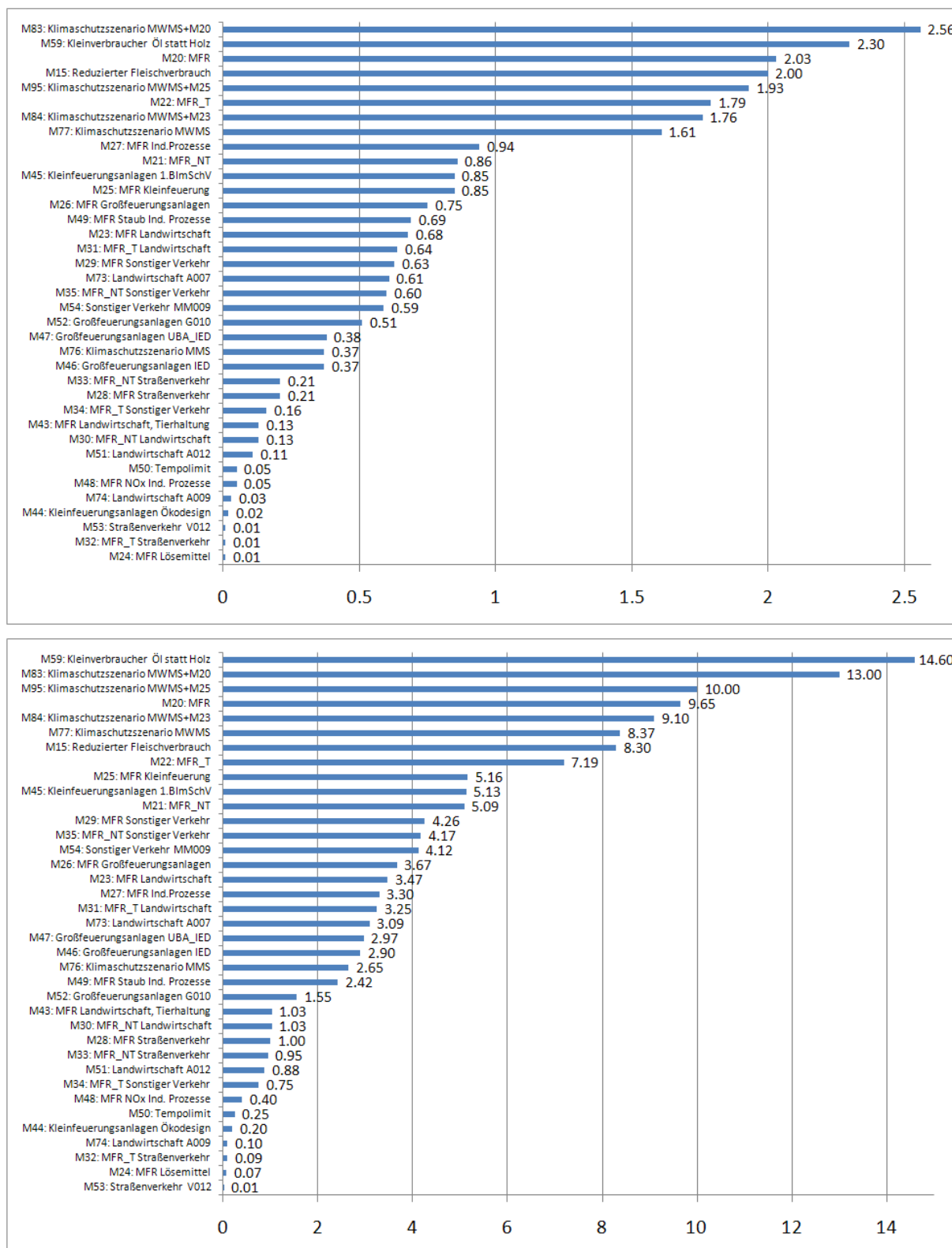
Abbildung 6-2 Maximale berechnete absolute Änderung (Abnahmen sind positiv) der PM10-Jahresmittelwerte in \mu\text{g}/\text{m}^3 (oben) und maximale relative Änderung in % (unten) in Deutschland bezogen auf die Referenz 2020.
