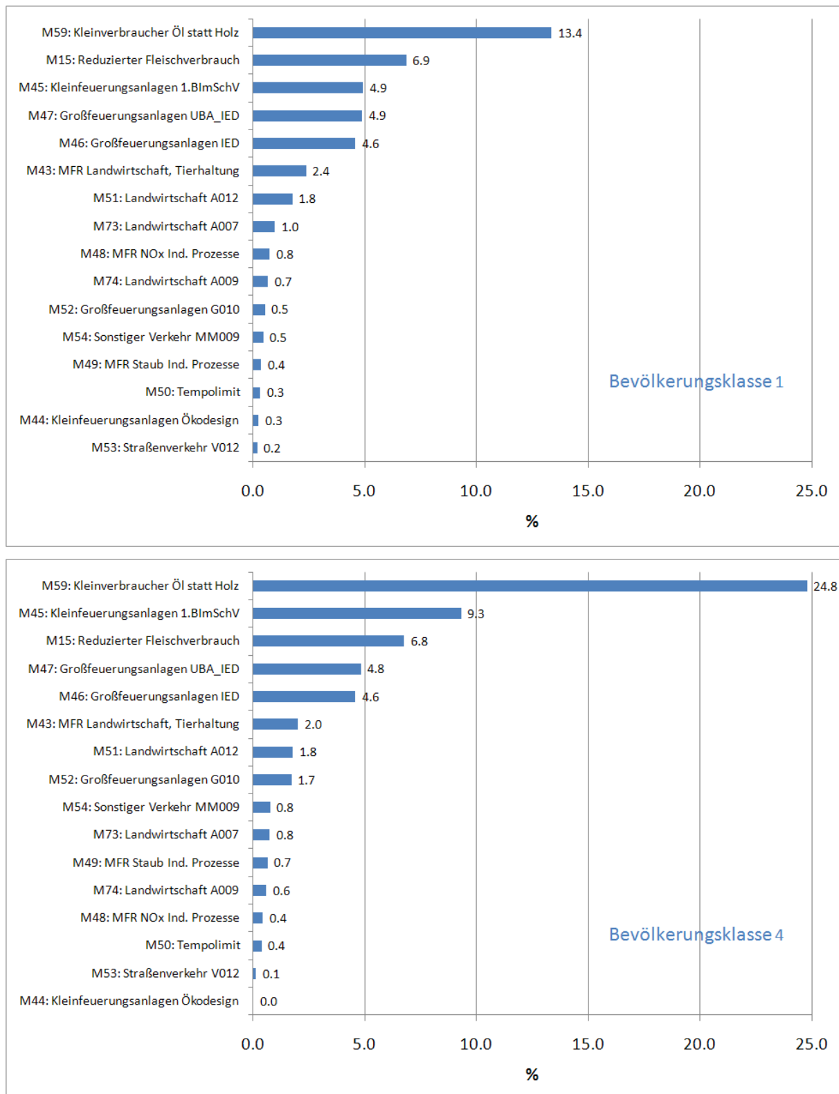
Abbildung 7-18 Bevölkerungsgewichtete relative PM 2.5 -Minderungspotenziale aller Einzelszenarien, d.h. der Szenarien, die nicht zu der alle Einzelmaßnahmen zusammenfassenden MFR-Gruppe gehören für die Bevölkerungsklassen 1 und 4. Die Potenziale geben für jede Maßnahme das Potenzial in % der Minderung an, die für die Referenz 2020 (PM 2.5 -Minderung von 2005 bis 2020) berechnet wird.
