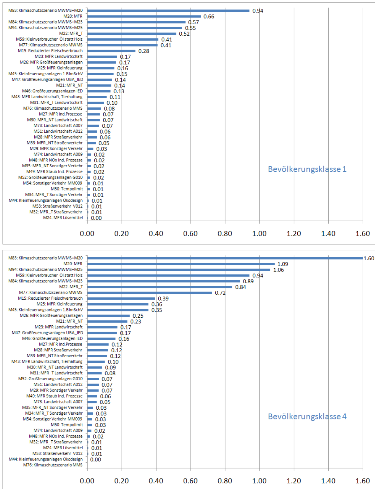
Abbildung 6-1 Bevölkerungsgewichtete PM10-Minderungspotenziale für die Bevölkerungsklassen 1 und 4. Die Potenziale geben für jede Maßnahme die berechnete absolute Änderung (Abnahmen sind positiv) der PM10-Jahresmittelwerte in \mu\text{g}/\text{m}^3 bezogen auf die Referenz 2020 an.
