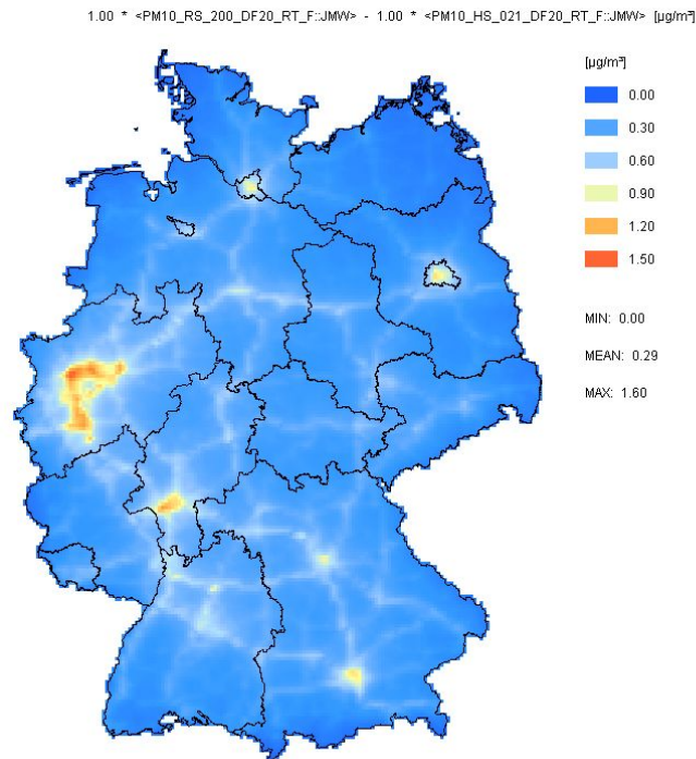
Abbildung 5-18 Beitrag ( \mu\text{g}/\text{m}^3 ) der Verursachergruppe „Road transport brake and tyre wear“ (SNAP 7-4) zu den PM10-Jahresmitteln der Referenz 2020 (siehe Abbildung 4-1).
