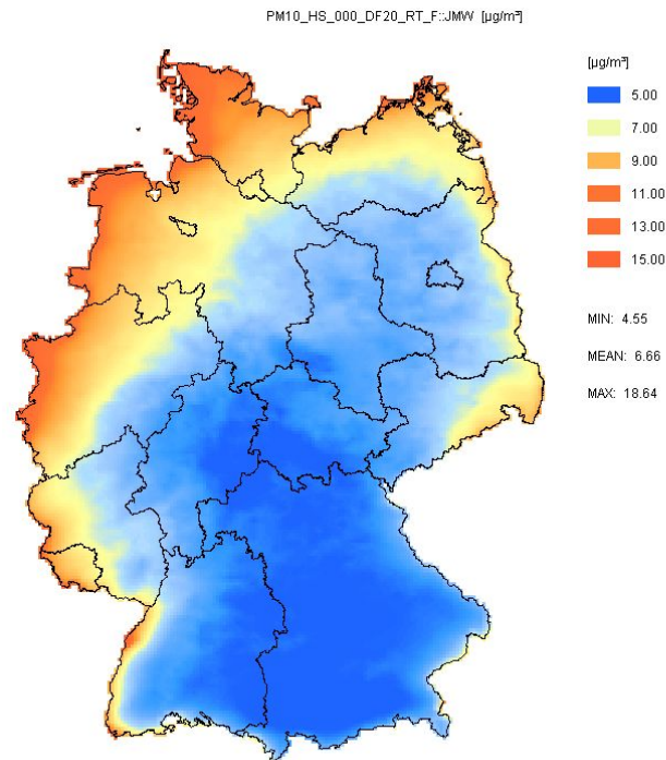
Abbildung 5-1 PM10-Jahresmittelwerte 2020 in \mu\text{g}/\text{m}^3 in Deutschland (2020) ohne die deutschen Emissionen.
