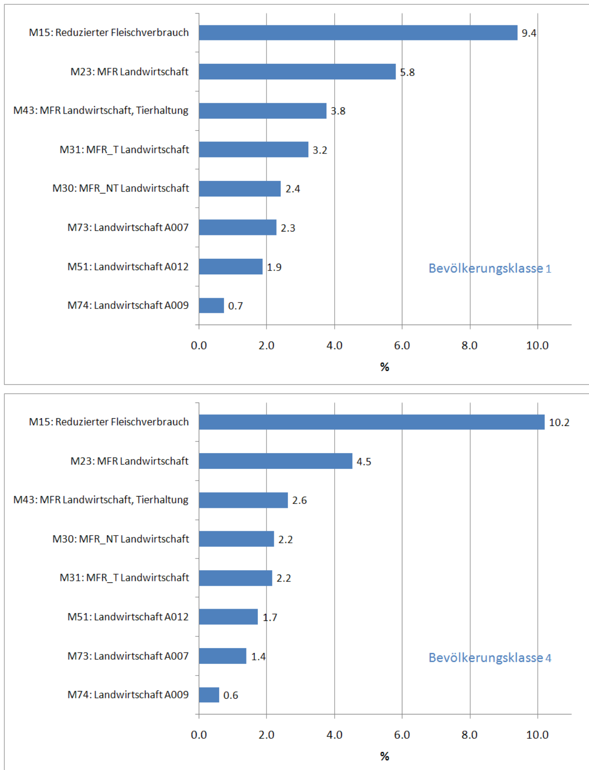
Abbildung 6-6 Bevölkerungsgewichtete relative PM10-Minderungspotenziale aller Szenarien der Verursachergruppe Landwirtschaft für die Bevölkerungsklassen 1 und 4. Die Potenziale geben für jede Maßnahme das Potenzial in % der Minderung an, die für die Referenz 2020 (PM10-Minderung von 2005 bis 2020=100%) berechnet wird.
