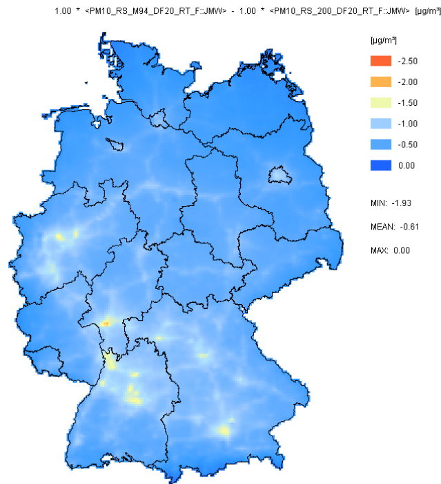
Abbildung 5-100 Absolute Änderung der PM10-Jahresmittelwerte in \mu\text{g}/\text{m}^3 bezogen auf die Referenz 2020 für Maßnahmenpaket M94 (Klimaschutzszenario MWMS+MFR-Kleinf Feuerungsanlagen). Die Änderung wird berechnet als: M94-Referenz 2020. Negative Zahlen sind Abnahmen. MIN, MEAN und MAX geben den Konzentrationsbereich (MIN und MAX) der Änderung sowie die mittlere Änderung (MEAN) über Deutschland an.
