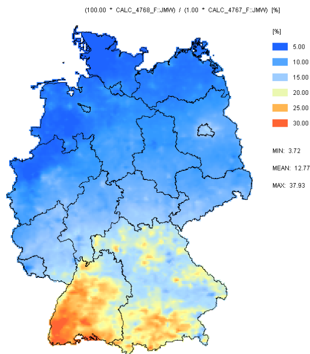
Abbildung 5-7 Anteil (%) der Verursacherguppe „Small combustion sources“ (SNAP 2) am PM10-Immissionsbeitrag der deutschen Emissionen zur Referenz 2020 (siehe Abbildung 5-3).
