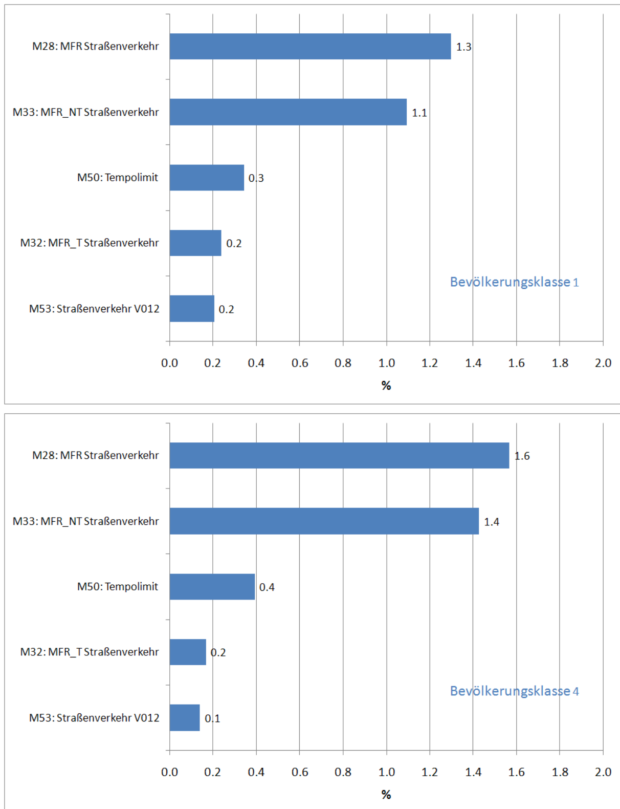
Abbildung 7-16 Bevölkerungsgewichtete relative PM2.5-Minderungspotenziale aller Szenarien der Verursachergruppe Straßenverkehr für die Bevölkerungsklassen 1 und 4. Die Potenziale geben für jede Maßnahme das Potenzial in % der Minderung an, die für die Referenz 2020 (PM2.5-Minderung von 2005 bis 2020) berechnet wird.
