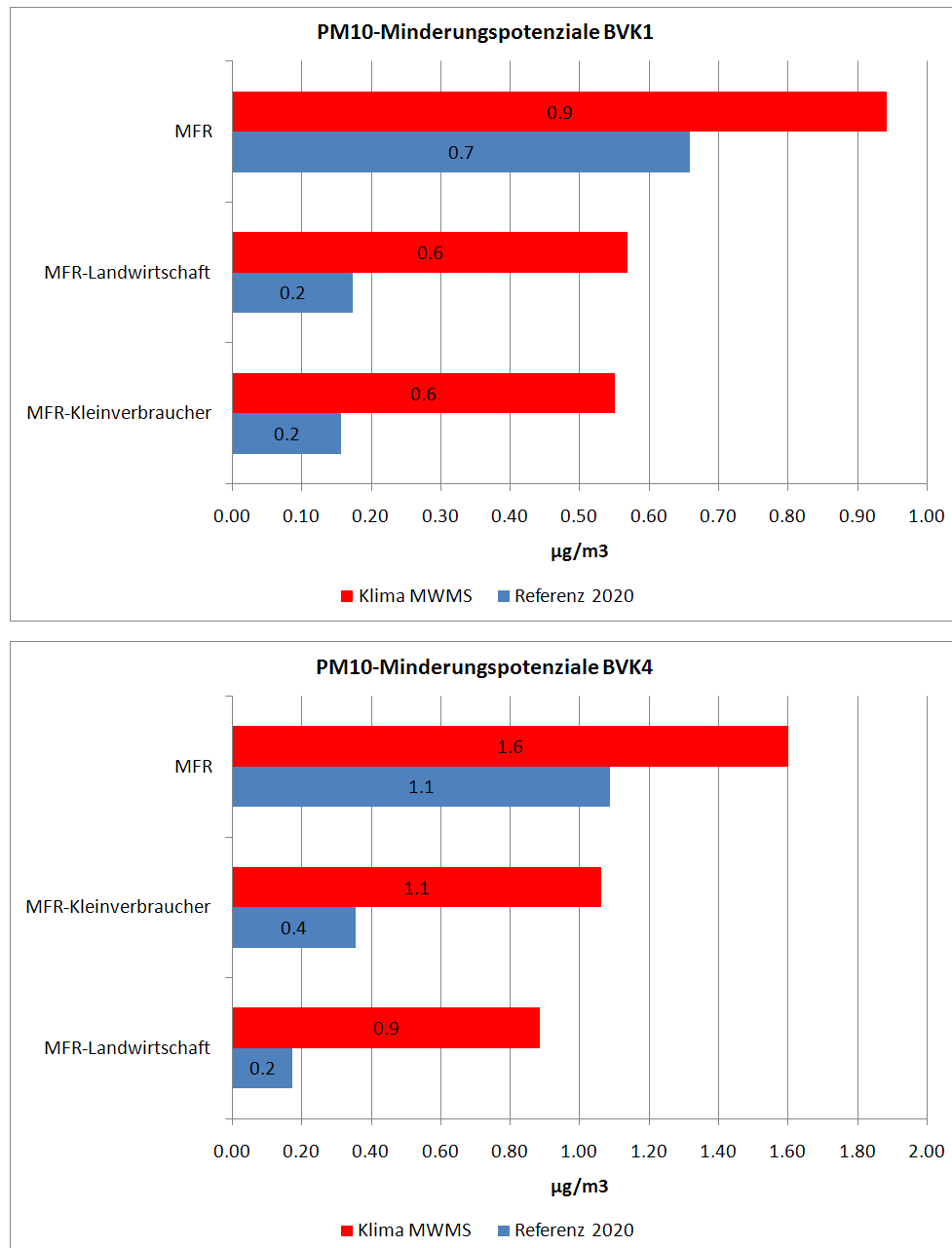
Abbildung 8-3 Absolute Minderungen der PM10-Jahresmittelwerte in \mu\text{g}/\text{m}^3 , die ausgehend von den Konzentrationen der Referenz 2020 durch die zusätzlichen Maßnahmen des MFR-Szenarios (M20 und M83), des MFR-Szenarios Landwirtschaft (M23 und M84) und des MFR-Szenarios Kleinf Feuerungsanlagen (M25 und M94) erreicht werden können. Mittlere bevölkerungsgewichtete Abnahmen der Jahresmittelwerte für die 6 Bewertungsklassen. Ländliche Regionen (BVK1) und Ballungsräume (BVK4).
