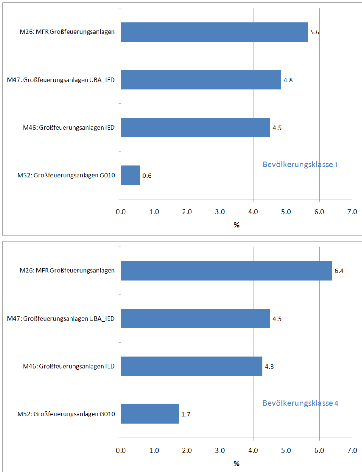
Abbildung 6-8 Bevölkerungsgewichtete relative PM10-Minderungspotenziale aller Szenarien der Verursachergruppe Großfeuerungsanlagen für die Bevölkerungsklassen 1 und 4. Die Potenziale geben für jede Maßnahme das Potenzial in % der Minderung an, die für die Referenz 2020 (PM10-Minderung von 2005 bis 2020=100%) berechnet wird.
