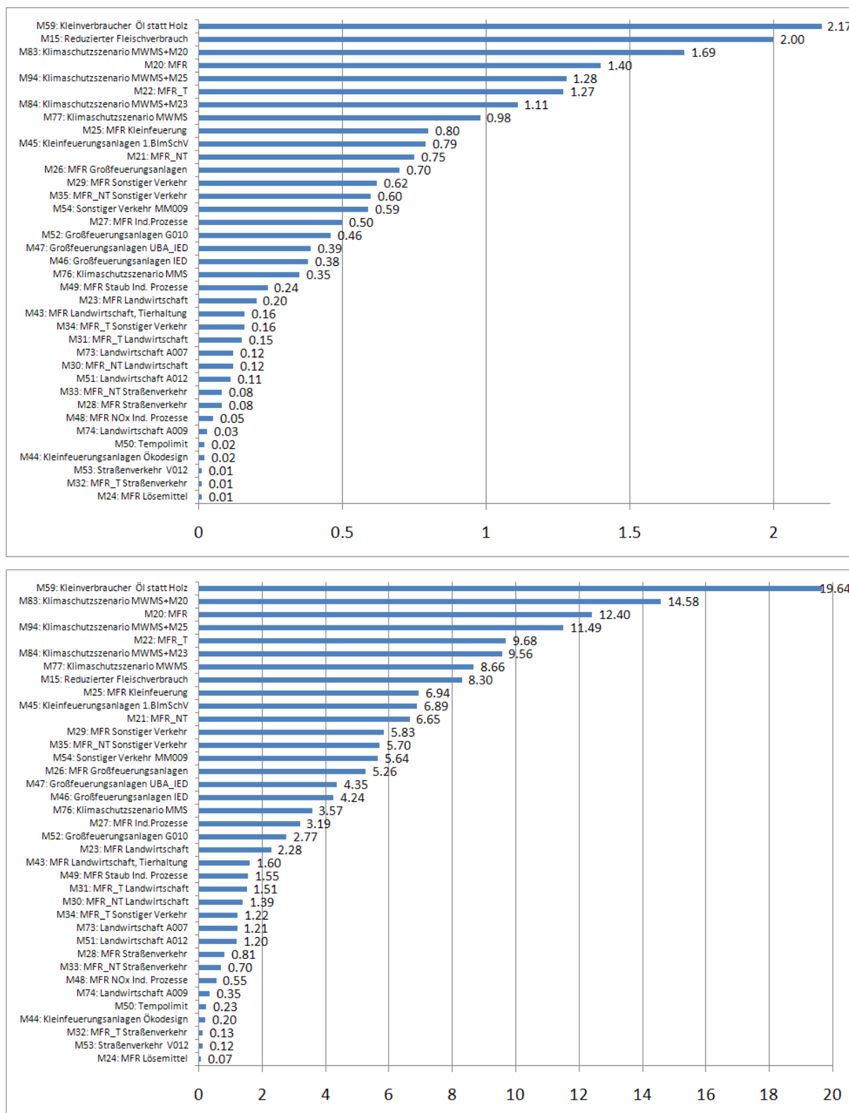
Abbildung 7-8 Maximale berechnete absolute Änderung der PM 2.5 -Jahresmittelwerte in \mu\text{g}/\text{m}^3 (oben) und maximale relative Änderung in % (unten) in Deutschland bezogen auf die Referenz 2020.
