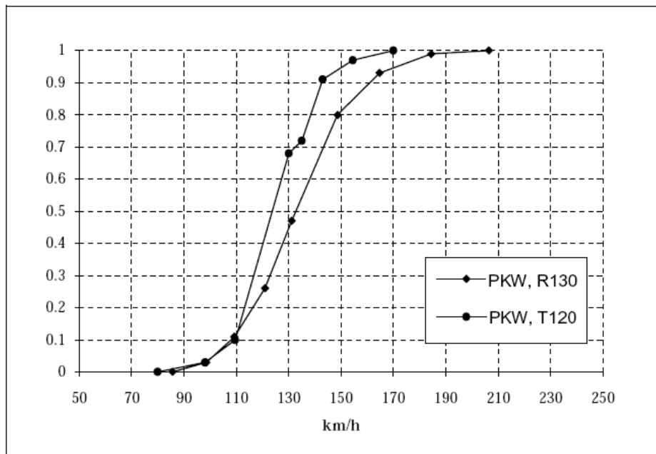
Fig 1 Wunschgeschwindigkeitsverteilungen für PKW auf zweistreifigen Autobahnen [Maier, 2004]
