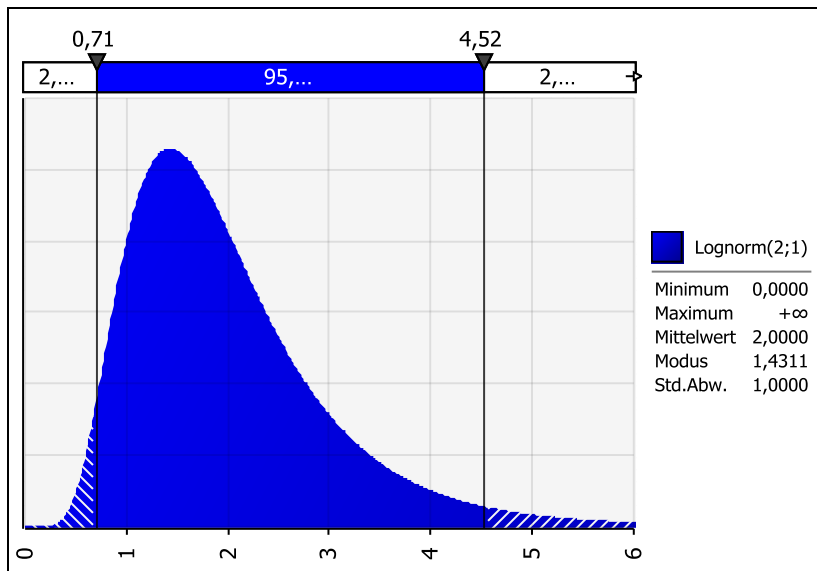
Abbildung 5: Beispiel Lognormalverteilung
