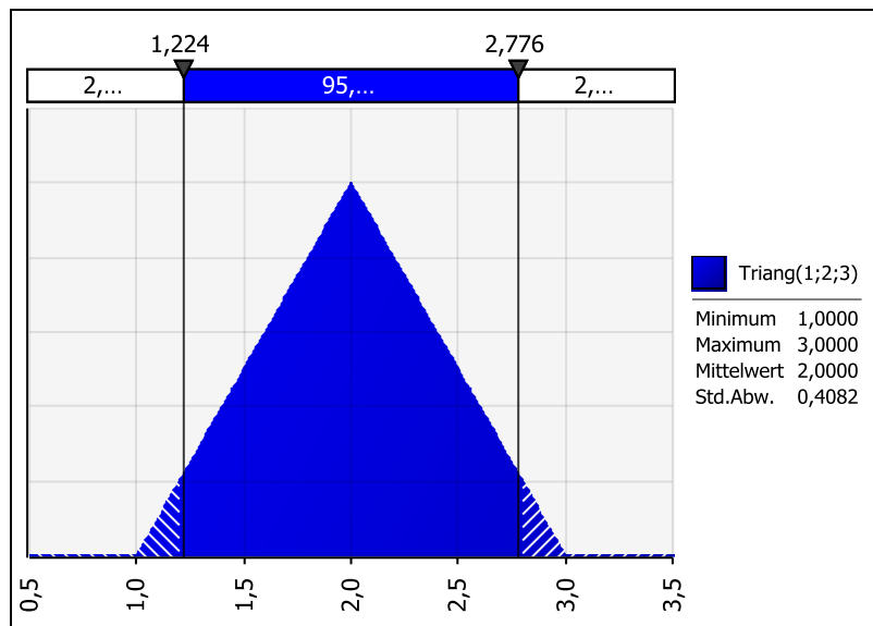
Abbildung 3: Beispiel Dreiecksverteilung
