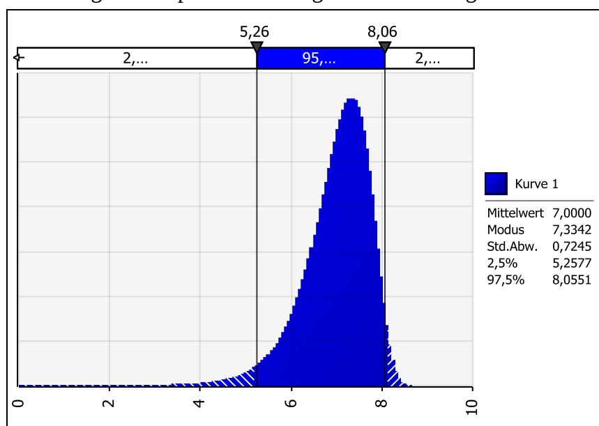
Abbildung 6: Beispiel inverse Lognormalverteilung
