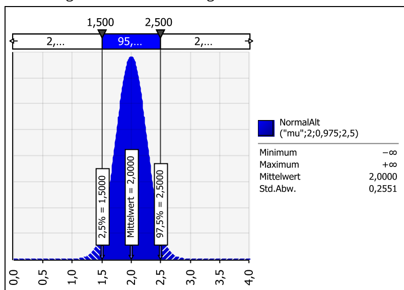
Abbildung 1: Normalverteilung mit Konfidenzintervall
