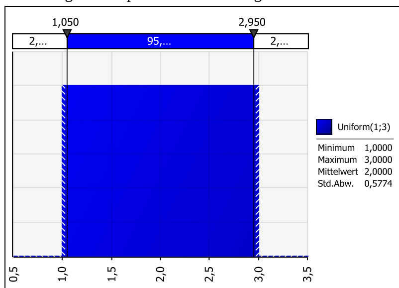
Abbildung 4: Beispiel Gleichverteilung
