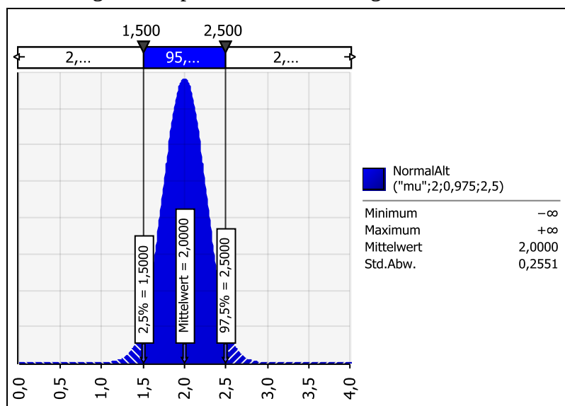
Abbildung 2: Beispiel Normalverteilung
