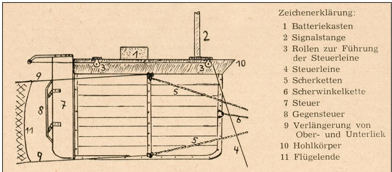
Abb. 5.7: Das Scherbrett mit Steuervorrichtung, schematische Darstellung (KLUST 1956)
