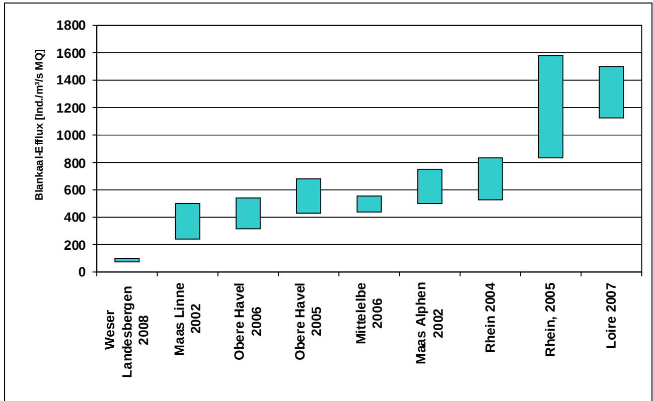
Abb. 6.12: Umfang der jährlichen Blankaalabwanderung in verschiedenen Flüssen, bezogen auf 1 m³/s MQ, Minimal- und Maximalwerte, nach Daten von BRUIJS et al. (2003), KLEIN-BRETELIER et al. (2007), SIMON & FLADUNG (2009), SCHWEVERS et al. (2010a) und FEUNTEUN (2007, mündl. Mitt.)
