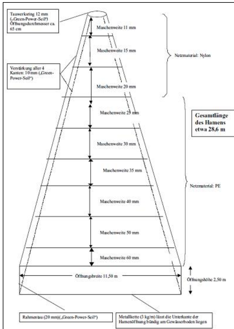
Abb. 5.20: Aufbau des von SCHMALZ (2010) an der Walkmühle an der Werra eingesetzten Hamens zur Beprobung des Turbinendurchflusses von maximal 14 \text{ m}^3/\text{s} (schematisch)
