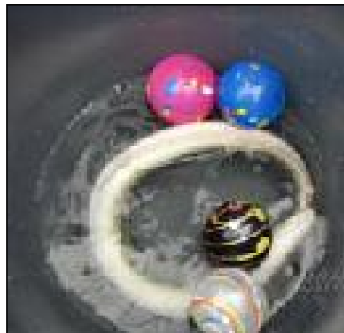
Abb. 5.71: Von HI-Z Turb'n-Tags werden markierte Fische an die Wasseroberfläche befördert, wo sie eingesammelt und auf Verletzungen hin untersucht werden können (BARAN et al. 2010)
