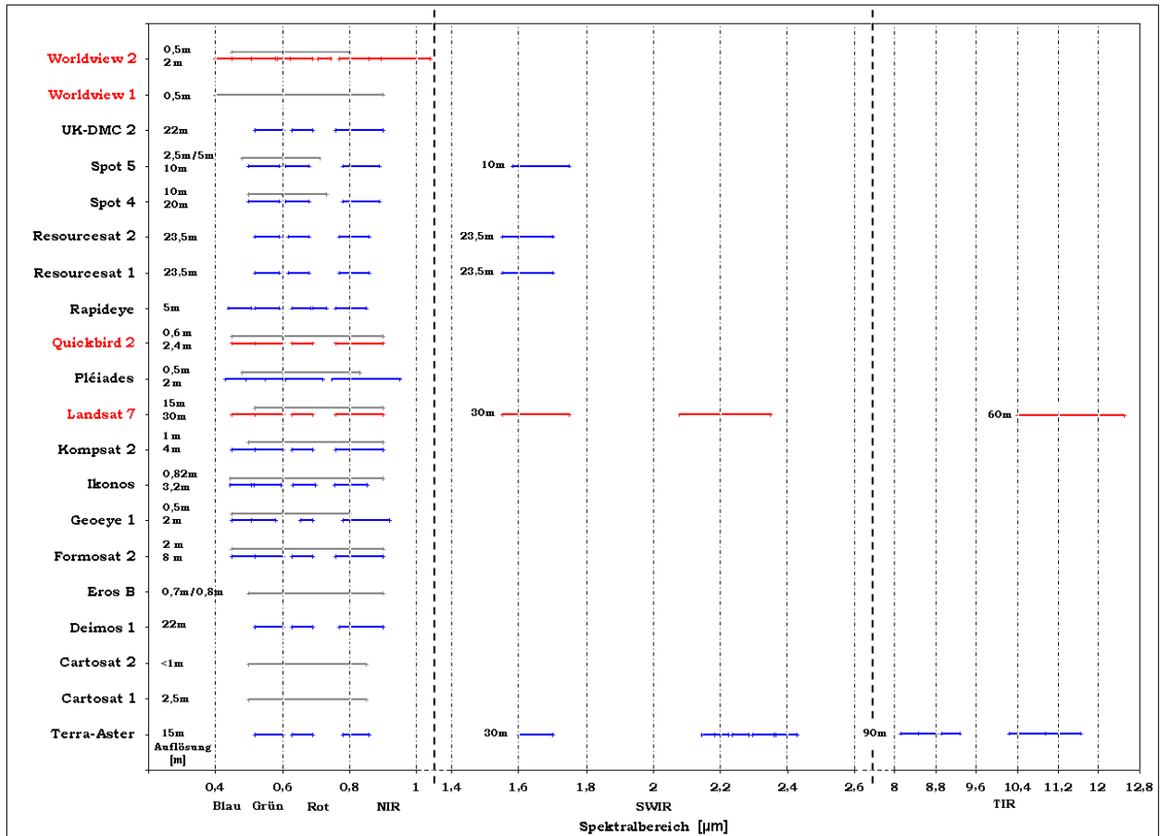
Abbildung 2: Übersicht über die multispektralen und räumlichen Auflösungen aktueller Fernerkundungssatelliten – rot markierte Satelliten wurden im Projekt verwendet
