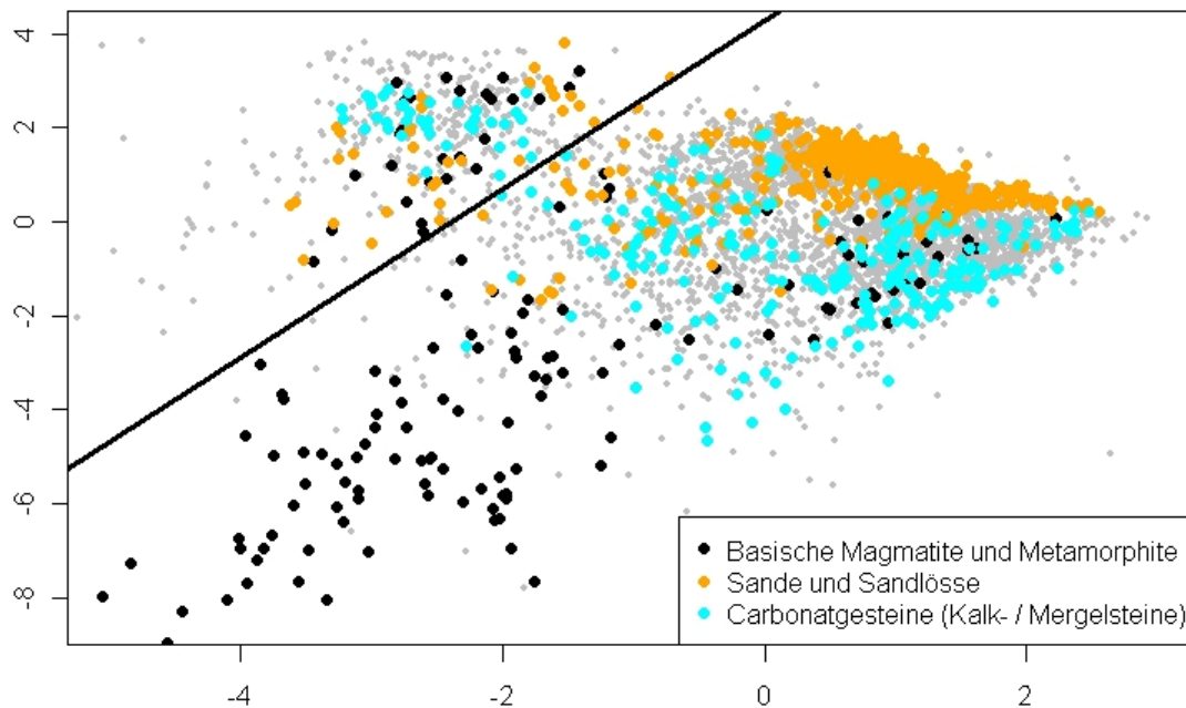
Abbildung 17: Bodenausgangsgestein
