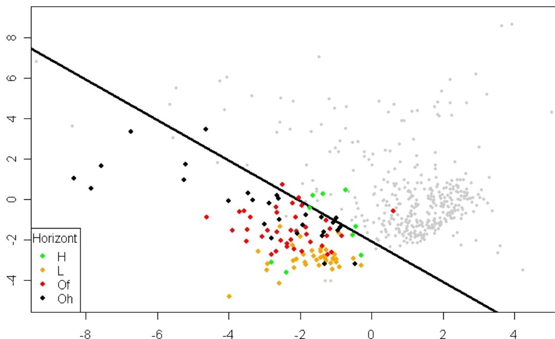
Abbildung 24: Organische Horizonte
