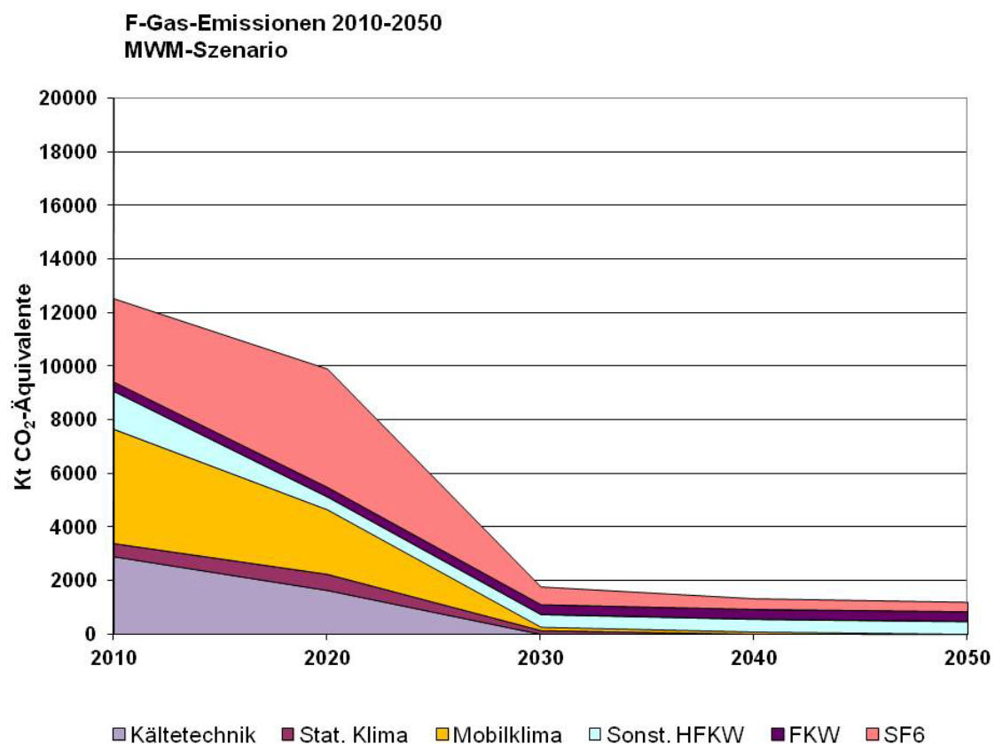
Abbildung 4-A: Projektionen der Emissionen fluoriertener Treibhausgase im Szenario „mit weiteren Maßnahmen“ bis 2050.
