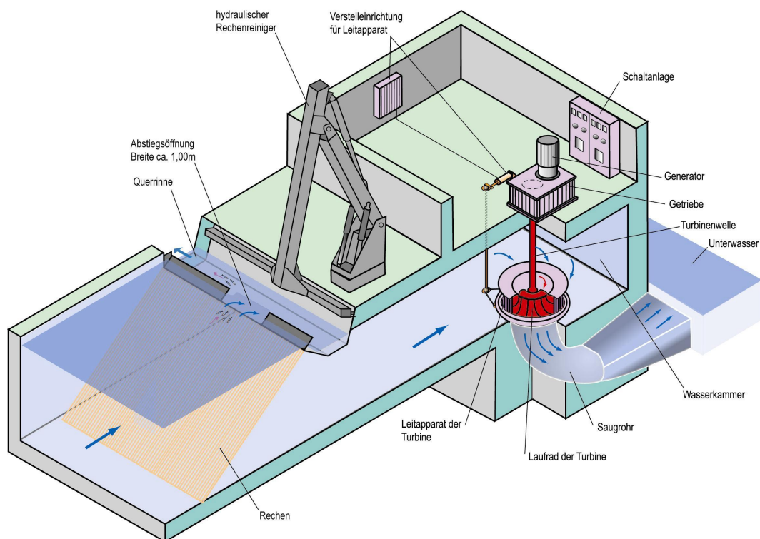
Abb. 5.16: Aufbau einer Wasserkraftanlage mit einem Fischschutzrechen und einer oberen Bypass-Rinne für den Abstieg von Lachssmolts
