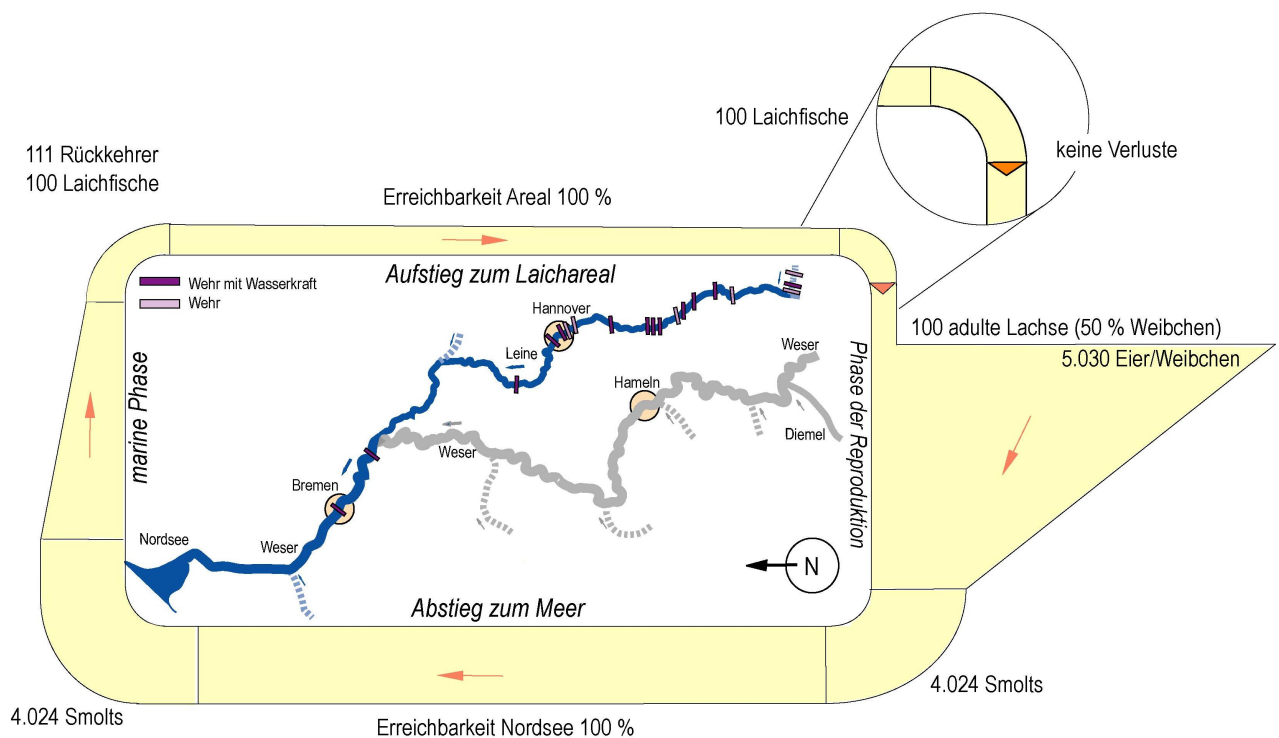
Abb. 5.11: Lebenszyklus des Lachses, berechnet mit populationsbiologischen Parameterwerten für den Selbsterhalt der Population und ohne Verluste an Querbauwerken oder Wasserkraftanlagen
