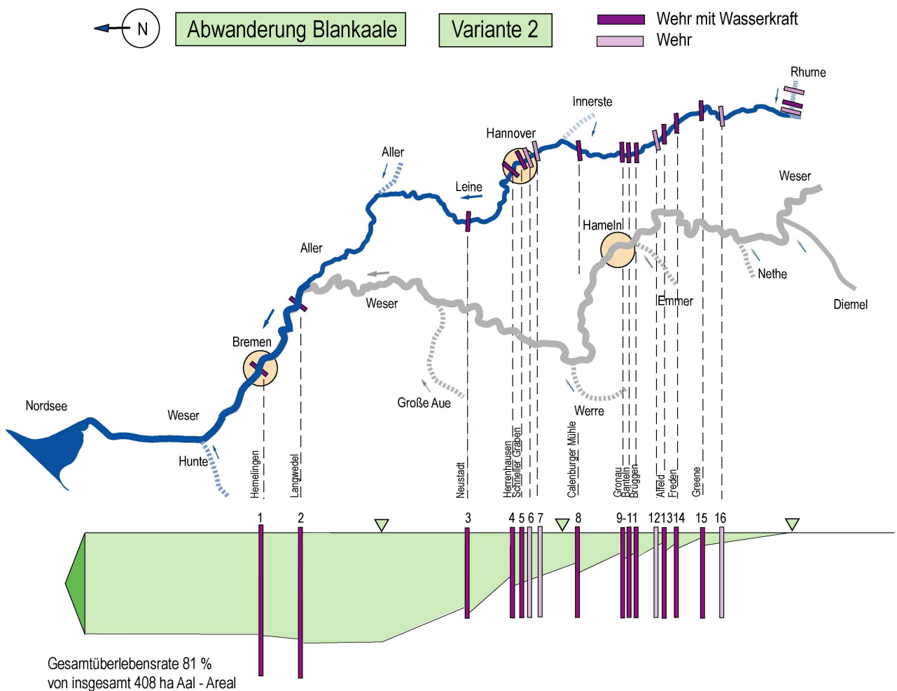
Abb. 5.14: Gesamtüberlebensrate für Aale aus den Leine-Arealen bei Variante 2
