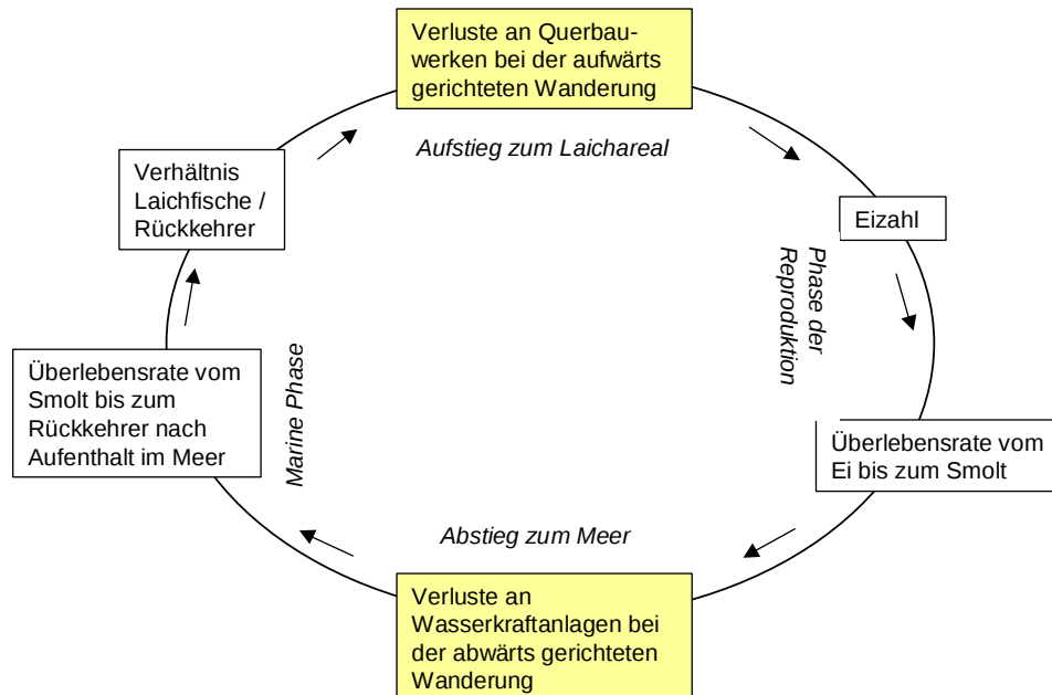
Abb. 4.13: Parameter des Berechnungsmodells zur Abbildung des Lebenszyklus des Atlantischen Lachses (weiß: populationsdynamische Parameter, gelb: Verluste an Querbauwerken und Wasserkraftanlagen)
