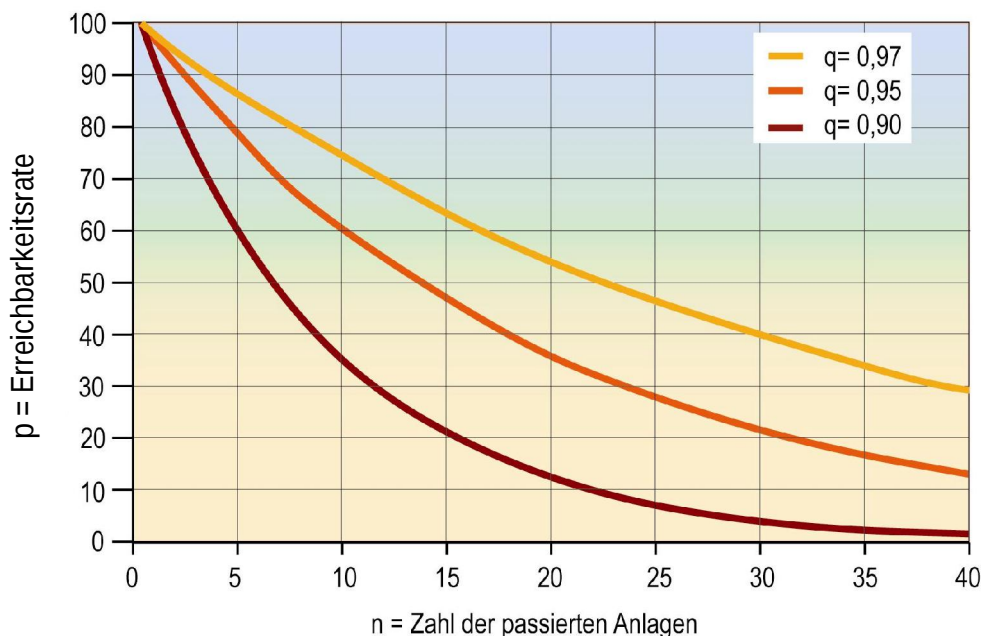
Abb. 4.12: Kumulierte Erreichbarkeitsrate p auf- oder abwandernder Fische bei der Passage von n Standorten mit der lokalen Überlebensrate q (DUMONT et.al. 2005)
