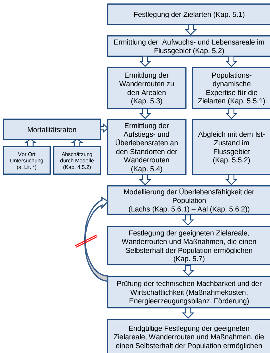
Abb. 5.1: Fließdiagramm Ergebnisse der Flussgebietsstrategie
