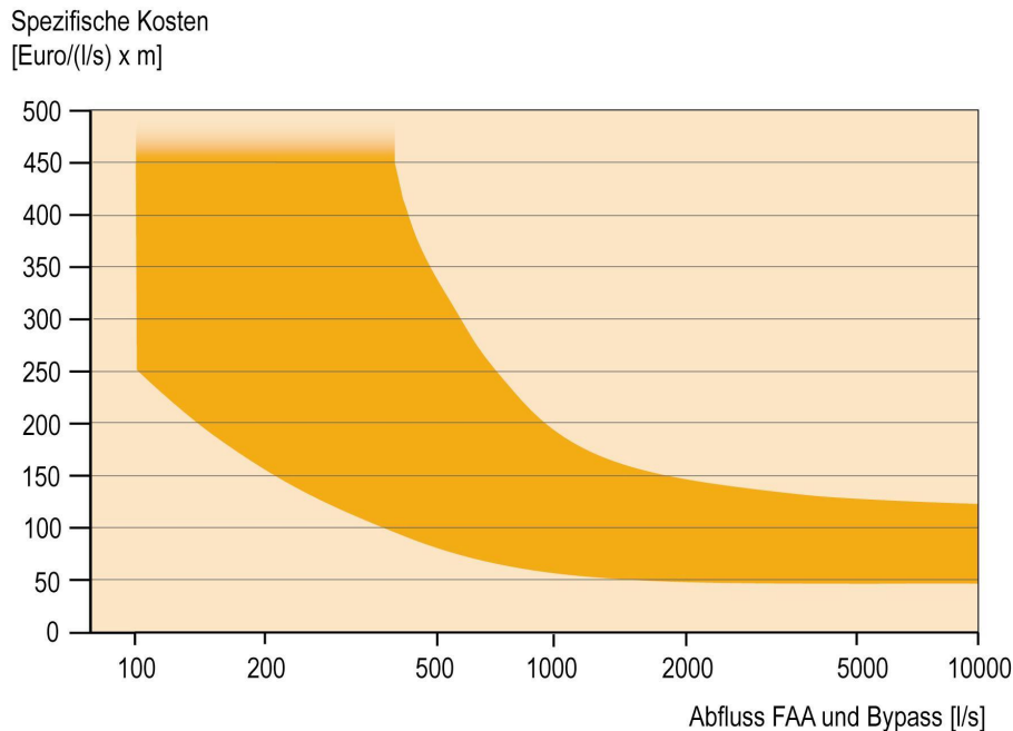
Abb. 4.14: Spezifische Investitionskosten für Fischaufstiegsanlagen, bezogen auf den Abfluss zur Kostenermittlung und die Absturzhöhe
