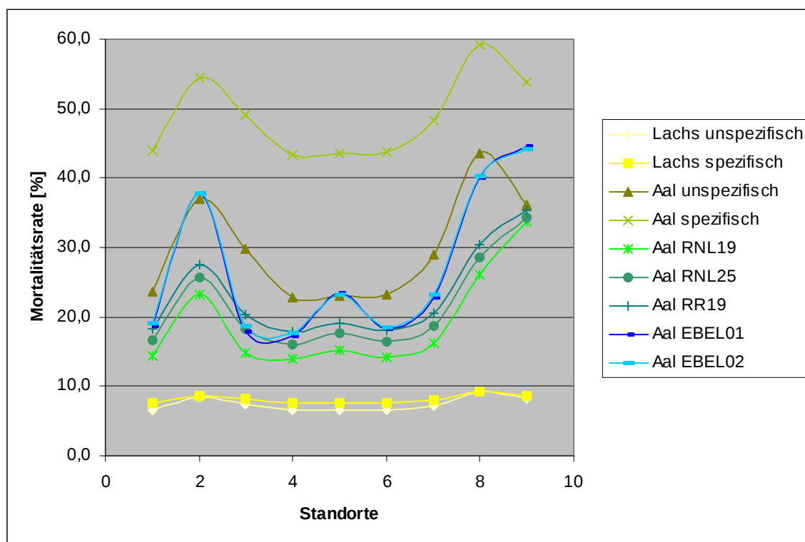
Abb. 4.10: Vergleich der mit den Modellen ermittelten Mortalitätsraten von Blankaaalen bei der Passage von Kaplan-Turbinen
