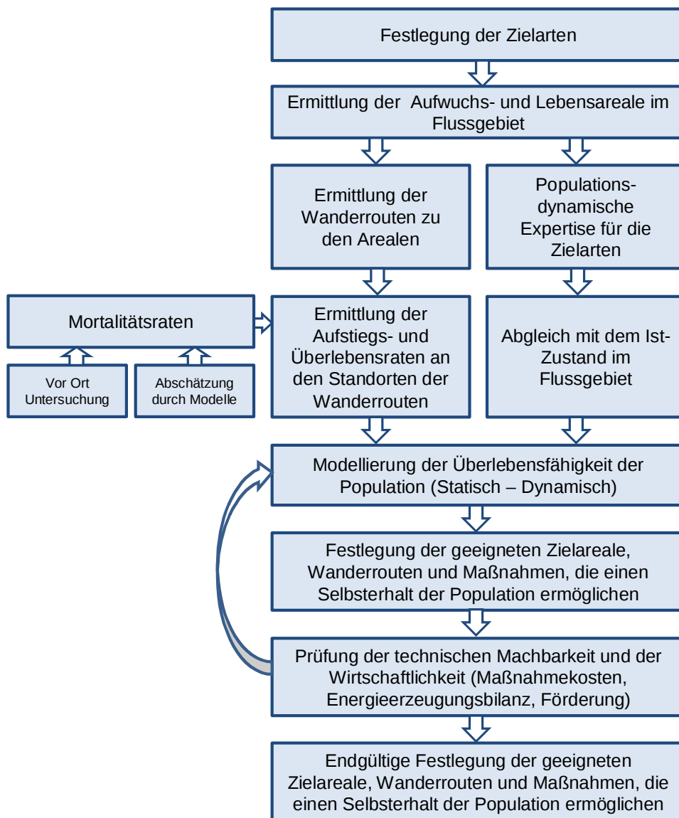
Abb. 8.1: Ablaufschema Flussgebietsstrategie
