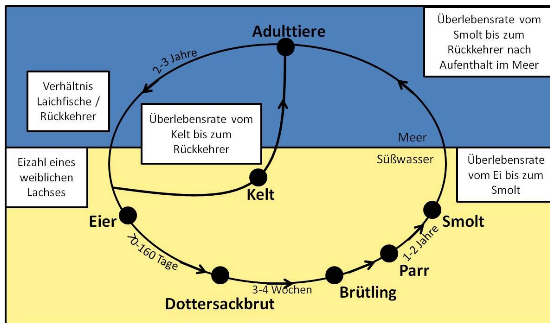
Abb. 4.11: aus THIEL u. MAGATH (2010): Lebenszyklus des Atlantischen Lachses Salmo salar (Linnaeus, 1758) mit Angabe der Lebenszyklus-Abschnitte, für die Teilüberlebensraten ermittelt wurden.
