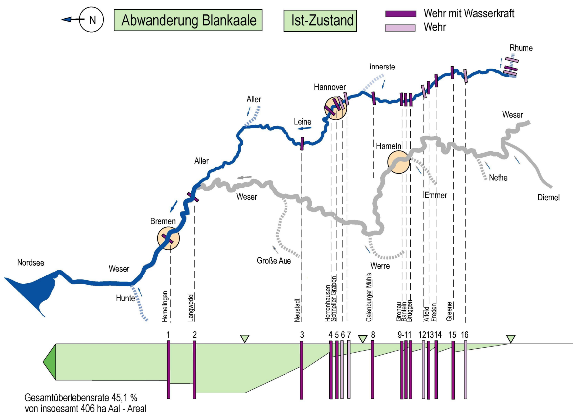
Abb. 5.6: Gesamtüberlebensrate für Aale aus den Leine-Arealen im Ist-Zustand
