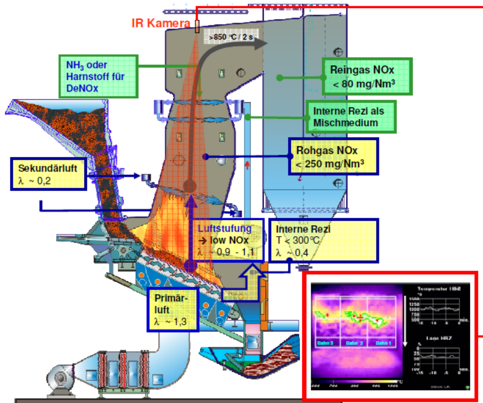
Abbildung 19: Prozessschema für das Very-Low-NO x -Verfahren (NO x -Werte bezogen auf Abgasvolumenstrom i.N. tr. bei 11 Vol.-% O 2 ) [Kor-10].
