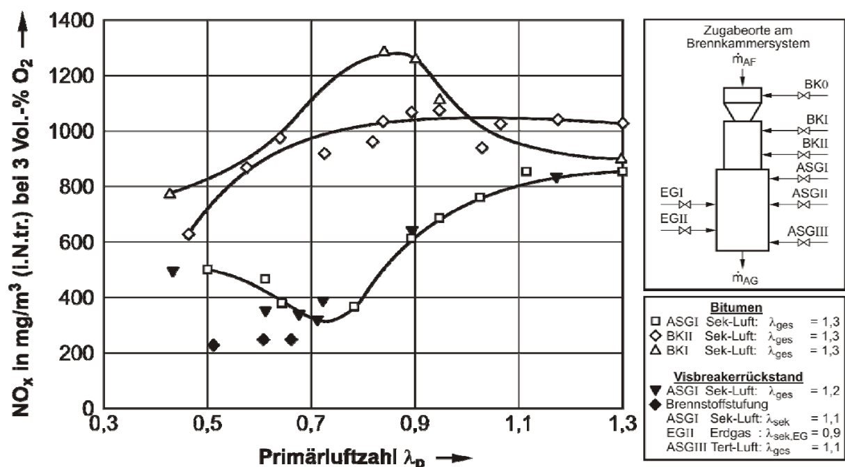
Abbildung 8: Einfluss der Primärluftzahl, des Zugabeortes der Sekundärluft und der Brennstoffstufung auf die \text{NO}_x -Emissionen bei Bitumen und Visbreakerrückständen [MaJ-91].
