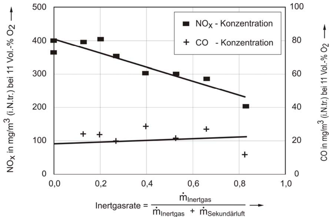
Abbildung 18: NO x - und CO-Rohgaskonzentration in Abhängigkeit von der Inertgasrate, d.h. in Abhängigkeit des die Sekundärluft \dot{m}_{\text{Sekundärluft}} ersetzenden Inertgases \dot{m}_{\text{Inertgas}} in der Nachverbrennungszone [ScB-92].
