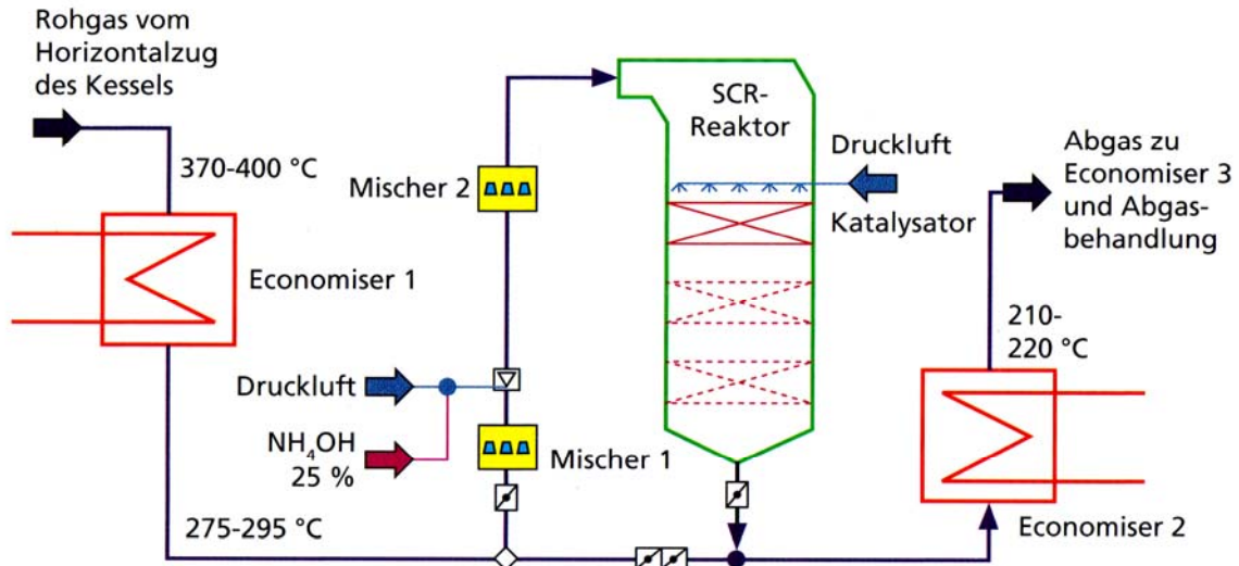
Abbildung 42: Vereinfachtes Prozessfließbild eines High-Dust-SCR mit Plattenkatalysator (Abfallverbrennungsanlage Brescia, Italien) [Schü-08].
