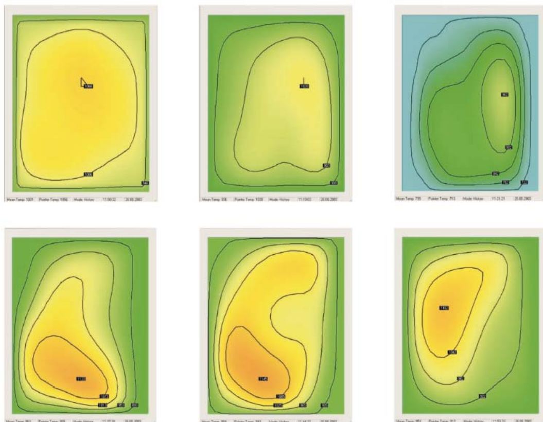
Abbildung 29: Temperaturen in der agam-Messebene einer Abfallverbrennungsanlage innerhalb einer Stunde [vdH-08].
