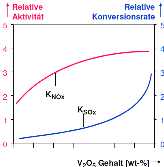
Abbildung 46: Relative \text{NO}_x -Reduktionsaktivität und \text{SO}_2 -Konversionsrate in Abhängigkeit des \text{V}_2\text{O}_5 -Gehaltes eines SCR-Katalysators (Quelle: Johnson Matthey Catalysts (Germany) GmbH).
