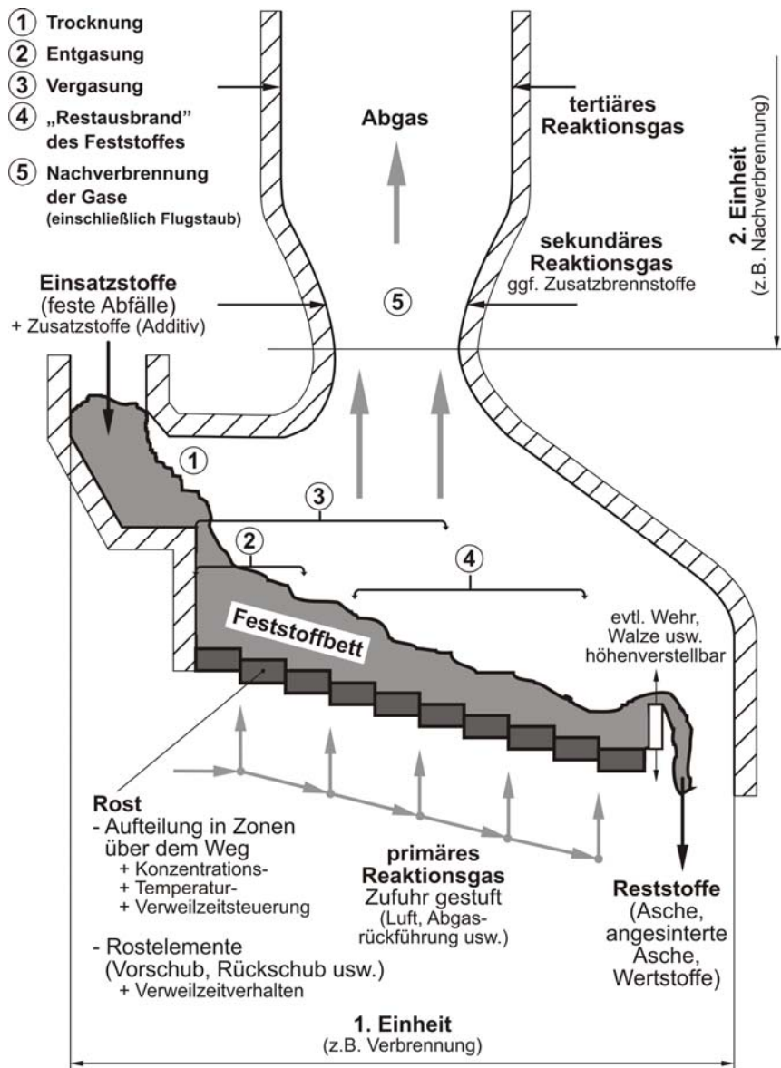
Abbildung 13: Feststoffumsatz auf einem Rost [ScSc-93].
