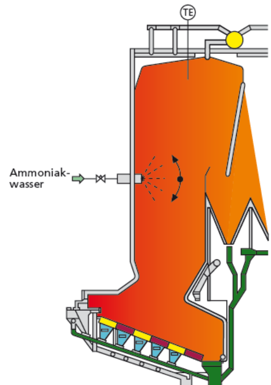
Abbildung 36: Eindüslung von Ammoniakwasser mit Winkeldüsen in einer Ebene [Th-05].
