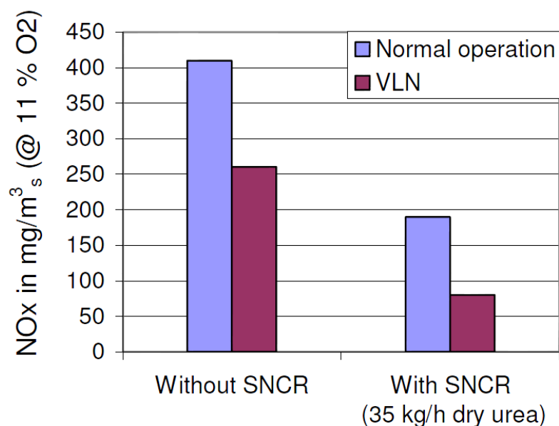
Abbildung 21: Versuchsergebnisse der \text{NO}_x -Minderung mit dem VLN-Verfahren in der Abfallverbrennungsanlage Thiverval/Frankreich 2008 [Go-10].
