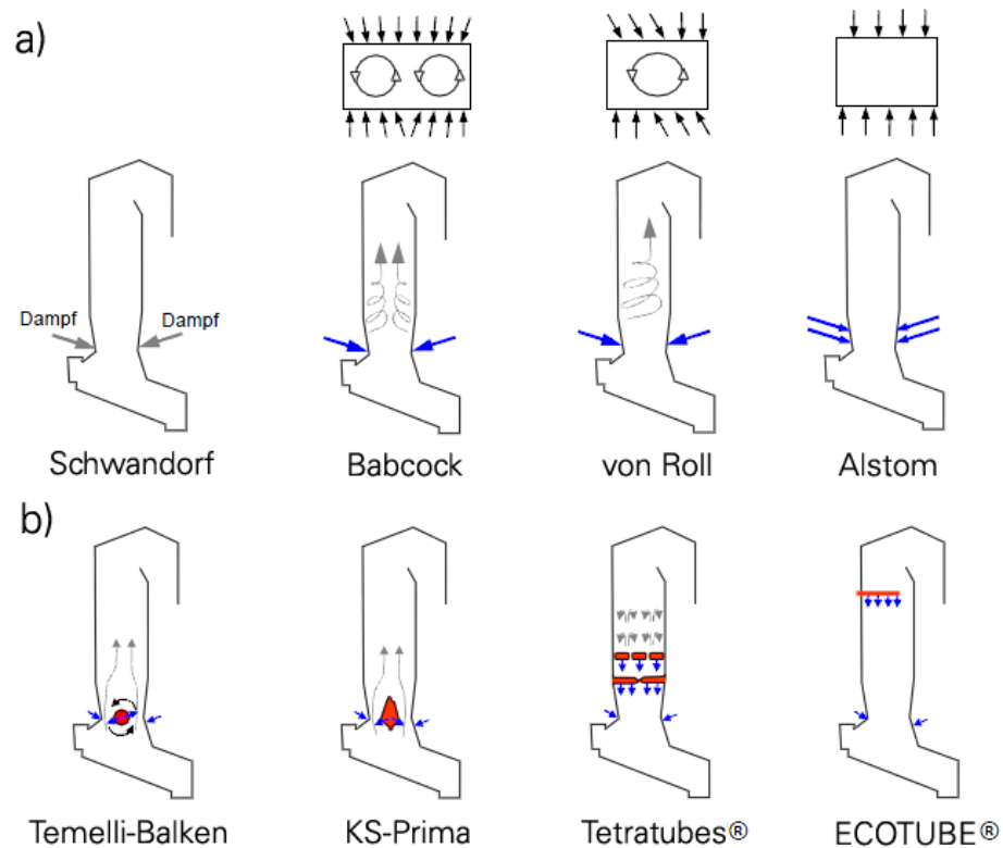
Abbildung 23: Verschiedene Möglichkeiten zur Abgashomogenisierung: a) Eindüsungssysteme; b) Einbauten mit Eindüsung [Schu-07].
