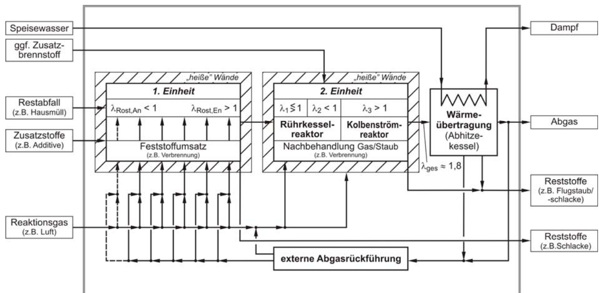
Abbildung 14: Schematische Darstellung der getrennten Prozessführung bei stückigen Abfällen [ScB-91] (bearbeitet).
