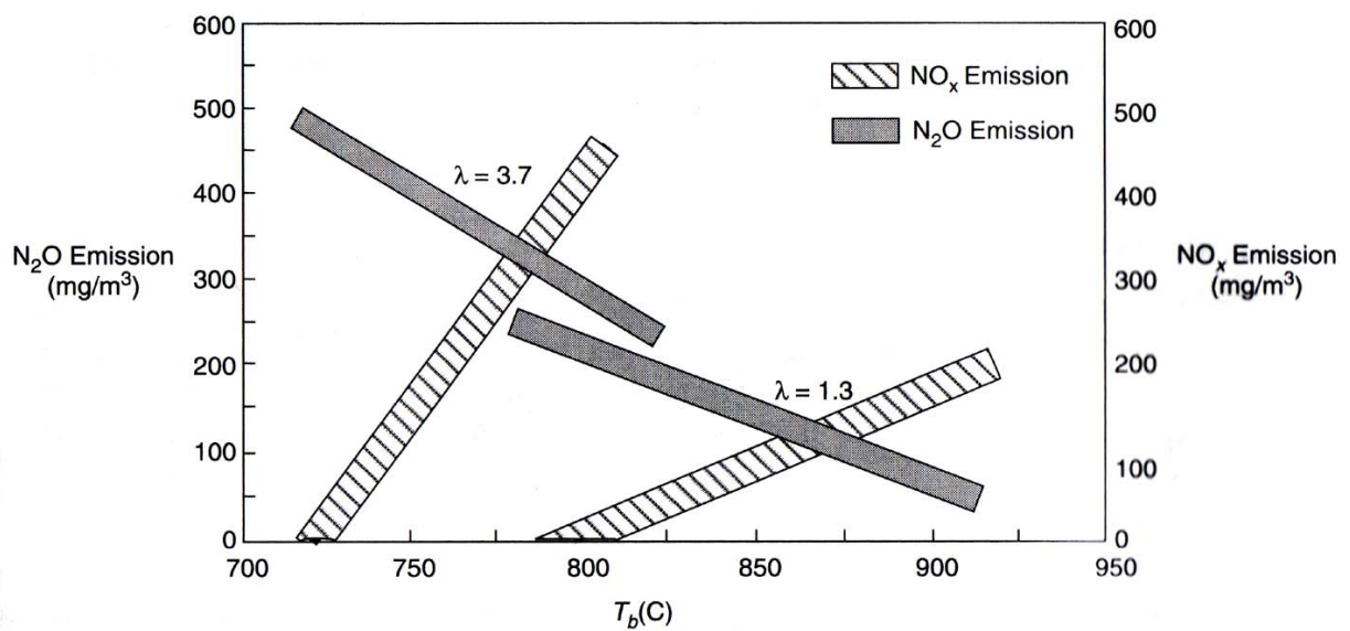
Abbildung 55: NO_x - und N_2O -Emissionen in Abhängigkeit von Temperatur bei einer Wirbelschichtfeuerung mit niederflüchtigen, bituminösen Kohlen. Dicke der Linien stellt die Streuung der Messdaten dar (Quelle: Braun, 1987) [Bas-05].
