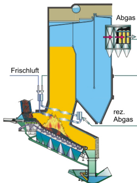
Abbildung 17: Rezirkulation des gekühlten und entstaubten Abgases über die Sekundärluftzuführung (Quelle: offizielle Webseite der Fa. Martin GmbH).
