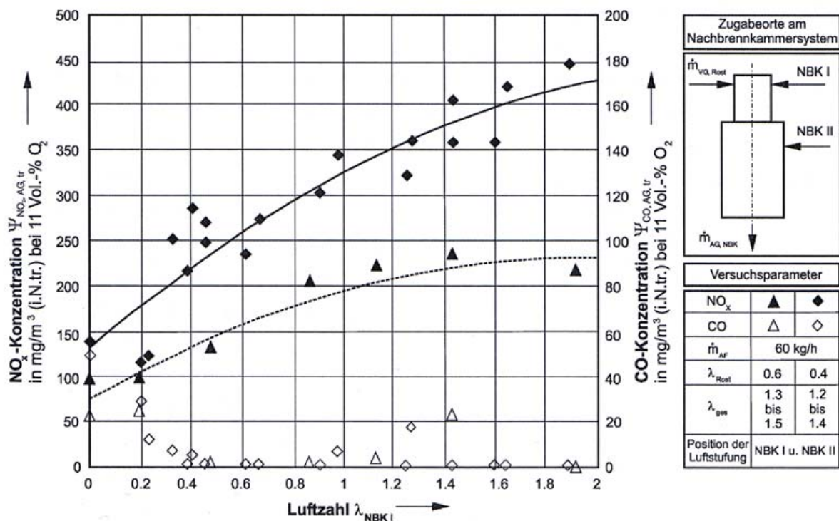
Abbildung 15: \text{NO}_x - und \text{CO} -Konzentrationen in Abhängigkeit von der Luftzahl \lambda_{\text{NBK I}} bei verschiedenen Luftzahlen \lambda_{\text{Rost}} [BeS-97].
