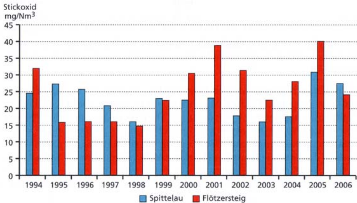
Abbildung 52: Jahresmittelwerte \text{NO}_x von MVA Spittelau und MVA Flötzersteig (beide Anlagen in Wien, Österreich, 1994 - 2006) [KiA-07].
