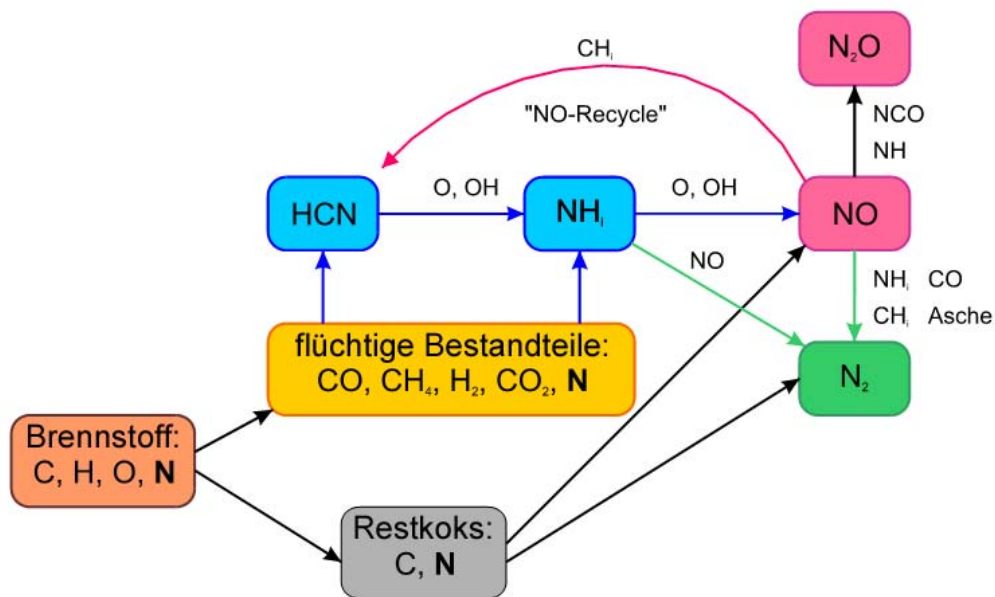
Abbildung 7: Bildungswege von NO und \text{N}_2\text{O} über den Brennstoff-Stickstoff.
