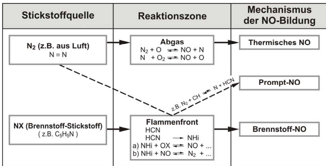
Abbildung 2: Schematische Darstellung der verschiedenen Mechanismen zur NO-Bildung [DeS-81].
