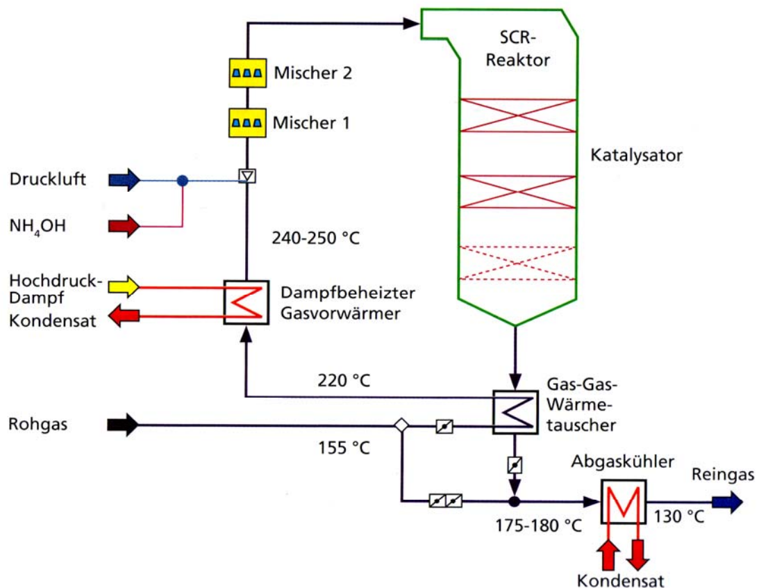
Abbildung 43: Vereinfachtes Prozessfließbild eines Tail-End-SCR mit Wärmeverschiebungssystem und Dampf-Gas-Vorwärmer (Biomasseverbrennungsanlage Hengelo, Niederlande) [Schü-08].
