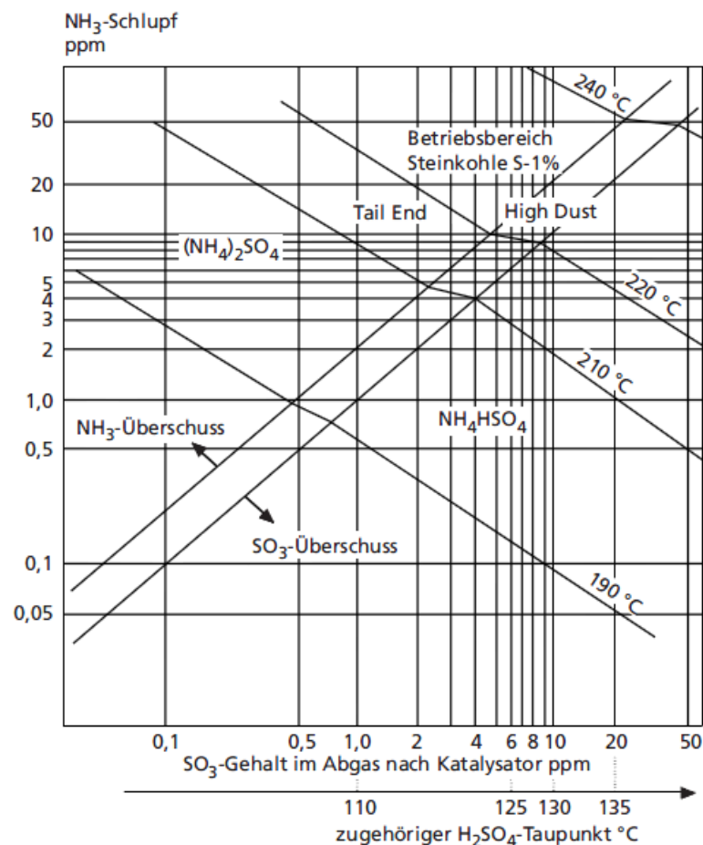
Abbildung 9: Bildungstemperaturen von Ammoniumhydrogensulfat und Ammoniumsulfat in Abhängigkeit von der \text{NH}_3 - und \text{SO}_3 -Konzentration im Abgas [Ve-98].
