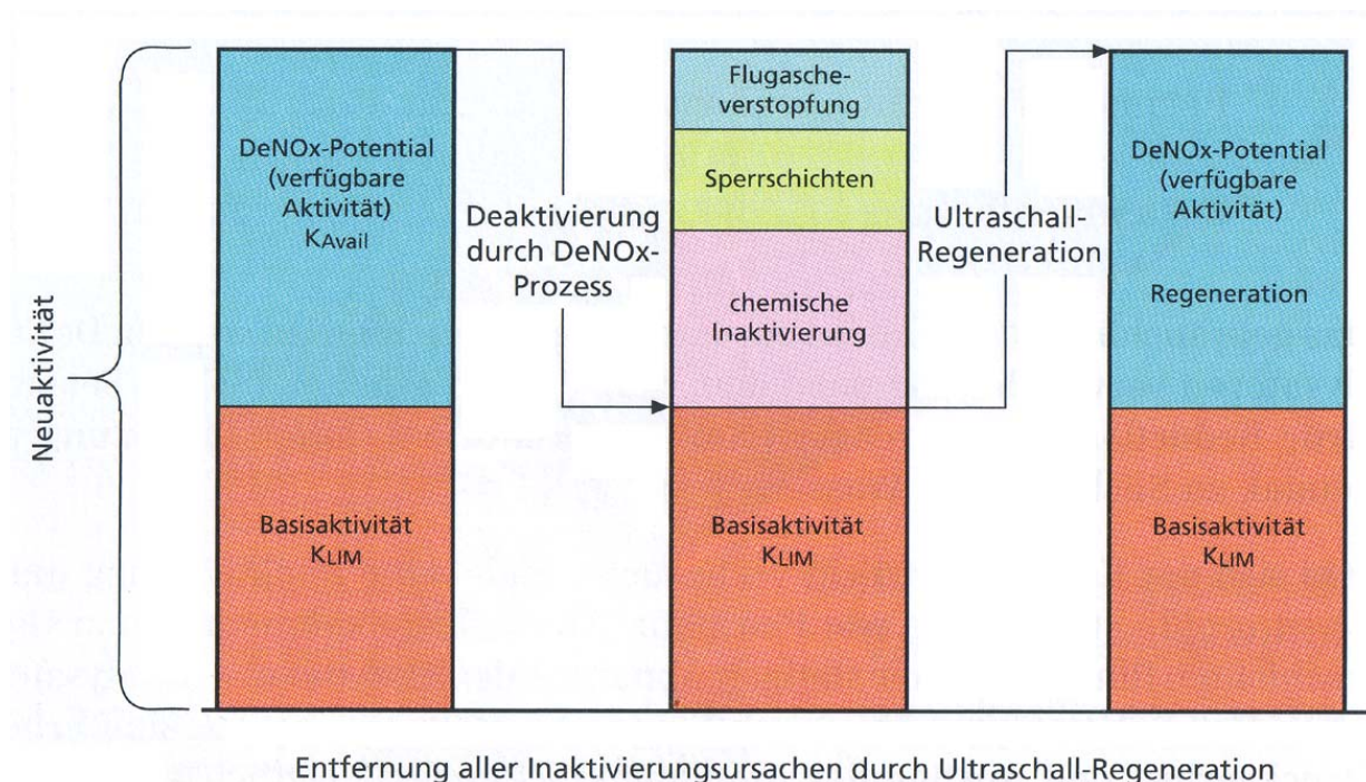
Abbildung 49: Prinzip der Ultraschall-Regeneration von SCR-Katalysatoren [EbS-08].
