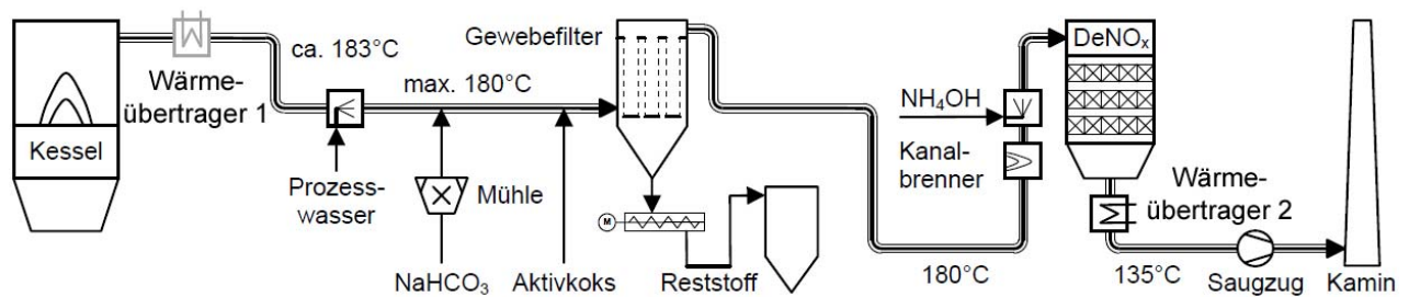
Abbildung 58: Vereinfachtes Verfahrensfliessbild für eine Abfallverbrennungsanlage mit Trockensorptionsverfahren mit Natriumbicarbonat und Tail-End-SCR-Verfahren [BeK-11].
