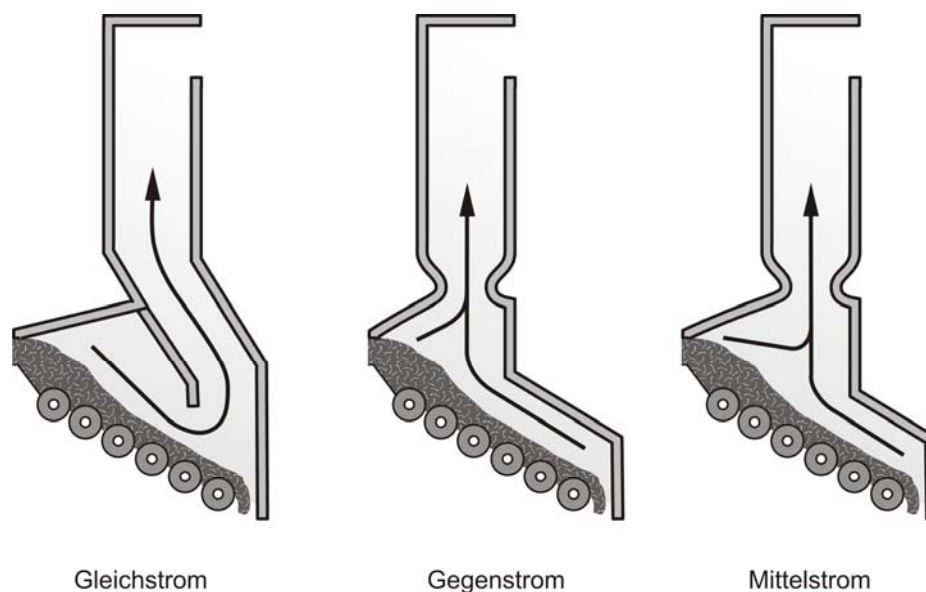
Abbildung 12: Gasstromführung bei Rostsystemen [ScB-01].
