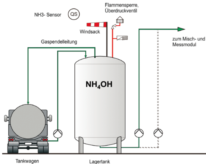
Abbildung 26: Vereinfachtes Fließbild für ein Ammoniakwasserlager [vdHL-10].
