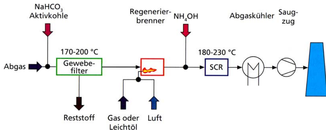
Abbildung 50: Vereinfachtes Fließbild der Abgasreinigung in Abfallverbrennungsanlagen mit einem SCR-Katalysator hinter dem Trockensorptionsverfahren mit Natriumbicarbonat [Schü-08] (bearbeitet).
