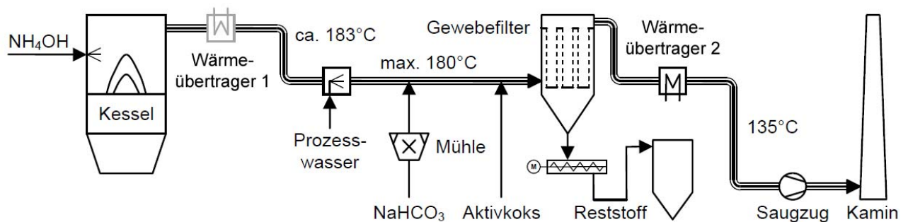
Abbildung 57: Vereinfachtes Verfahrensfliessbild für eine Abfallverbrennungsanlage mit SNCR-Verfahren und Trockensorptionsverfahren mit Natriumbicarbonat [BeK-11].
