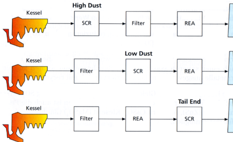
Abbildung 41: Schaltungsvarianten der SCR-Anlage in der Abgasreinigungskette [SchS-08].
