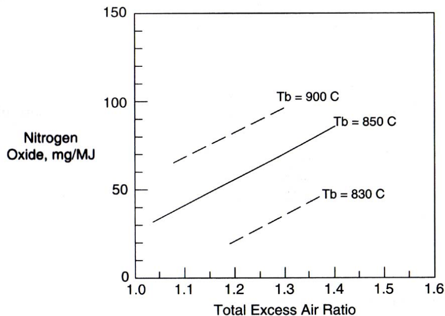
Abbildung 54: Energiebezogene NO_x -Emissionen in Abhängigkeit von Temperatur und Luftüberschuss [Bas-05].
