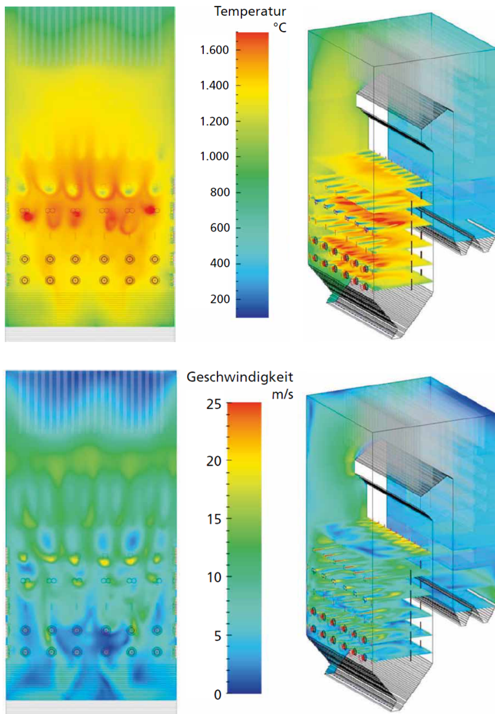
Abbildung 38: CFD-Simulation für einen mit Steinkohle und Biomasse befeuerten Kessel [HuT-10] (bearbeitet).
