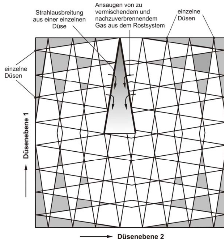
Abbildung 22: Möglichkeiten der Anordnung von Düsenfeldern in zwei Ebenen über einem Strömungsquerschnitt zur Herstellung eines „Rührkessel“-Elementes [ScB-91].
