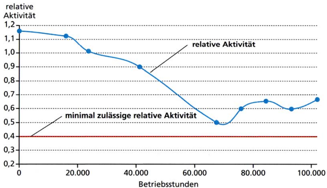
Abbildung 47: Verlauf der relativen Gesamtaktivität eines dreilagigen Katalysators [KiA-07].
