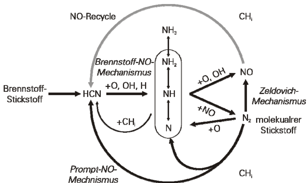
Abbildung 3: Kombination der NO-Bildungsmechanismen [Ko-90].
