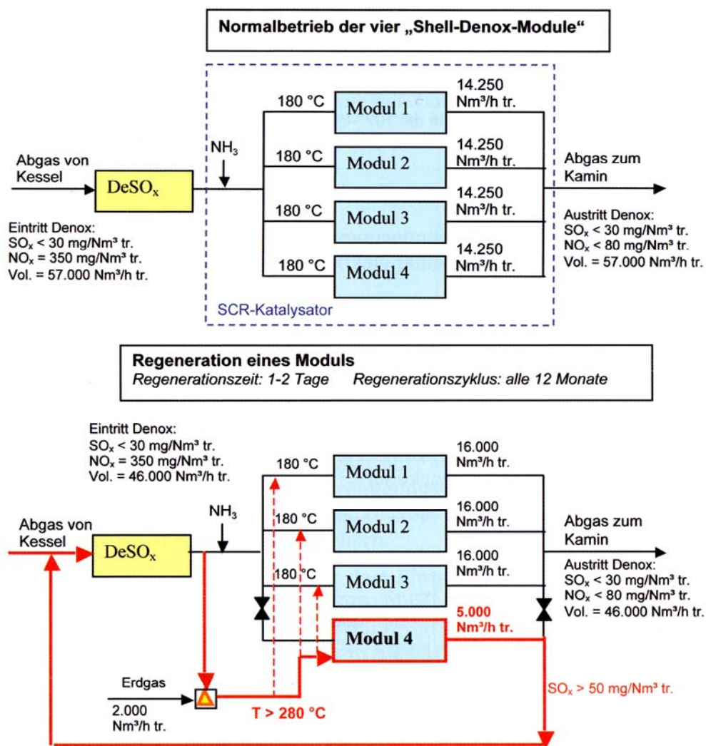
Abbildung 51: Aufbau und Regeneration des Niedertemperaturkatalysators in der Müllverbrennungsanlage Paris, Carrier-sur-Seine (Quelle: Shell, environmental catalysts & systems) [KaK-11].
