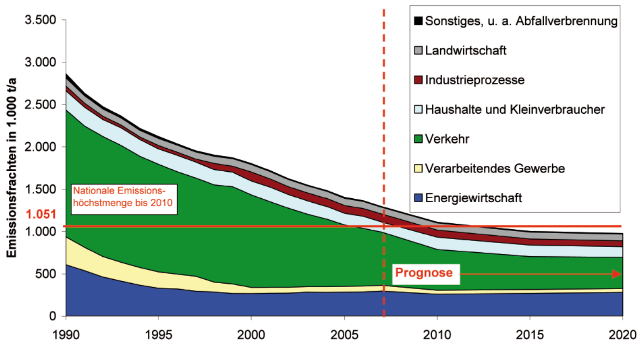
Abbildung 1: Entwicklung der \text{NO}_x -Emissionen in Deutschland von 1990 bis 2007 sowie Prognose bis 2020. (Quelle: Umweltbundamt: Emissionen ausgewählter Luftschadstoffe nach Quellengruppen in Deutschland 1990 bis 2007) [Löt-10].
