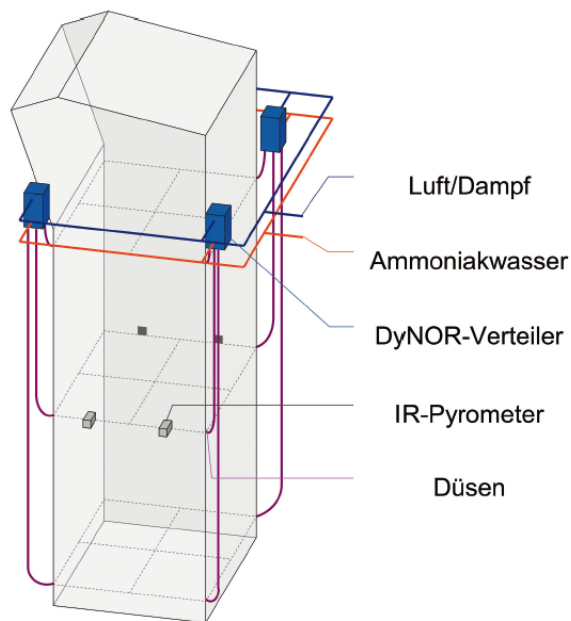
Abbildung 33: SNCR-Verfahren mit Infrarot(IR)-Strahlungspyrometer [BaS-10].
