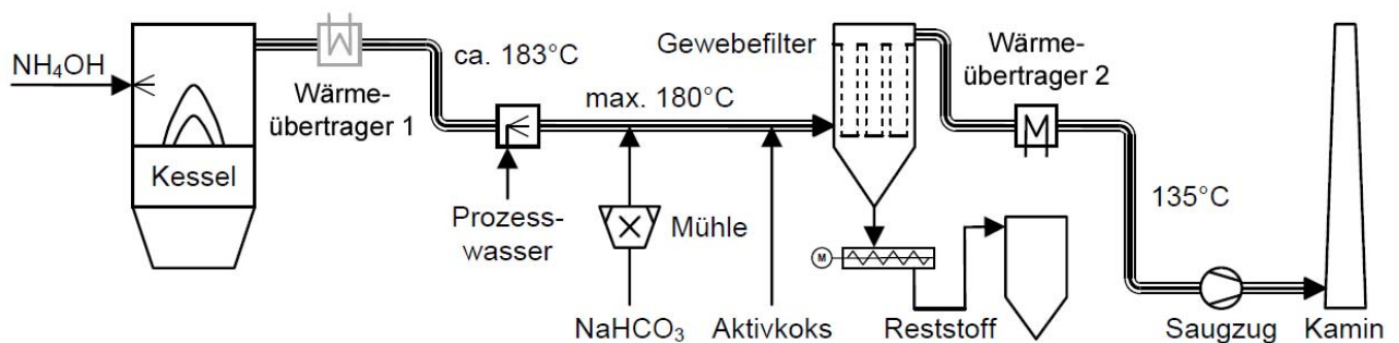
Abbildung 59: Vereinfachtes Verfahrensfliessbild für eine Abfallverbrennungsanlage mit SNCR-Verfahren und Trockensorptionsverfahren mit Natriumbicarbonat [BeK-11].
