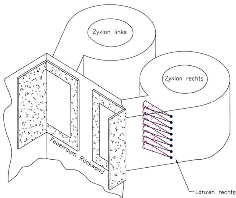
Abbildung 56: Positionierung der Eindüslanzen am Zyklon einer zirkulierenden Wirbelschichtfeuerung [TuM-10].
