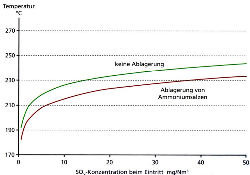
Abbildung 48: Betriebstemperaturen für SCR-Anlagen in Abhängigkeit der \text{SO}_x -Konzentration [Fu-09].
