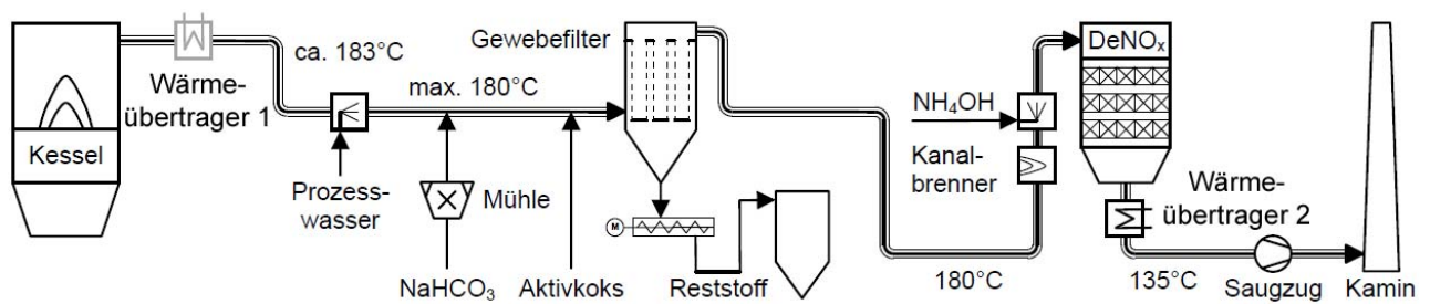
Abbildung 60: Vereinfachtes Verfahrensfliessbild für eine Abfallverbrennungsanlage mit Trockensorptionsverfahren mit Natriumbicarbonat und Tail-End-SCR-Verfahren [BeK-11].
