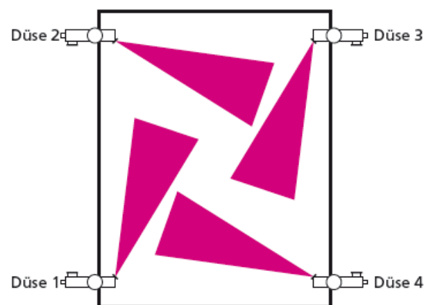
Abbildung 35: Tangentiale Eindüstechnik mit Zweistoff-Winkeldüsen in Abfallverbrennungsanlagen [DiN-02].
