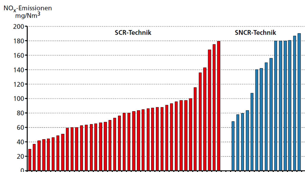
Abbildung 11: \text{NO}_x -Emissionen beim Einsatz von SCR- und SNCR-Technik in der Abfallverbrennung [La-08].
