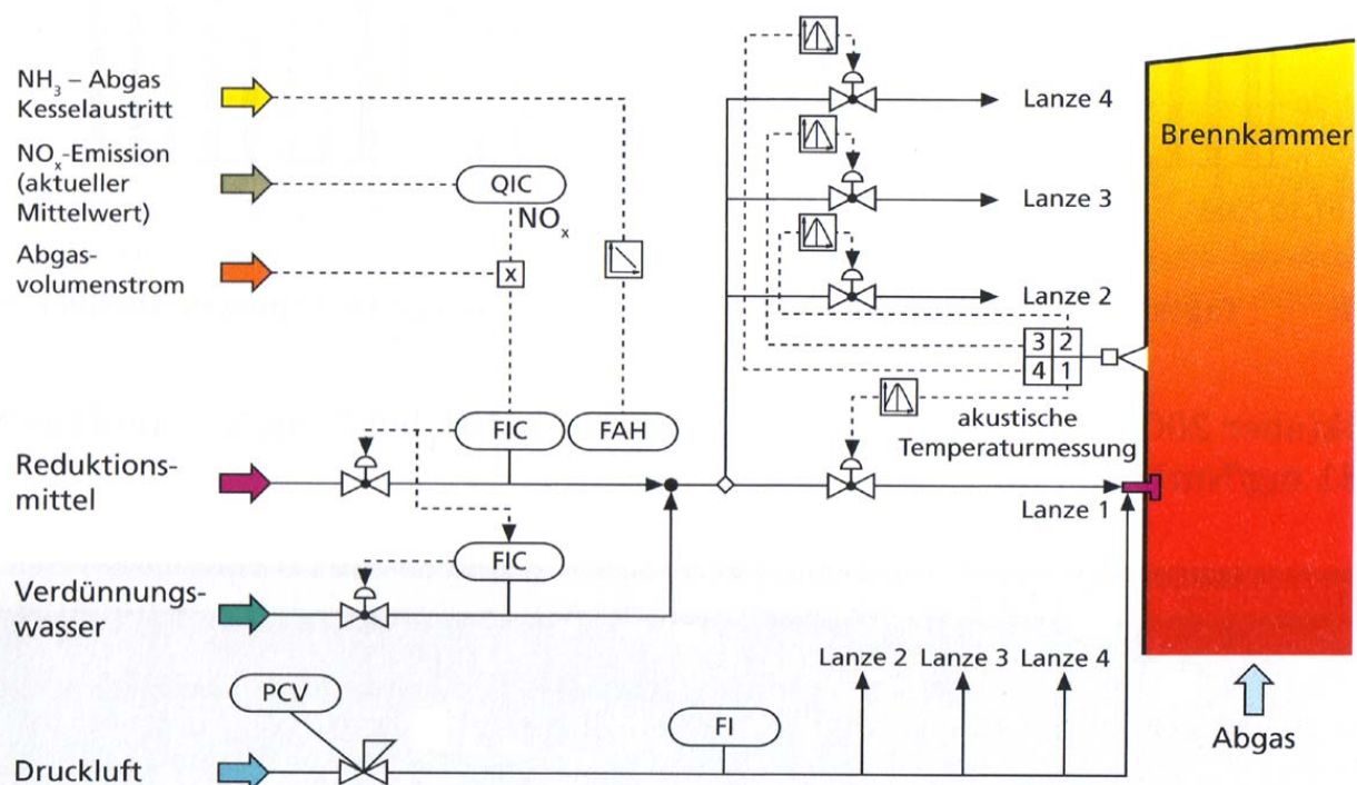
Abbildung 37: Steuerung der Reduktionsmitteldosierung - Lanzeneinzelreglung - in Kombination mit akustischer Temperaturmessung [Rey-09].
