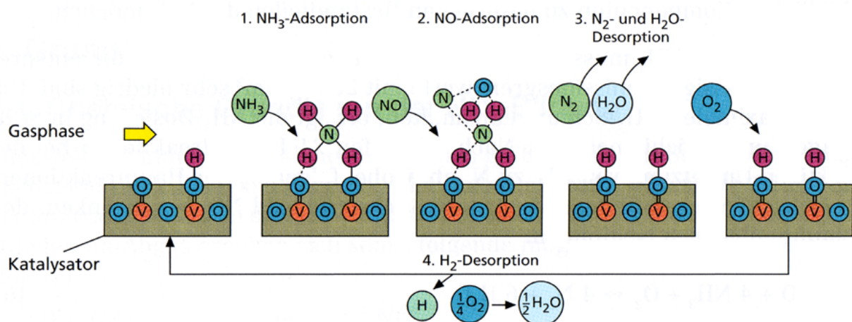
Abbildung 40: Schematische Darstellung der Reaktionen an den aktiven Zentren des Katalysators [Krü-08].
