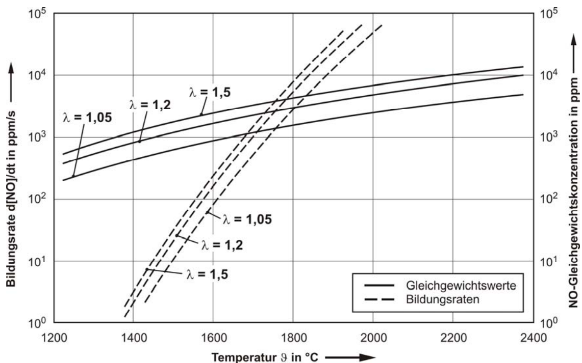
Abbildung 4: NO-Bildung nach dem Zeldovich-Mechanismus für eine Erdgasverbrennung [LeR-79].
