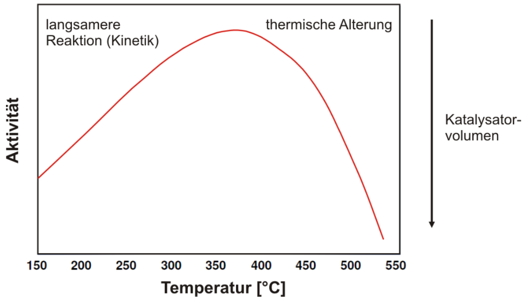
Abbildung 45: Typische Aktivitätskurve eines vanadiumhaltigen SCR-Katalysators auf Basis Titanoxid (Quelle: Johnson Matthey Catalysts (Germany) GmbH; bearbeitet).
