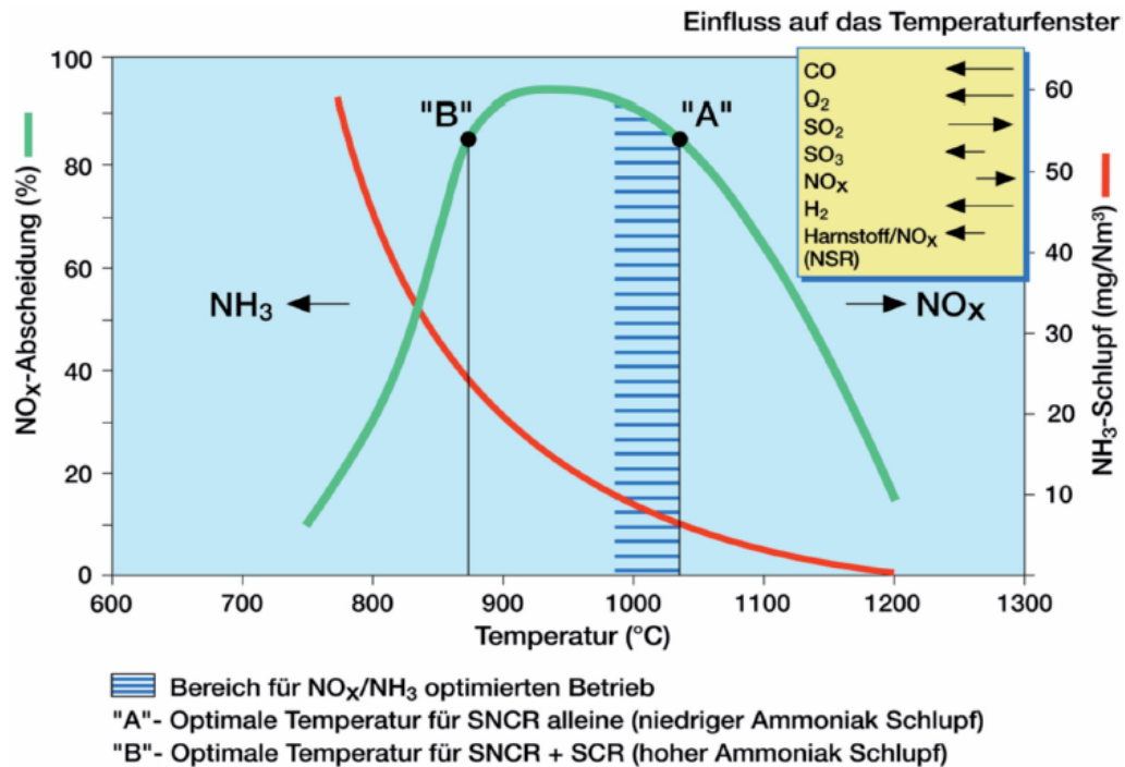
Abbildung 24: NO x -Reduzierung in Abhängigkeit von der Temperatur [vdH-11].
