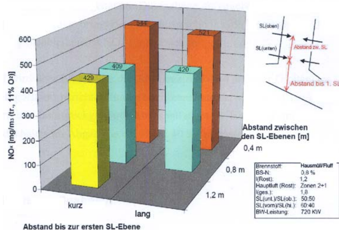
Abbildung 16: \text{NO}_x -Konzentrationen bei Variation der Verweilzeit vor und zwischen den Sekundärluftebenen [WaD-03].
