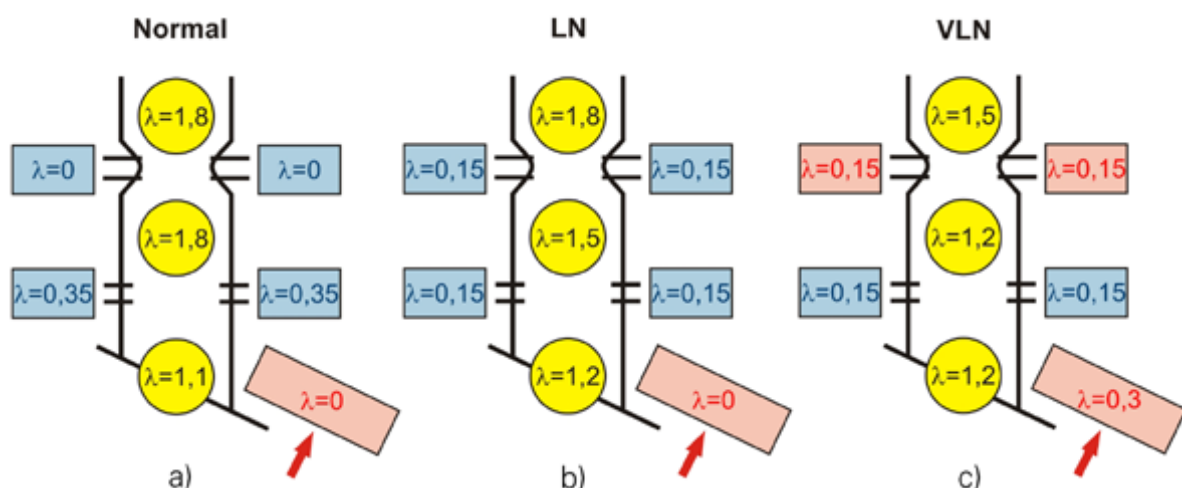
Abbildung 20: Verteilung der Verbrennungsluft bzw. Abgasrezirkulation bei verschiedenen Primärmaßnahmen (Quelle: offizielle Webseite der Fa. MARTIN GmbH).
