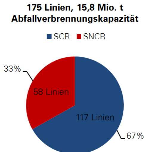
Abbildung 10: SCR-Anlagen in deutschen Hausmüllverbrennungsanlagen [Scha-08].
