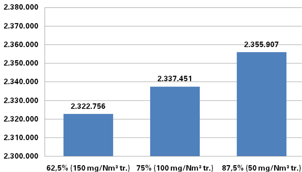
Abbildung 62: Vergleich der Betriebsmittelkosten für die Abgasreinigung mit SCR-Verfahren für unterschiedliche NO x -Reduktionsleistungen (Einheit: €/Jahr).
