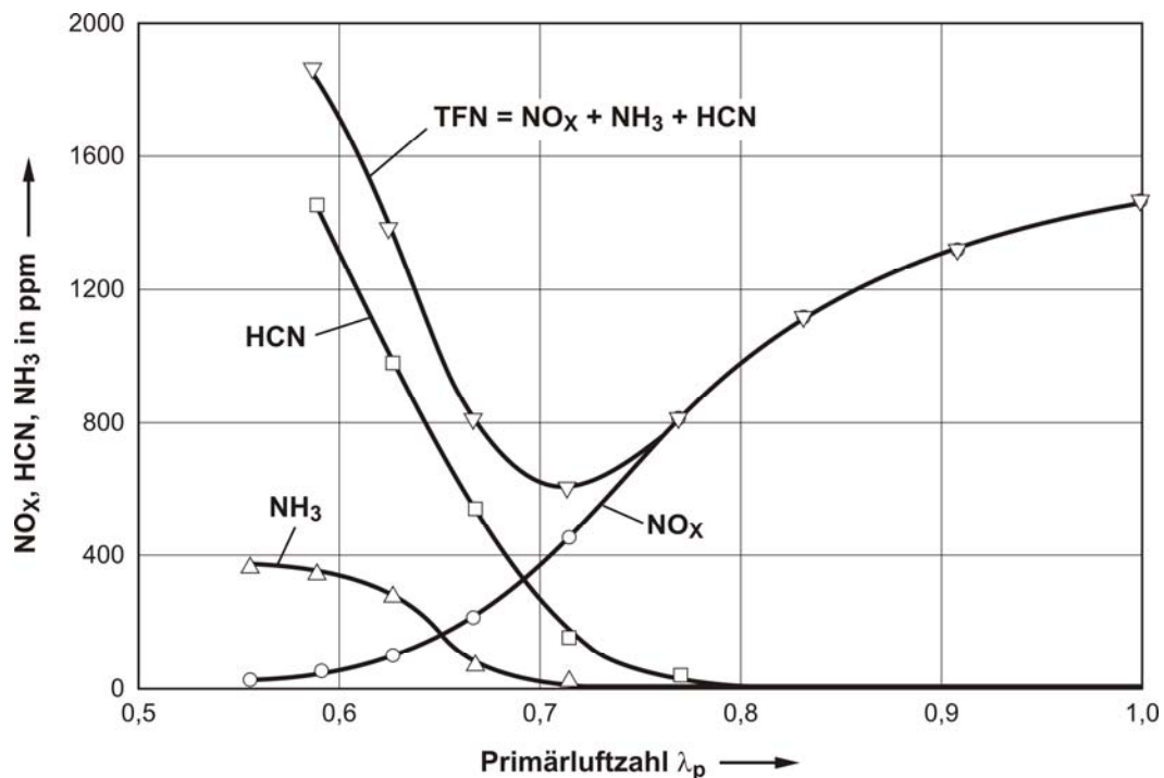
Abbildung 6: Einfluss der Primärluftzahl auf die Bildung von \text{NO}_x , \text{HCN} und \text{NH}_3 bei einer mit Methylamin ( \text{CH}_3\text{NH}_2 ) dotierten Propan-Luft-Vormischflamme (aus [EbJ-83] nach [Kr-86]).
