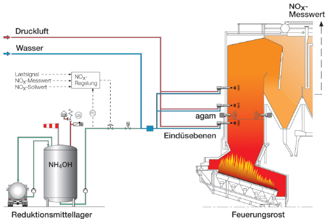
Abbildung 34: Verfahrensfliessbild einer mit agam optimierten SNCR-Anlage mit Ammoniakwasser [vdHL-11].
