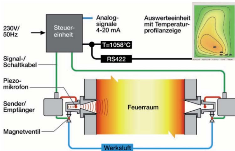
Abbildung 30: Prinzipieller Aufbau des akustischen Gastemperaturmesssystems (agam) [vdH-08].
