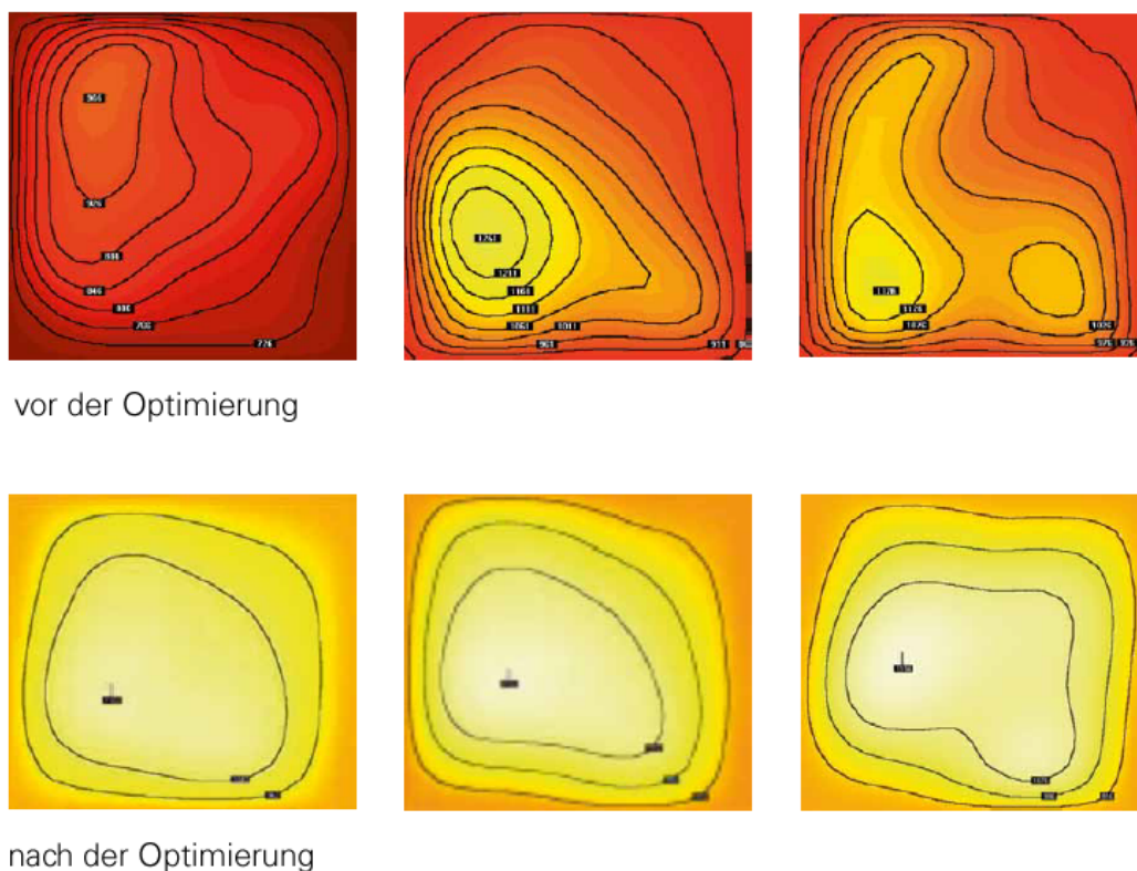
Abbildung 32: Temperaturverteilung (°C) über den Feuerraumquerschnitt vor und nach der Optimierung mit einem akustischen Gastemperaturmesssystem [HuT-10].
