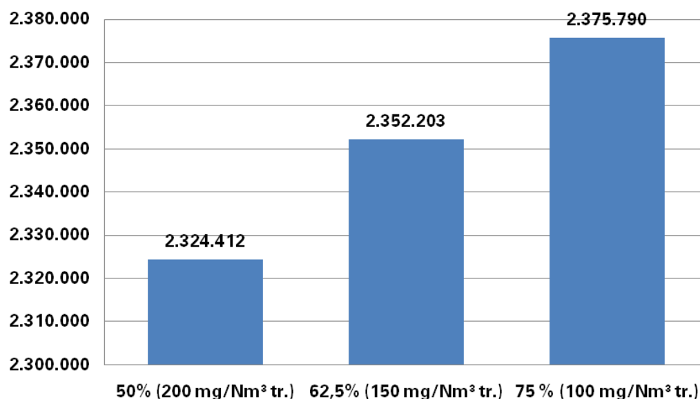
Abbildung 61: Vergleich der Betriebsmittelkosten für die Abgasreinigung mit SNCR-Verfahren für unterschiedliche NO x -Reduktionsleistungen (Einheit: €/Jahr).
