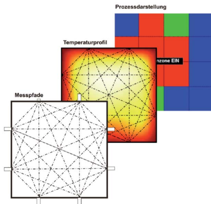
Abbildung 31: Beispiel für die Anordnung und Aufteilung der Messstellen des akustischen Gastemperaturmesssystems (agam) [vdH-11].
