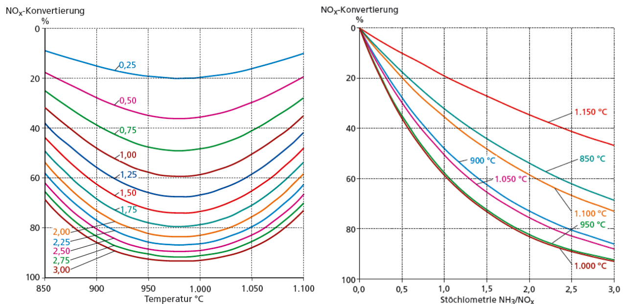
Abbildung 27: \text{NO}_x -Konvertierung nach dem SNCR-Verfahren in Abhängigkeit von Stöchiometriefaktoren und Temperaturen [DiN-02].
