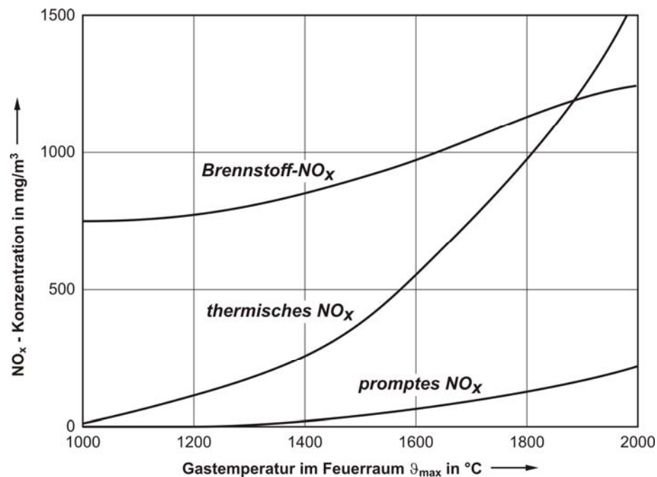
Abbildung 5: Verlauf der NO x -Bildung in Abhängigkeit von der maximalen Gastemperatur im Feuerraum für unterschiedliche Bildungsmechanismen in einer Kohlenstaubfeuerung [ScS-85].
