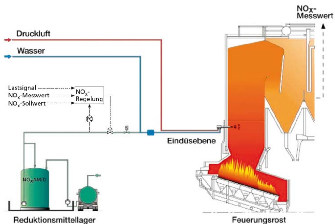
Abbildung 28: Verfahrensfliessbild einer klassischen SNCR-Anlage mit Harnstofflösung [vdH-08].
