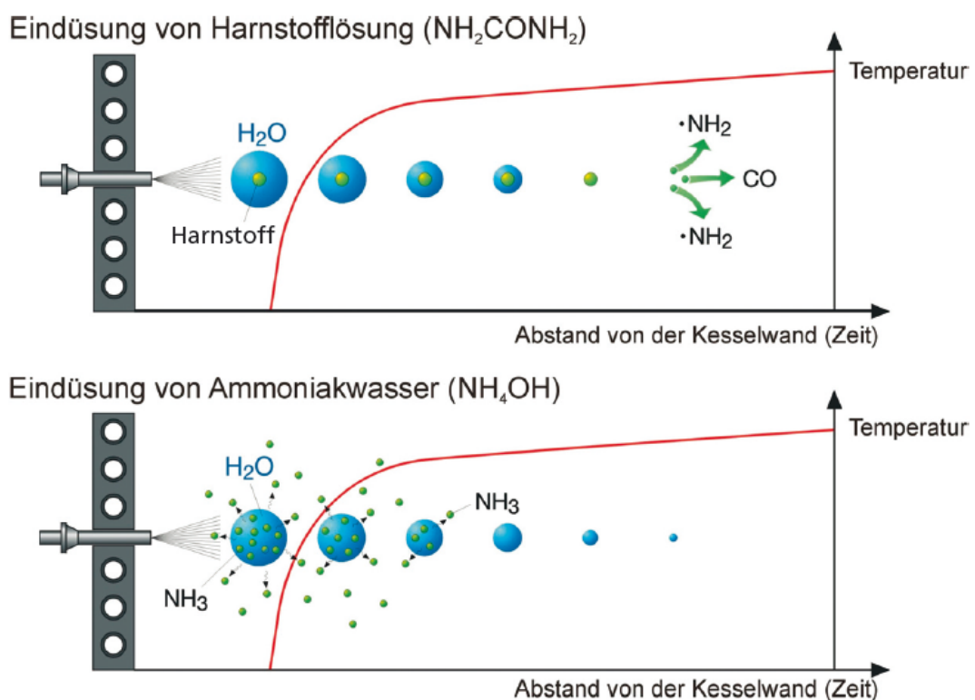
Abbildung 25: \text{NO}_x -Reduzierung mit Harnstofflösung im Vergleich zu Ammoniakwasser [vdH-08].
