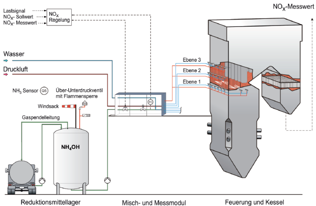
Abbildung 53: Vereinfachtes Verfahrensfliessbild für ein Kombi-Verfahren mit einem Plattenkatalysator im Kessel [vdH-11].
