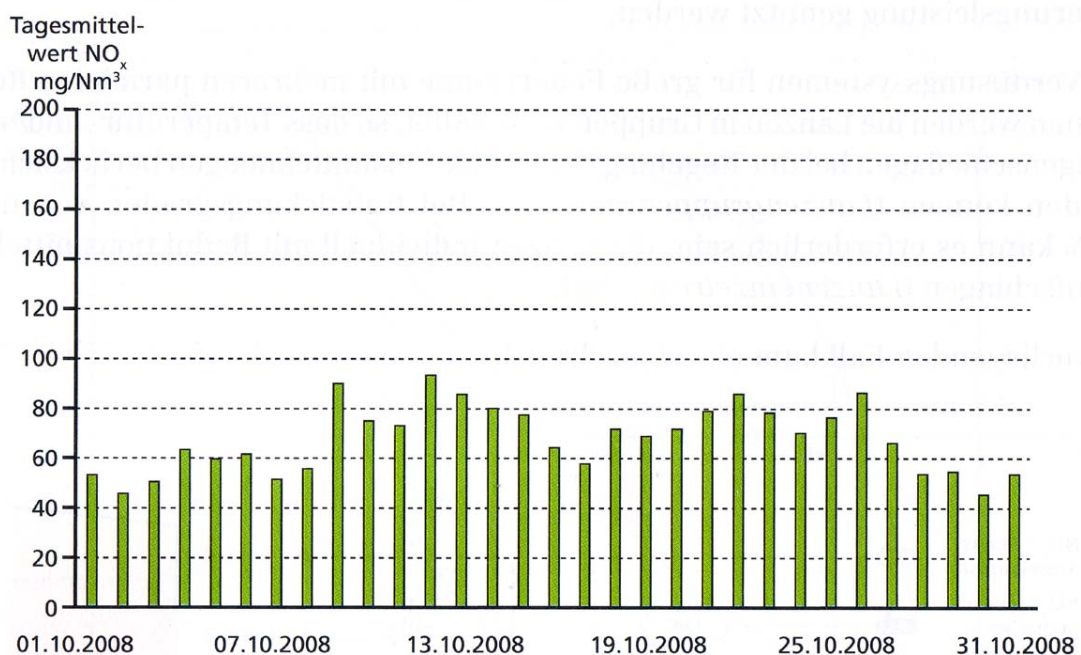
Abbildung 39: Tagesmittelwerte der \text{NO}_x -Emissionen der Anlage Linköping (Schweden) im Oktober 2008 [Rey-09].
