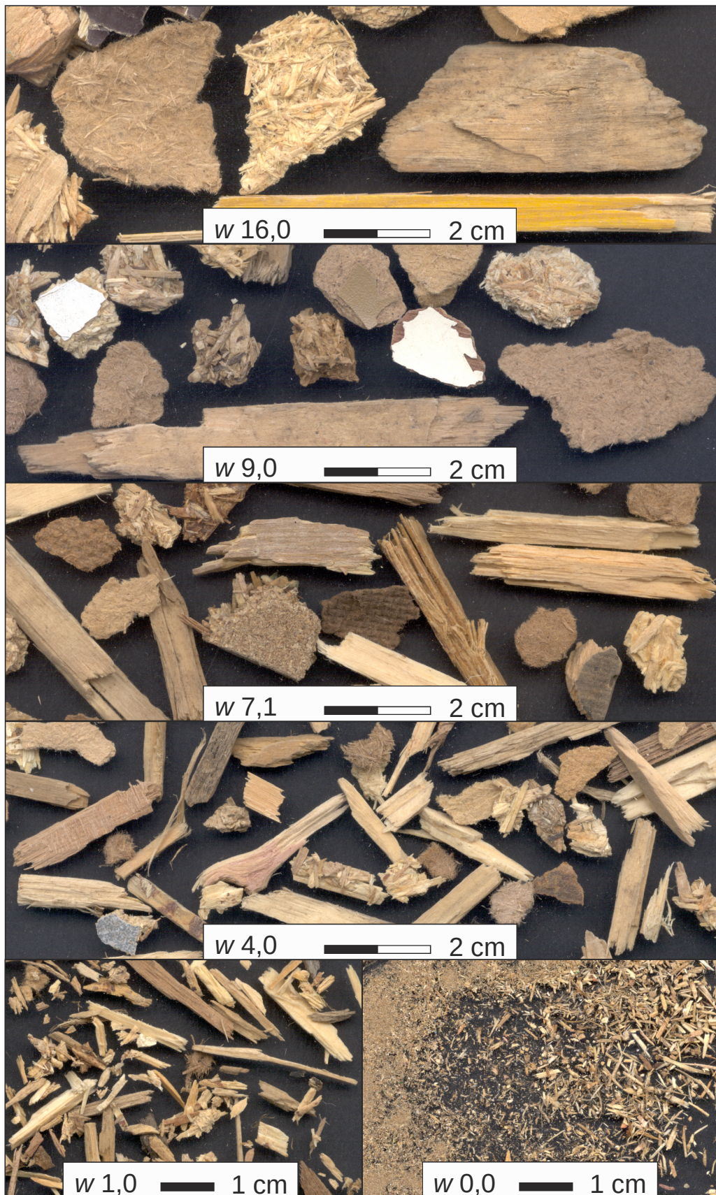
Untersuchungsmaterial 2_1: Fotografische Darstellung der Siebrückstände, Nennöffnungsweite w in mm.
