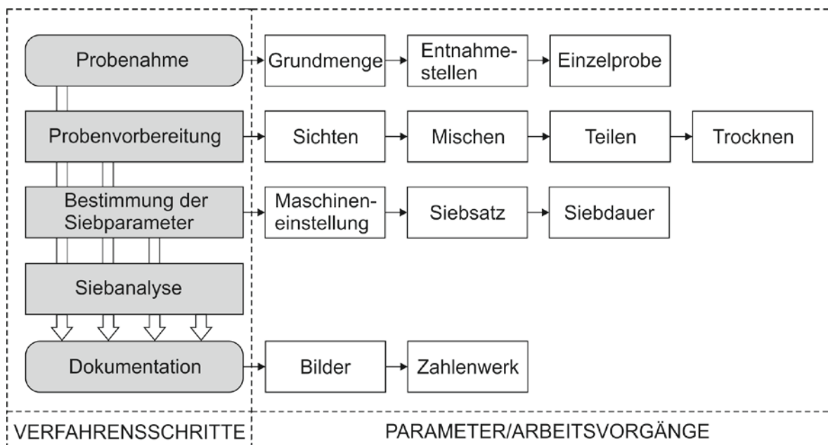
Abbildung 6: Verfahrensschritte, Parameter und Arbeitsvorgänge für die Siebanalyse von Hackschnitzeln.
