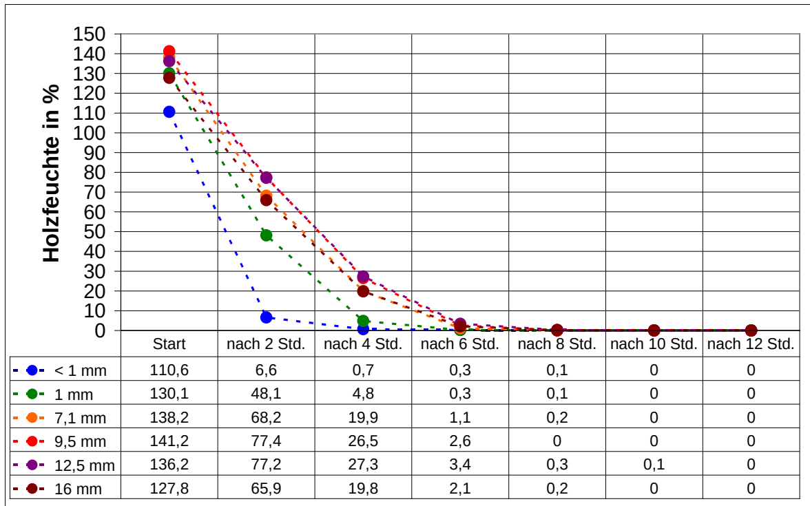
Abbildung 3: Trocknungsverhalten von sechs Fraktionen aus dem Untersuchungsmaterial 1 - Holzfeuchte.
