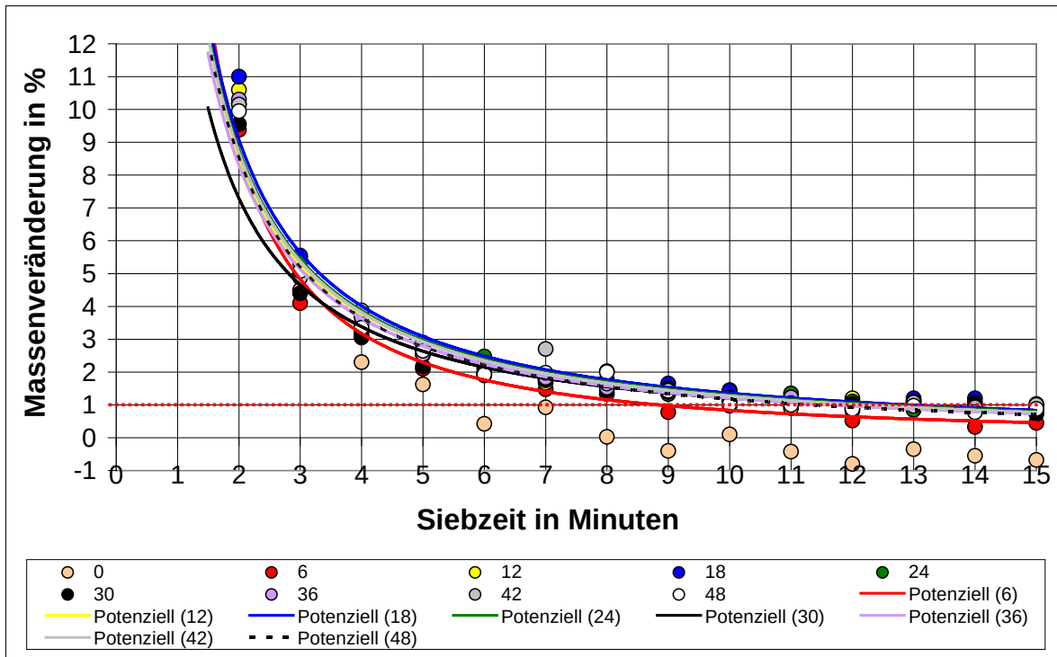
Abbildung 4: Massenveränderungen der Durchgänge durch das Sieb mit der Nennöffnungsweite 1 mm nach jeweils einer Minute Siebung für Proben mit unterschiedlich langen Trocknungszeiten (0 bis 48 Stunden); ein Datenpunkt stellt den Mittelwert von vier Analysenproben dar.
