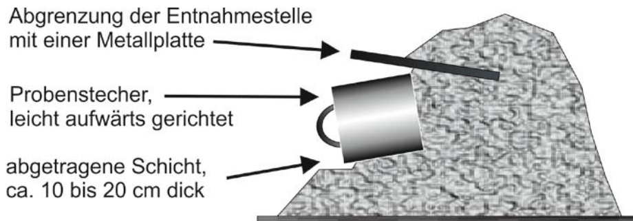
Abbildung 8: Prinzipskizze zur Entnahme einer Einzelprobe.
