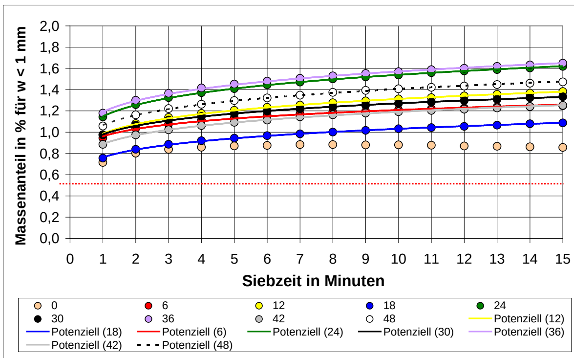
Abbildung 5: Massenanteile der Durchgänge (atro) durch das Sieb mit der Nennöffnungsweite 1 mm bezogen auf die Einwaagen (atro) nach jeweils einer Minute Siebung für Proben mit unterschiedlich langen Trocknungszeiten (0 bis 48 Stunden); ein Datenpunkt stellt den Mittelwert von vier Analysenproben dar.
