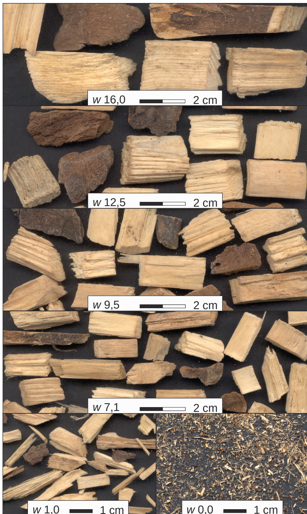
Untersuchungsmaterial 3: Fotografische Darstellung der Siebrückstände, Nennöffnungsweite w in mm.
