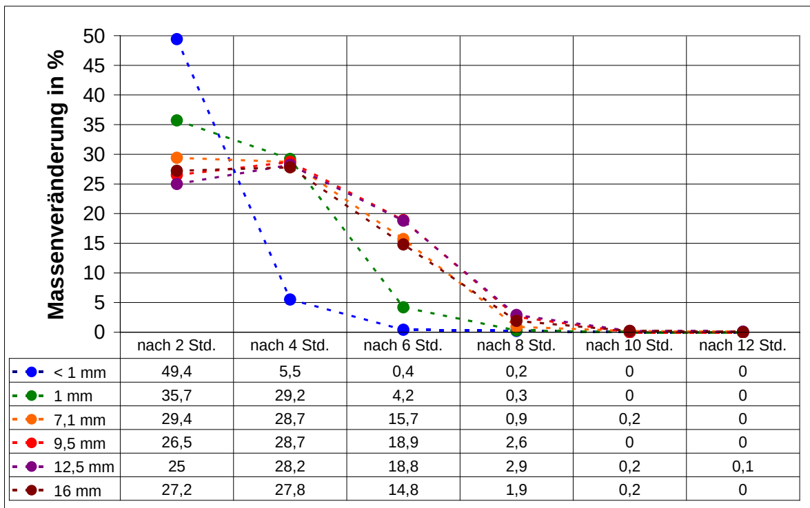
Abbildung 2: Trocknungsverhalten von sechs Fraktionen aus dem Untersuchungsmaterial 1 - Massenveränderung.
