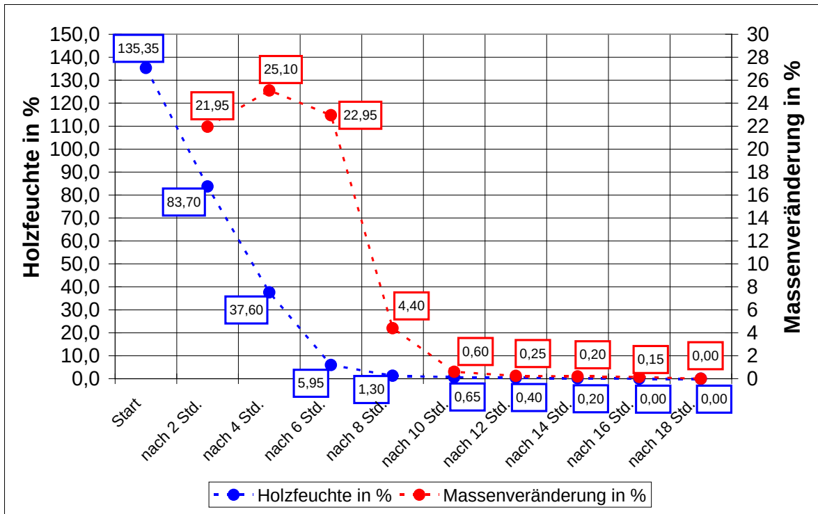
Abbildung 1: Trocknungsverhalten einer Probe aus unterschiedlich großen Hackschnitzeln (Untersuchungsmaterial 1) mit zunehmender Trocknungsdauer.
