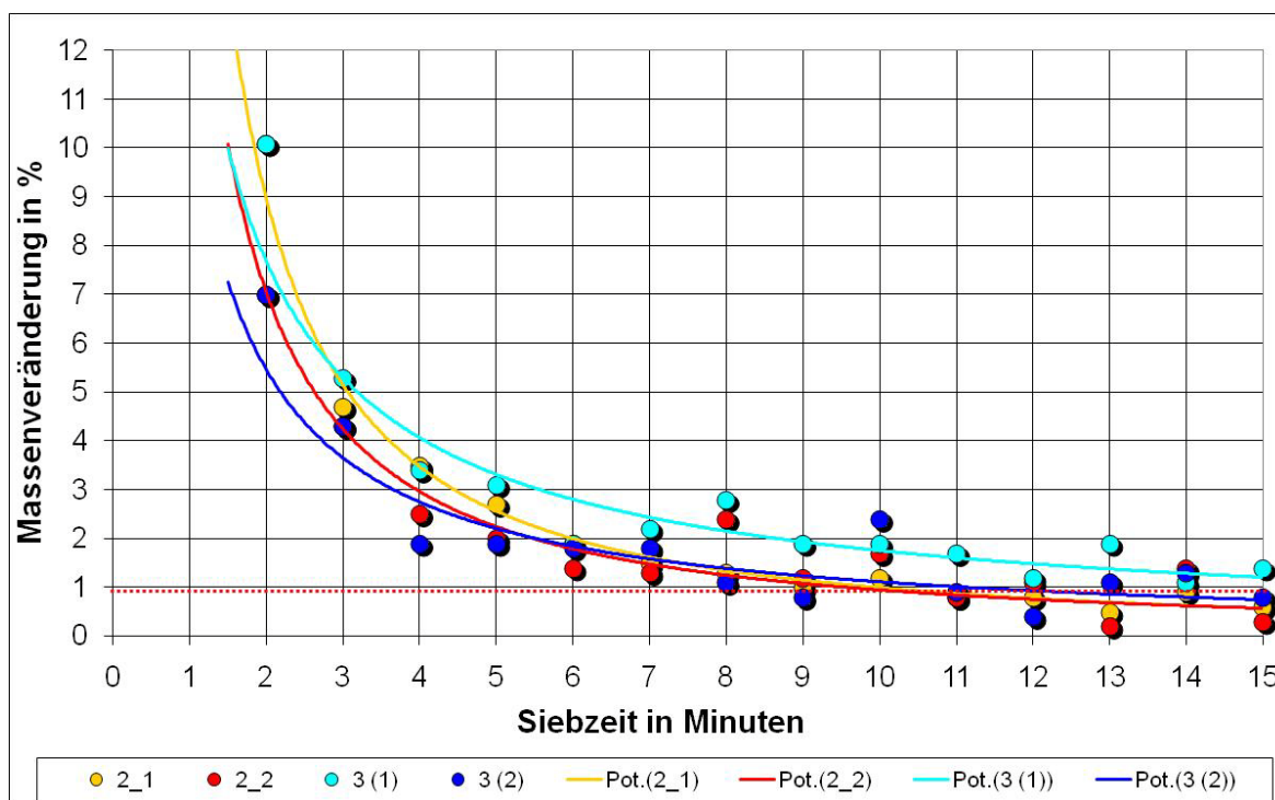
Abbildung 12: Diagramm zur Ermittlung der Siebdauer für die Untersuchungsmaterialien 2_1, 2_2 und 3. Für das Untersuchungsmaterial 3 werden die Werte von zwei Versuchen aufgeführt [3 (1), 3 (2)].
