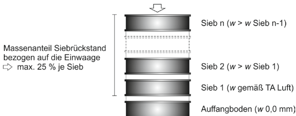
Abbildung 10: Prinzipskizze zum Aufbau des Siebsatzes (w: Nennöffnungsweite des Siebes).
