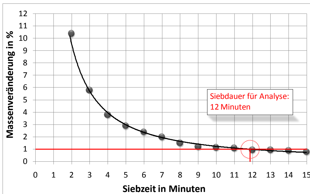
Abbildung 11: Exemplarische Darstellung zur Ermittlung der Siebdauer.
