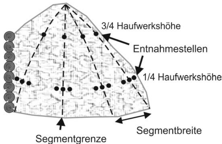
Abbildung 7: Prinzipskizze zu Segmentgrenzen mit Entnahmestellen bei einem kegelförmigen Haufwerk, das nicht umlaufend beprobt werden kann.
