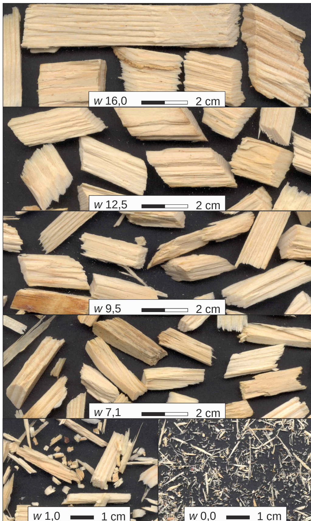
Untersuchungsmaterial 1: Fotografische Darstellung der Siebrückstände, Nennöffnungsweite w in mm.
