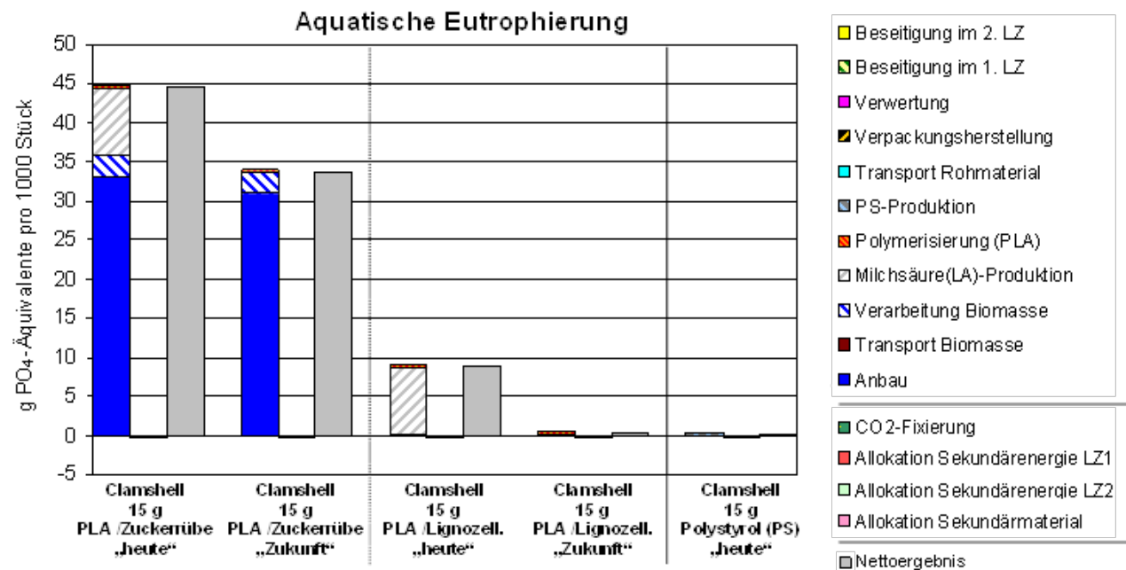
Abbildung 24: Ökobilanzieller Vergleich von Klappdeckelschalen aus PLA und PS (Ergebnisse für den Indikator aquatische Eutrophierung)
