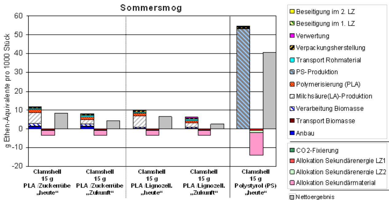
Abbildung 21: Ökobilanzieller Vergleich von Klappdeckelschalen aus PLA und PS (Ergebnisse für den Indikator Sommersmog POCP)
