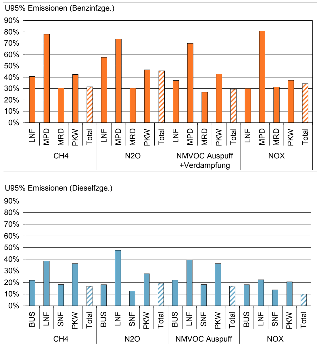
Abb. 11: Unsicherheit der Auspuff-Emissionen je Fahrzeugkategorie - Ebene 3 (volle Balken) und aggregiert auf Stufe Straßenverkehr - Ebene 2 (schraffierte Balken).
