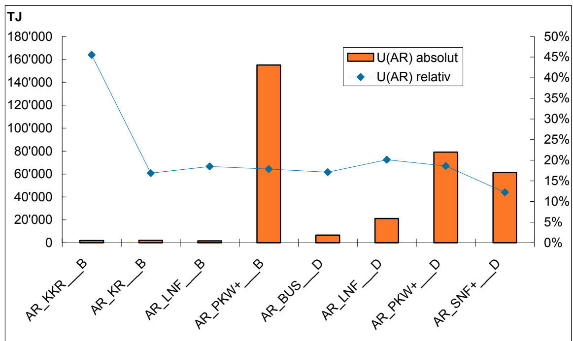
Abb. 9 Unsicherheiten Aktivitätsraten für die Fahrzeugkategorien, d.h. auf Ebene 3 (Fahrzeugkategorien). Säulen: absolute Werte in TJ, Punkte: relative Werte in Prozent des Mittelwerts.
