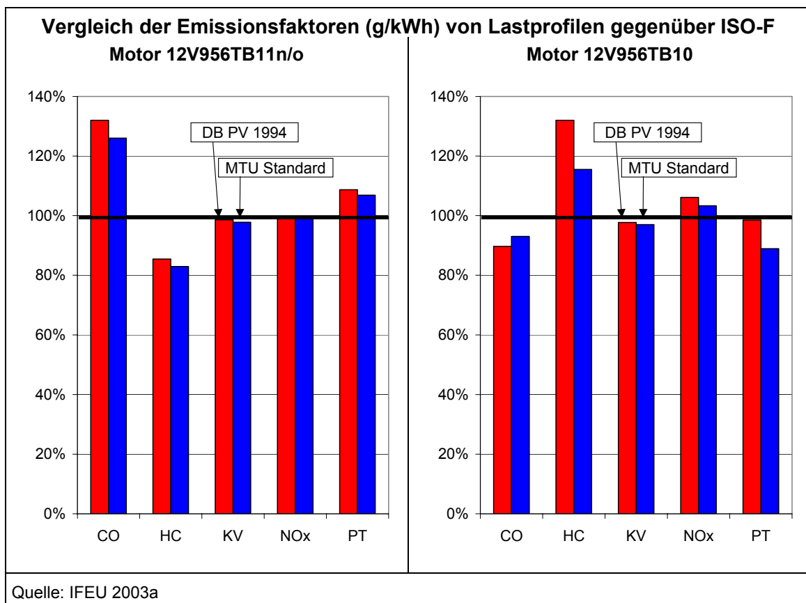
Abb. 13 Emissionsfaktoren verschiedener Lastprofile im Vergleich zum ISO-F-Zyklus
