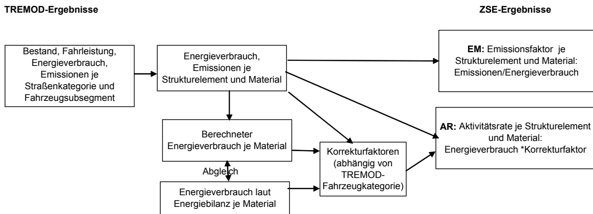
Abb. 1 Übergabe der Aktivitätsraten und Emissionsfaktoren des Straßenverkehrs von TREMOD in das ZSE
