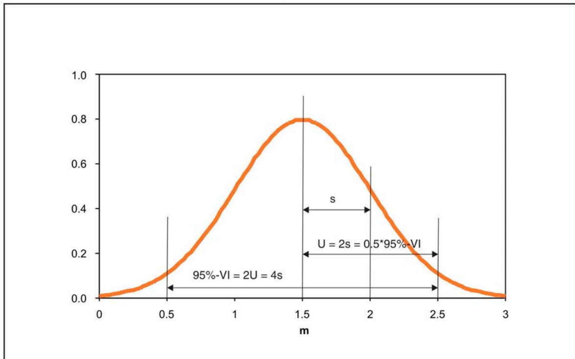
Abb. 2 Standardabweichung s , Unsicherheit U (95%) und 95%-Vertrauensintervall bei einer Normalverteilung.
