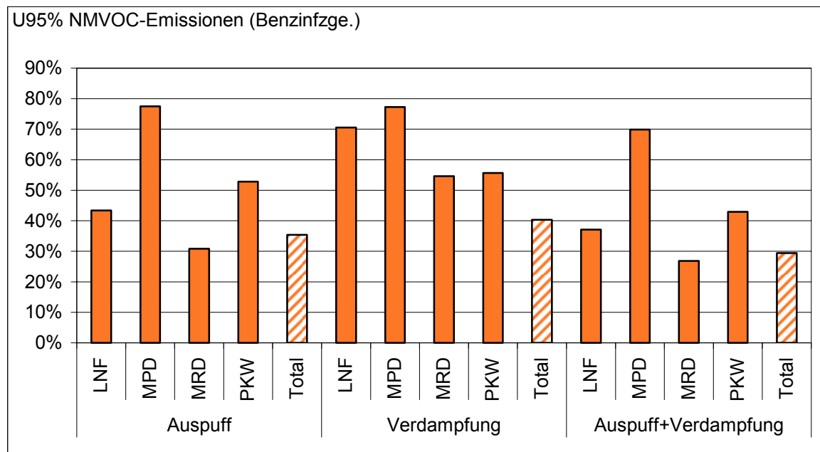
Abb. 12: Unsicherheit der NMVOC-Emissionen je Fahrzeugkategorie - Ebene 3 (volle Balken) und aggregiert auf Stufe Straßenverkehr - Ebene 2 (schraffierte Balken) und differenziert nach Auspuff und Verdampfung sowie die Summe.
