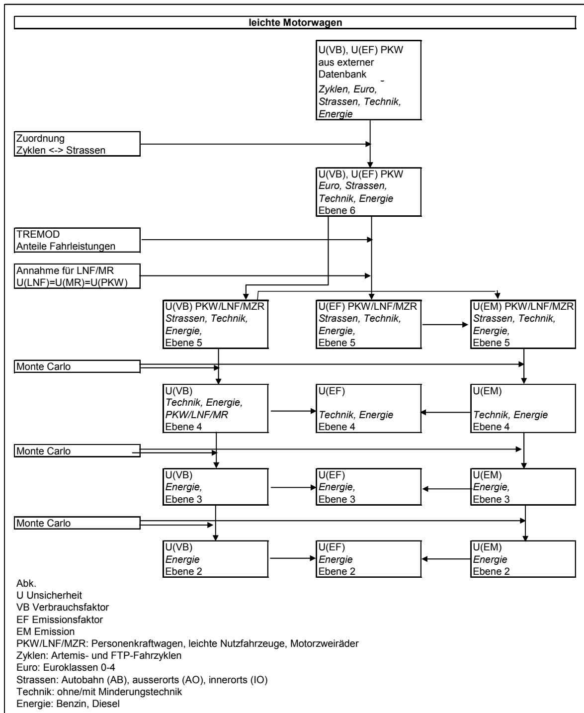
Abb. 5 Vorgehen zur Bestimmung der Unsicherheiten für leichte Motorwagen (PKW, LNF, MZR), ausgehend von Messdaten (INFRAS 2009a).
