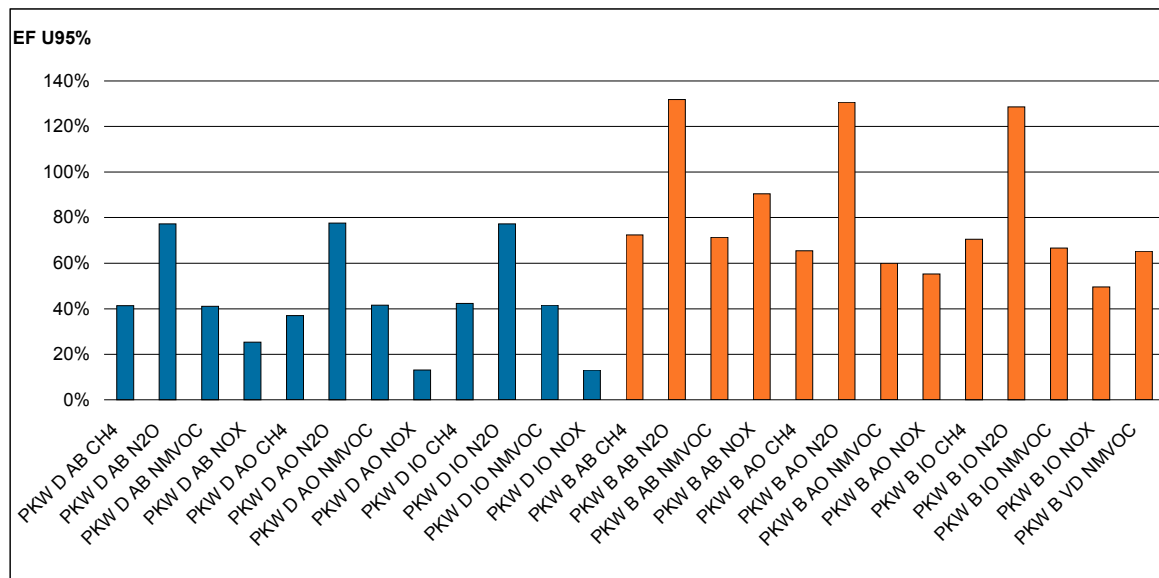
Abb. 10 Unsicherheiten Emissionsfaktoren PKW mit Minderungstechnik je Straßenkategorie und Schadstoffe (Ebene 5). Blau: Diesel. Orange: Benzin. Quelle: (INFRAS 2009a)
