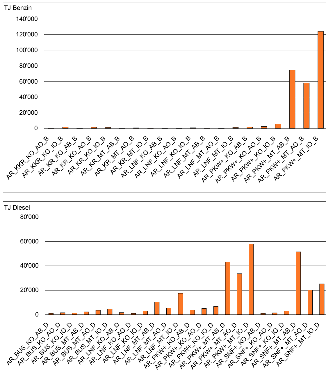
Abb. 7 Unsicherheiten der Aktivitätsraten Straßenverkehr 2007 (absolut in TJ). Oben Benzin, unten Diesel. Kodierung x-Achse: (Aktivitätsrate)_(Fz.kat.)_(Minderungstechnik)_(Straßenkategorie)_(Kraftstoff).
