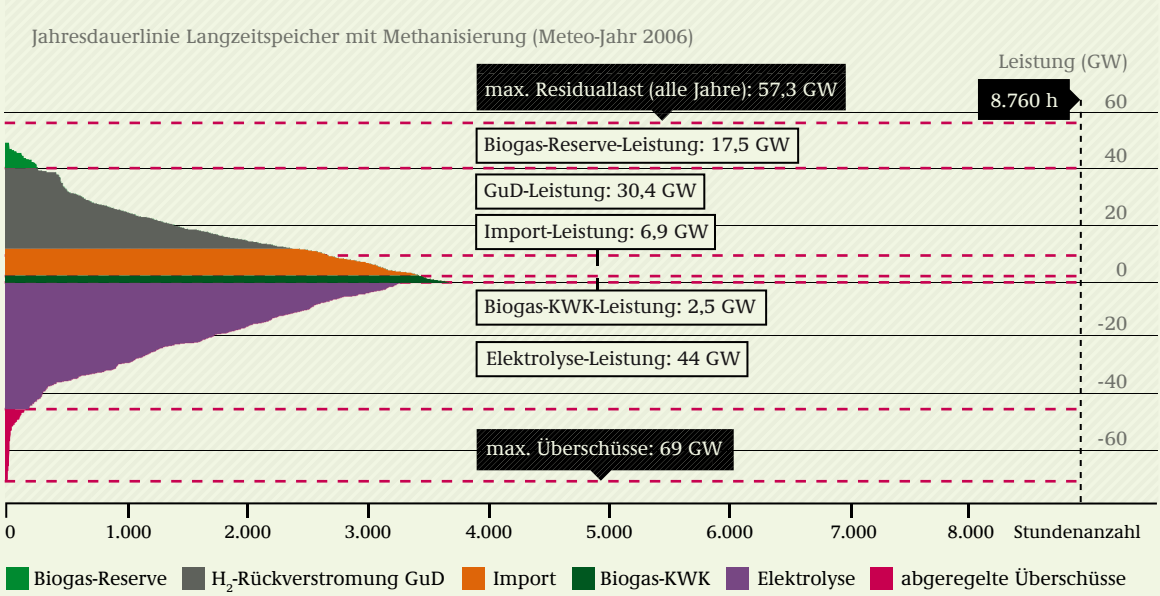
ABB 10-14 JAHRESDAUERLINIE VON ELEKTROLYSE/METHANISIERUNG, METHAN-RÜCKVERSTROMUNG, BIOGASVERSTROMUNG UND IMPORTEN IM JAHR 2050, FÜR
