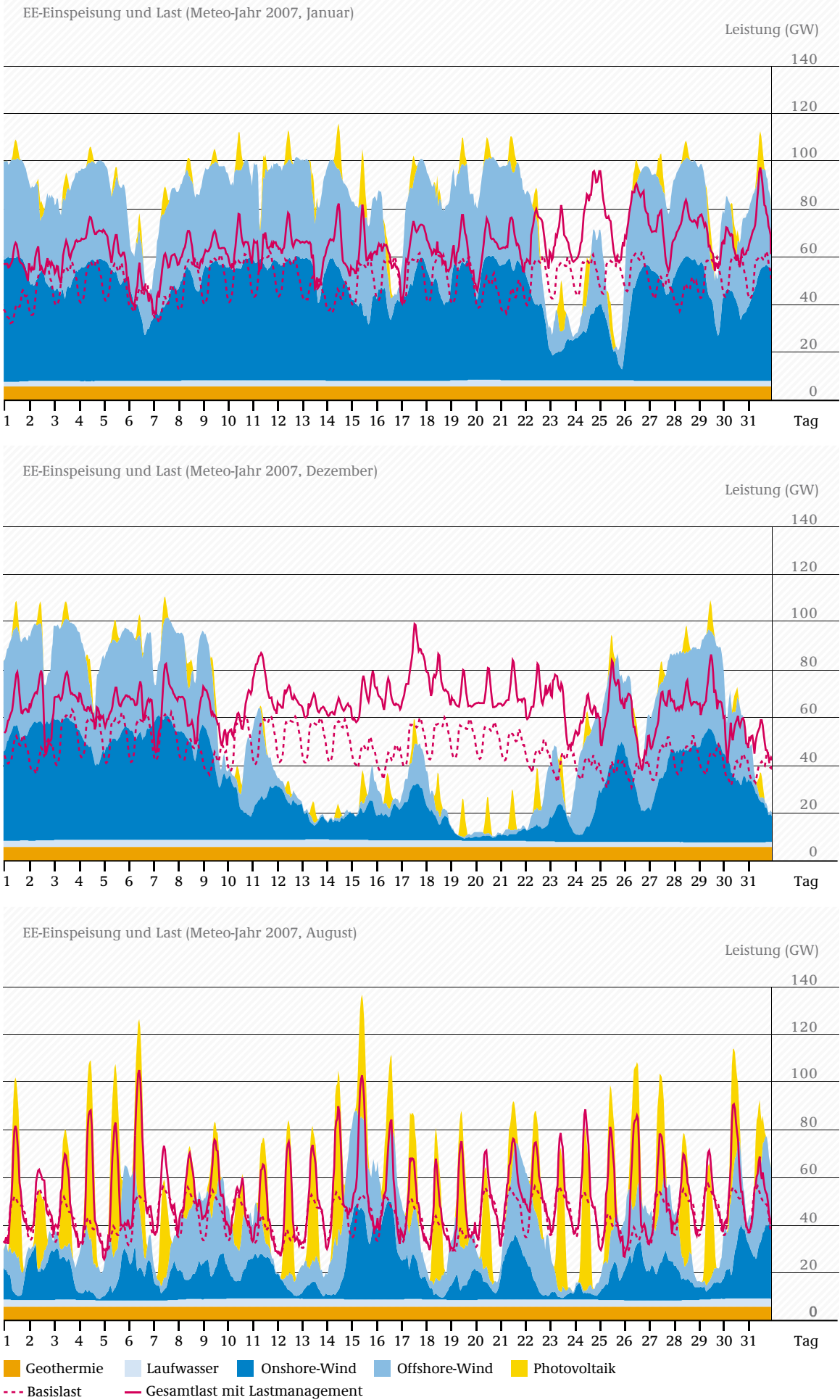
ABB 7-10 BEISPIELE FÜR DIE EINSPEISUNG DER ERNEUERBAREN ENERGIEN IM JAHR 2050, BASIEREND AUF DEM WETTER JAHR 2007 – JANUAR (OBEN), DEZEMBER (MITTE), AUGUST (UNTEN)
