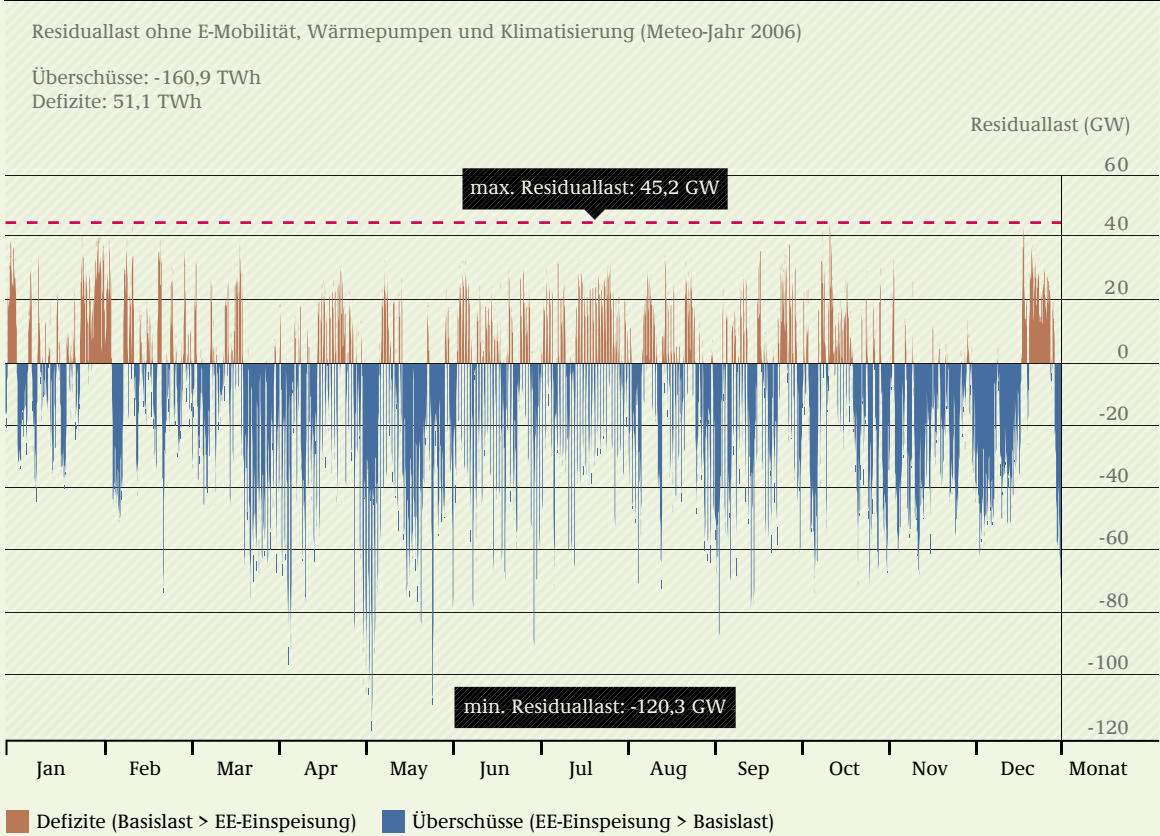
ABB 10-9 RESIDUALE BASISLAST IM JAHRE 2050, FÜR DIE WETTER-JAHRE 2006-2009
