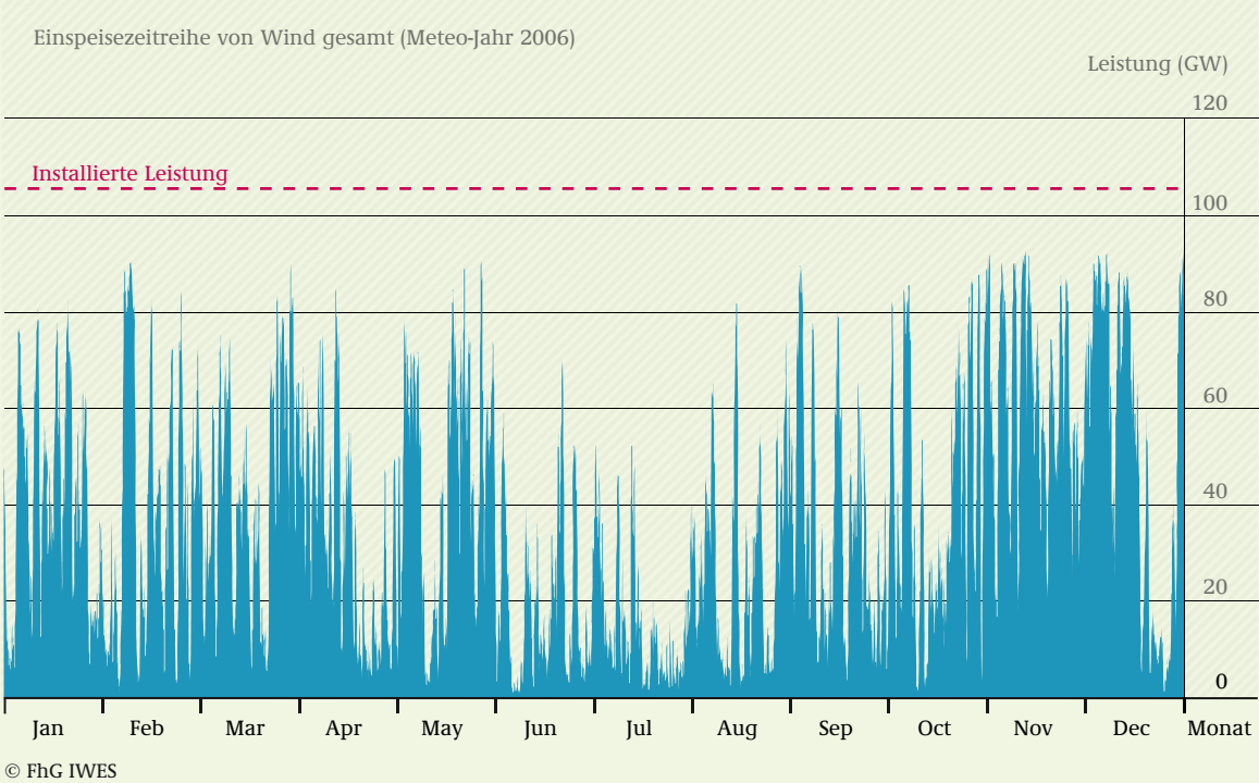
ABB 10-4 MITTLERE STÜNDLICHE EINSPEISUNG WIND GESAMT (ONSHORE UND OFFSHORE) IM JAHR 2050, FÜR ALLE WETTER-JAHRE 2006-2009
