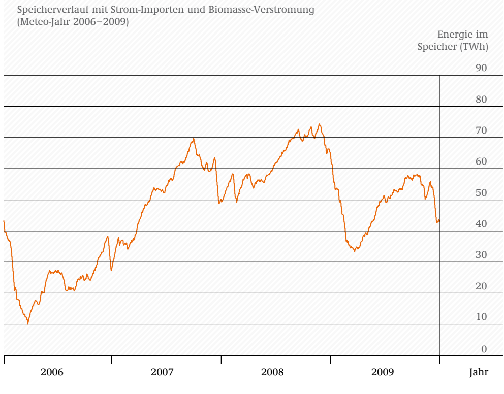
ABB 7-23 FÜLLSTAND DES METHANSPEICHERS FÜR DEN GESAMTEN BETRACHTUNGSZEITRAUM 2006-2009
