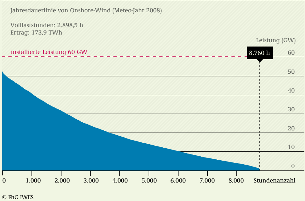
ABB 10-7 JAHRESDAUERLINIE DER WINDENERGIE (ONSHORE OFFSHORE, GESAMT) IM JAHR 2050, FÜR DAS WETTER-JAHR 2008
