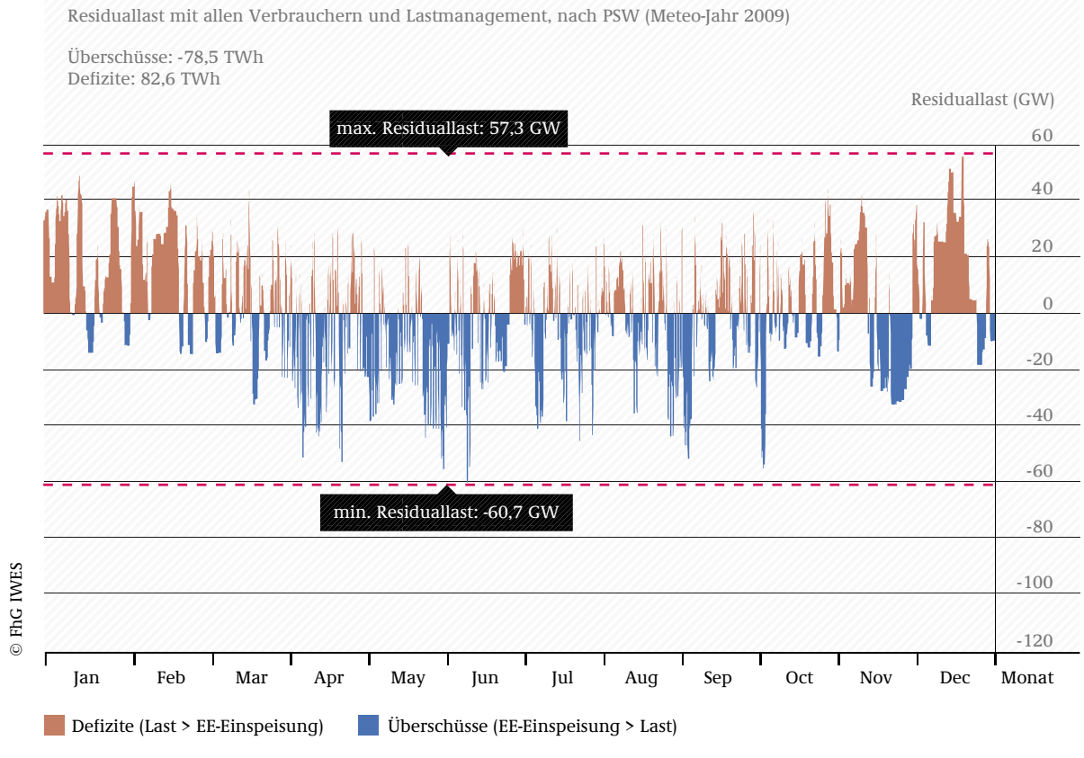
ABB 7-13 RESIDUALE GESAMTLAST (UNTER BERÜCKSICHTIGUNG VON LASTMANAGEMENT UND PUMPSPEICHERN) FÜR DAS JAHR 2050, BASIEREND AUF DEM WETTER-JAHR 2009
