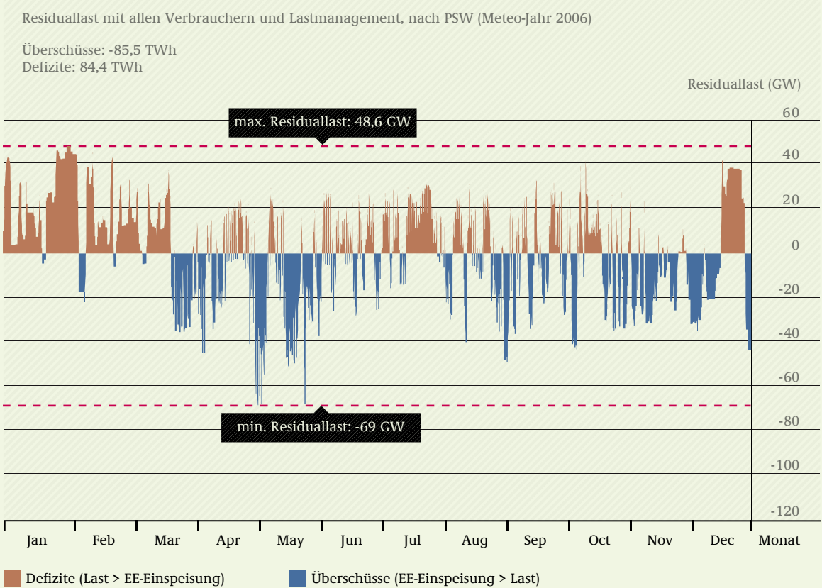
ABB 10-11 RESIDUALE GESAMTLAST UNTER BERÜCKSICHTIGUNG VON LASTMANAGEMENT UND PUMPSPEICHERN IM JAHR 2050, FÜR DIE WETTER-JAHRE 2006-
