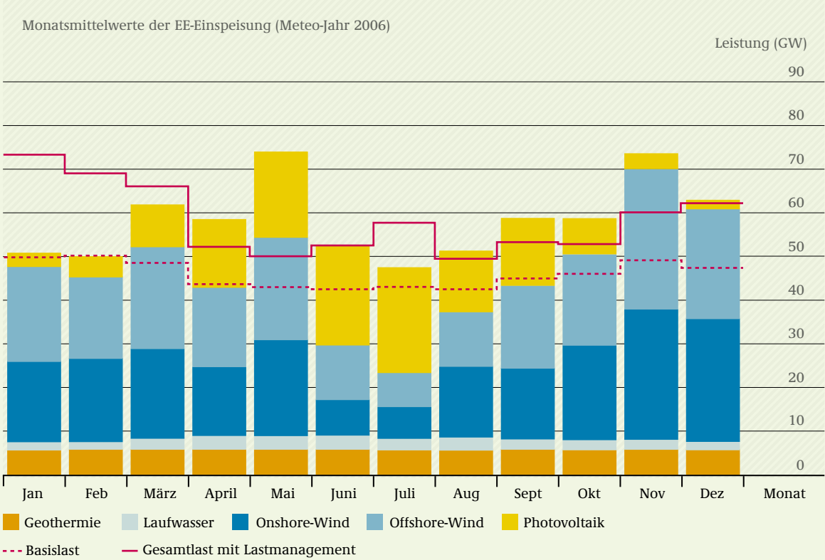
ABB 10-5 MONATLICHE EINSPEISUNG ALLER ERNEUERBAREN ENERGIEN, INKL. DARSTELLUNG DER LAST VOR UND NACH DEM LASTMANAGEMENT IM JAHR 2050,
