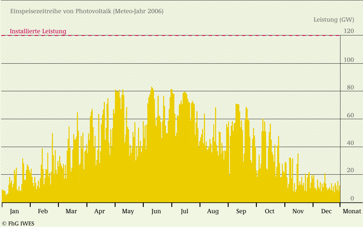
ABB 10-1 MITTLERE STÜNDLICHE EINSPEISUNG PHOTOVOLTAIK IM JAHR 2050, FÜR ALLE WETTER-JAHRE 2006-2009
