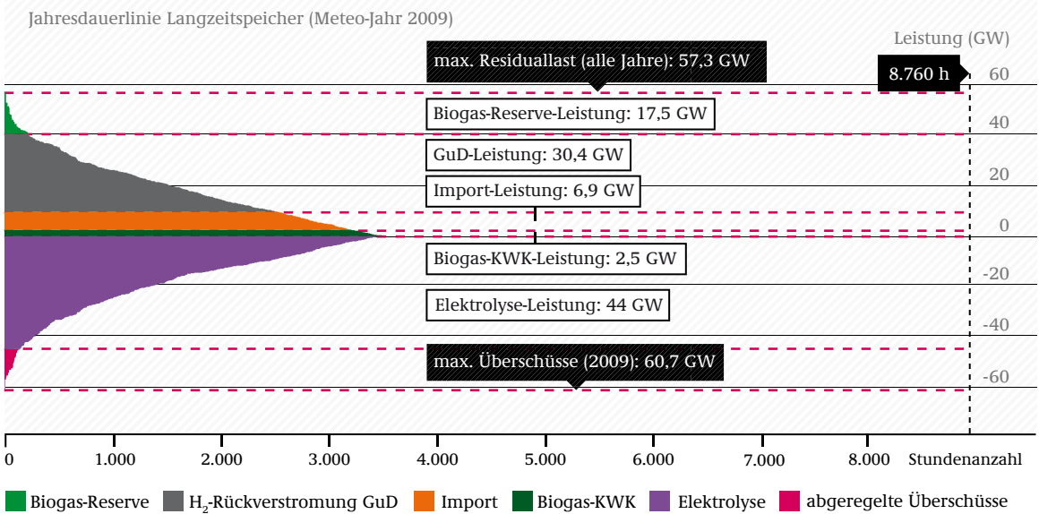
ABB 7-21 JAHRESDAUERLINIE VON ELEKTROLYSE, WASSERSTOFFRÜCKVERSTROMUNG, BIOGASVERSTROMUNG UND IMPORTEN IM JAHR 2050, BASIEREND AUF DEM WETTER-JAHR 2009 209
