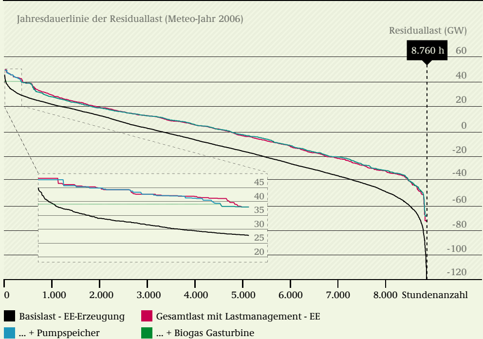
ABB 10-12 JAHRESDAUERLINIE VON REDIDUALER BASISLAST, RESIDUALER GESAMTLAST UND RESIDUALER GESAMTLAST MIT PUMPSPEICHERN
