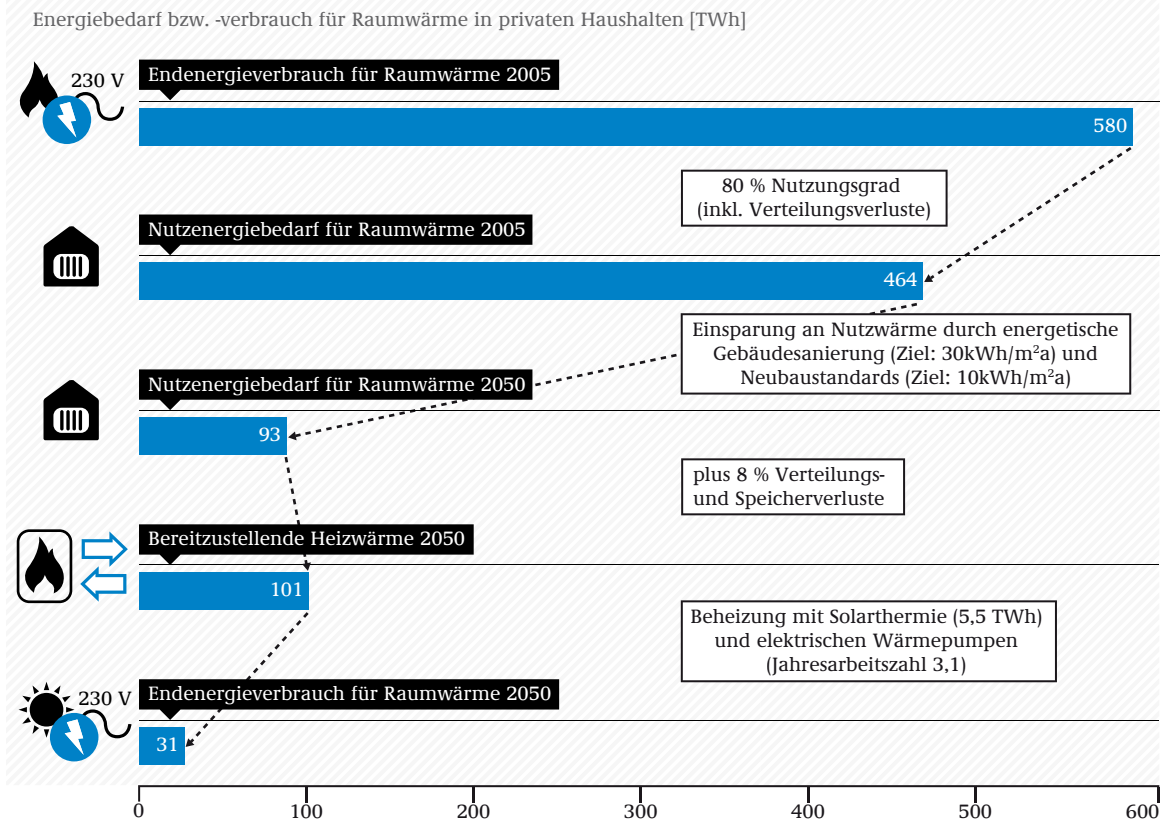
ABB 3-2 VORGEHENSWEISE BEI DER BERECHNUNG DES ENDENERGIEBEDARFS DER HAUSHALTE FÜR RAUMWÄRME IM JAHR 2050
