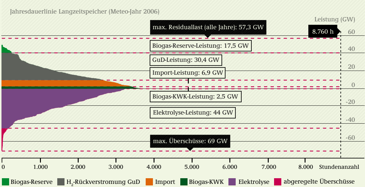
ABB 10-13 JAHRESDAUERLINIE VON ELEKTROLYSE, WASSERSTOFFRÜCKVERSTROMUNG, BIOGASVERSTROMUNG UND IMPORTEN IM JAHR 2050, FÜR DIE WETTER-
