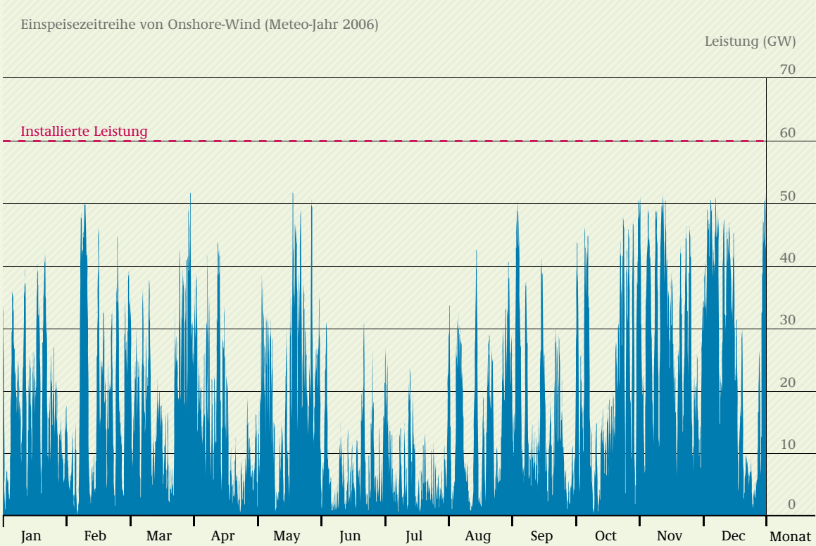
ABB 10-2 MITTLERE STÜNDLICHE EINSPEISUNG ONSHORE-WIND IM JAHR 2050, FÜR ALLE WETTER-JAHRE 2006-2009
