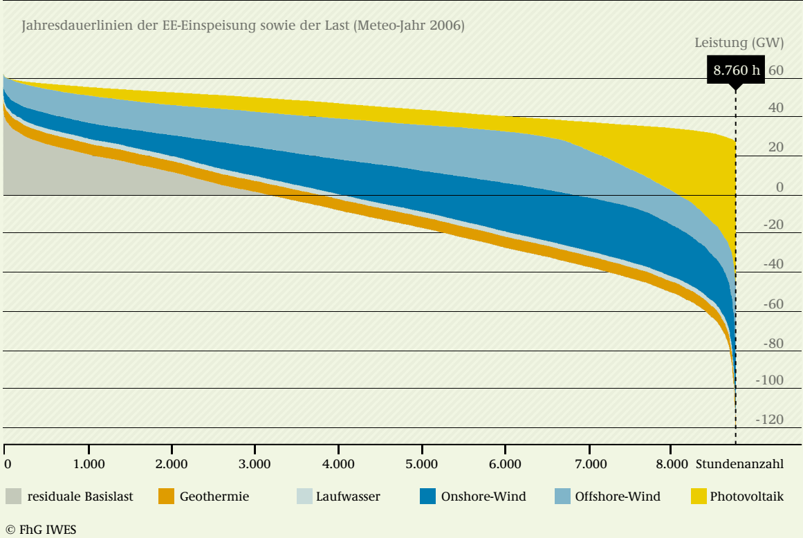
ABB 10-6 JAHRESDAUERLINIEN DER EINSPEISUNG ERNEUERBARER ENERGIEN IM JAHR 2050, FÜR ALLE WETTER-JAHRE 2006-2009
