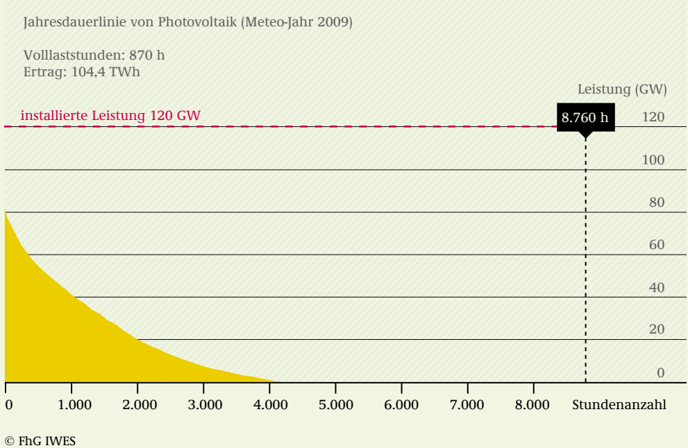
ABB 10-8 JAHRESDAUERLINIE DER EE - PHOTOVOLTAIK, WASSERKRAFT, GEOTHERMIE IM JAHR 2050, FÜR DAS WETTER-JAHR 2009
