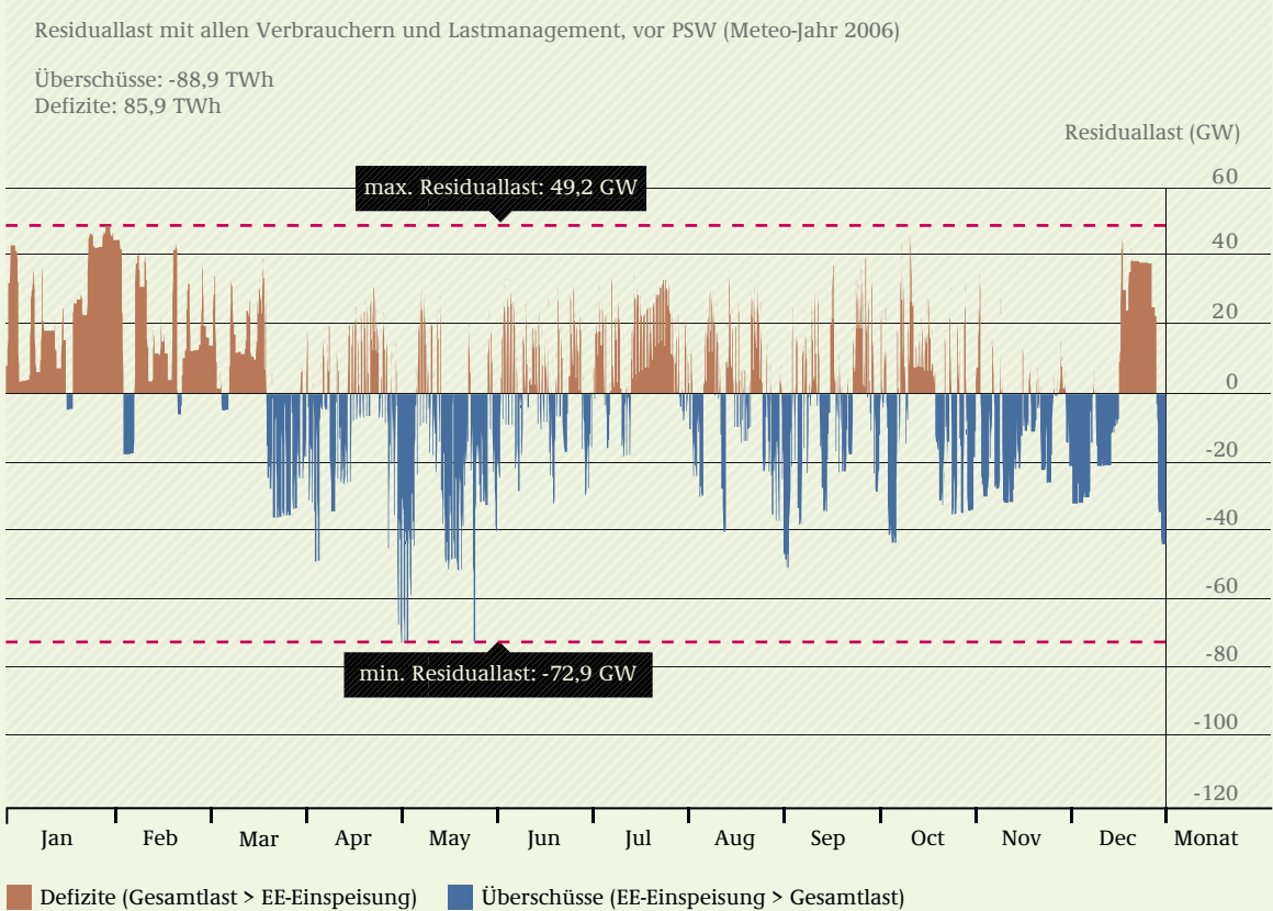
ABB 10-10 RESIDUALE GESAMTLAST UNTER BERÜCKSICHTIGUNG VON LASTMANAGEMENT, OHNE PUMPSPEICHER, IM JAHR 2050, FÜR DIE WETTER-JAHRE 2006-
