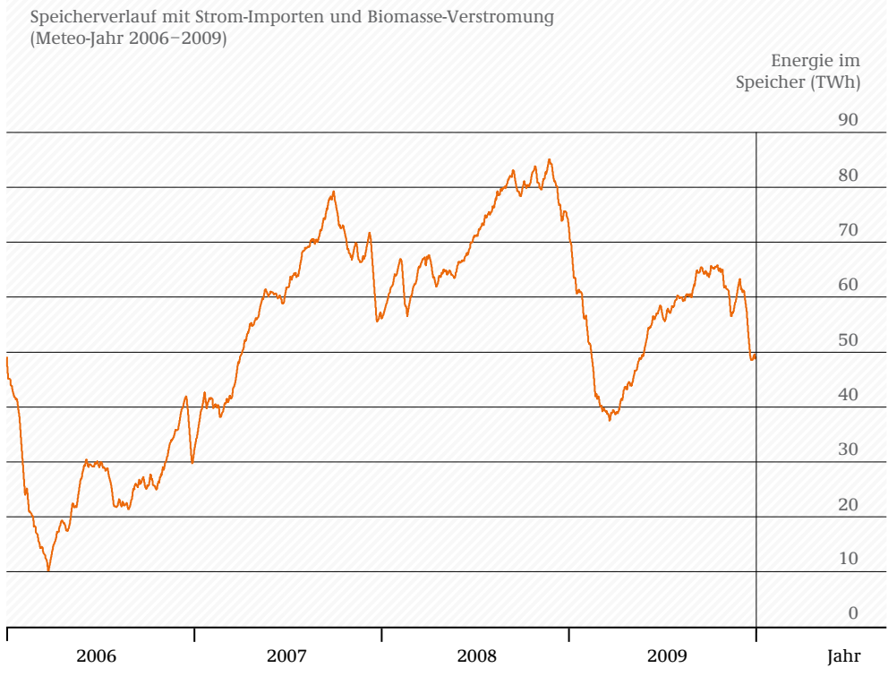
ABB 7-20 FÜLLSTAND DES WASSERSTOFFSPEICHERS FÜR DEN GESAMTEN BETRACHTUNGSZEITRAUM 2006-2009
