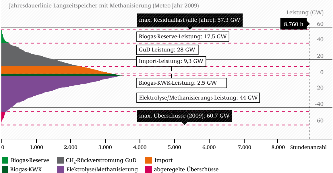
ABB 7-24 JAHRESDAUERLINIE VON ELEKTROLYSE/METHANISIERUNG, METHAN-RÜCKVERSTROMUNG, BIOGASVERSTROMUNG UND IMPORTEN IM JAHR 2050, BASIEREND AUF DEM WETTER-JAHR 2009 210
