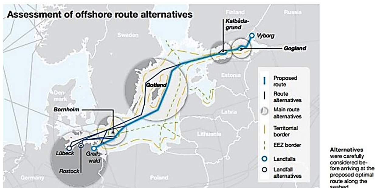
Рисунок 1: Трасса трубопровода «Nord Stream»
