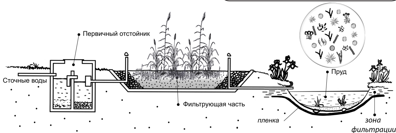
Рис. 22. Почвенный фильтр с прудом.
