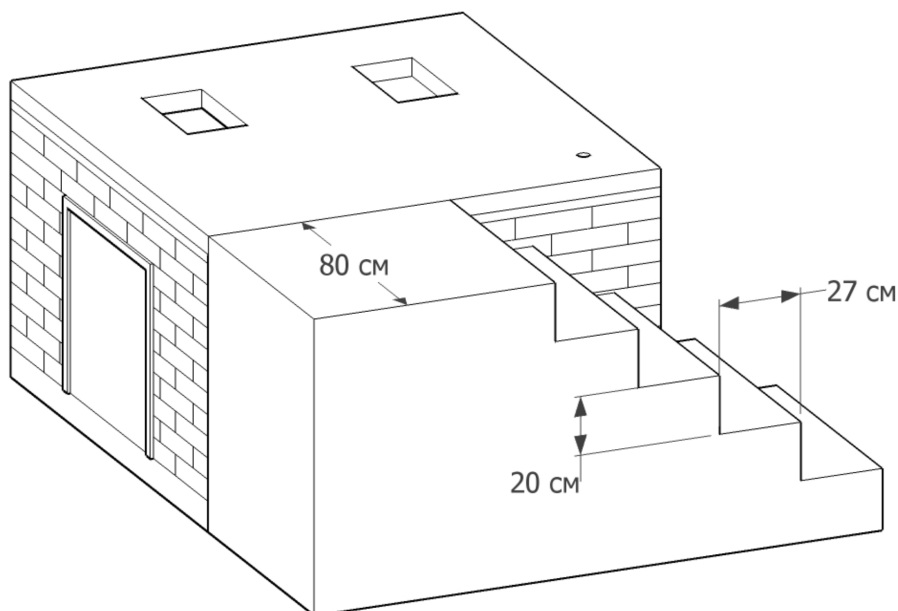
рис. 9. Расположение лестницы.
