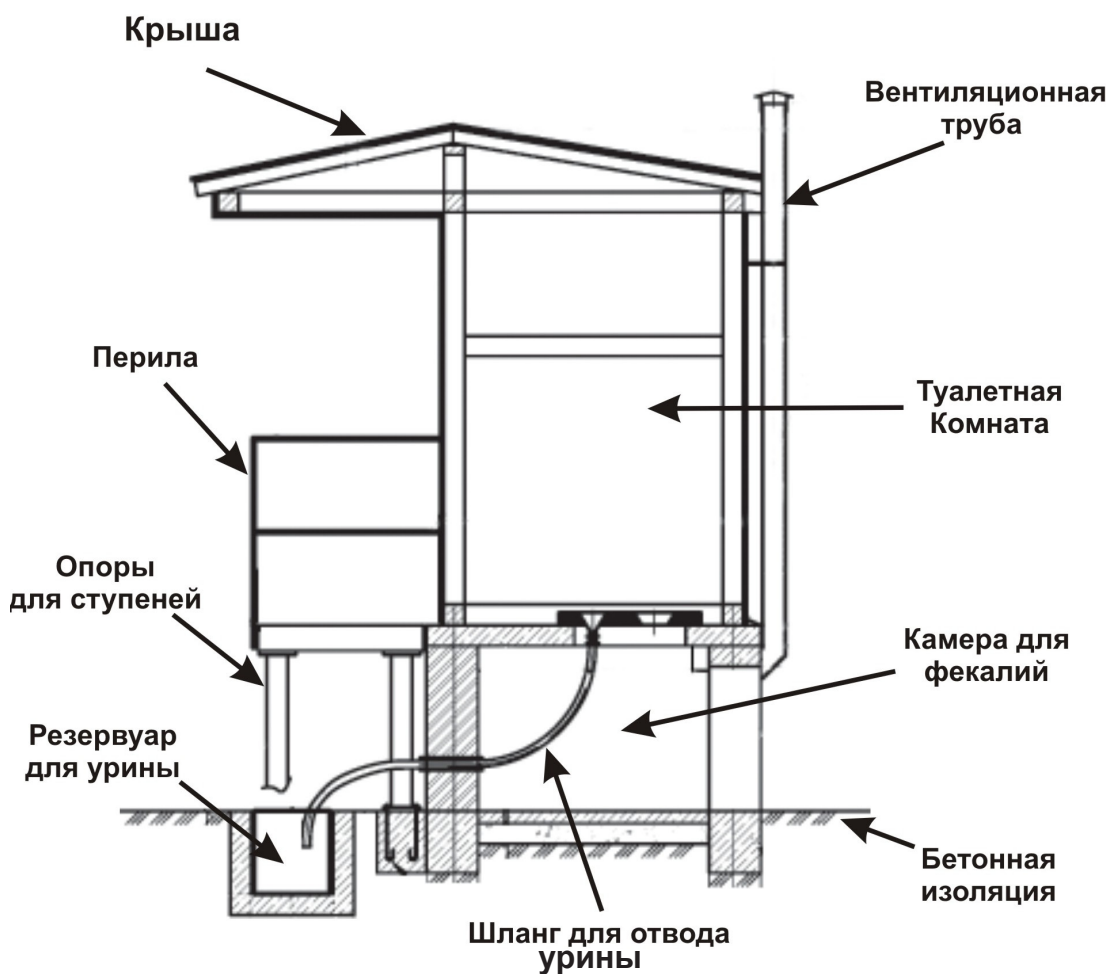
рис. 2. Схема туалета «Экосан».
