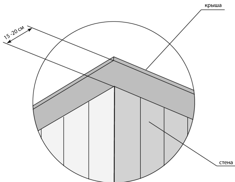
рис. 8. Отступ кровли над стенами.
