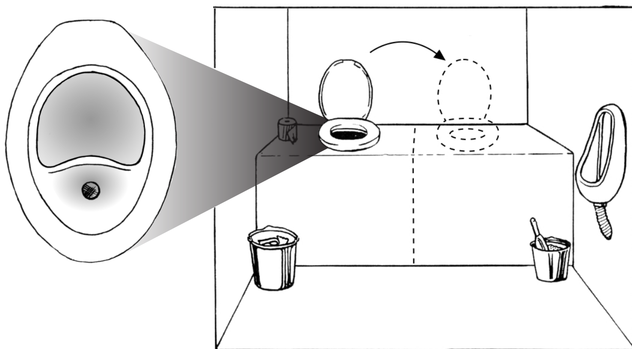
рис.14. Внутреннее устройство туалета «экосан».
