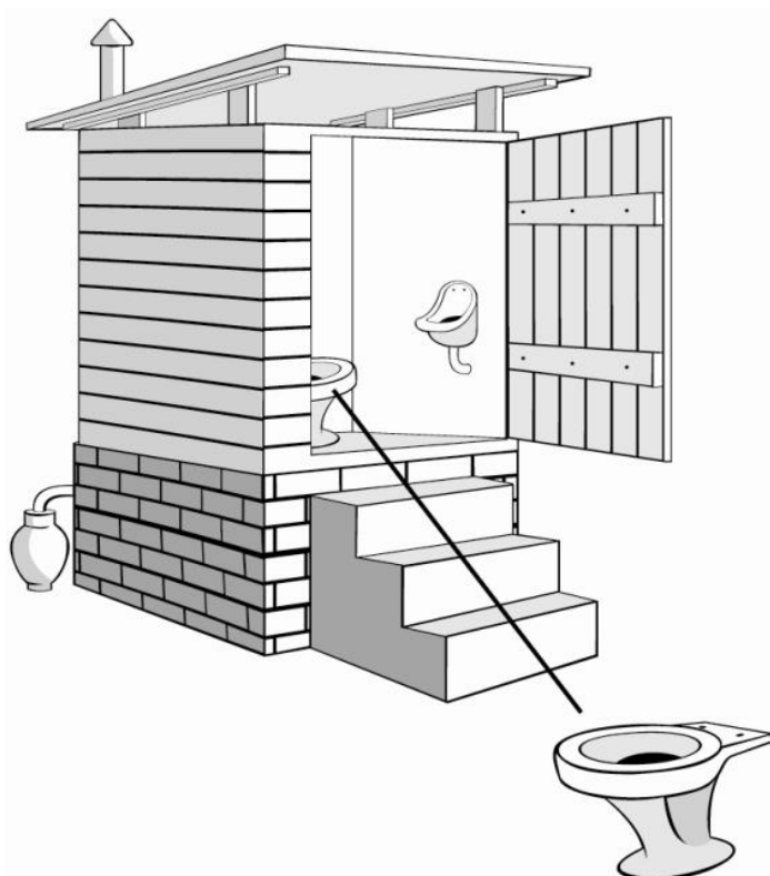
рис. 1. Внешний вид сухого туалета.
