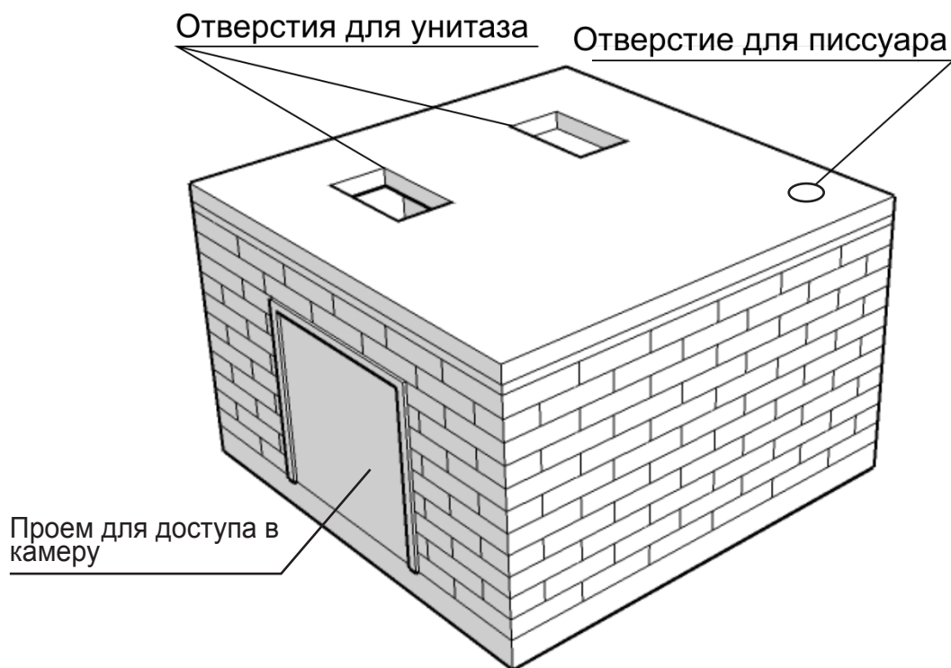
рис. 7. Устройство надкамерного перекрытия туалета.
