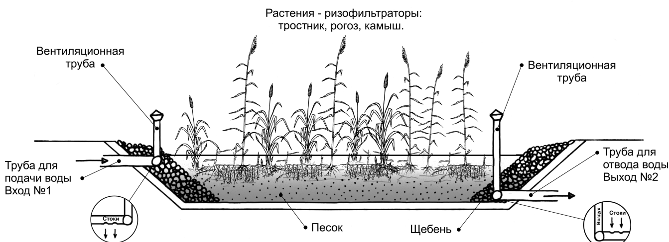
Рис. 17. Устройство фильтрующей части.
