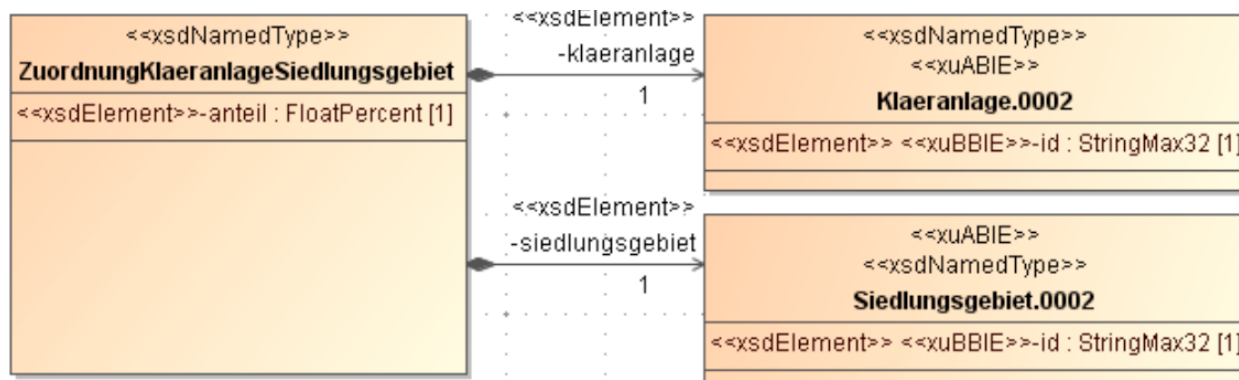
Abbildung 13: Nutzung spezifischer XUBetrieb-Komponenten durch Komposition
