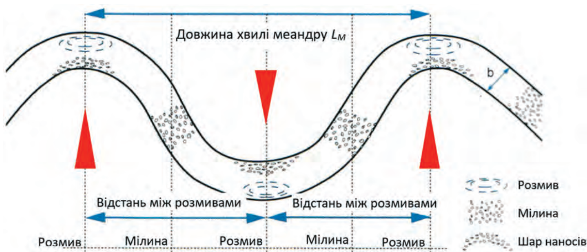
Рисунок 7: Можливе розташування бун у водотоках, які у природному стані мали б незначну та правильну кривизну русла. Червоні трикутники позначають буни. (Джерело: Gebler 2005, змінено)
