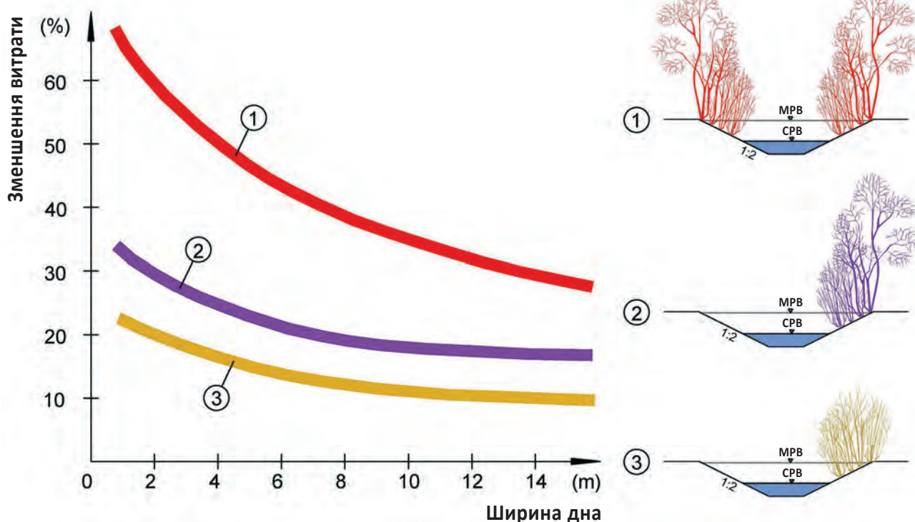
Рисунок 15: Зниження пропускної спроможності русла через прибережні дерева у профілі водотоку в залежності від цільової рослинності та ширини русла. (Джерело: за SCHICHTEL und STERN 2002, змінено Stowasserplan GmbH & Co. KG, із DWA 2020 b)
