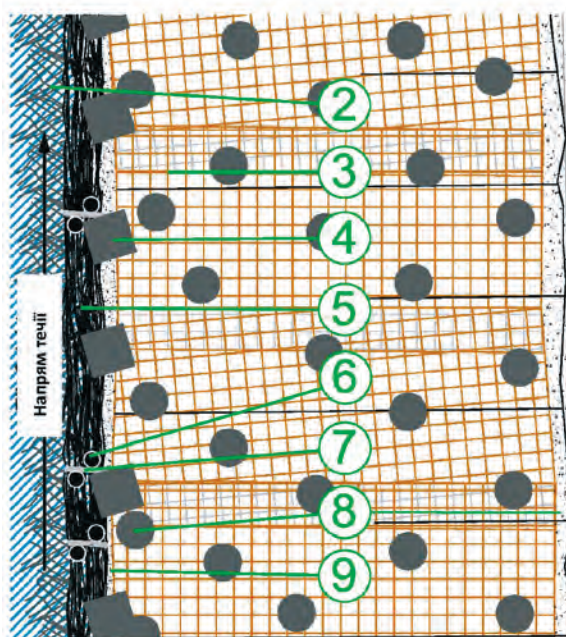
Рисунок 26: Типова технологічна карта «Жива фашина з підстилкою на схилі, садінням вільхи і живцями» (Рисунок: ©StowasserService)
