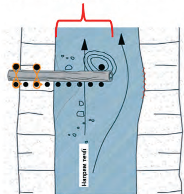
Рисунок 11: До поняття гідравлічно ефективної довжини. (Джерело: StowasserService GmbH & Co. KG 2015, від TLUG 2015, змінено)
