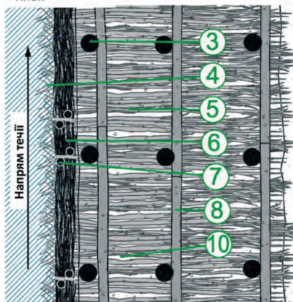
Рисунок 22: Типовий варіант технологічної карти «Вистилання хмизом із живою фашиною для укріплення основи схилу» (Рисунок: © StowasserService)
