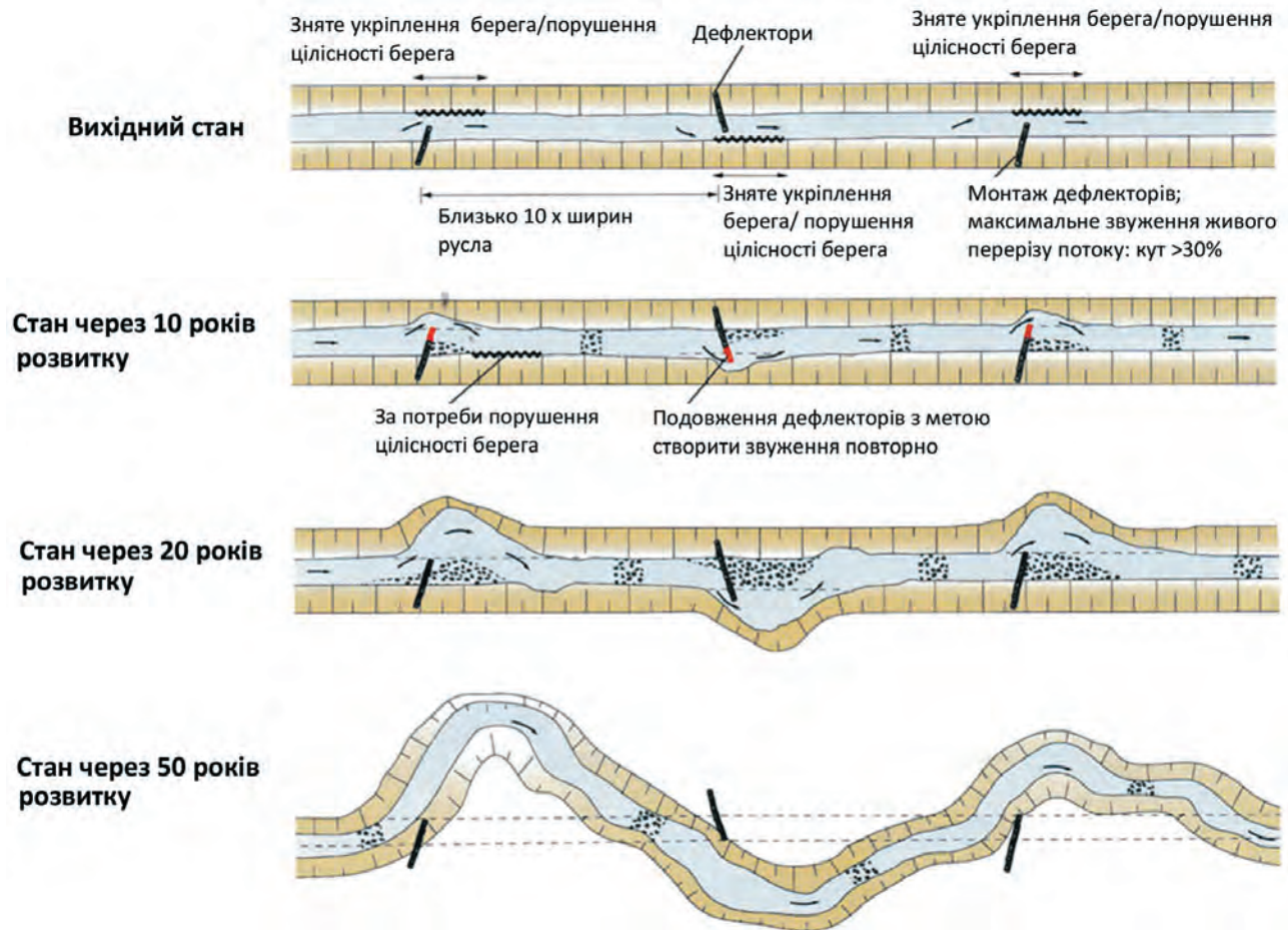
Рисунок 8: Часова послідовність можливих сценаріїв розвитку раніше спрямленого водотоку, розвиток якого ініційовано спорудами типу бун. (Джерело: Gebler 2005)
