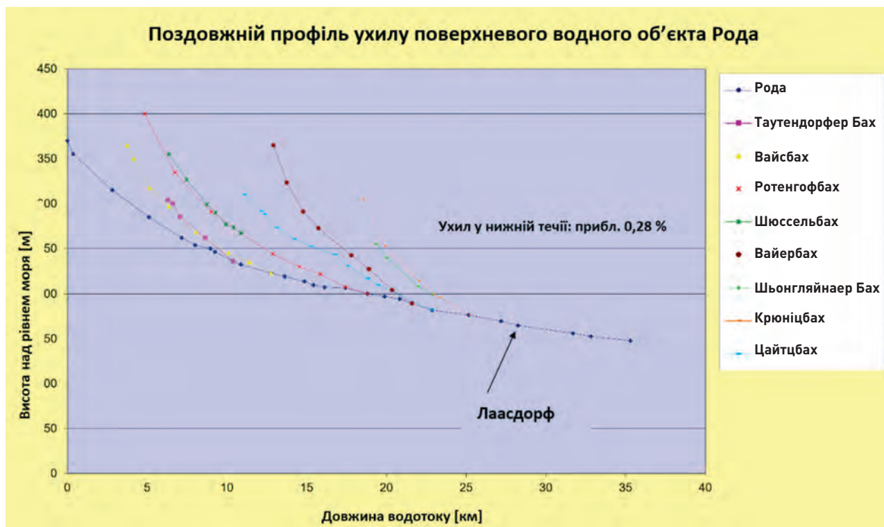
Рисунок 17: Поздовжній профіль ухилу Роди та її приток (поверхневий водний об'єкт Рода). (Джерело: власний рисунок М. Dittrich 2004)
