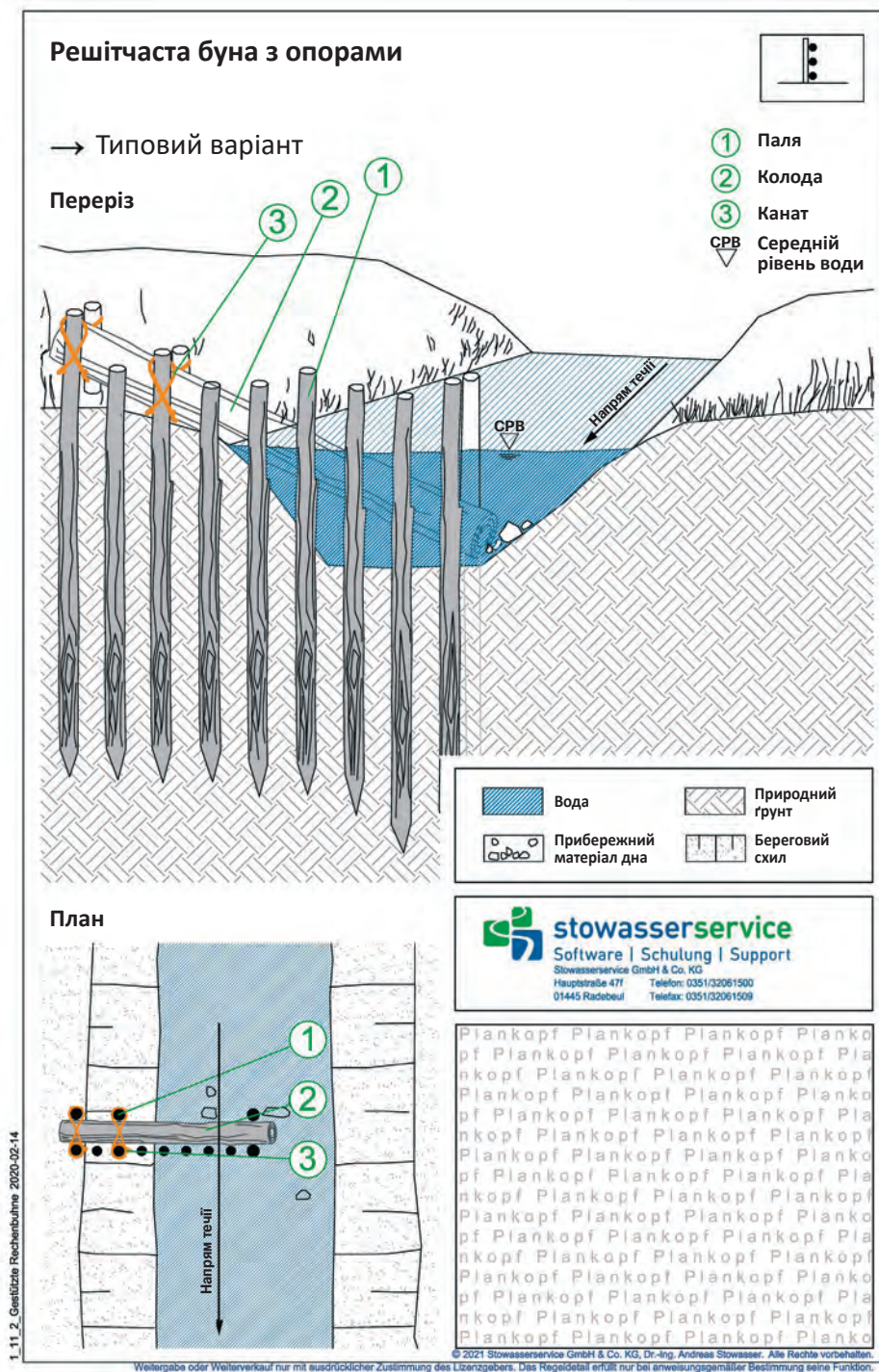
Рисунок 9: Типовий варіант технологічної карти (поперечний переріз і план) решітчастої буни з опорами, повністю виготовленої з небіологічних матеріалів. (Джерело: StowasserService GmbH & Co. KG 2015, від TLUG 2015)
