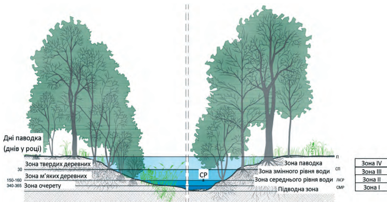
Рисунок 4: Поперечний розріз зонування берегів водотоку. (Джерело: за SMUL 2005, від TLUG 2018, змінено) (Скорочення праворуч: див.таблицю нижче – прим. пер.)
