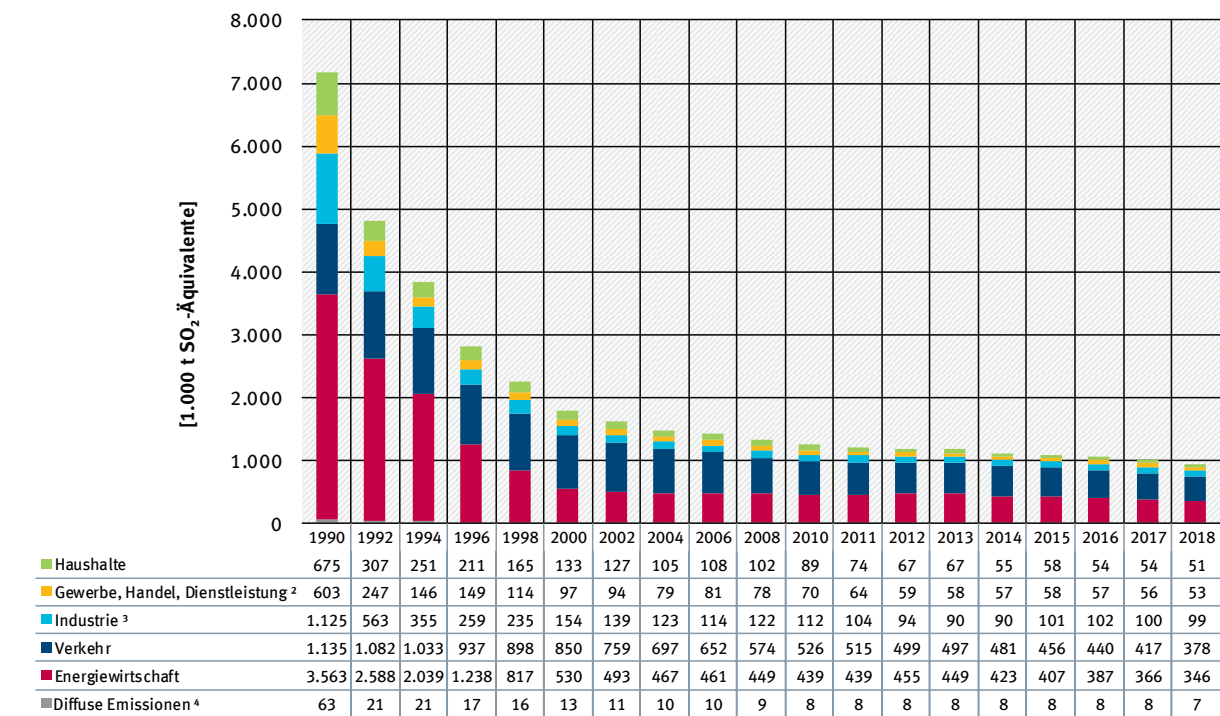
Abbildung 6: Entwicklung der energiebedingten Emissionen von Säurebildnern 1 nach Quellgruppen 1990-2018
