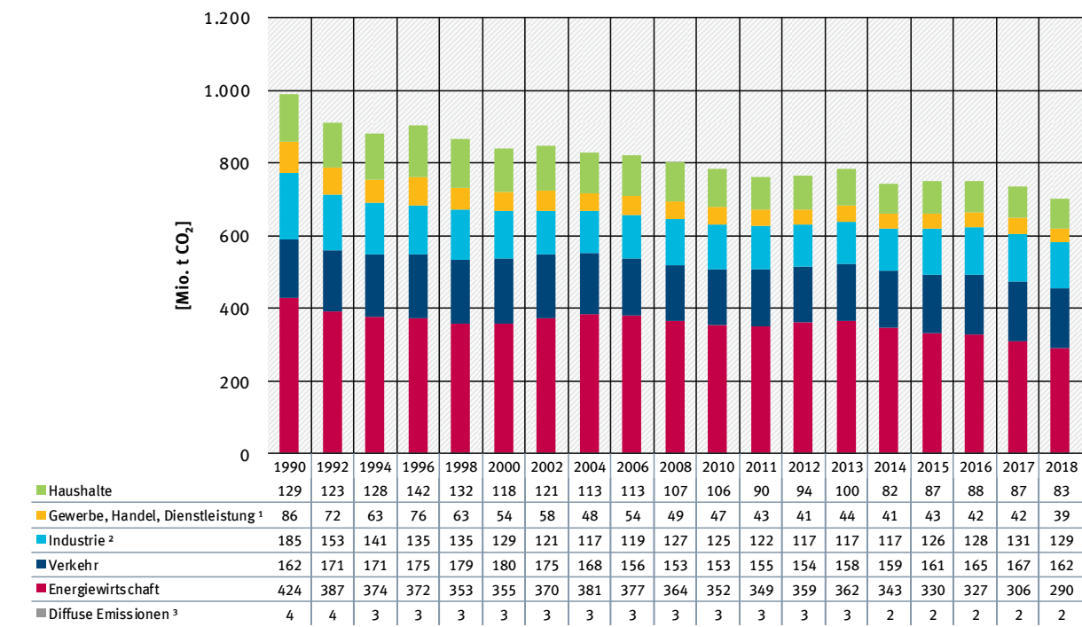
Abbildung 4: Entwicklung der energiebedingten CO 2 -Emissionen 1990-2018
