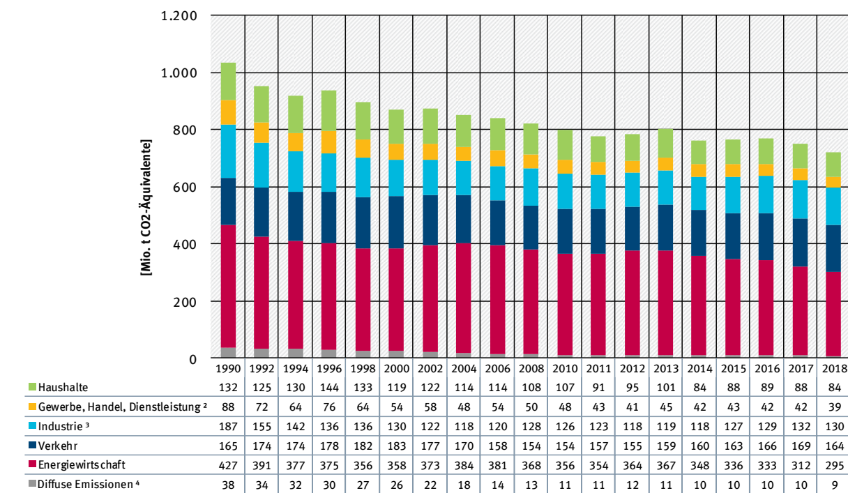
Abbildung 2: Entwicklung der energiebedingten THG-Emissionen 1 1990-2018
