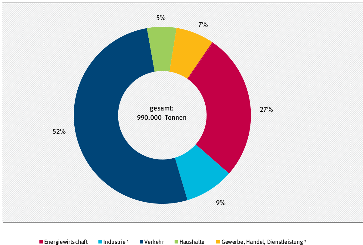
Abbildung 9: Anteile der Quellgruppen an den energiebedingten NO x -Emissionen im Jahr 2018
