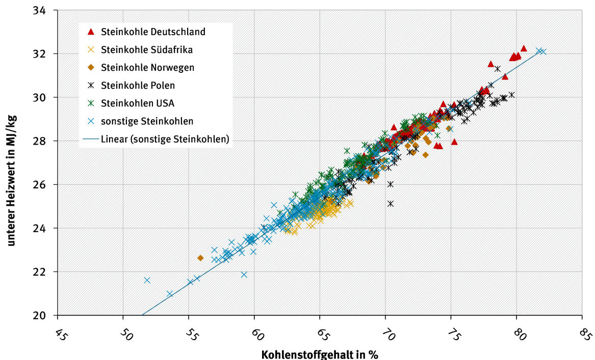
Abbildung 118: Verhältnis zwischen Kohlenstoffgehalten und Heizwerten für verschiedene Steinkohlenqualitäten
