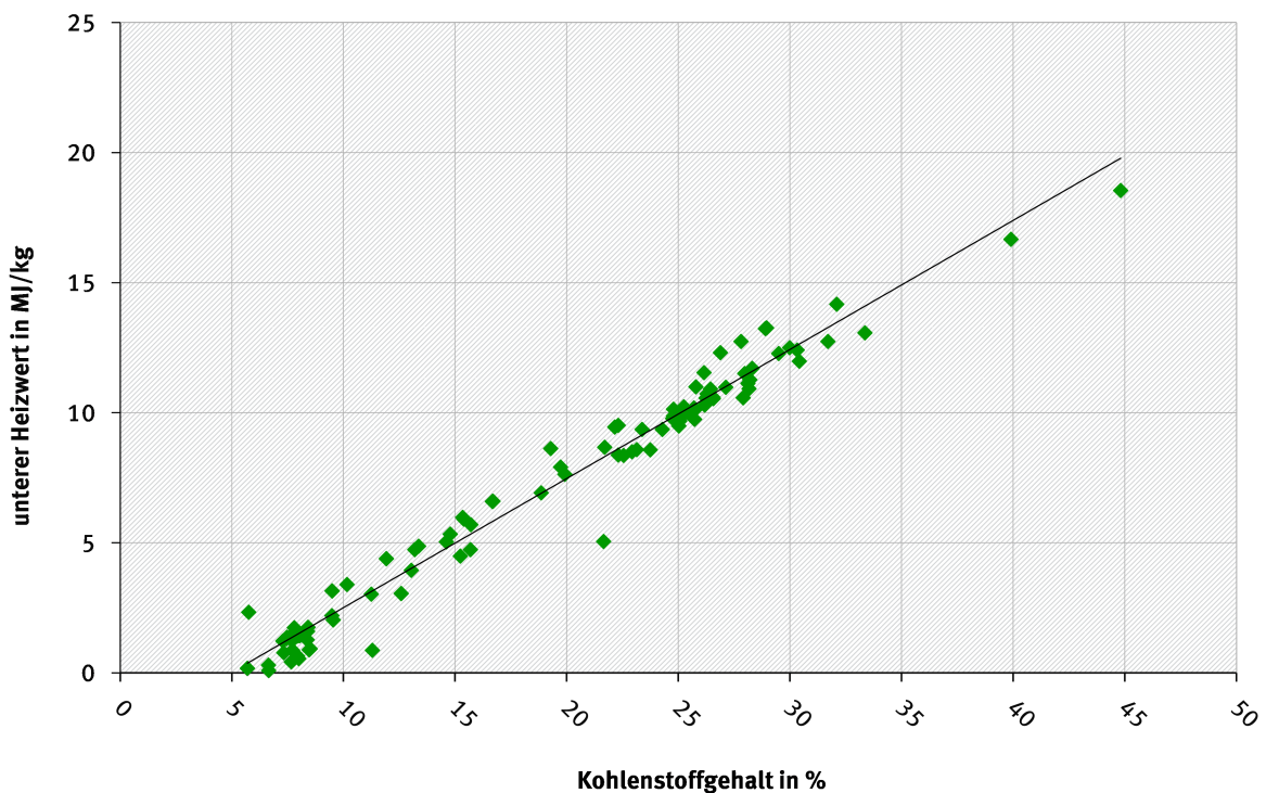
Abbildung 120: Verhältnis zwischen Kohlenstoffgehalten und Heizwerten für verschiedene Klärschlämme
