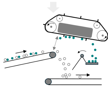
Magnetscheider (Eisenmetalle)
