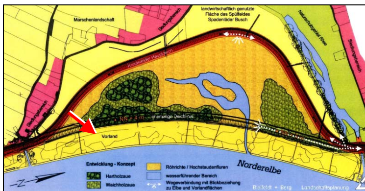
Zustand vor und nach der Deichrückverlegung: Entlang der Norderelbe die alte Deichtrasse mit Vorland; landeinwärts verschoben die neue realisierte Trasse mit dem erweiterten Deichvorland.
