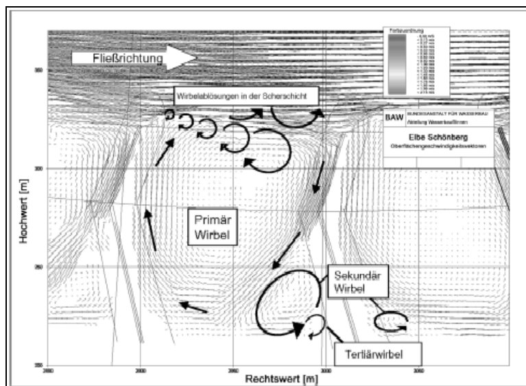
Typische Strömungsprofil und die wesentlichen Wirbelstrukturen bei einer nicht überströmten Knickbuhne.
