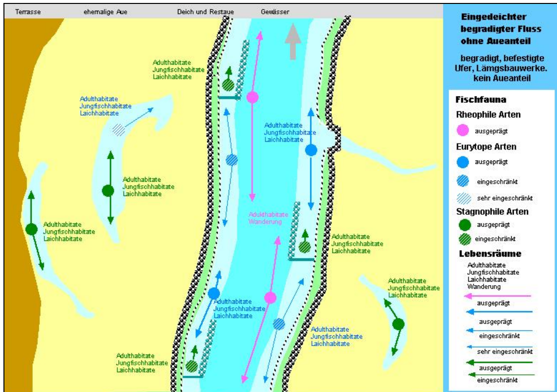
Abb. 16: Raumnutzung der Fischfauna – Modell 6: Eingedeichter, begradigter Fluss mit Längsbauwerken und ohne nennenswerten Aueanteil
