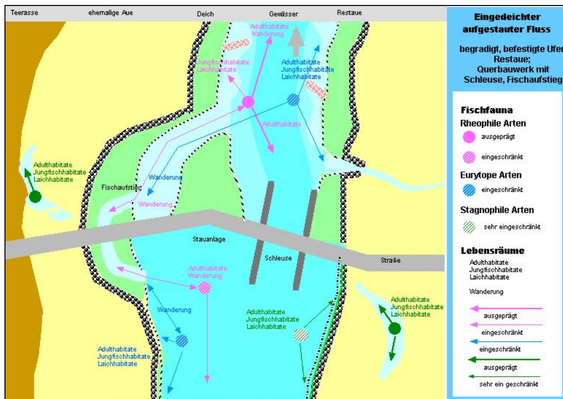
Abb. 17: Raumnutzung der Fischfauna – Modell 7: Eingedeichter, aufgestauter Fluss
