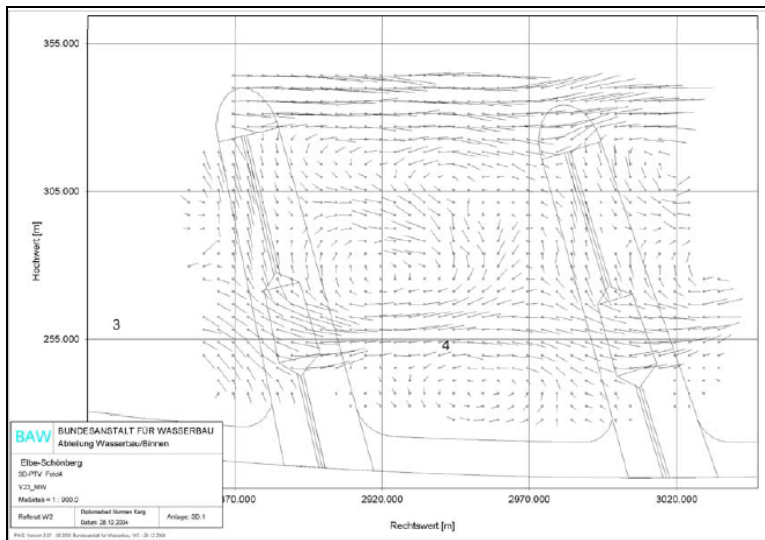
Strömungsbild aus einem Simulationsversuch mit einer Absenkbühne in Form eines breiten, V-förmigen Durchrisses.
