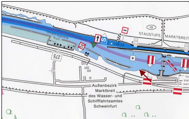
Planausschnitt aus Übersichtsplan zur Bundeswasserstraße Main.
