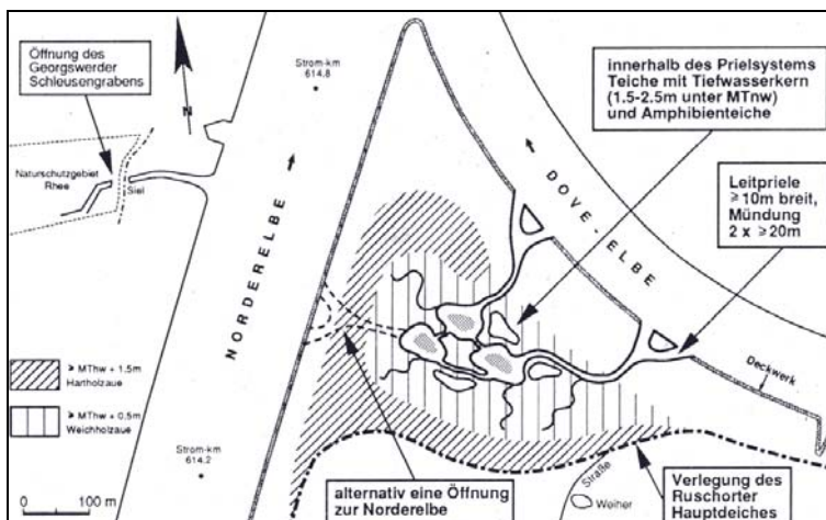
Ursprüngliche Planung der Deichrückverlegung mit mehreren Anbindungen zum Hauptstrom.
