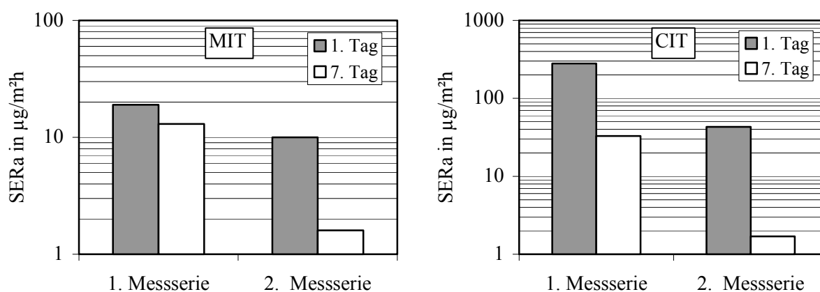
Abbildung 12: Vergleichsmessung für MIT und CIT aus Farbe 8 auf Glas, bei der 1. Messserie wurde die Farbe direkt und bei der 2. Messserie 283 Tage nach Erstöffnung aufgetragen.
