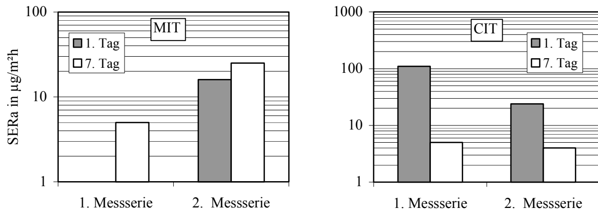
Abbildung 13: Vergleichsmessung für MIT und CIT aus Farbe 9 auf Glas, bei der 1. Messserie wurde die Farbe direkt und bei der 2. Messserie 198 Tage nach Erstöffnung aufgetragen.
