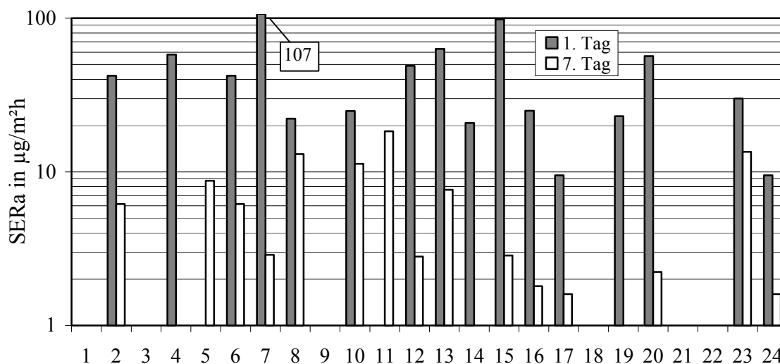
Abbildung 4. Flächenspezifische MIT-Emissionsraten (gemessen mit der FLEC) ein und sieben Tage nach Auftrag. MIT liegt für die Farben 1, 3, 9, 18, 21, 22 grundsätzlich, für die Farben 5 und 11 nach einem Tag und für die Farbe 14 nach 7 Tagen unter der BG; für die Farben 4 und 19 liegt kein 7-Tagewert vor.
