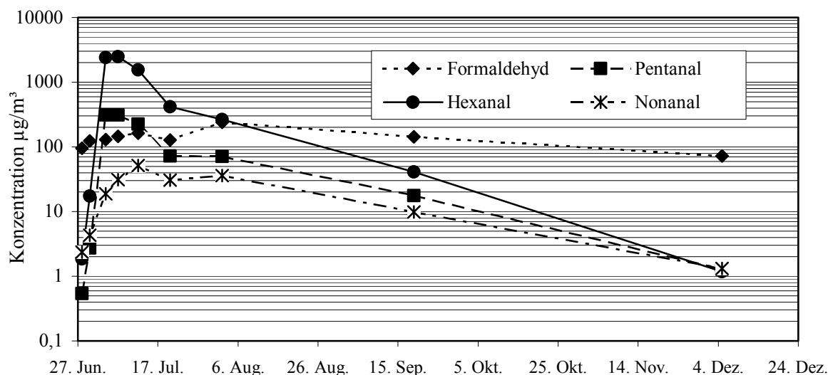
Abbildung 22: Zeitlicher Verlauf der Konzentrationen ausgewählter Aldehyde nach Anstrich mit Farbe 21.
