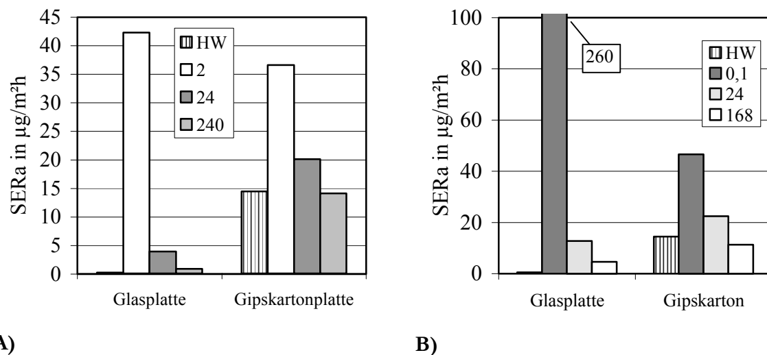
Abbildung 19: Vergleich der Formaldehydmission aus Farben nach Auftrag auf Glasplatte oder Gipskarton (Angaben jeweils in Stunden). A) Farbe 8 im "Weißen Elefanten". B) Farbe 13 in der FLEC. (HW = Hintergrundwert)
