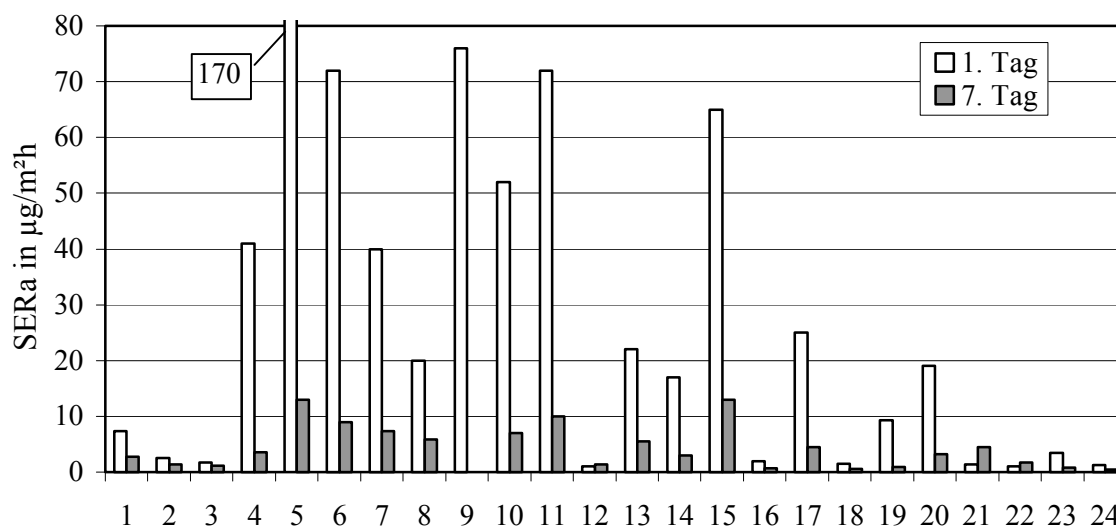
Abbildung 16: Formaldehyd- \text{SER}_a ( \mu\text{g}/\text{m}^2\text{h} ) der Farben auf Glas nach 1 Tag und 7 Tagen, gemessen mit der FLEC. (Für Farbe 9 liegt kein 7-Tagewert vor)
