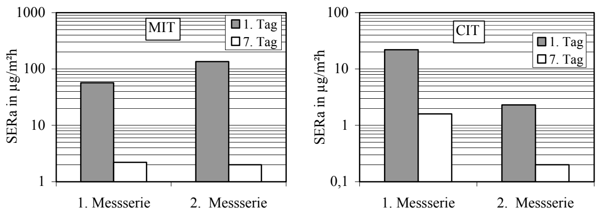
Abbildung 15: Vergleichsmessung für MIT und CIT aus Farbe 20 auf Glas, bei der 1. Messserie wurde die Farbe direkt und bei der 2. Messserie 98 Tage nach Erstöffnung aufgetragen.
