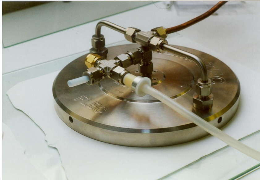
Abbildung 2. Emissionsmesszelle, FLEC.
