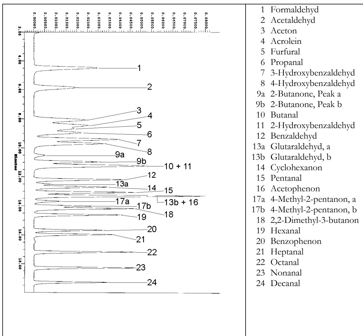
Abbildung A-1: Chromatogramm einer Standardmischung aller mit der gewählten Methode quantifizierbarer Aldehyde und Ketone. Die Hydrazone von 2-Butanon, Glutaraldehyd und 4-Methyl-2-pentanon splitten in zwei Peaks a und b auf.
