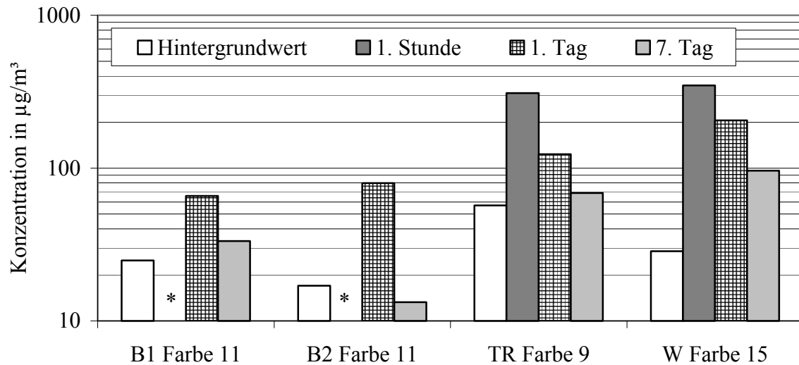
Abbildung 18: Formaldehyd-Konzentrationen in zwei Büroräumen (B1, B2), einem Testraum (TR) und in einer Wohnung (W) vor während und nach dem Streichen. *: nicht bestimmt
