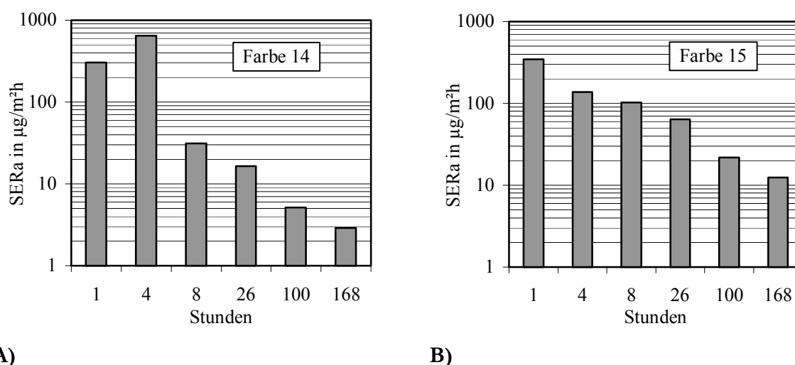
Abbildung 17: Unterschiedliches Abklingverhalten von Formaldehyd bei den Farben 14 (A) und 15 (B). Farbe 14 zeigt einen hohen Anfangswert gefolgt von einem schnellen Absinken, wohingegen Farbe 15 über einen längeren Zeitraum auf höherem Niveau emittiert.
