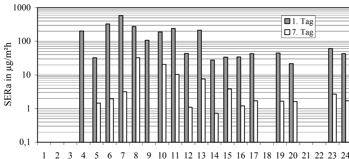
Abbildung 5. Flächenspezifische CIT-Emissionsraten (gemessen mit der FLEC) ein und sieben Tage nach Auftrag. Für die Farben 1, 2, 3, 18, 21 und 22 ist grundsätzlich kein CIT nachweisbar, für die Farben 4 und 9 liegen keine 7-Tagewerte vor.
