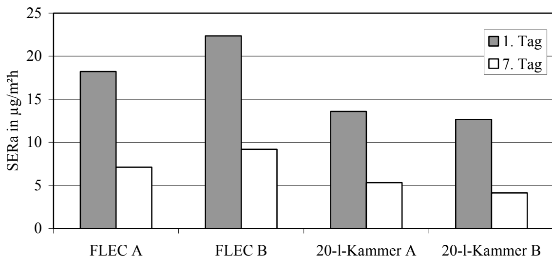
Abbildung A-2: Formaldehyd Emissionsraten in µg/m 2 h. Vergleich der verschiedenen Kammertypen und Reproduzierbarkeit der Messungen mit Farbe 4 (300 Tage nach Gebindeöffnung).
