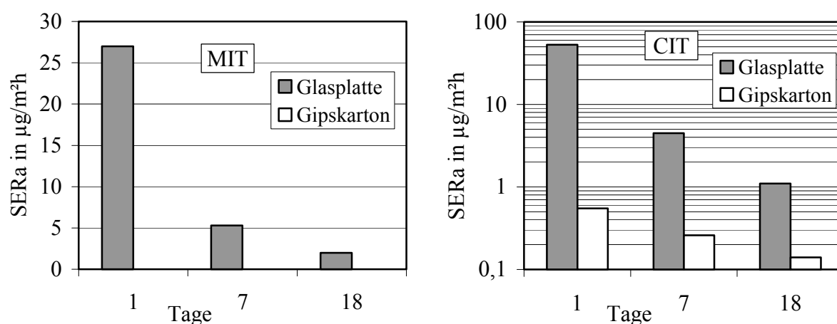
Abbildung 10. MIT- und CIT- SER_a von Farbe 8, aufgetragen auf Glasplatte und GK-Platte, bestimmt im "Weißen Elefanten".
