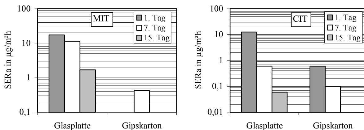
Abbildung 11. MIT- und CIT-SER a von Farbe 13, aufgetragen auf Glasplatte und GK-Platte, bestimmt in der FLEC.
