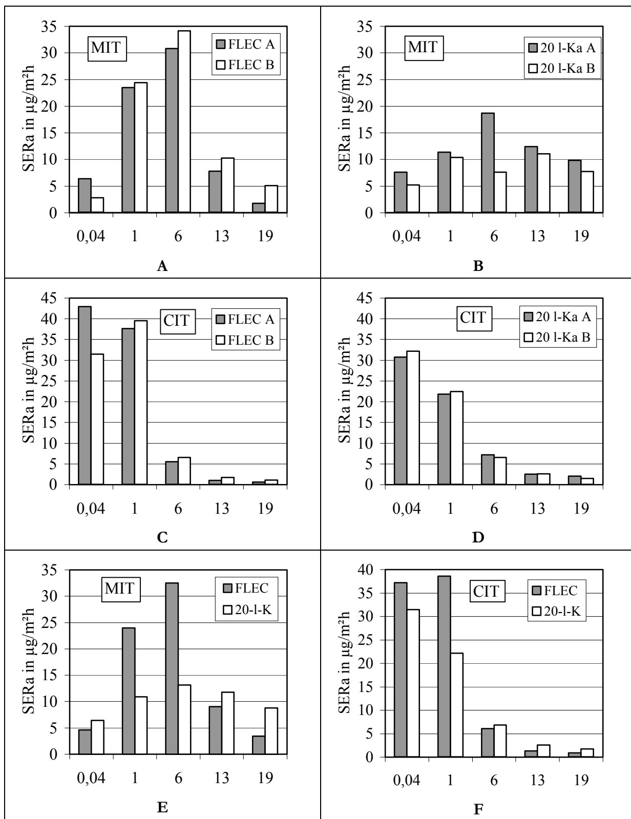
Abbildung A-1: CIT- und MIT- Emissionsraten in \text{g}/\text{m}^2\text{h} nach Tagen: Vergleich der verschiedenen Kammertypen und Reproduzierbarkeit der Messungen mit Farbe 4 (300 Tage nach Gebindeöffnung).
