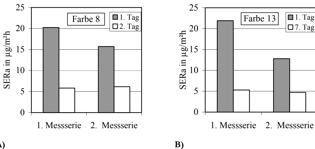
Abbildung 20: Einfluss der Lagerung auf die Emission von Formaldehyd.
