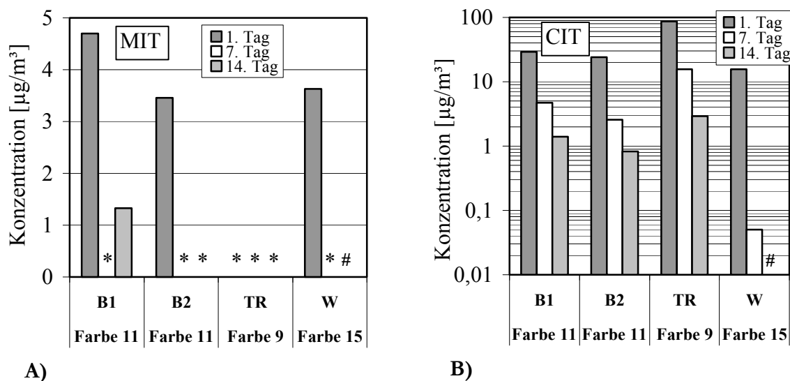
Abbildung 7. MIT- und CIT-Konzentrationen in verschiedenen Räumen 1, 7 und 14 Tage nach dem Streichen.
