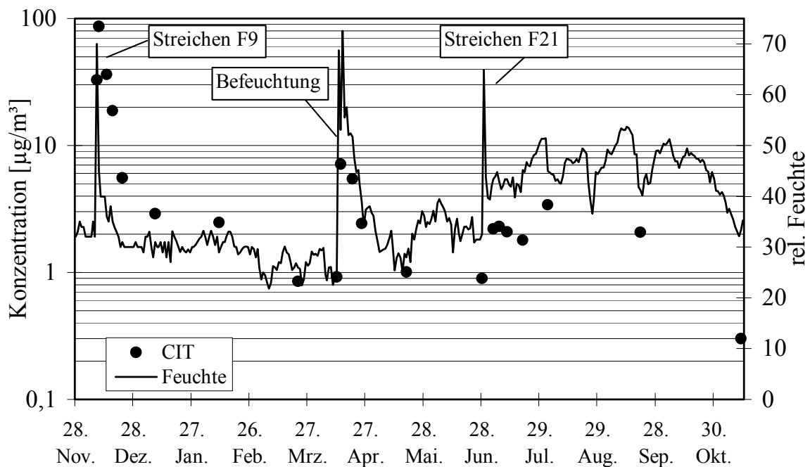
Abbildung 9. CIT-Konzentrationen im Raum eines Testhauses nach Ausbringen der Farbe 9. Einfluss der künstlichen Feuchteänderung nach 5 Monaten, Einfluss des Ausbringens einer zweiten biozidfreien Farbe (Farbe 21) und der erhöhten natürlichen Feuchte und Temperatur in der Sommerperiode.
