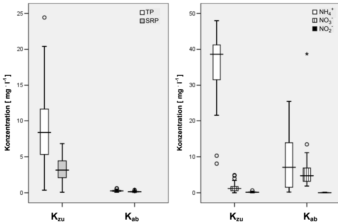
Abbildung 3: Zulauf- und Ablaufkonzentrationen der Kläranlage Leipzig-Rosental für TP, SRP, \text{NH}_4^+ , \text{NO}_3^- , \text{NO}_2^- (September 2002 bis Dezember 2004). Der Boxplot besteht aus Median, 25 bzw. 75 % Perzentile und dem kleinsten bzw. größten Wert (ohne Ausreißer) der Verteilung. Extremwerte sind mit einem Stern bzw. Kreis dargestellt.
